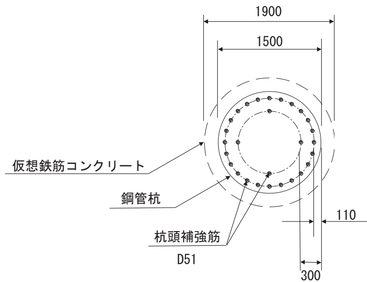
図 3-42 仮想鉄筋コンクリート断面概念図
