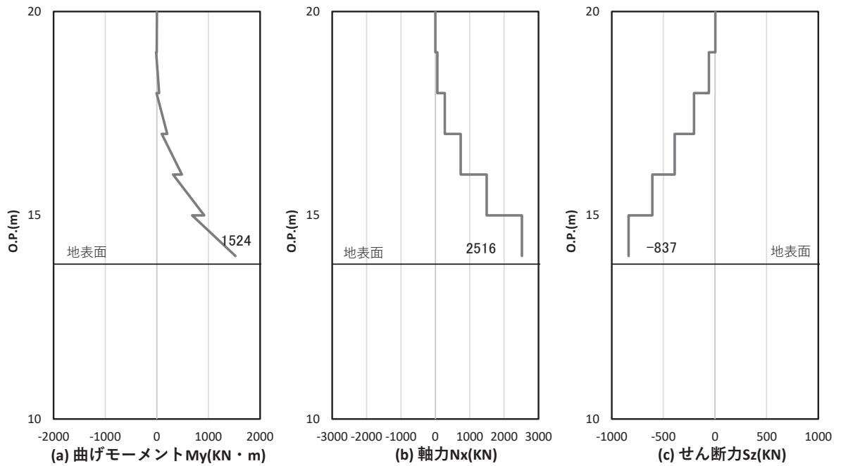
図 5-9(1) 鋼製支柱の曲げ・軸力系の破壊に対する照査における照査時刻での断面力 (断面①, S d - D 2 (++) , t = 25.55\text{s} )
