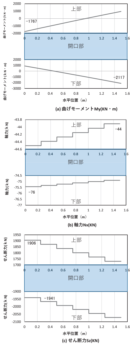
図 5-25(1) コンクリート及び鉄筋の曲げ・軸力系の破壊に対する照査における 最大曲げモーメント発生時刻での断面力 (断面⑦開口部, S_d - D2 (-+) , t = 6.93s , M_y 最大) 解析ケース③: 地盤物性のばらつき ( -1\sigma ) を考慮した解析ケース
