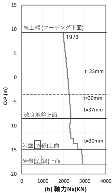
図 5-47 基礎地盤の支持性能照査時刻での軸力（押し込み時） (断面②, S d - D 2 (++) , t = 23.56s) 解析ケース②：地盤物性のばらつき (+1σ) を考慮した解析ケース
