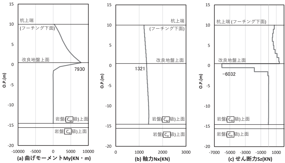
図 5-37 鋼管杭のせん断破壊に対する照査における照査時刻での断面力 (断面③, S d - D 2 (++) , t = 25.41s) 解析ケース② : 地盤物性のばらつき (+1σ) を考慮した解析ケース
