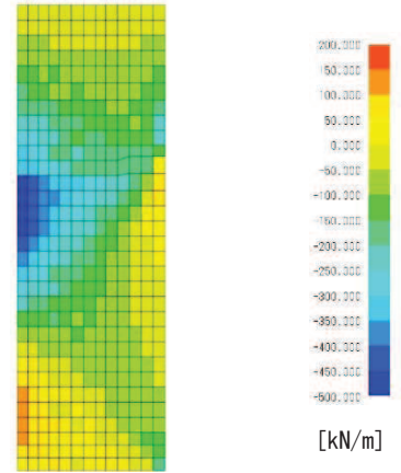
図 7-6(5) N_y 図
