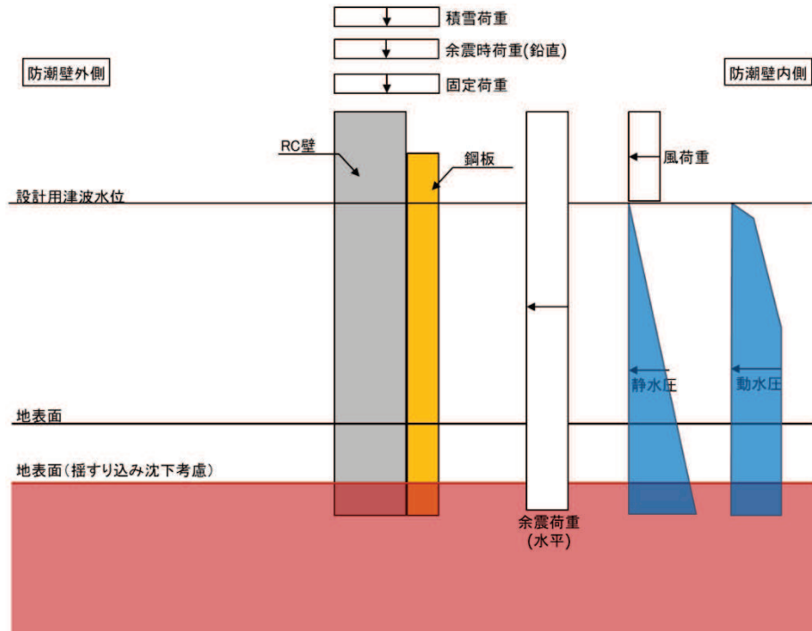
図 5-1 荷重の概念図 (防潮堤取り合い部)
