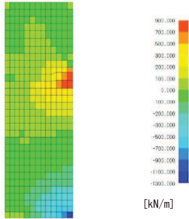
図 7-6(4) N_x 図
