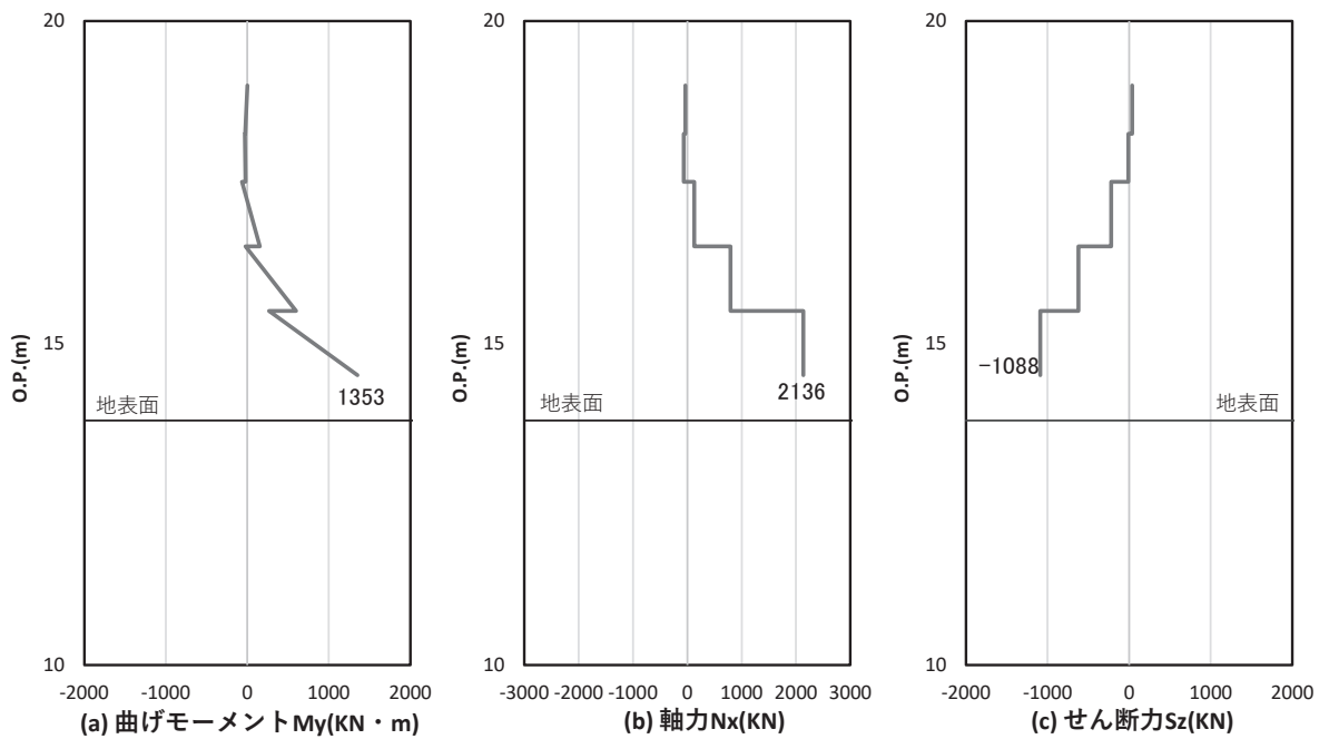
図 5-16(2) 鋼製支柱のせん断破壊に対する照査における照査時刻での断面力 (断面⑦張出部, S d - D 2 ( - + ), t = 6. 92s) 解析ケース①：基本ケース
