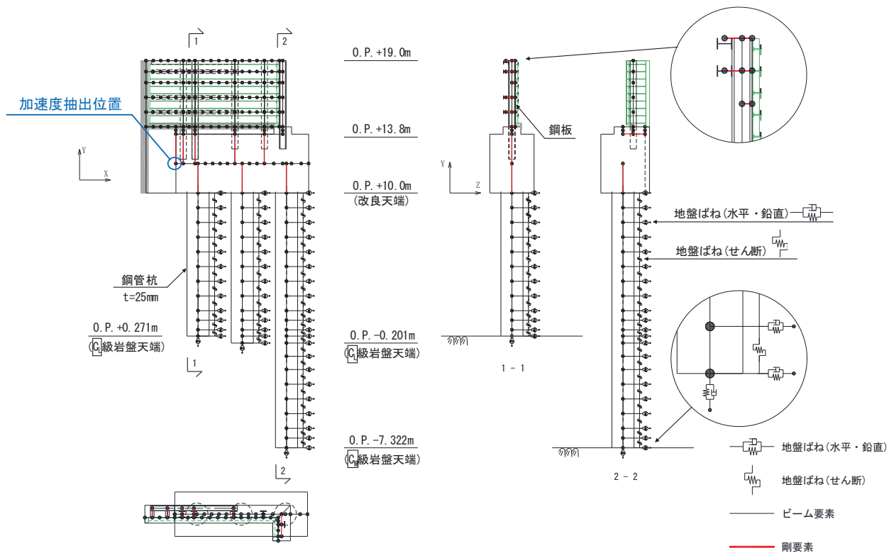
図 4-2 フーチング震度抽出モデル (鋼製遮水壁 (鋼板) 断面⑤)
