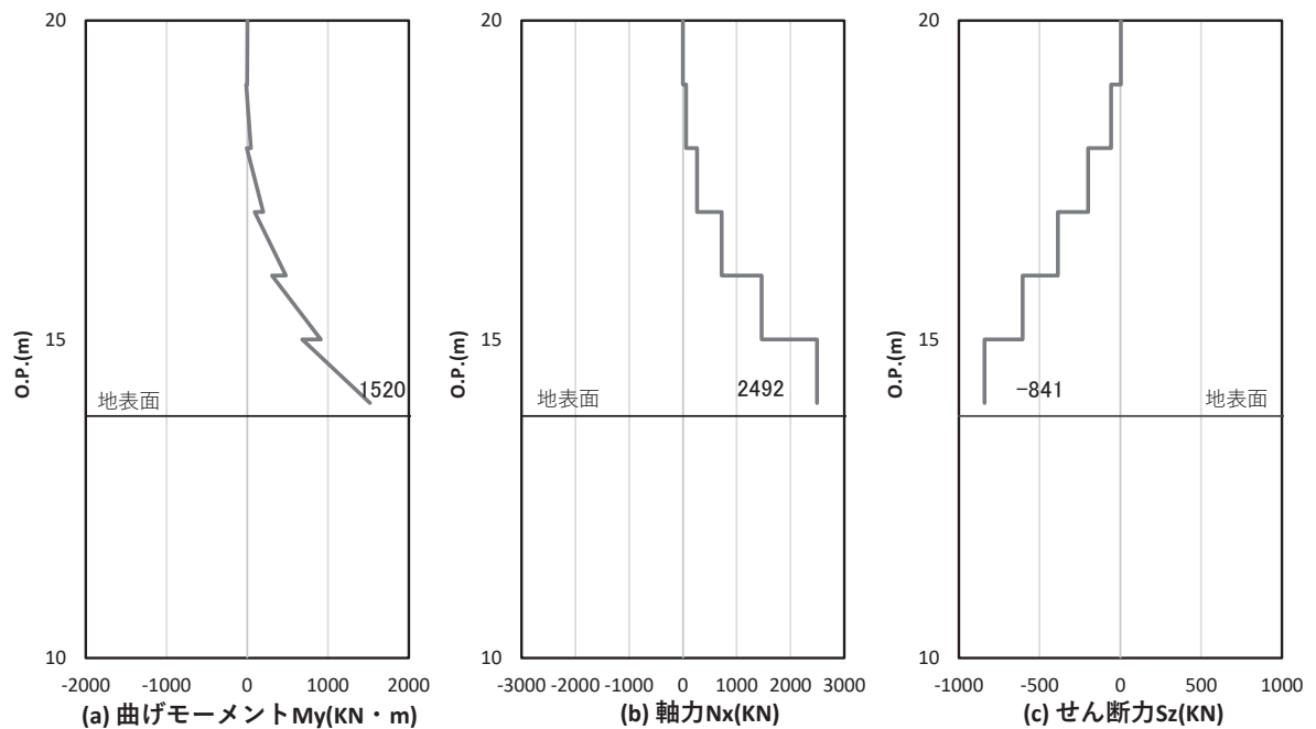
図 5-9(2) 鋼製支柱のせん断破壊に対する照査における照査時刻での断面力 (断面①, S d - D 2 (++) , t = 25.54\text{s} )
