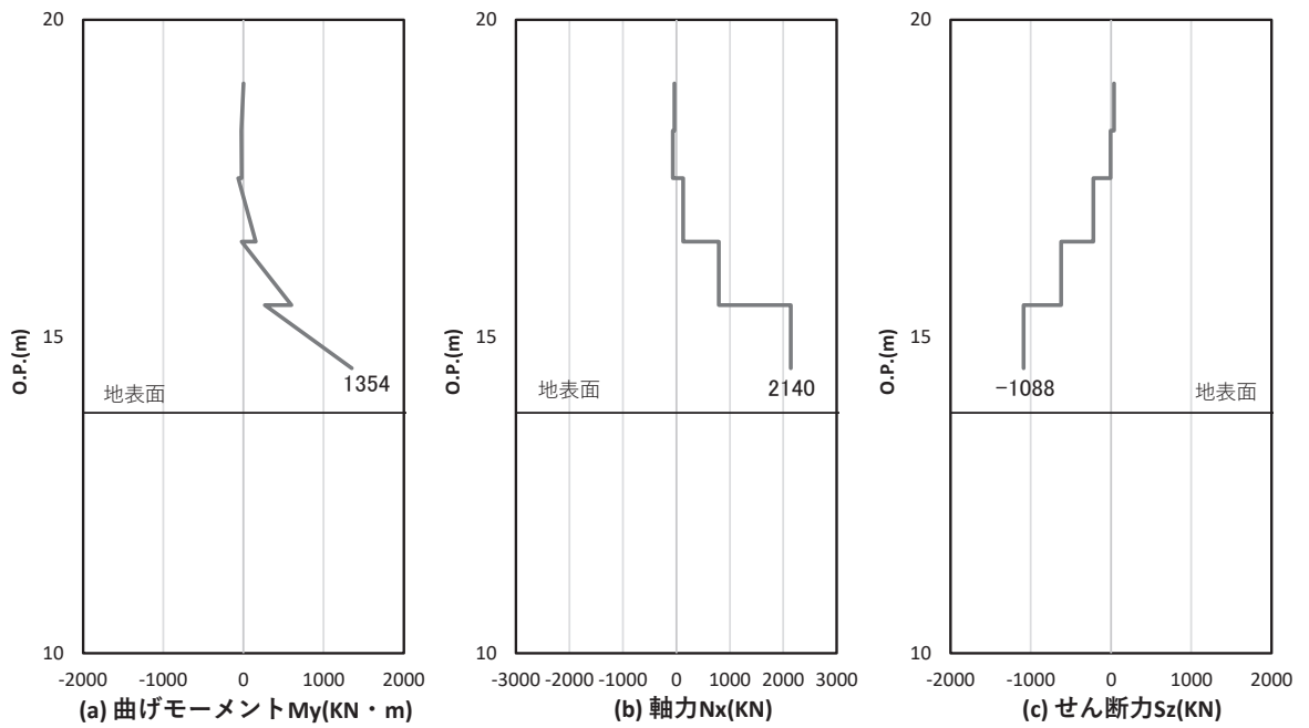
図 5-16(1) 鋼製支柱の曲げ・軸力系の破壊に対する照査における照査時刻での断面力 (断面⑦張出部, S d - D 2 ( - - ), t = 6. 92s) 解析ケース①：基本ケース
