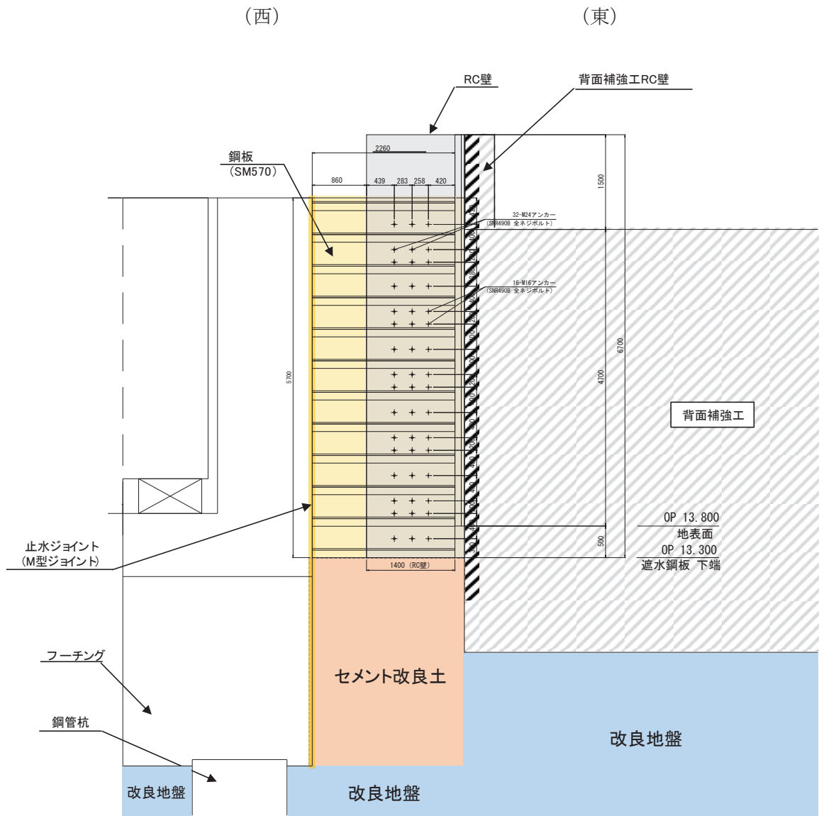
図1-10(1) 防潮堤取り合い部下部の止水対策の概要 (防潮堤取り合い部①)
