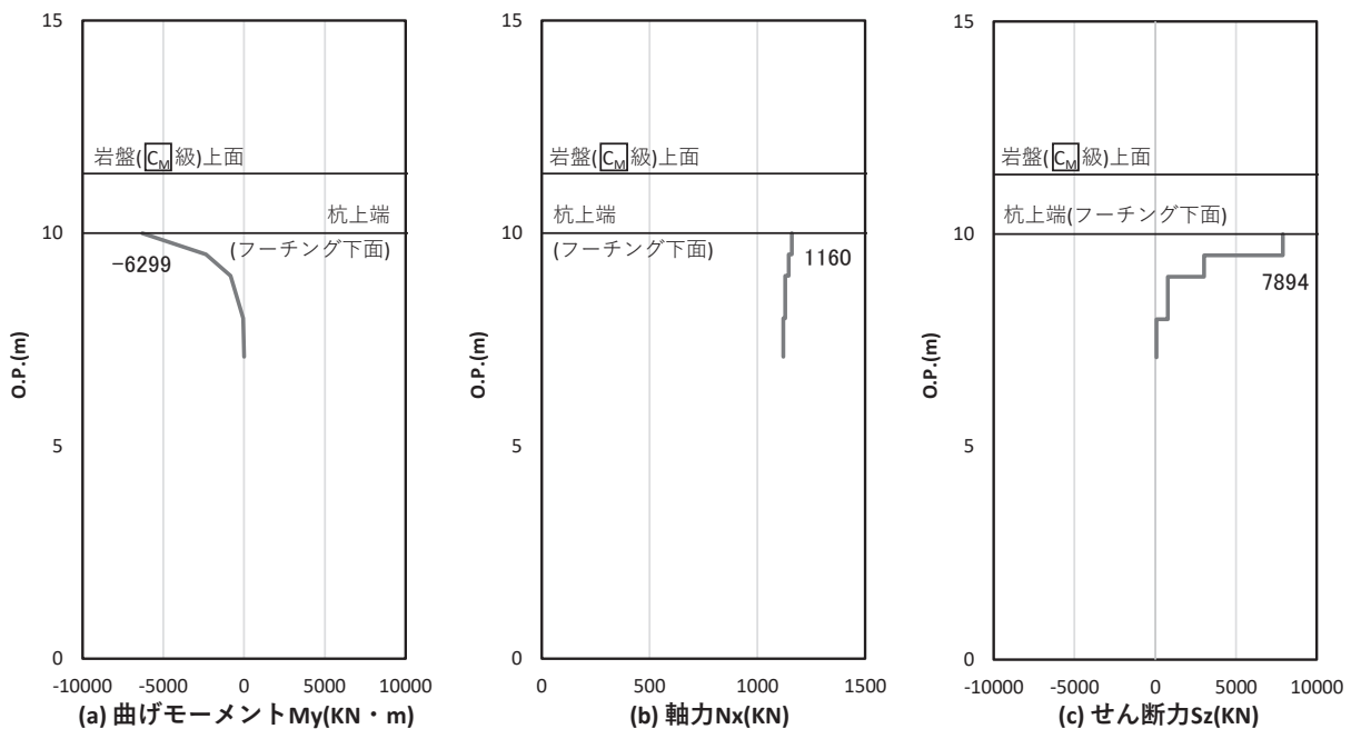
図 5-40 鋼管杭のせん断破壊に対する照査における照査時刻での断面力 (断面⑥, S d - D 2 ( - + ) , t = 8.55s)
