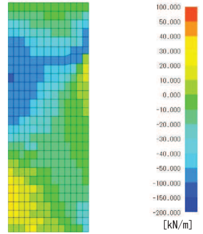
図 7-1 (5) N_y 図
