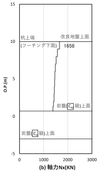
図 5-52 基礎地盤の支持性能照査時刻での軸力（押し込み時） （断面⑦， S d - D 2 （ +- ） ， t = 11.43s） 解析ケース③：地盤物性のばらつき（ -1\sigma ）を考慮した解析ケース
