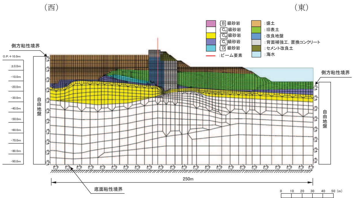
図 5-6(2) 解析モデル (防潮堤 (鋼管式鉛直壁) 断面②)
