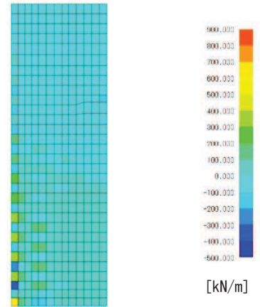
図 7-6(7) Q_y 図
