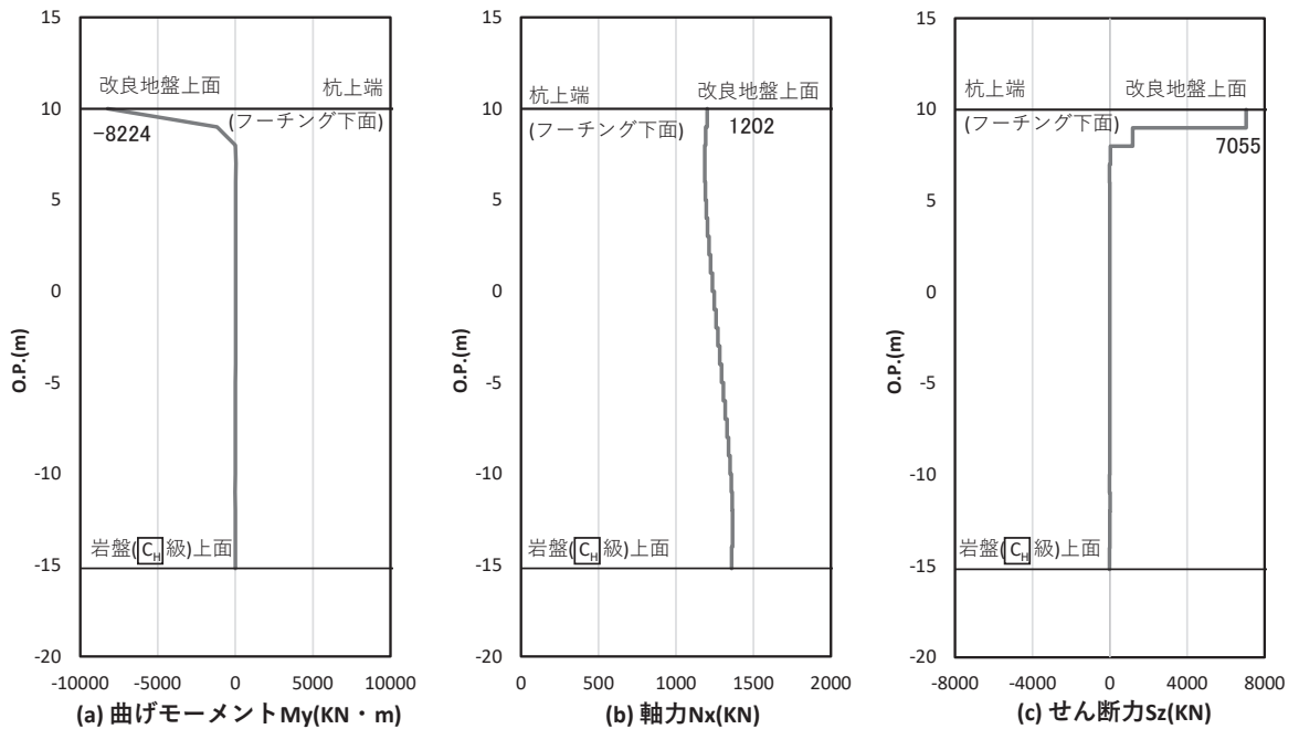
図 5-38 鋼管杭のせん断破壊に対する照査における照査時刻での断面力 (断面④, S d - D 2 (+-) , t = 25.07s) 解析ケース② : 地盤物性のばらつき (+1σ) を考慮した解析ケース
