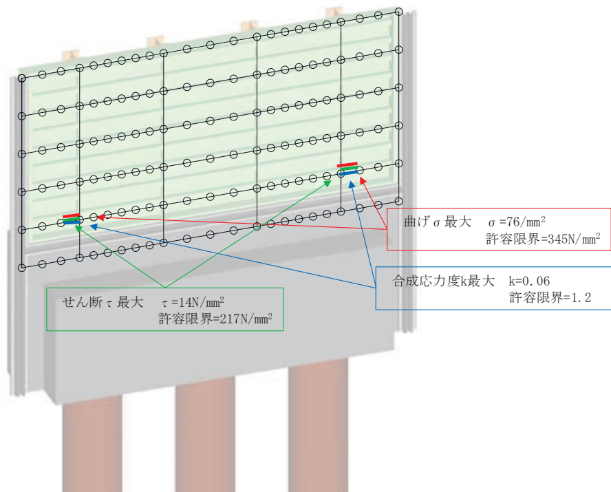
図 5-8 鋼板の曲げ・軸力系の破壊及びせん断破壊に対する最大照査値発生箇所 (断面⑧)
