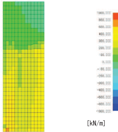
図 7-6(6) Q_x 図
