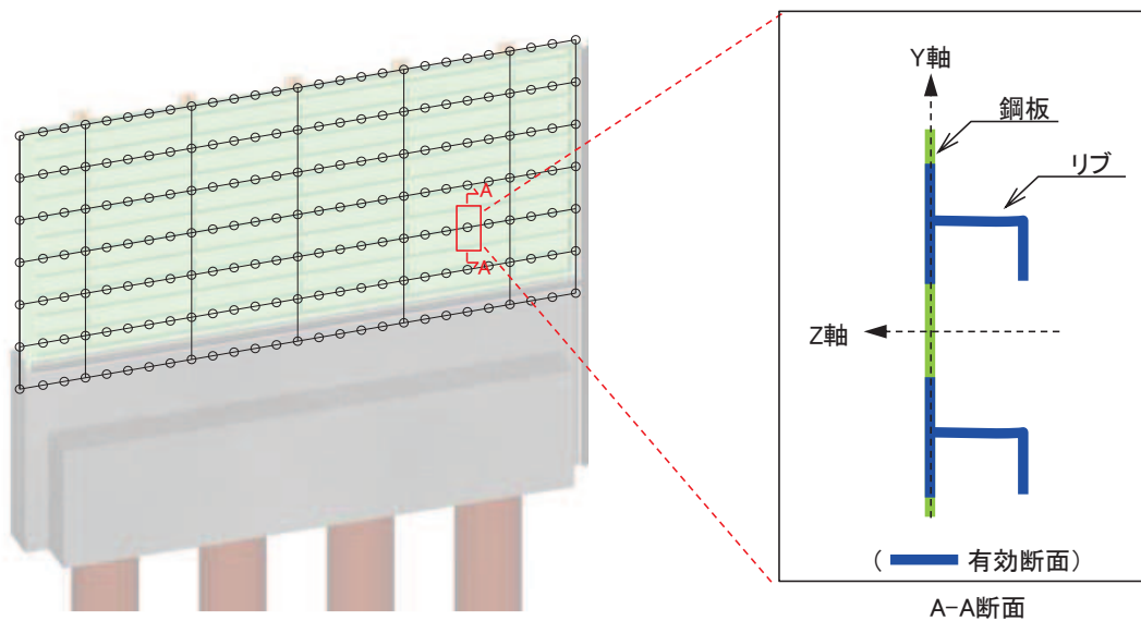
図 3-37 鋼製パネル断面形状
