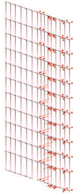
図 7-3(2) 反力図 (1.0Sd 水平_0.4Sd 鉛直)
