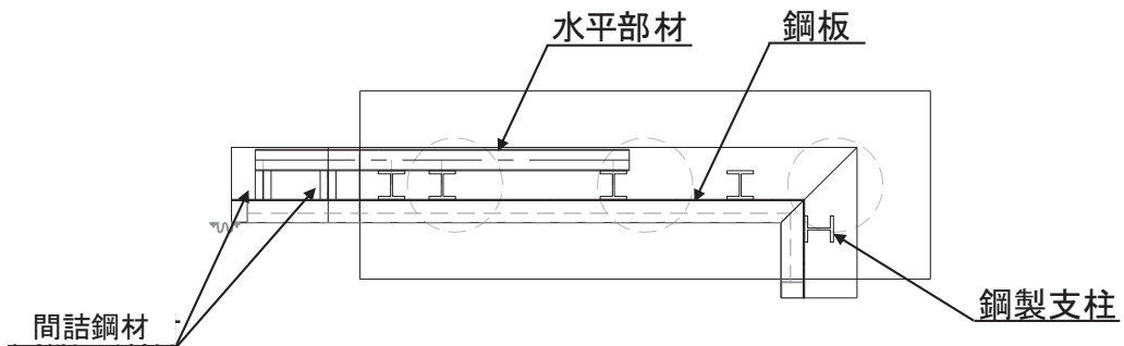
図 3-17 水平部材，間詰鋼材（断面⑤の例）
