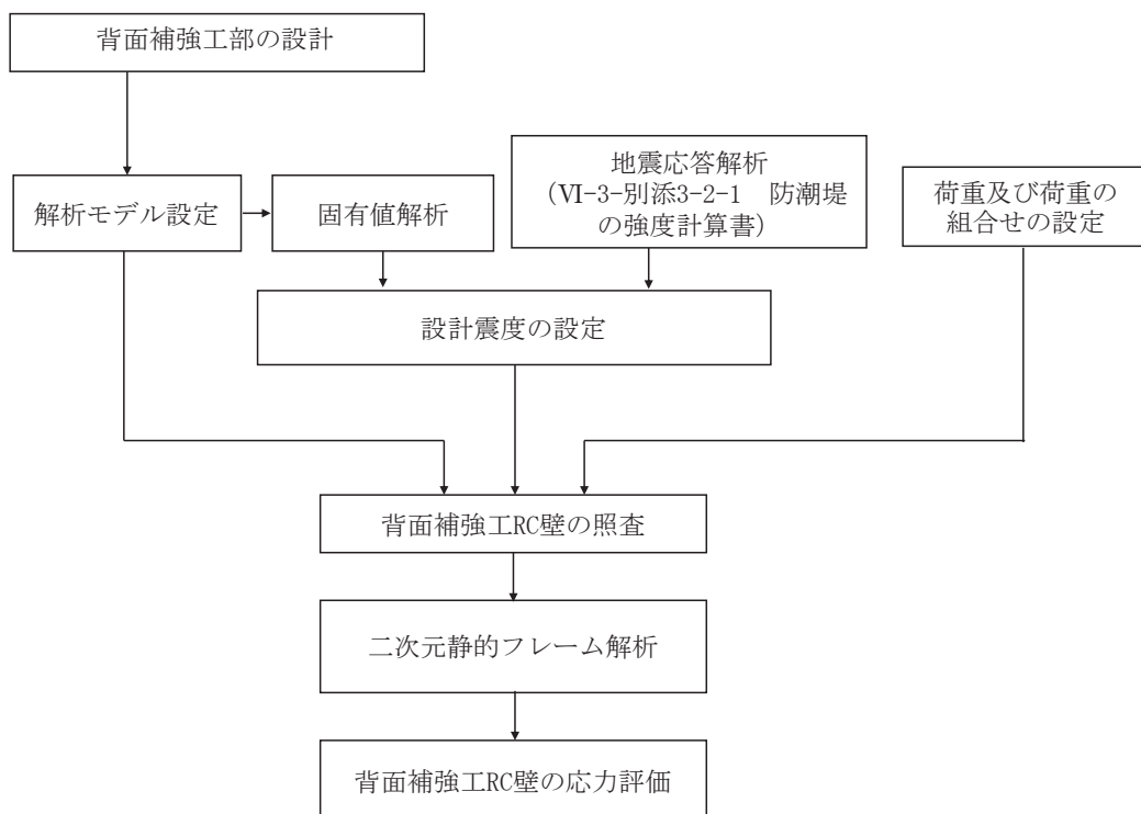
図 2-2 背面補強工部の評価フロー
