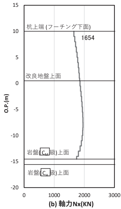
図 5-48 基礎地盤の支持性能照査時刻での軸力（押し込み時） （断面③，S d - D 2（--），t = 11.44s） 解析ケース③：地盤物性のばらつき（ -1\sigma ）を考慮した解析ケース
