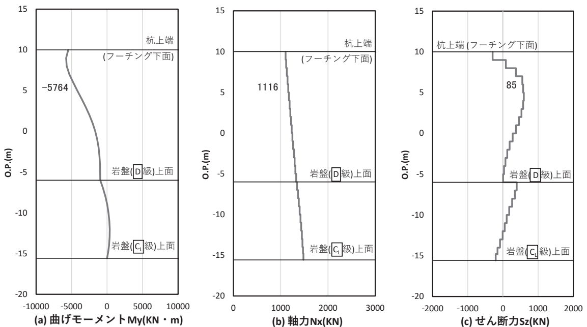
図 5-34 鋼管杭の曲げ・軸力系の破壊に対する照査における照査時刻での断面力 (断面⑧, S d - D 2 (-+), t = 13.37s) 解析ケース①: 基本ケース
