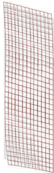
7次モード f_7=242.106 Hz
