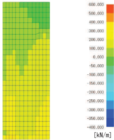
図 7-2(6) Q_x 図
