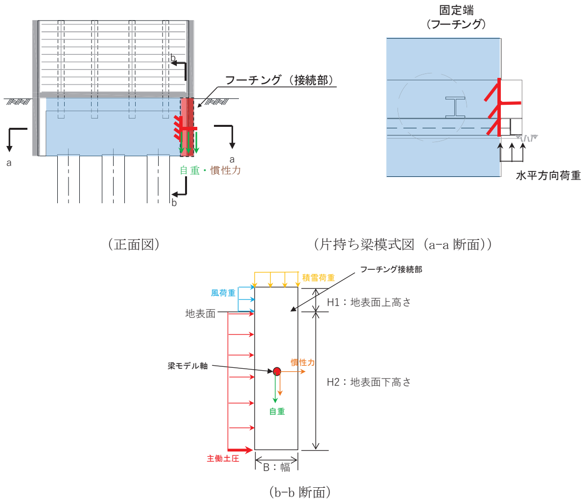
図 3-41 フーチング（接続部）評価用モデル概念図
