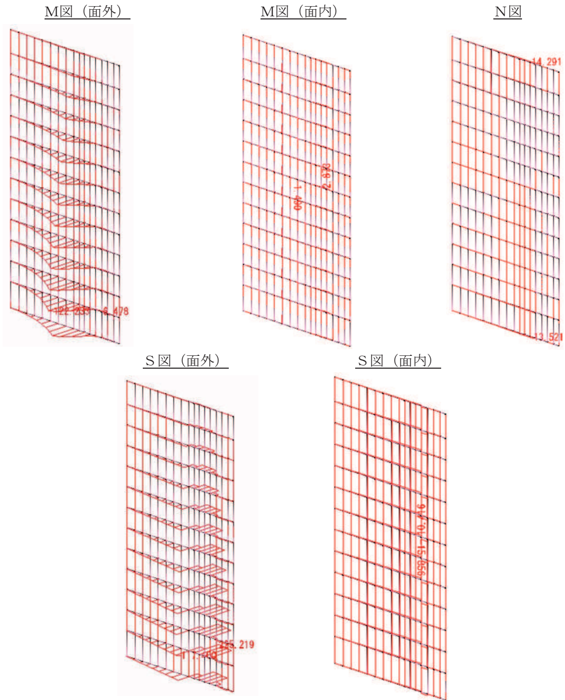
図7-7(1) 断面力図 (1.0Sd 水平_0.4Sd 鉛直)
