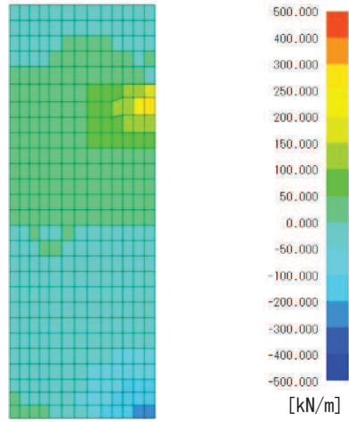
図 7-1 (4) N_x 図
