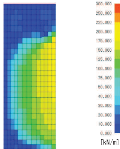
図 7-2(8) N_{xy} 図
