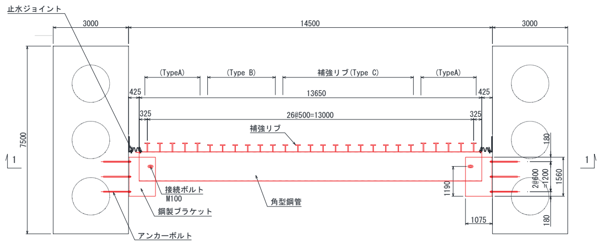
(平面図(2-2 断面))
