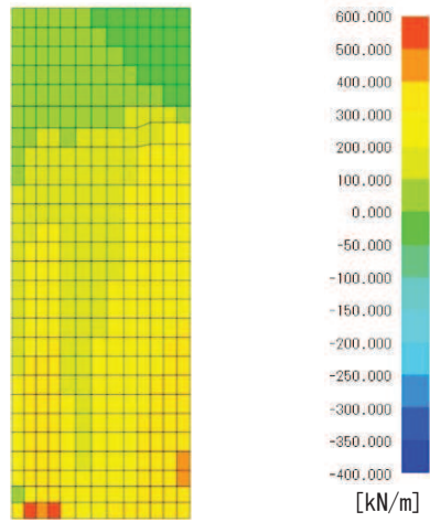
図 7-1 (6) Q_x 図
