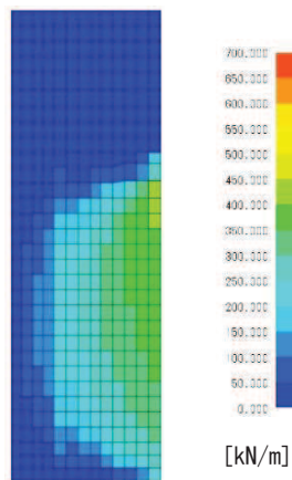
図 7-5(8) N_{xy}
