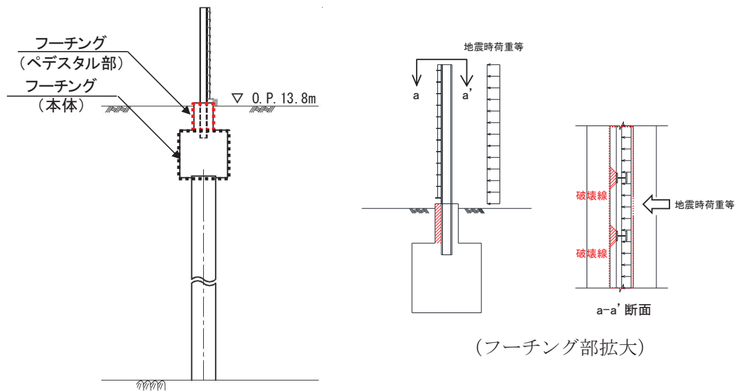
図 3-40 フーチング (ペDESTAL部) に作用する荷重概念図
