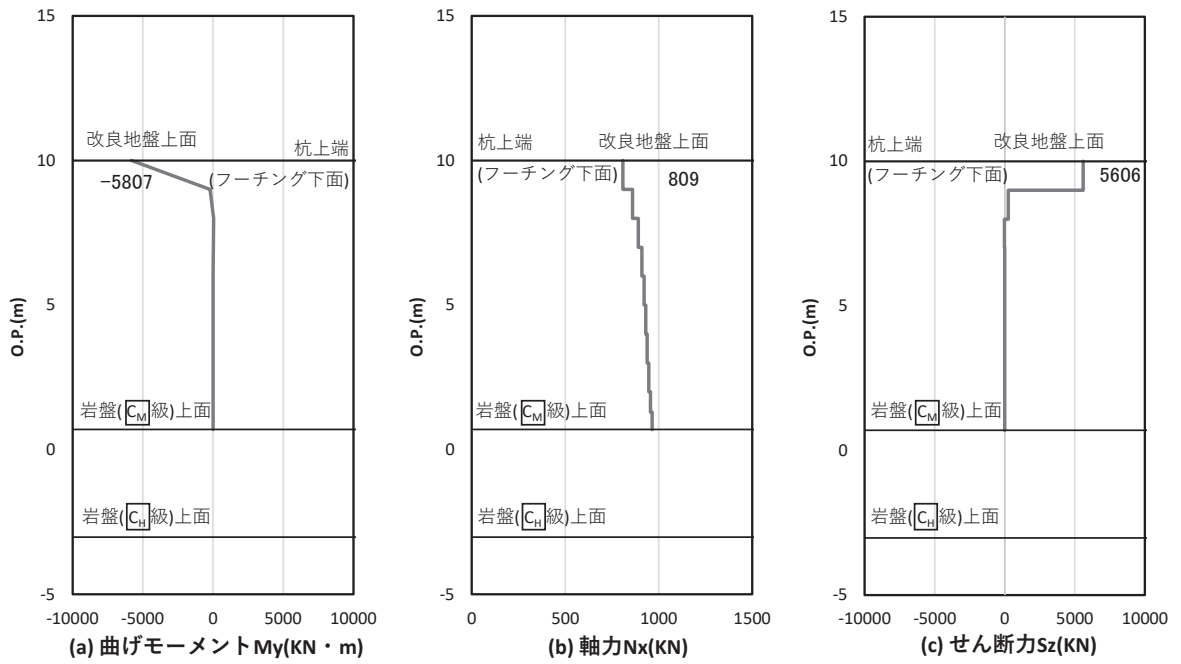
図 5-41 鋼管杭のせん断破壊に対する照査における照査時刻での断面力 (断面⑦, S d - D 2 (++) , t = 29.96s)
