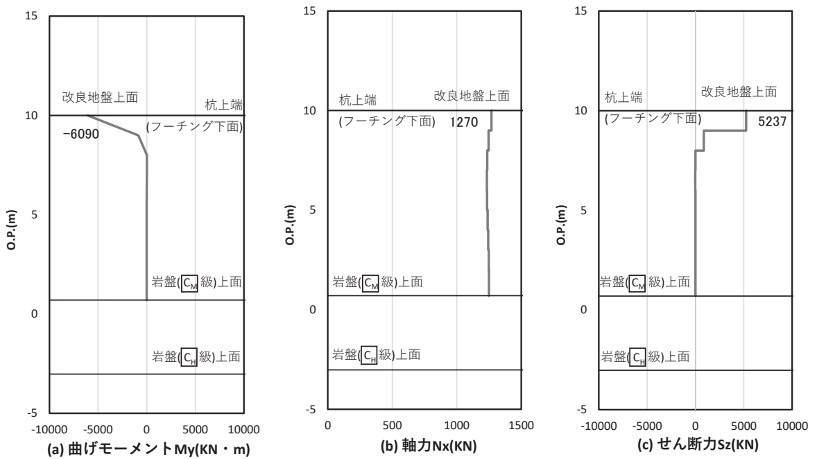
図 5-33 鋼管杭の曲げ・軸力系の破壊に対する照査における照査時刻での断面力 (断面⑦, S d - D 2 (++) , t = 6.84s) 解析ケース①: 基本ケース
