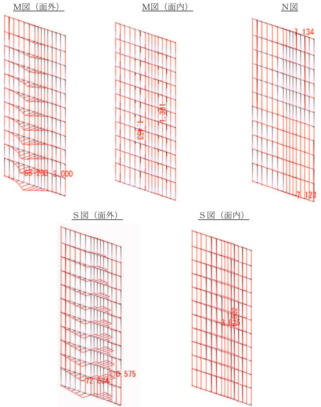
図7-3(1) 断面力図 (1.0Sd 水平_-0.4Sd 鉛直)
