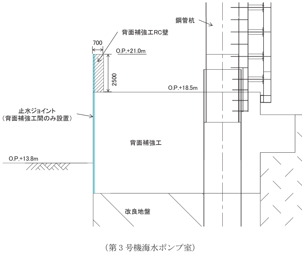
図1-11 背面補強工部の構造概要図 (断面図)
