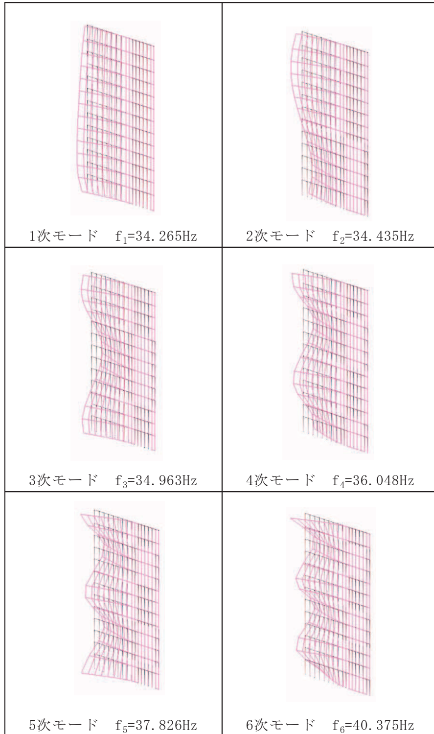
図4-7(1) 固有値解析結果 (モード図) (防潮堤取り合い部④)
