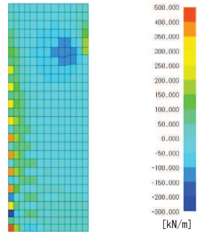
図 7-1 (7) Q_y 図
