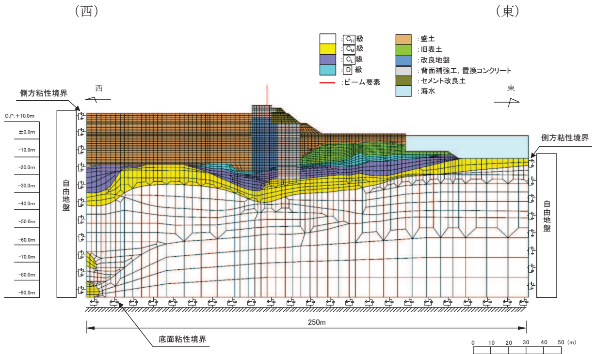
図 5-6(1) 解析モデル (防潮堤 (鋼管式鉛直壁) 断面①)
