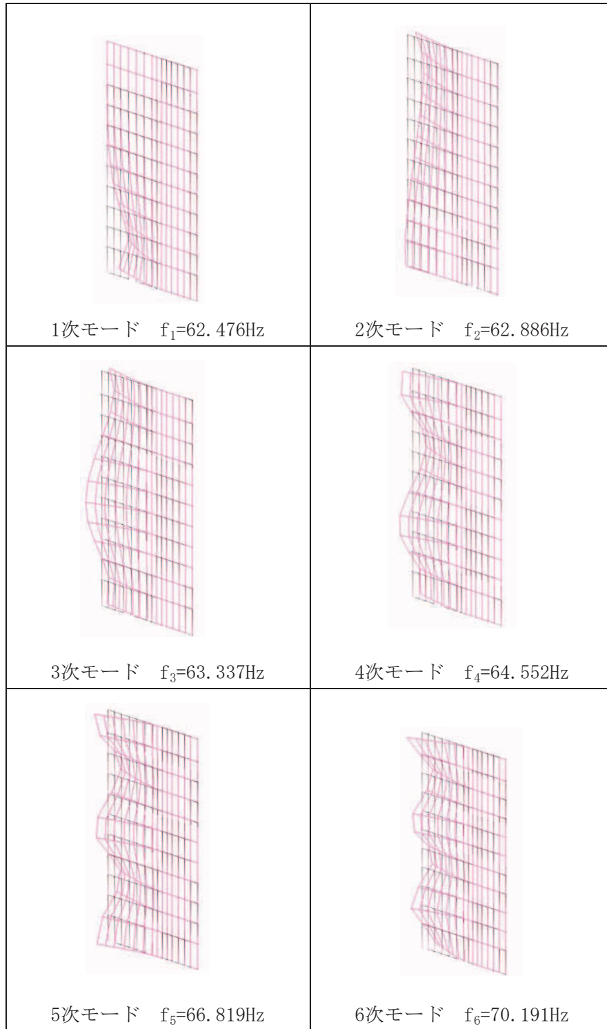
図4-6(1) 固有値解析結果 (モード図) (防潮堤取り合い部②)
