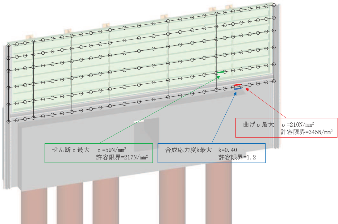
図 5-7(2) 鋼板の曲げ・軸力系の破壊及びせん断破壊に対する最大照査値発生箇所 (断面⑦張出部)
