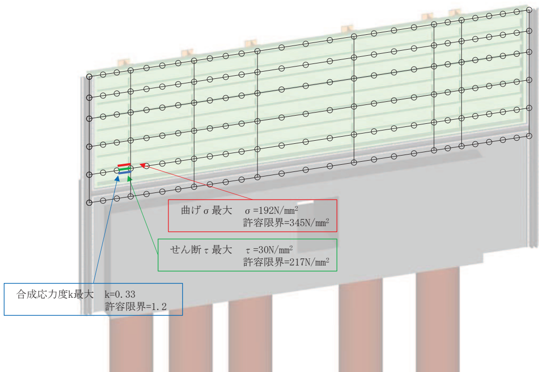
図 5-7(1) 鋼板の曲げ・軸力系の破壊及びせん断破壊に対する 最大照査値発生箇所（断面⑦一般部）
