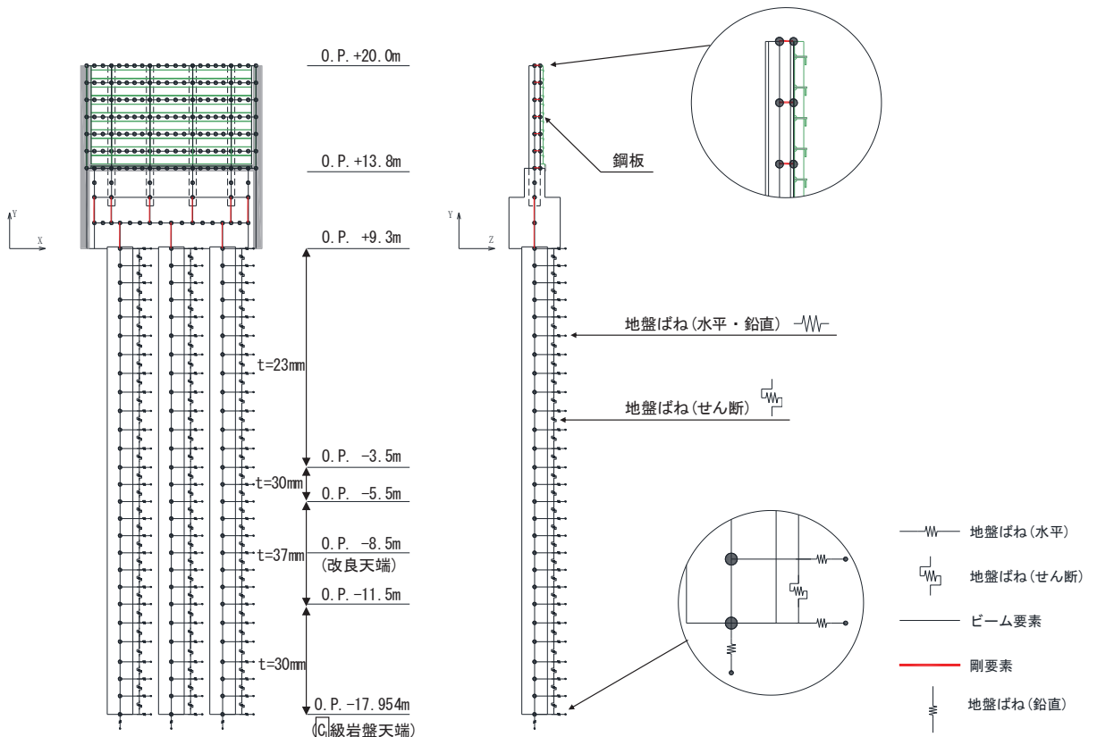
図 3-33 静的解析モデル（断面②の例）
