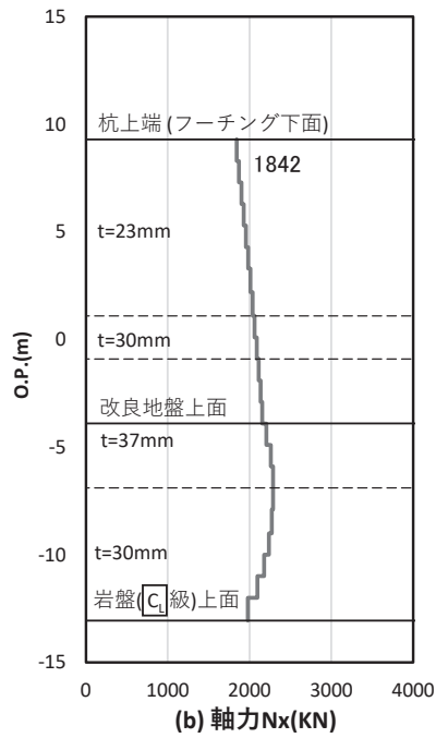
図 5-46 基礎地盤の支持性能照査時刻での軸力（押し込み時） (断面①, S d - D 2 (++) , t = 23.56s) 解析ケース③：地盤物性のばらつき (-1σ) を考慮した解析ケース
