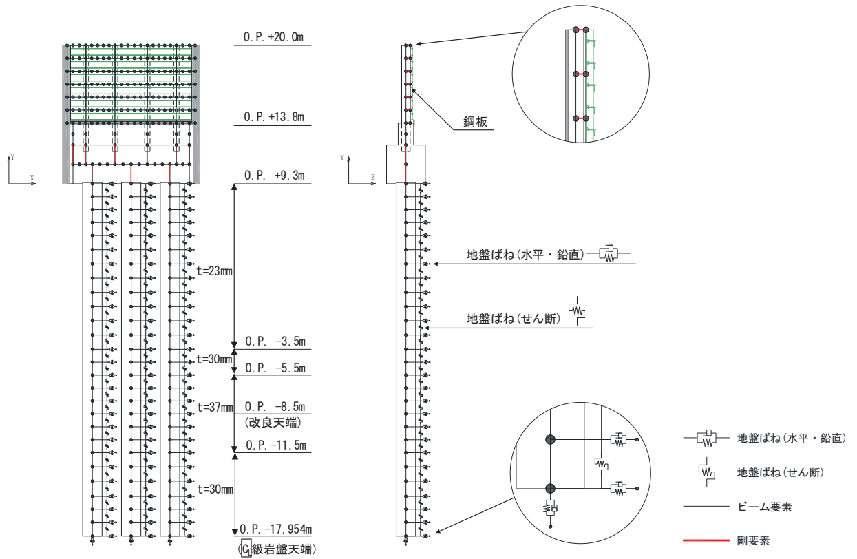
図 3-34 固有値解析モデル (断面②の例)
