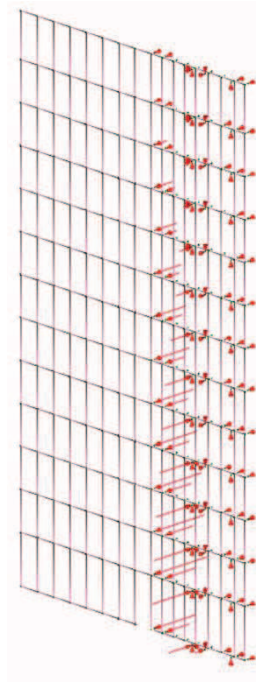
図 7-7(2) 反力图 (1.0Sd 水平_0.4Sd 鉛直)
