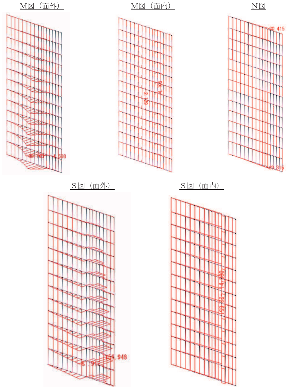
图 7-8(1) 断面力图 (0.4Sd 水平_1.0Sd 鉛直 ok)
