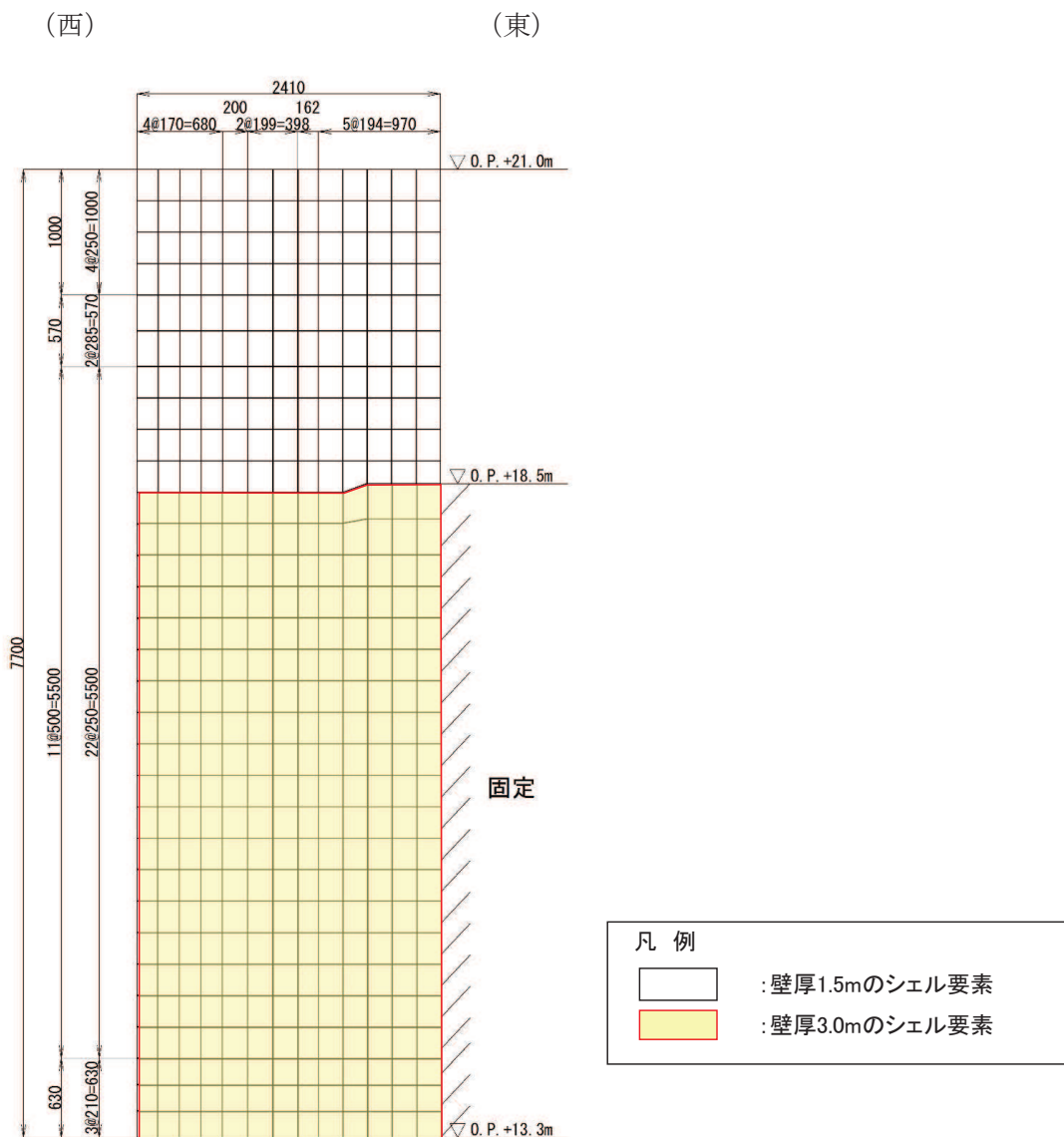
図 4-1 固有値解析モデル (RC 壁) (防潮堤取り合い部④の例)
