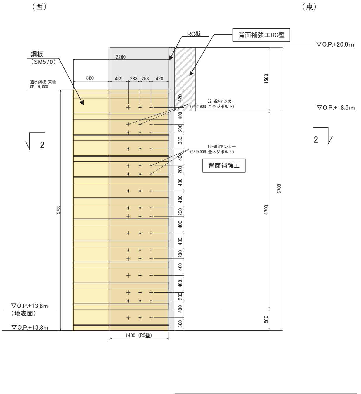
(正面図：1-1 断面)
