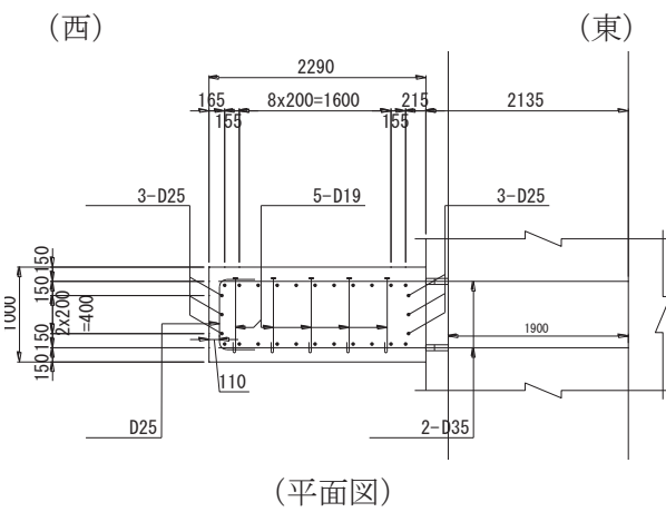
図 1-7 RC 壁の配筋概要図 (防潮堤取り合い部②)
