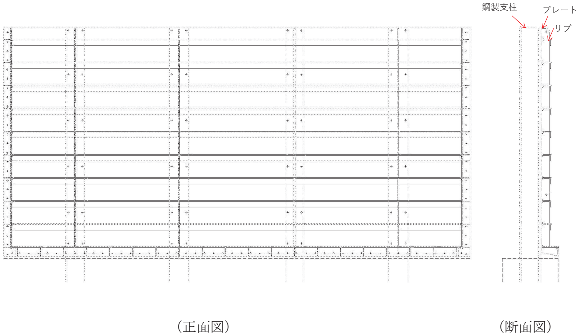
図 3-36 鋼板の構造図（正面図，断面図）
