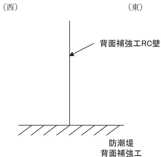
図 4-8 固有値解析モデル（背面補強工 RC 壁（第 2 号・第 3 号機海水ポンプ室）共通）
