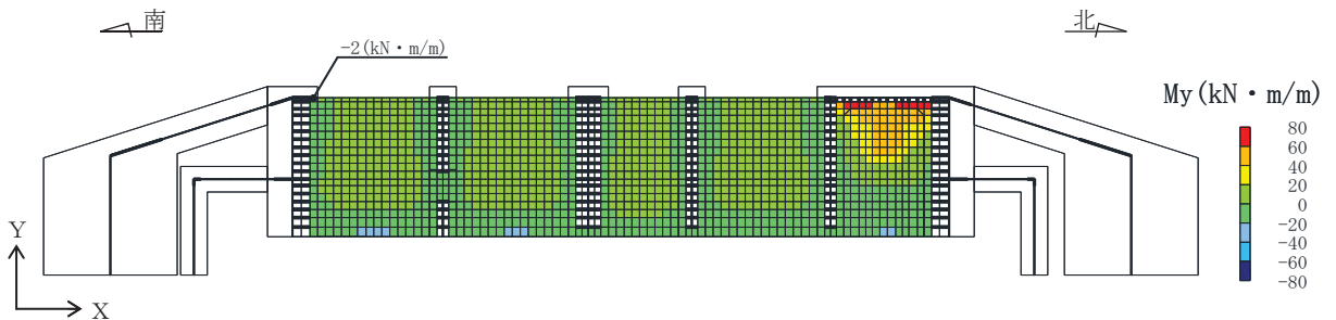
図4-28 曲げ・軸力系の破壊に対する照査値最大時の断面力分布図 (曲げモーメント (kN・m/m) : M_y ) (底版, 解析ケース③, S_s - F 2 (++) )
