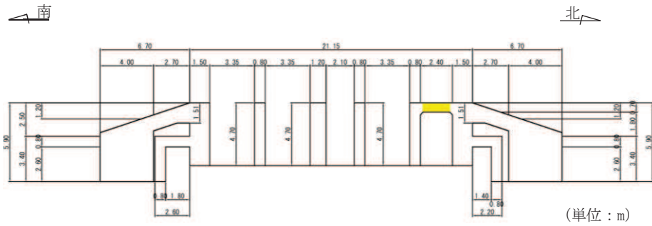
図2-11 Ccbによる耐震補強箇所(断面②)
