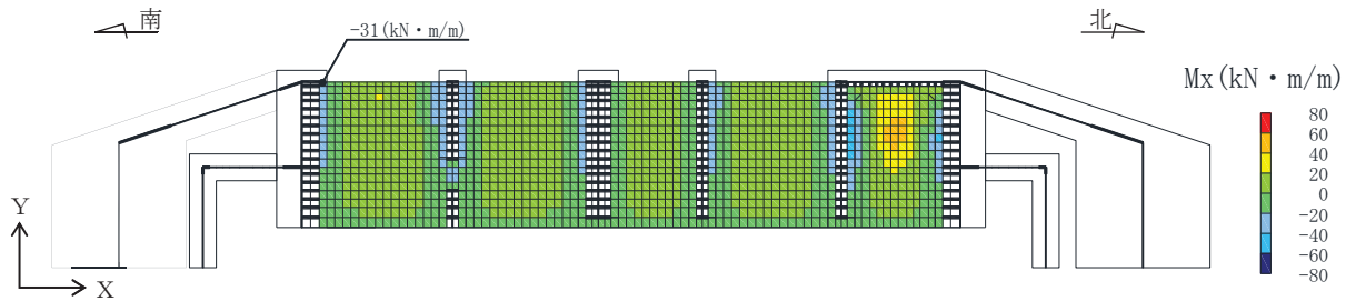
図4-27 曲げ・軸力系の破壊に対する照査値最大時の断面力分布図 (曲げモーメント (kN・m/m) : M_x ) (底版, 解析ケース③, S_s - F 2 (++) )
