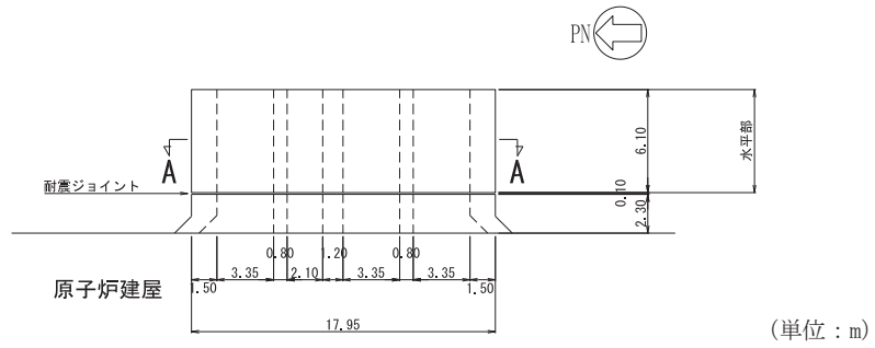
図3-1 原子炉機器冷却海水配管ダクト（水平部）の評価対象断面位置図
