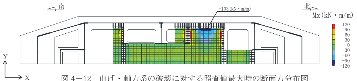
図4-12 曲げ・軸力系の破壊に対する照査値最大時の断面力分布図
