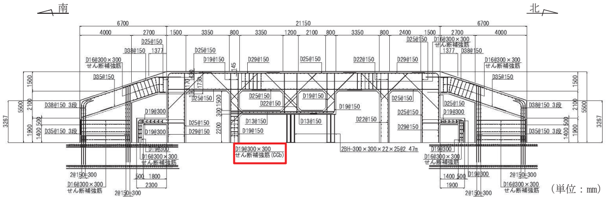
図 2-14 原子炉機器冷却海水配管ダクト（鉛直部）概略配筋図（断面②）
