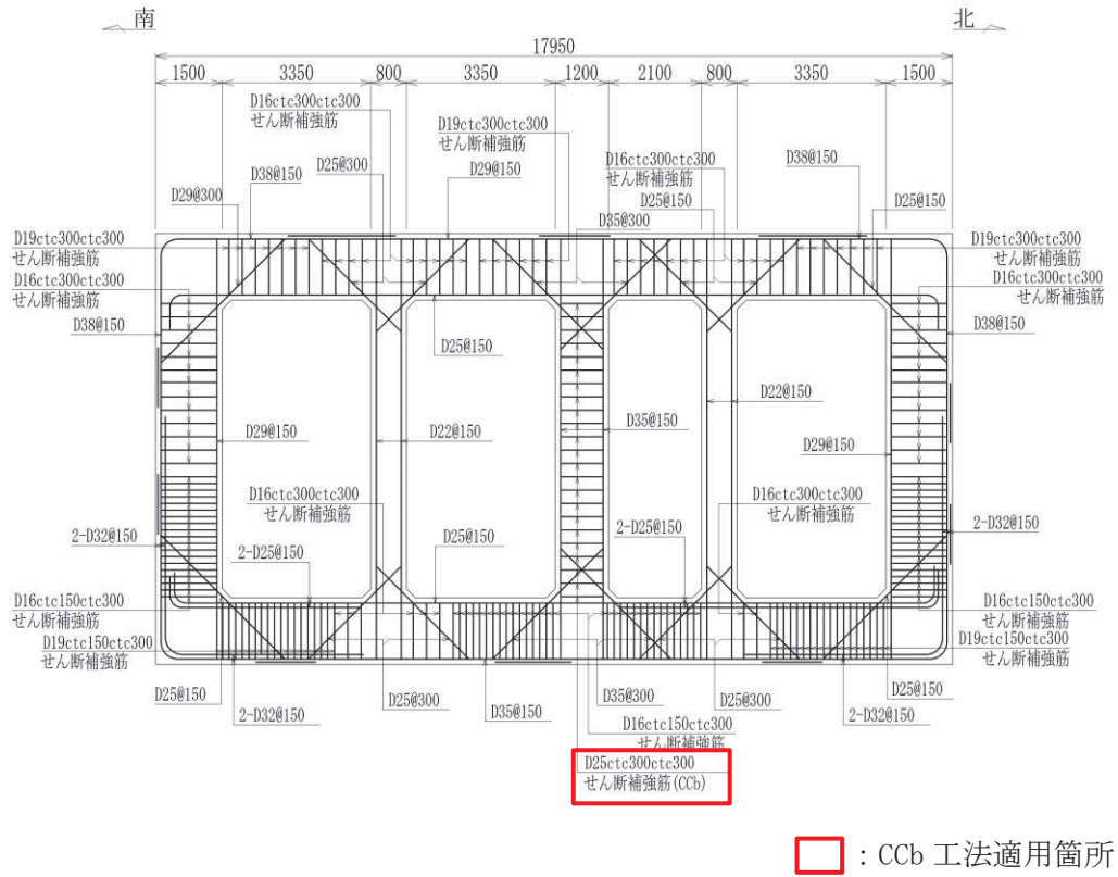
図 2-5 原子炉機器冷却海水配管ダクト（水平部）概略配筋図
