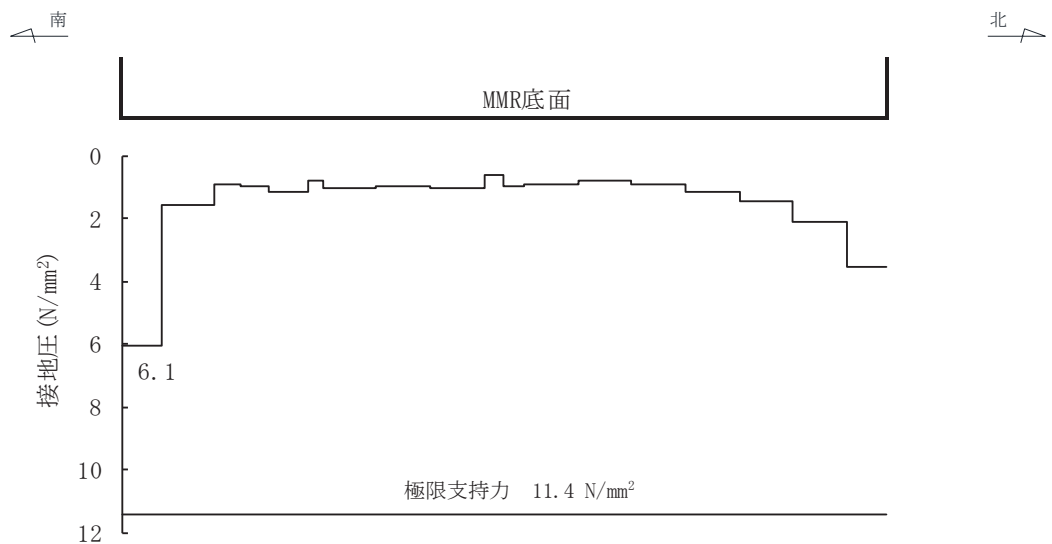
図 5-11 基礎地盤の最大接地圧分布図
