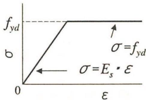
図 3-6 構造部材の非線形特性 (鉄筋の応力-ひずみ関係) (土木学会 2002 年 コンクリート標準示方書[構造性能照査編]より引用)
