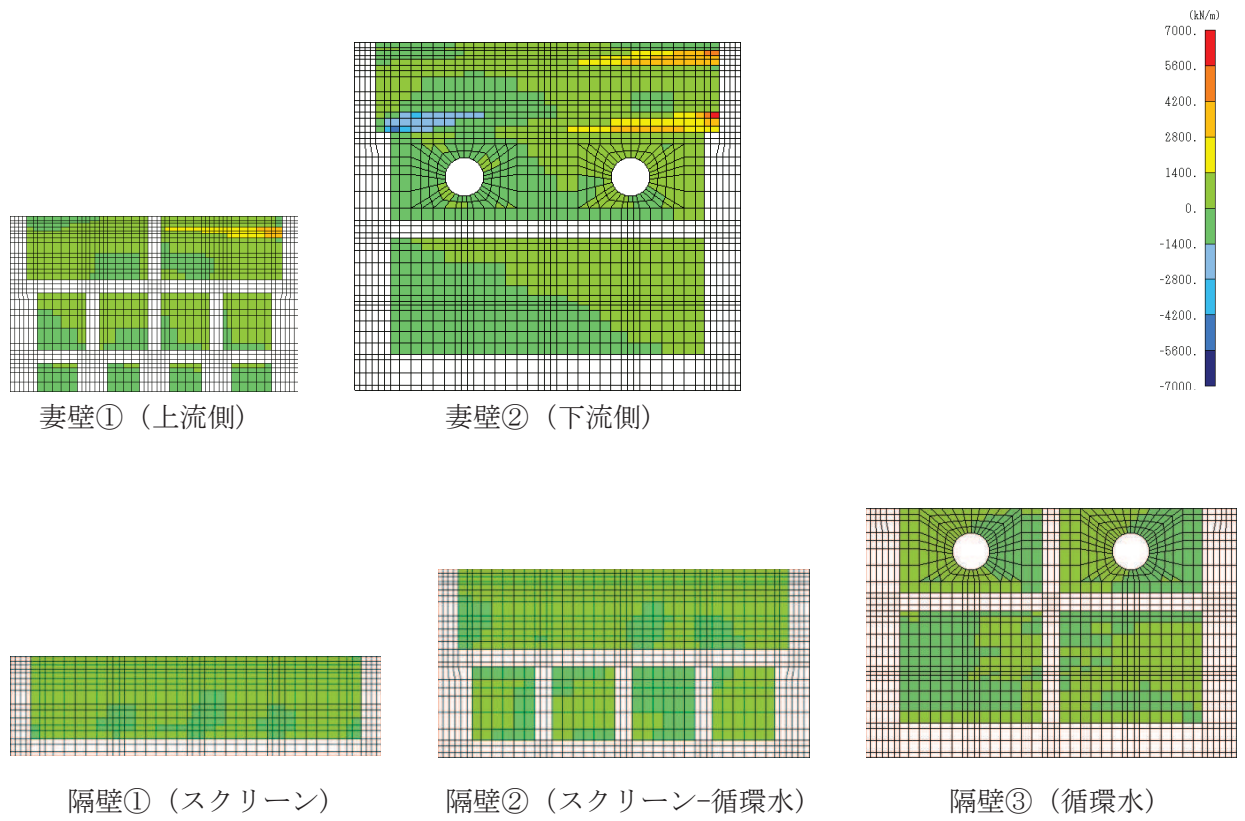
図 4-21(2) せん断破壊に対する照査値最大時の断面力分布図 (せん断力 (kN/m) : Q_x ) (導流壁②, 解析ケース⑥, S_s - D 2 (++) )
