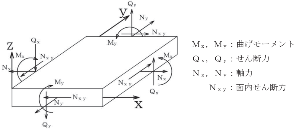
図4-7 シェル要素の各要素における断面力方向
