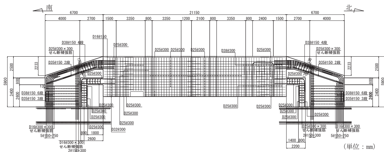
図 2-18 原子炉機器冷却海水配管ダクト（鉛直部）概略配筋図（断面⑥）
