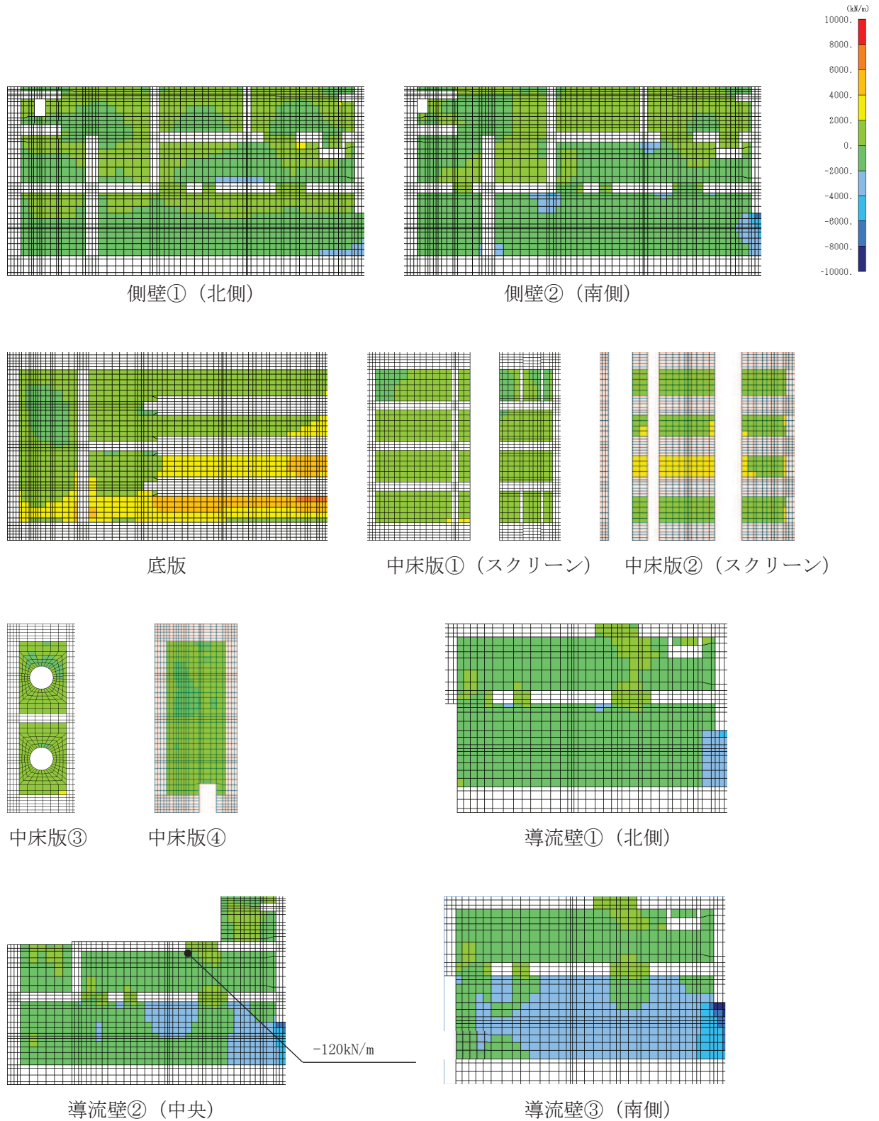
図 4-22(1) せん断破壊に対する照査値最大時の断面力分布図 (せん断力 (\text{kN/m}) : Q_y ) (導流壁②, 解析ケース⑥, S_s - D 2 (+ +) )
