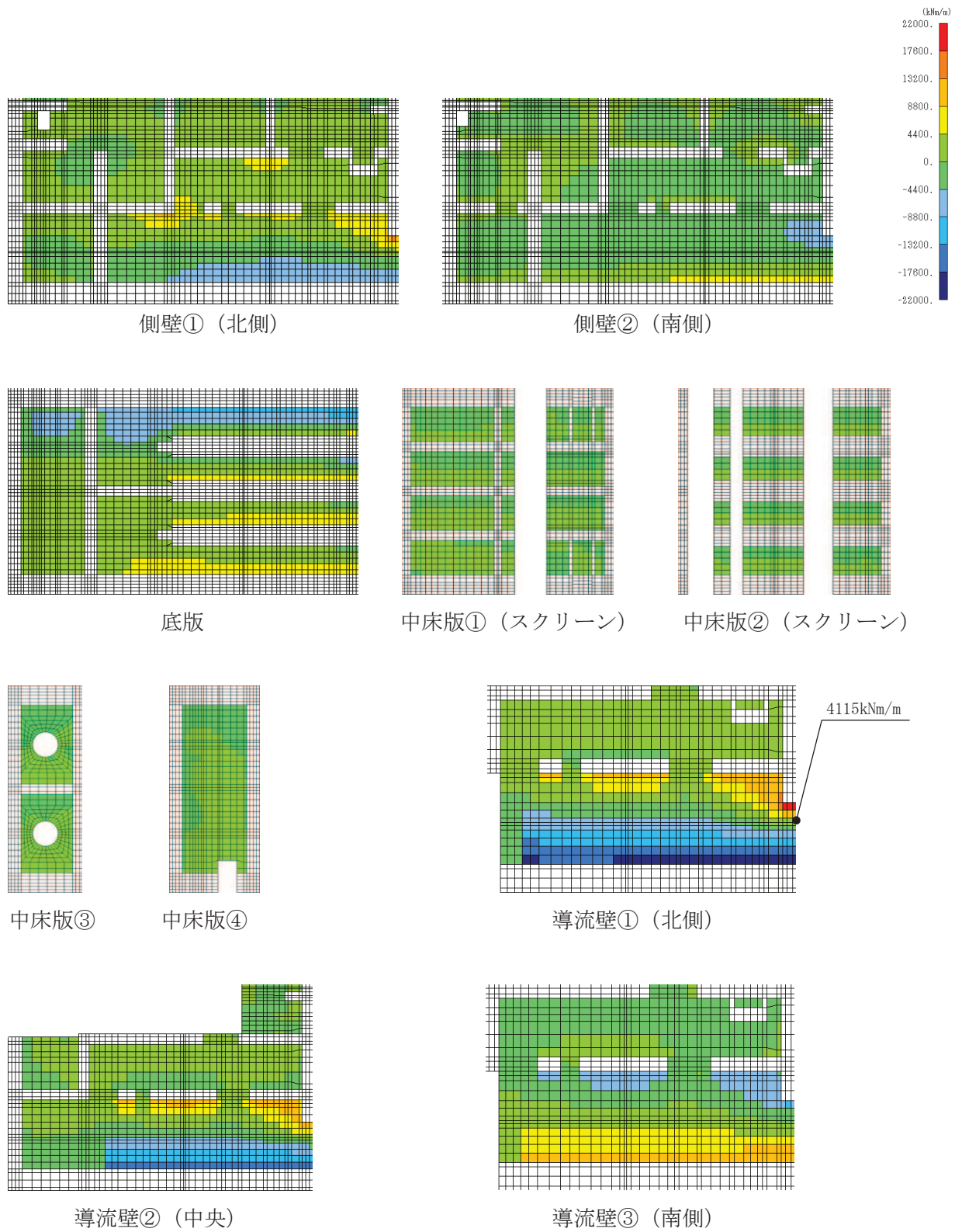
図 4-9(1) セン断破壊に対する照査値最大時の断面力分布図 (曲げモーメント (kN・m/m) : M_y ) (導流壁①, 解析ケース④, S_s - N1 (+ +) )
