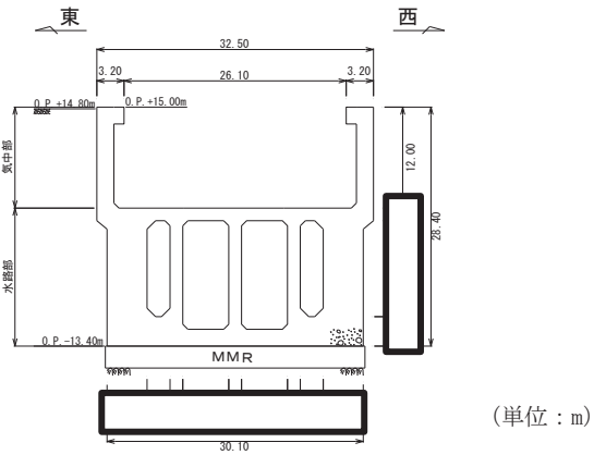
図 2-4 海水ポンプ室断面図 (B-B 断面, 東西 (補機ポンプエリア))
