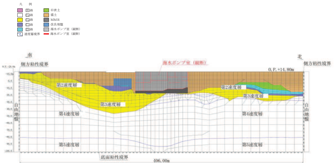
図 3-66 海水ポンプ室の地震応答解析モデル図 (D-D 断面, 南北)
