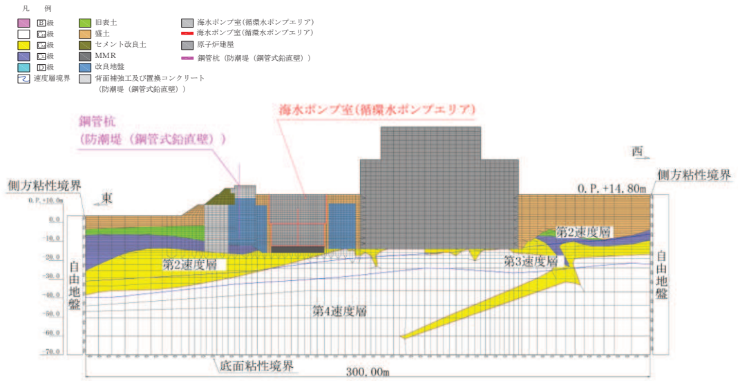
図 3-65 海水ポンプ室の地震応答解析モデル図 (C-C 断面, 東西 (循環水ポンプエリア))
