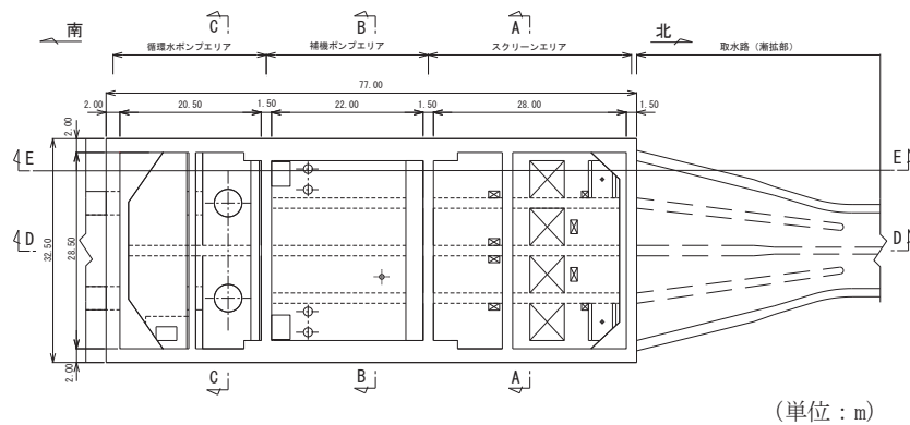
図 2-2 海水ポンプ室平面図
