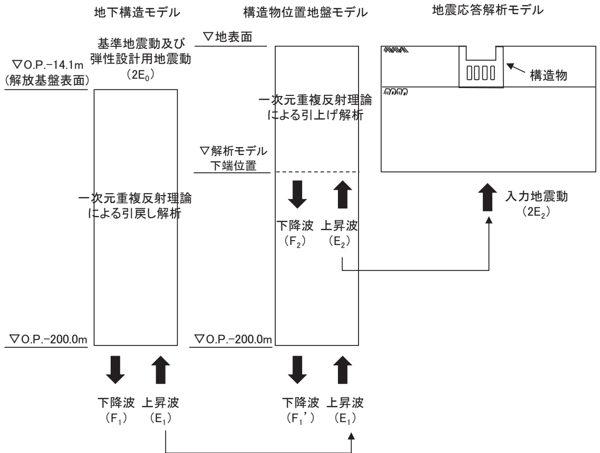
図 3-6 入力地震動算定の概念図（基準地震動 S_s 及び弾性設計用地震動 S_d ）
