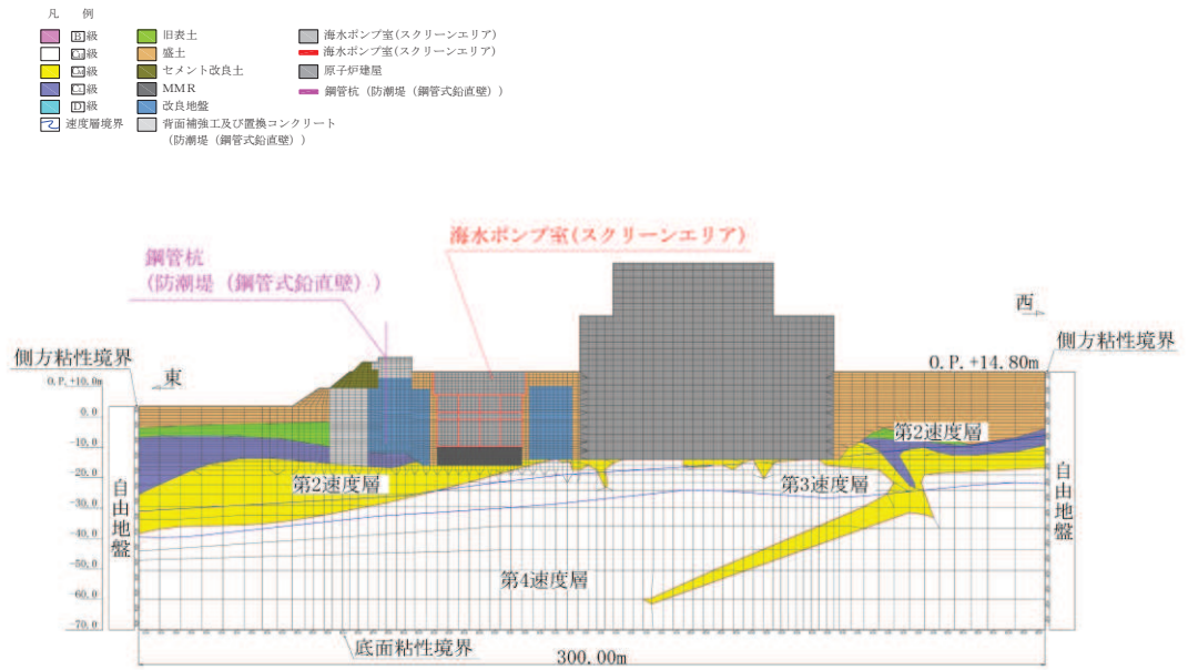
図 3-63 海水ポンプ室の地震応答解析モデル図 (A-A 断面, 東西 (スクリーンエリア))
