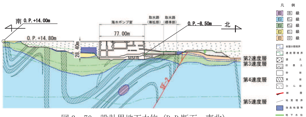
図 3-70 設計用地下水位 (D-D 断面, 南北)
