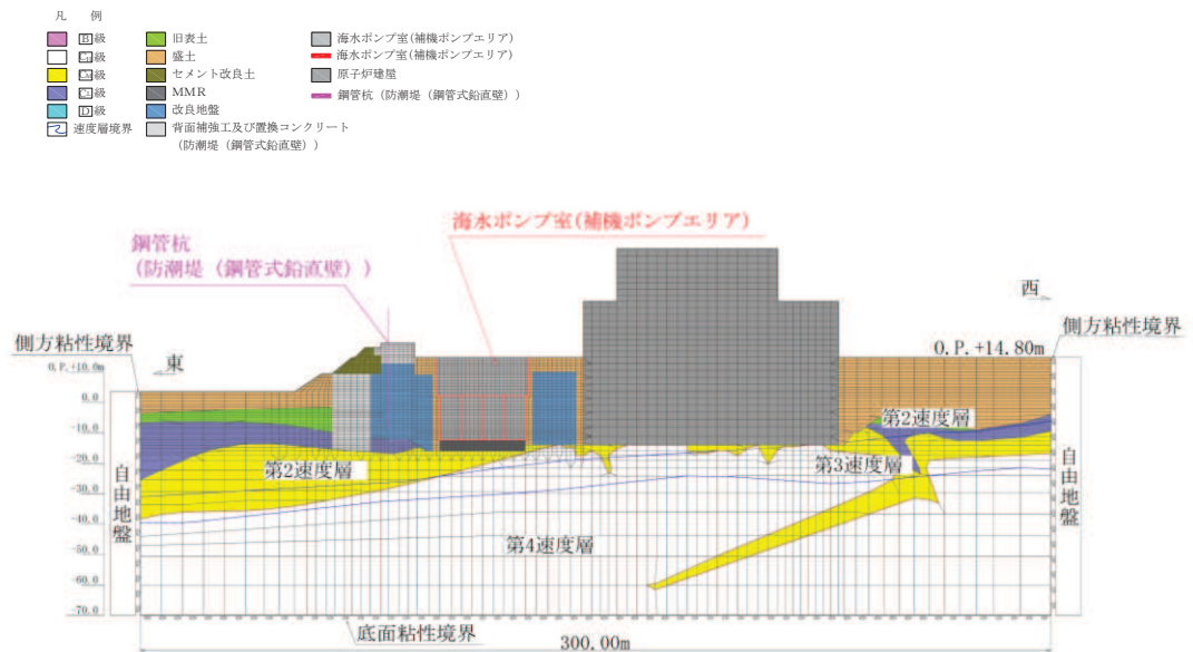
図 3-64 海水ポンプ室の地震応答解析モデル図 (B-B 断面, 東西 (補機ポンプエリア))
