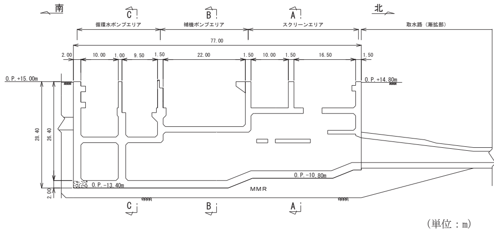
図 2-6 海水ポンプ室断面図 (D-D 断面)
