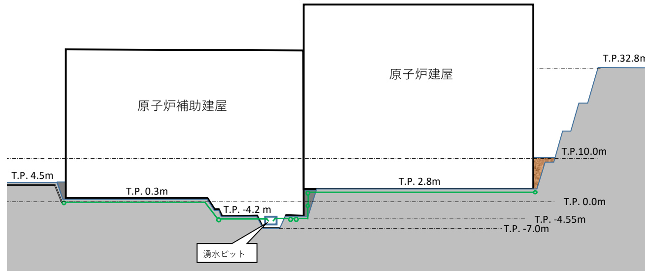
2-14図 集水管の配置と建屋基礎底面のレベル(A-A断面)
