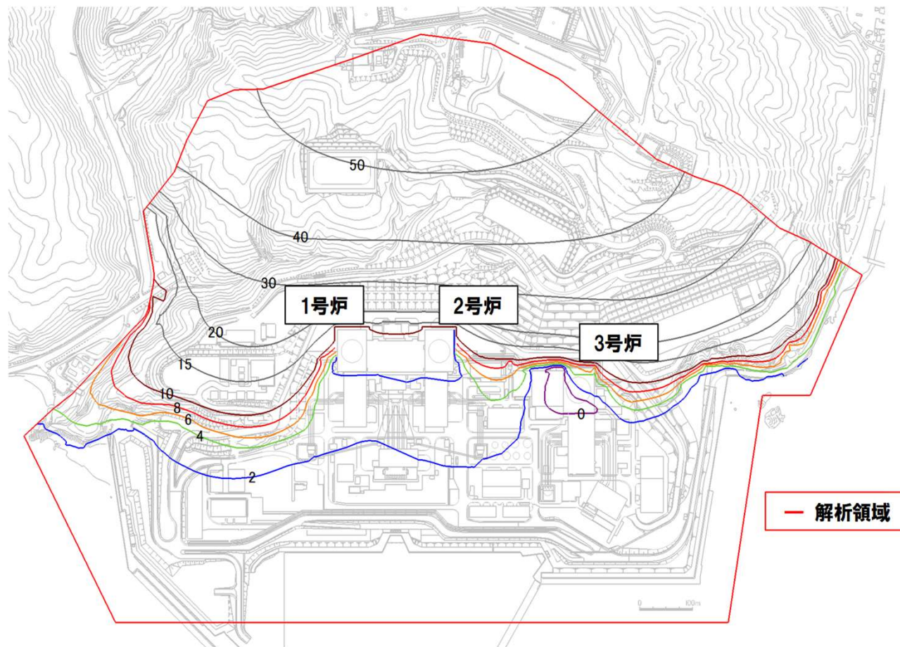
添付3-1図 三次元浸透流解析結果(定常状態・防潮堤設置前モデル)
