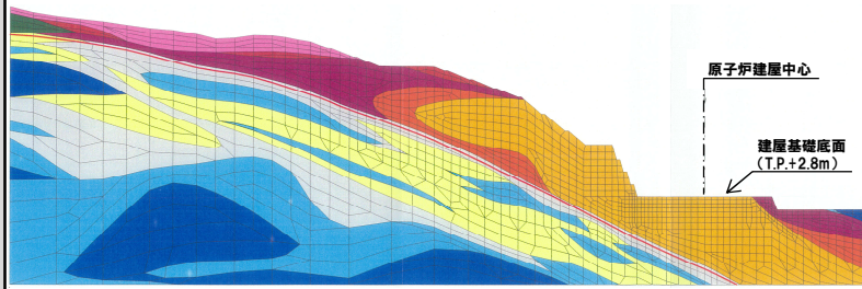
3号炉炉心断面
