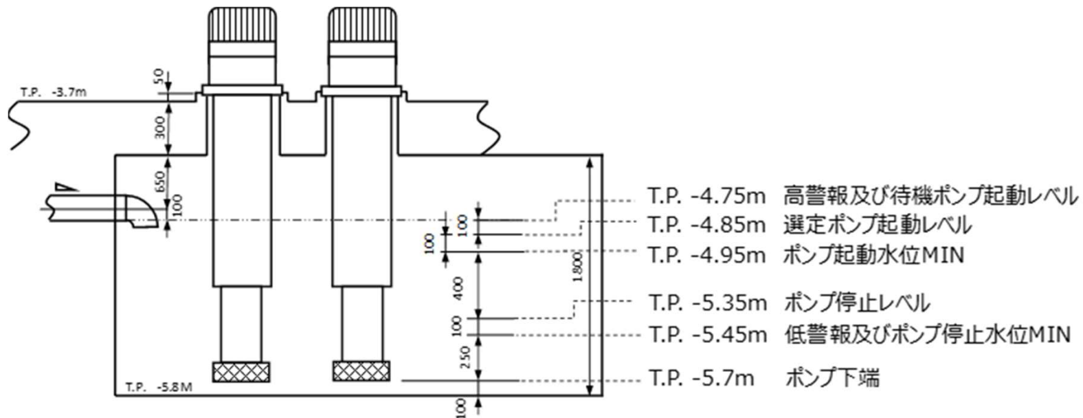
2-15図 地下水排水設備のうち湧水ピット断面図
