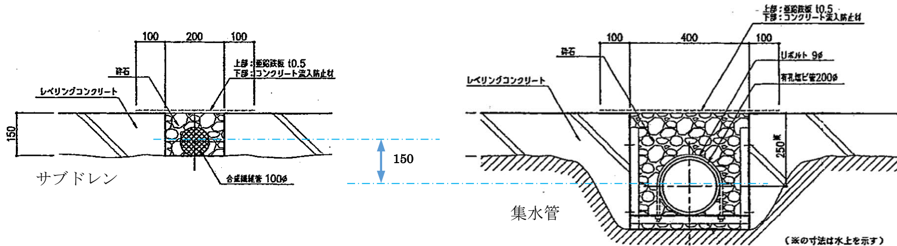
2-16図 地下水排水設備のうち集水管他の敷設断面図
