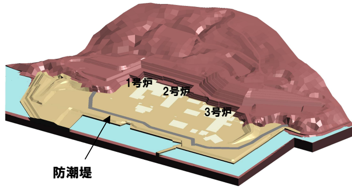
予測解析用モデル
