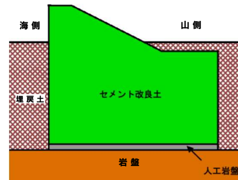
1-2図 防潮堤概要図
