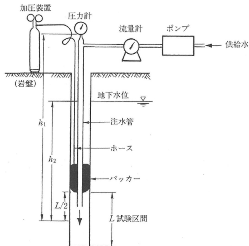
添付6-2図 現場透水試験(ルジオン試験)の概要図 (地盤調査の方法と解説(地盤工学会, 2013))
