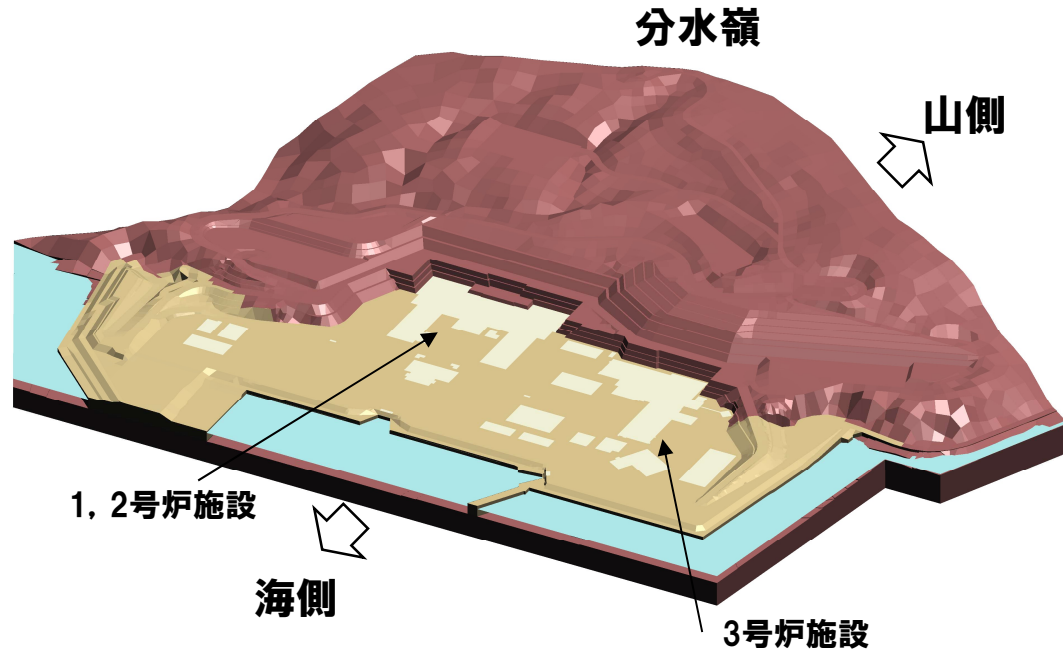
2-4図 解析モデル(妥当性検証解析用)鳥瞰図
