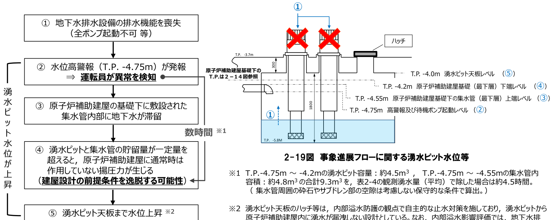
2-18図 機能喪失後の事象進展フロー
