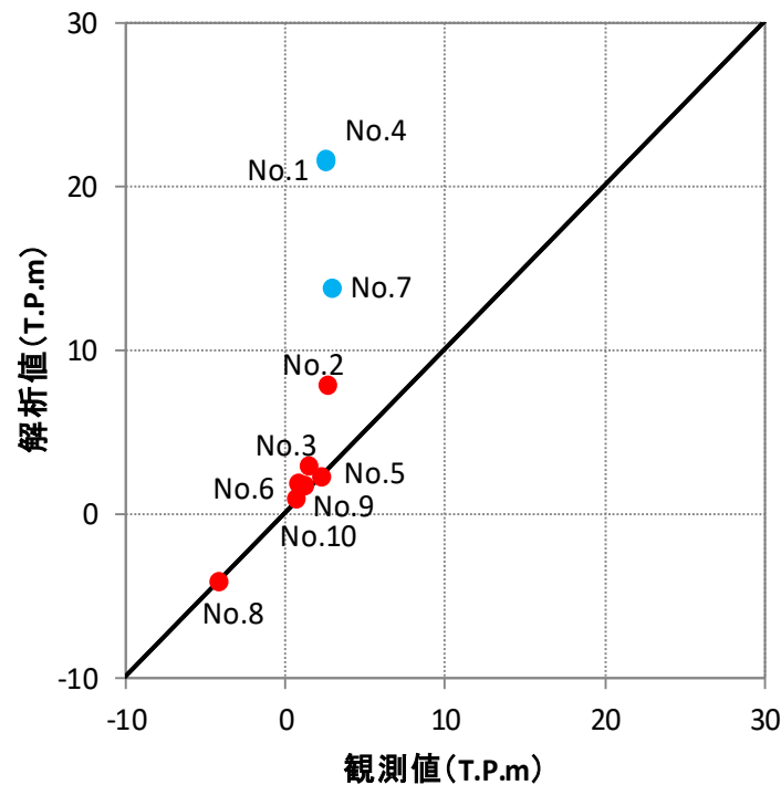
2-7図 観測値と解析値の比較(地下水位)
