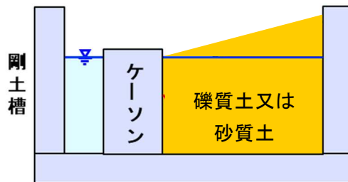
図-2 模型地盤のイメージ（傾斜あり護岸モデル）
