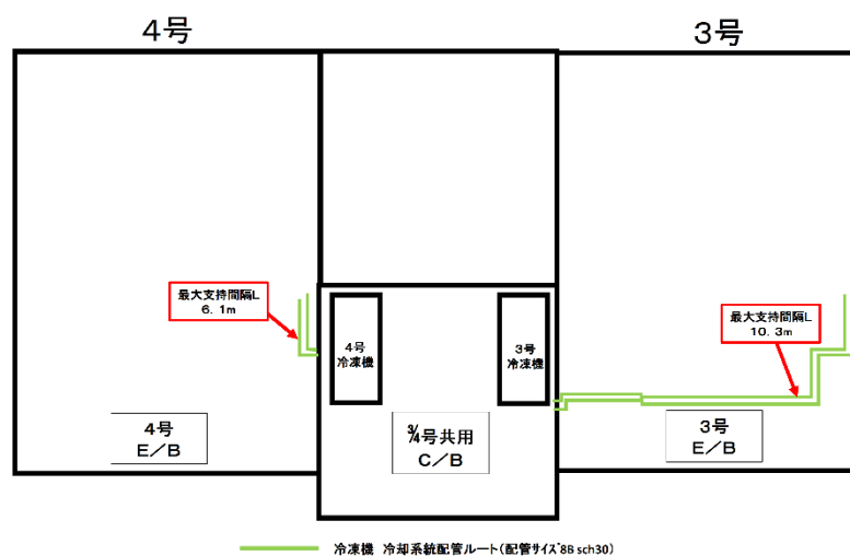
図 18-3-1 大飯3号との配管ルートの違い（配管サイズ 8B sch30 EL26.0m の例）
