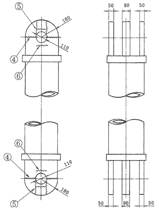
(c) サポートパイプ側ヒンジ
