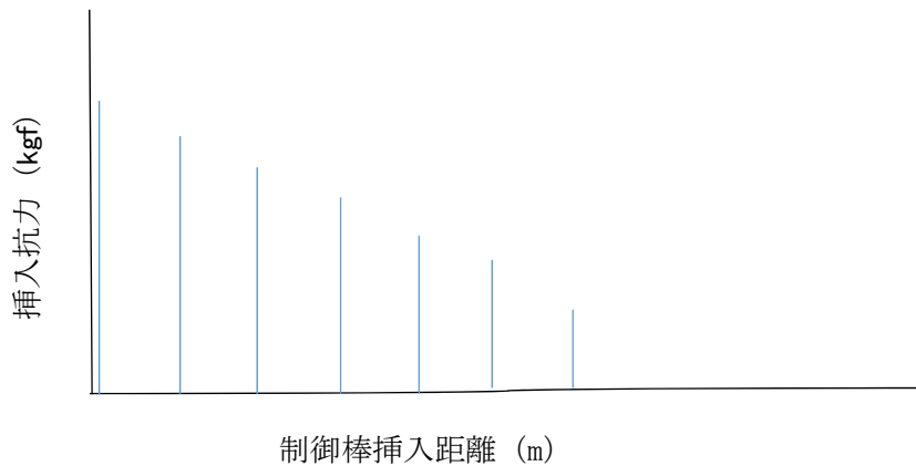
図 15-2-7 制御棒挿入時間解析へのインプットとなる GT案内板およびRCC摩耗による抗力イメージ
