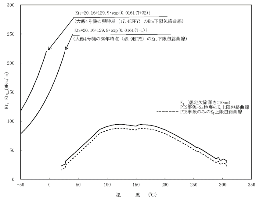
図 7-2 Ss 地震を考慮した PTS 評価結果
