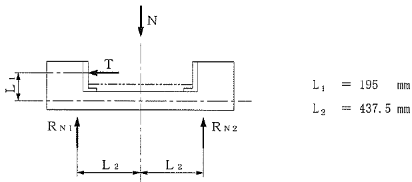
図9-1-3 サポートシューに作用する荷重
