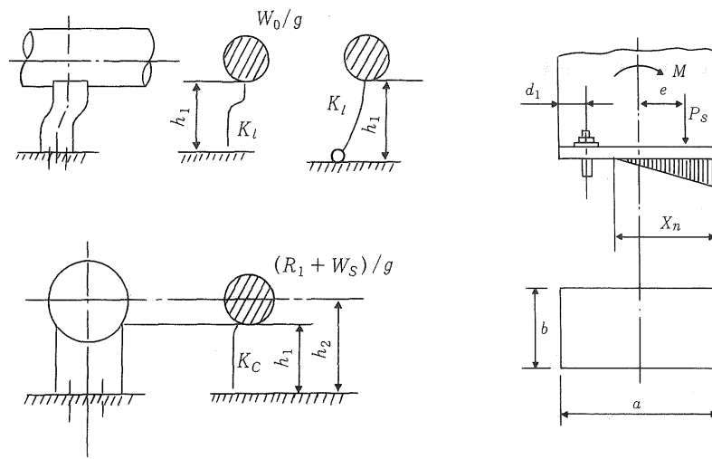
図1 解析モデル
