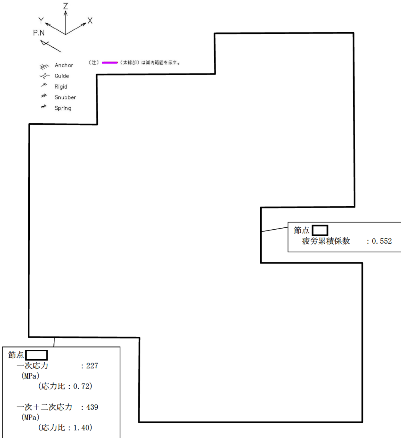
蒸気発生器ブローダウン系統配管 A-蒸気発生器ブローダウン配管 PEN#507CV外 CVBD内 【S s地震】
