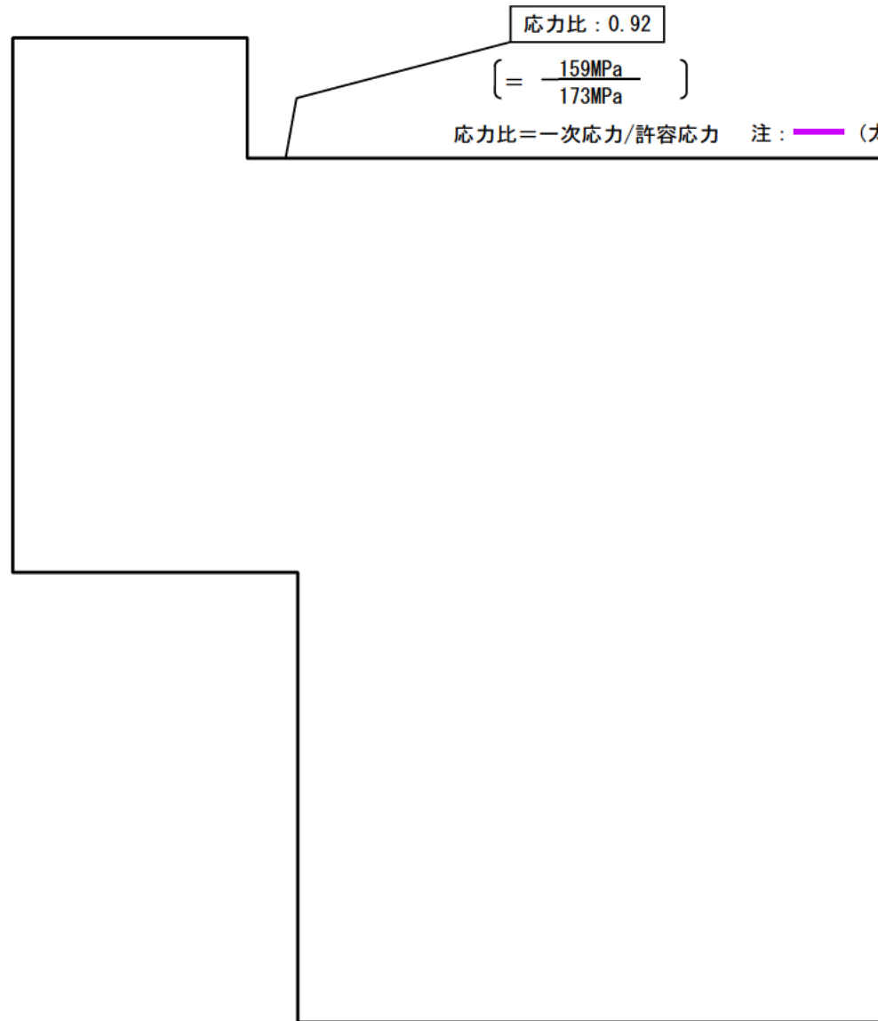
補助蒸気系統配管 スチームコンバータ加熱蒸気管
