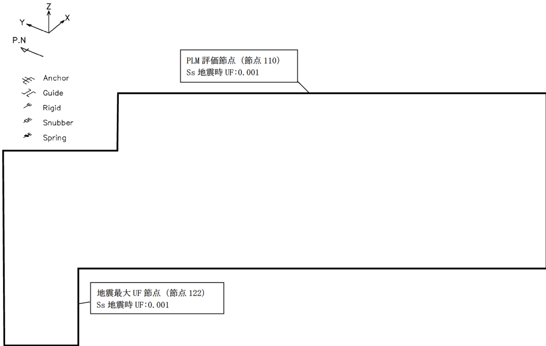
図 4-2-3 大飯 4 号炉 加圧器サージ配管 解析モデル
