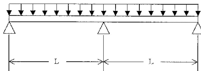
図 18-3-2 2スパン3点支持の等分布質量の連続梁モデル
