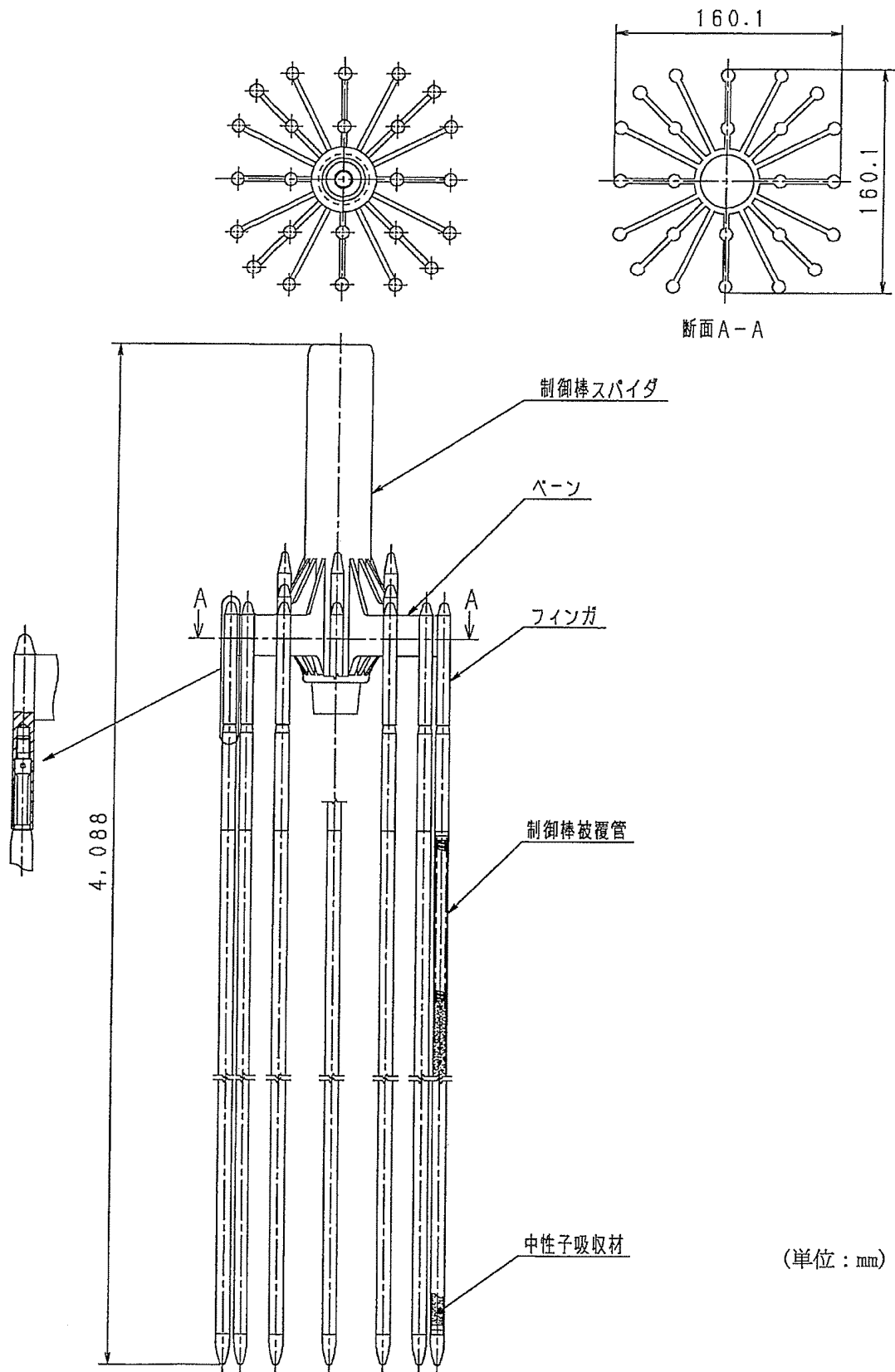
図15-1-1 17×17型制御棒クラスター構造図
