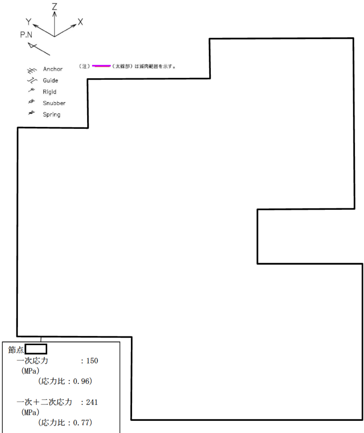
蒸気発生器ブローダウン系統配管 A-蒸気発生器ブローダウン配管 PEN#507CV外 CVBD内 【Sd地震】
