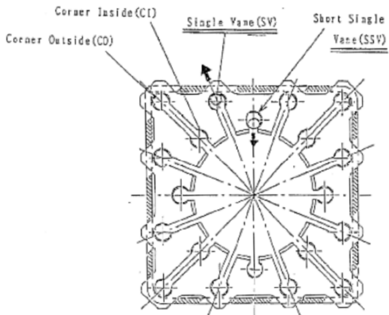
図 15-2-3 15×15GT の摩耗形態
