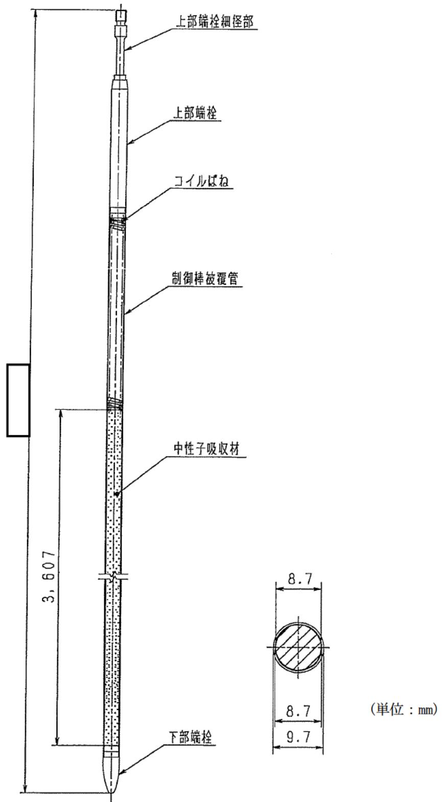
図15-1-2 17×17型制御棒構造図
