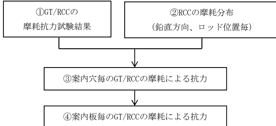
図15-2-1. GT/RCC摩耗による抗力の設定フロー
