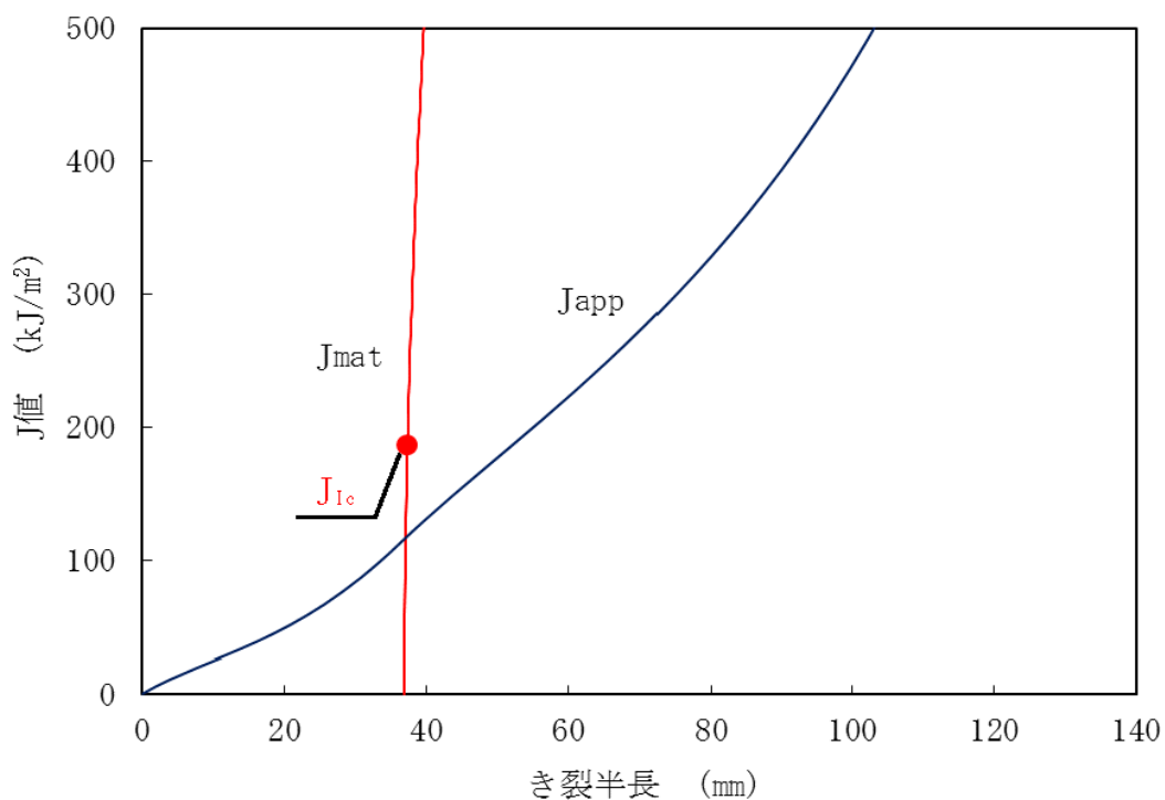
図7 ホットレグ直管の亀裂安定性評価線図
