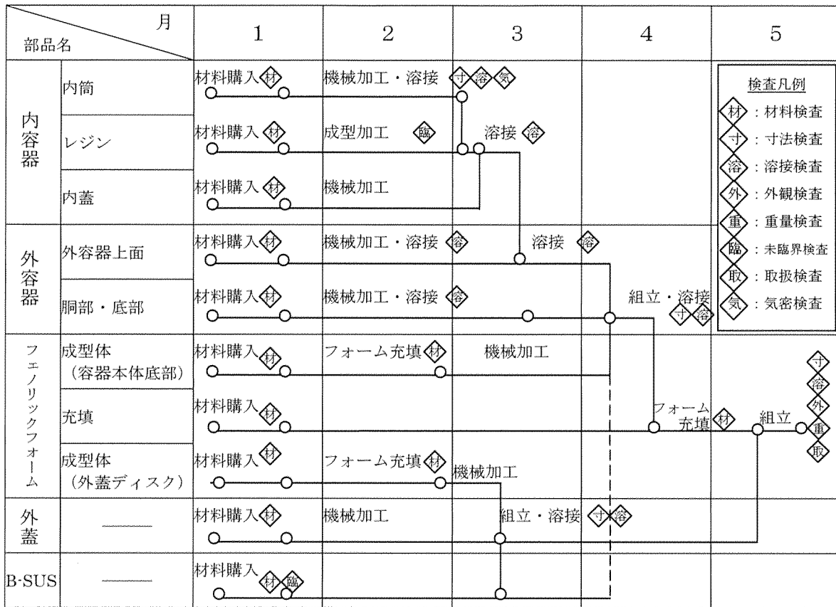
(ハ) 第1図 TNF-XI型輸送容器の製作スケジュール
