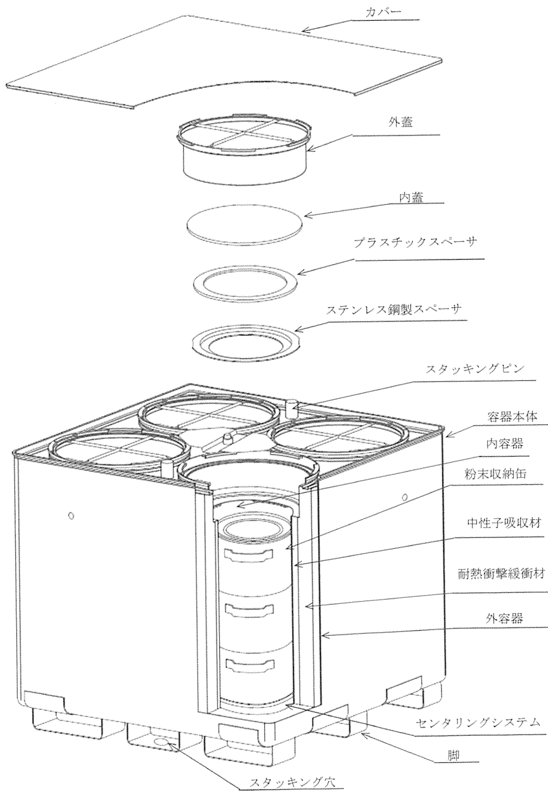
図1 TNF-XI型輸送物外観図
