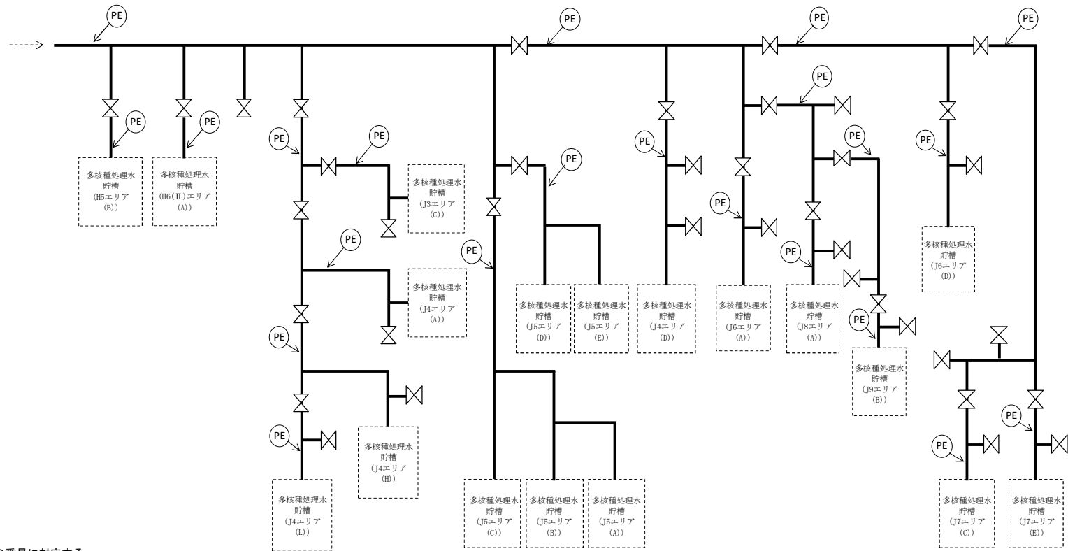
図-1 配管概略図 (13/18)
