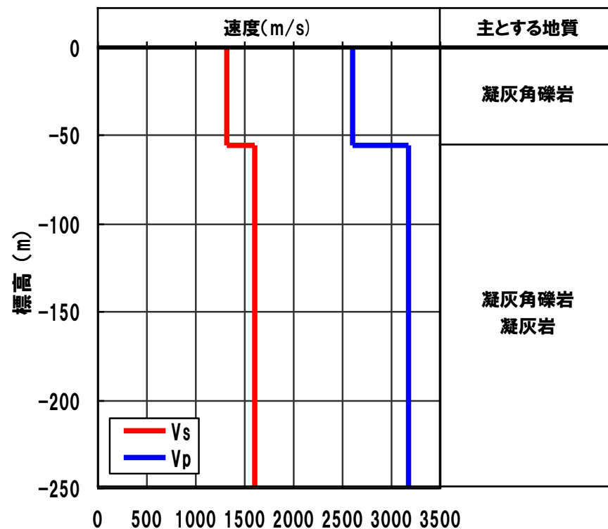
地震観測点PS検層結果
