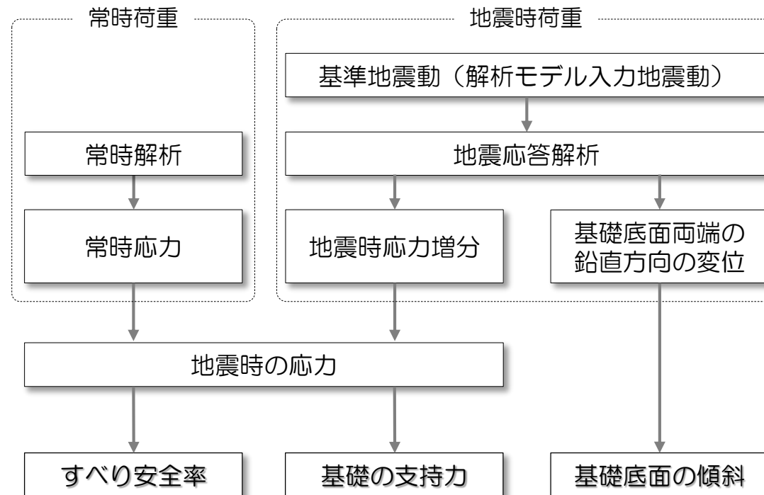
安定性評価フロー
