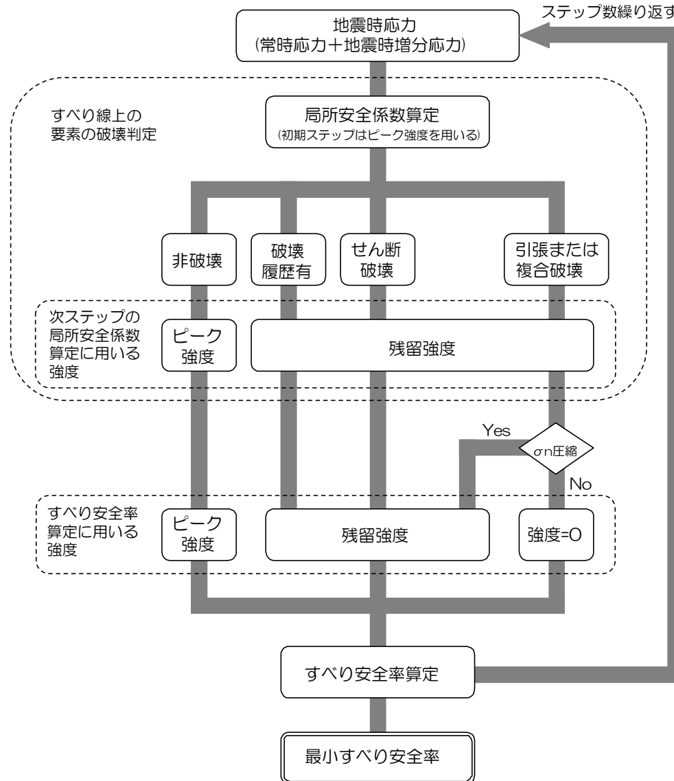
すべり安全率の算定フロー
