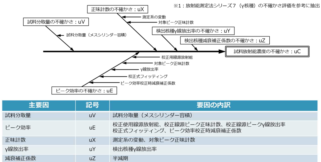
図 3.4-24 不確かさの要因のリスト (要因図とまとめ表)
