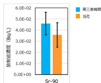
図 3.4-38 β核種分析装置による Sr-89, Sr-90 放射能濃度の拡張不確かさ (UC[Bq/L])
