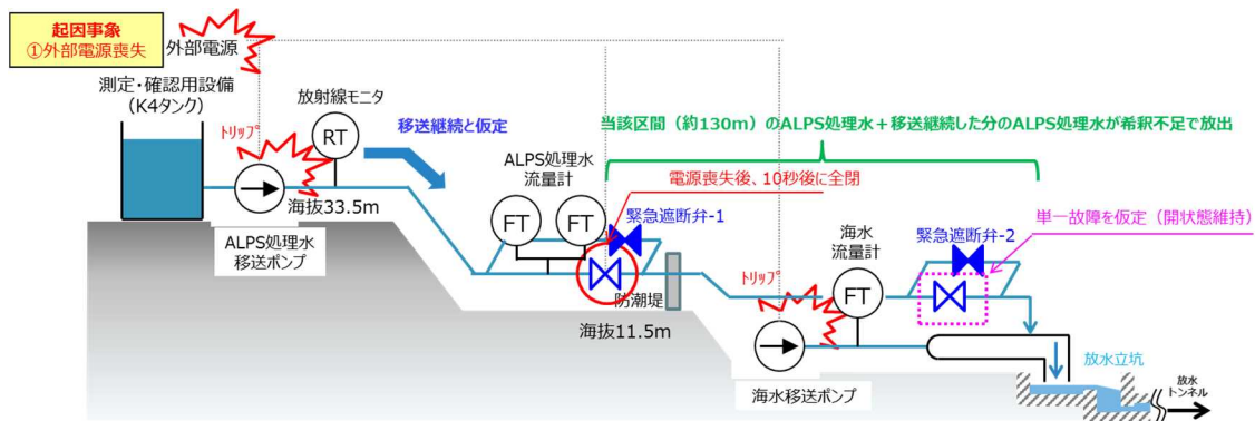
図 3.2-4 起回事象(1)「外部電源喪失」時の異常事象のイメージ
