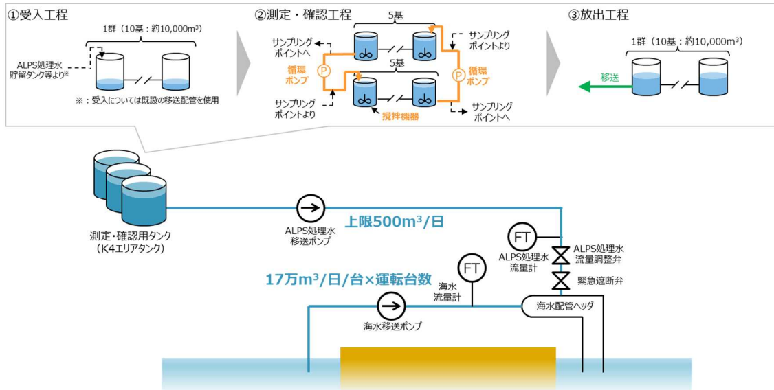
図 3.1-1 ALPS 処理水希釈放出設備の工程概要
