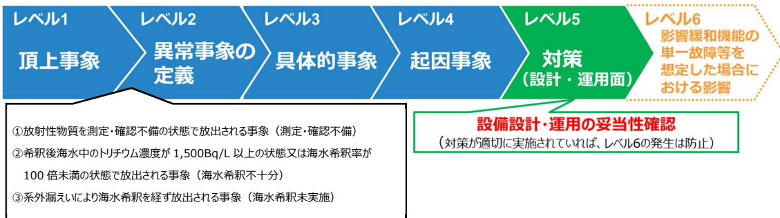
図 3.2-1 マスターロジックダイアグラム (MLD) による評価方法
