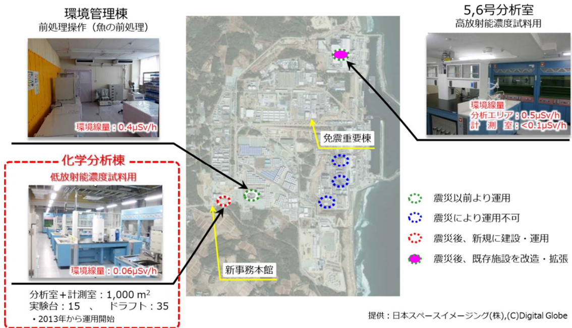
図 3.4-2 福島第一原子力発電所構内における分析施設
