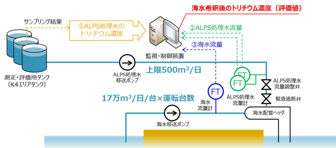
図 5.1.3.1-1 ALPS 処理水の混合希釈率の監視イメージ
