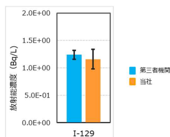
図 3.4-36 低バック液体シンチレーション計数装置による放射能濃度の拡張不確かさ (UC[Bq/L])
