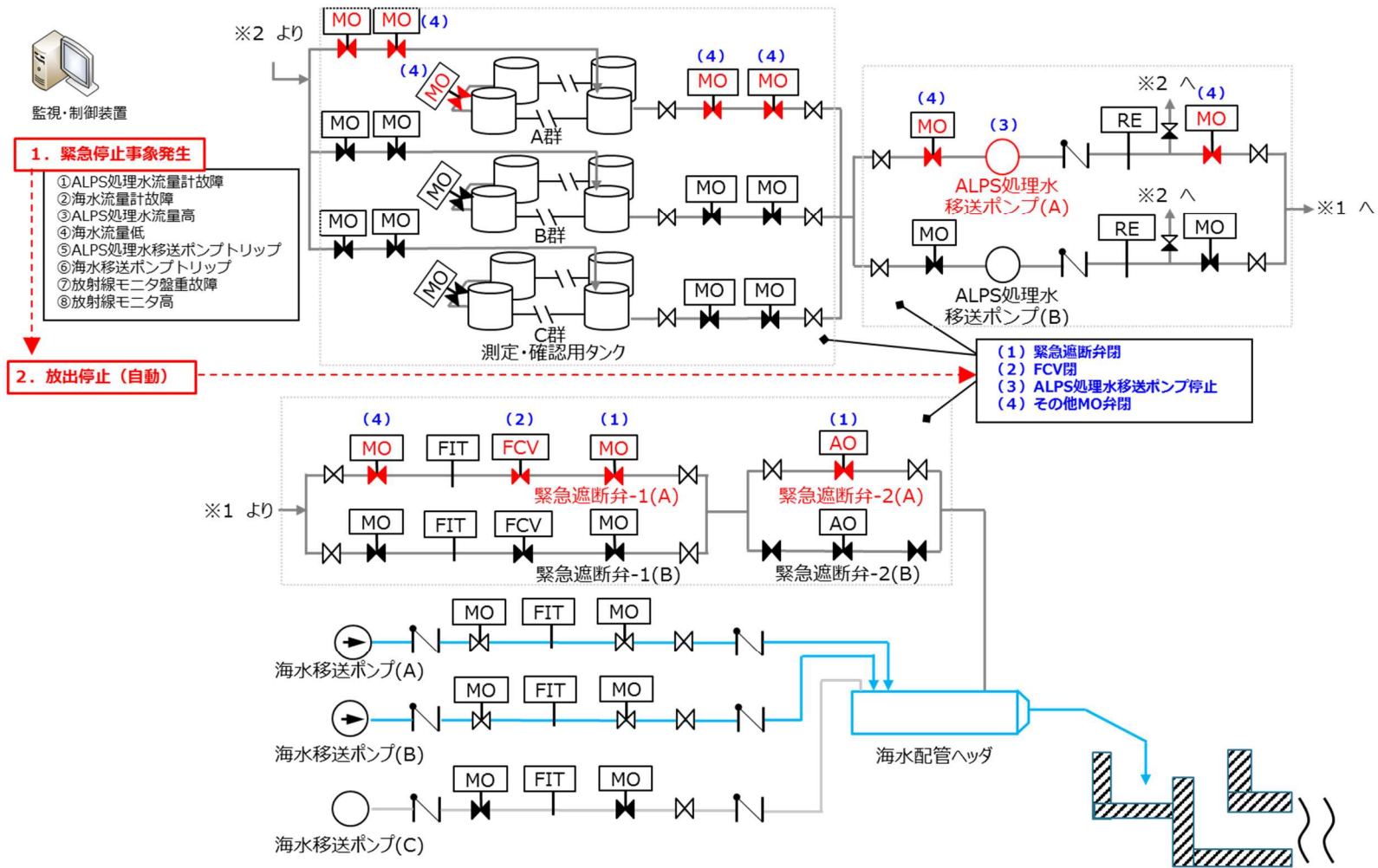
図 3.1-18 放出工程の設備状態 (緊急停止)
