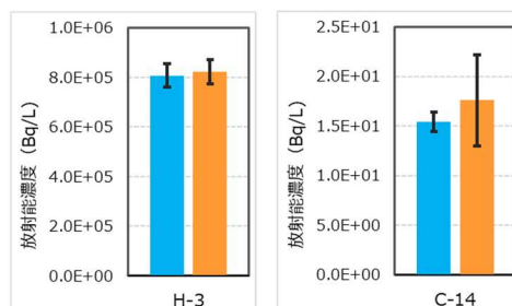
図 3.4-36 低バック液体シンチレーション計数装置による放射能濃度の拡張不確かさ (UC[Bq/L])
