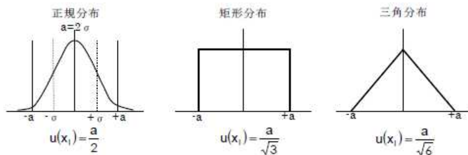
図 3.4-42 分布と不確かさへの変換式
