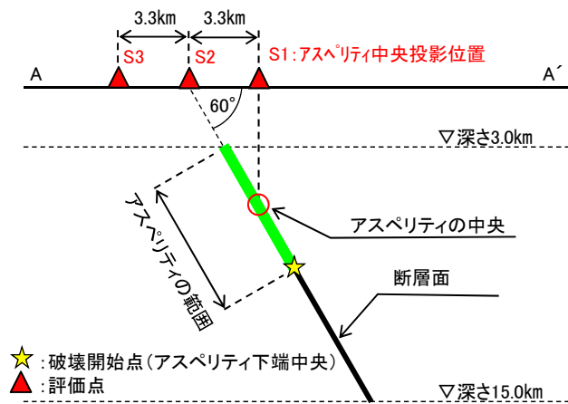
評価点の配置図(A-A'断面)
