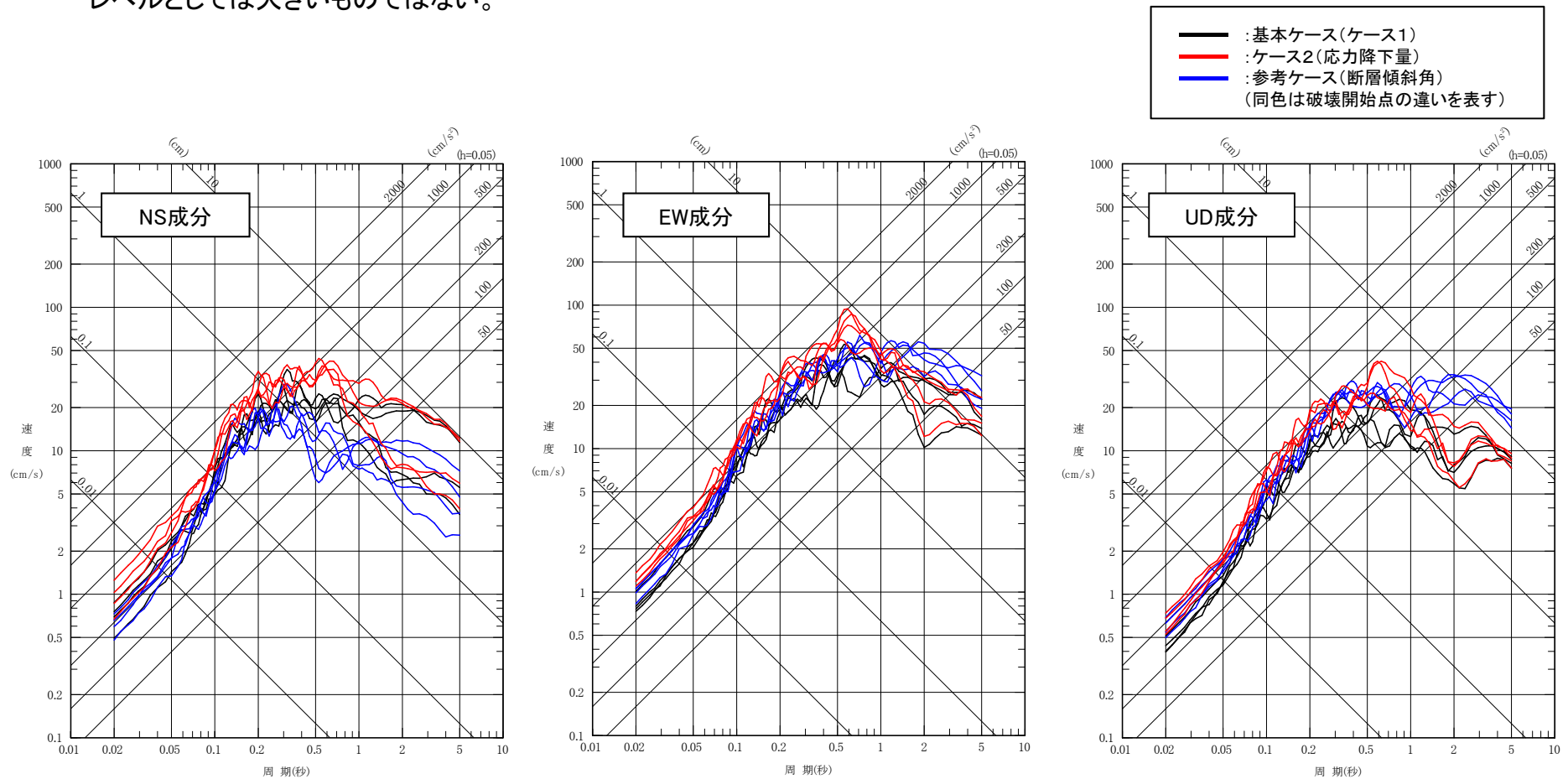
断層モデルを用いた手法による地震動評価 「横浜断層による地震」参考ケース(断層傾斜角)(PN基準)
