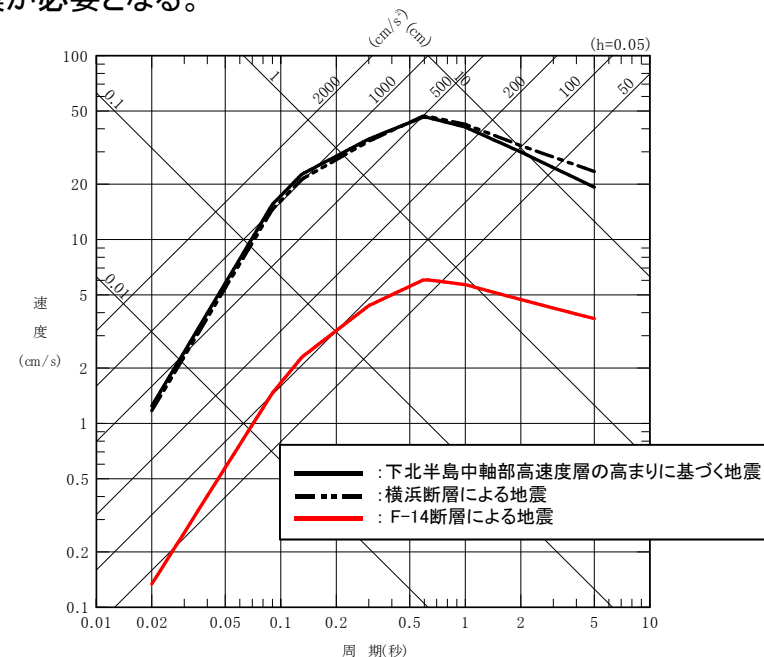
検討用地震及びF-14断層による地震の応答スペクトル 〔Noda et al.(2002), 水平方向, 内陸補正なし〕
