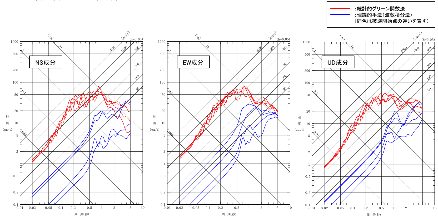
統計的グリーン関数法と理論的手法による地震動評価の比較(PN基準) 「下北半島中軸部高速度層の高まりに基づく地震」ケース2(地震規模)の応答スペクトル
