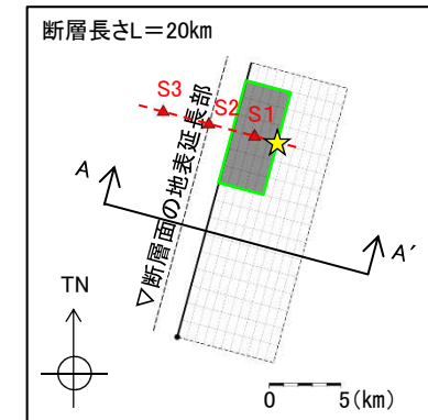
断層配置図
