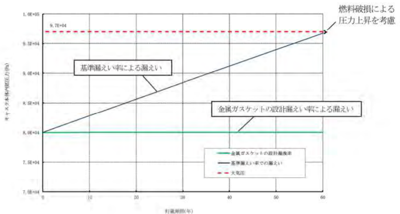
(b) 15×15 燃料収納時
