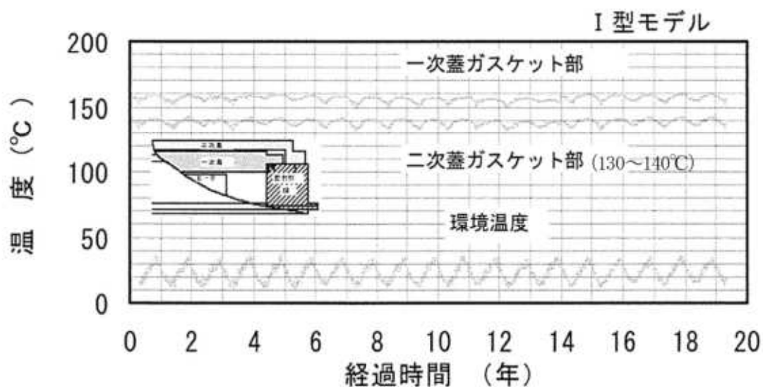
第7図 金属ガスケット（二次蓋）の長期密封性能試験結果（眼鏡型） (2)
