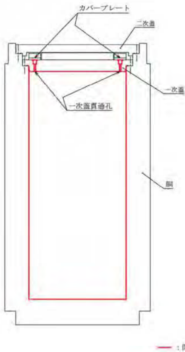
第1図(2/2) MSF-24P(S)型の閉じ込め構造 (基礎等に固定する設置方法)
