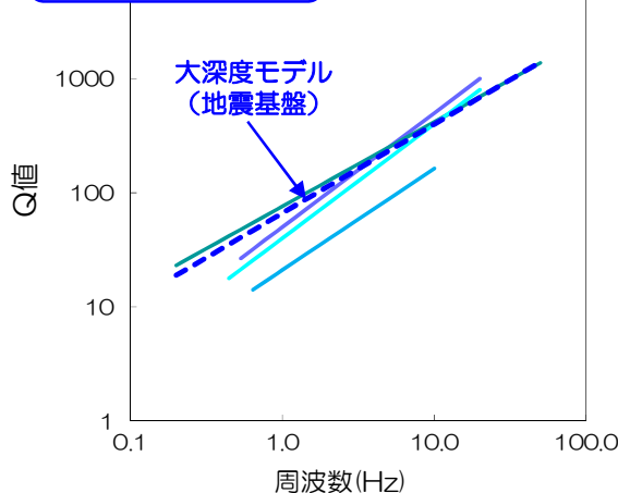
地震基盤のQ値との比較
