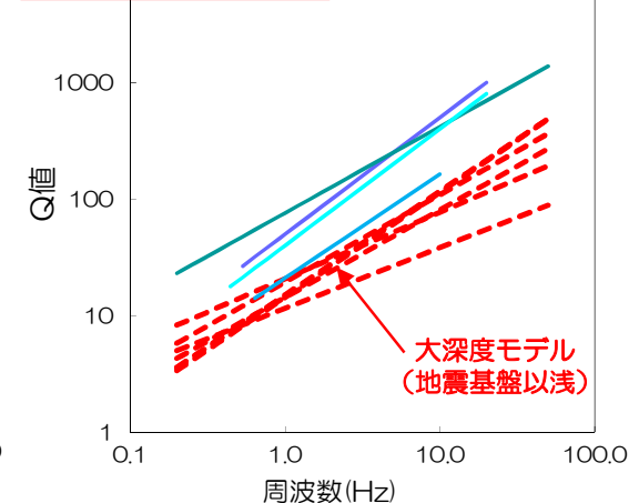
地震基盤以浅のQ値との比較
