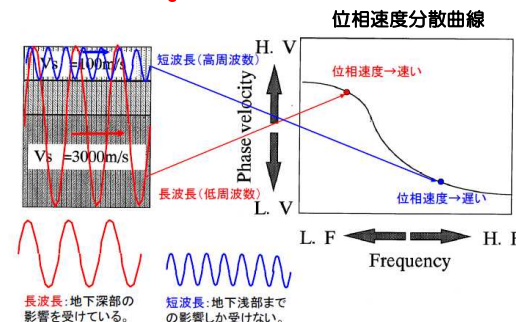
地下構造と位相速度の対応関係の概要
