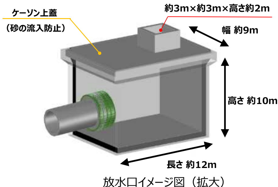
放水口イメージ図
