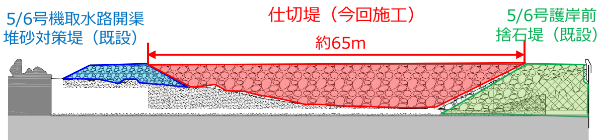
B-B断面図
