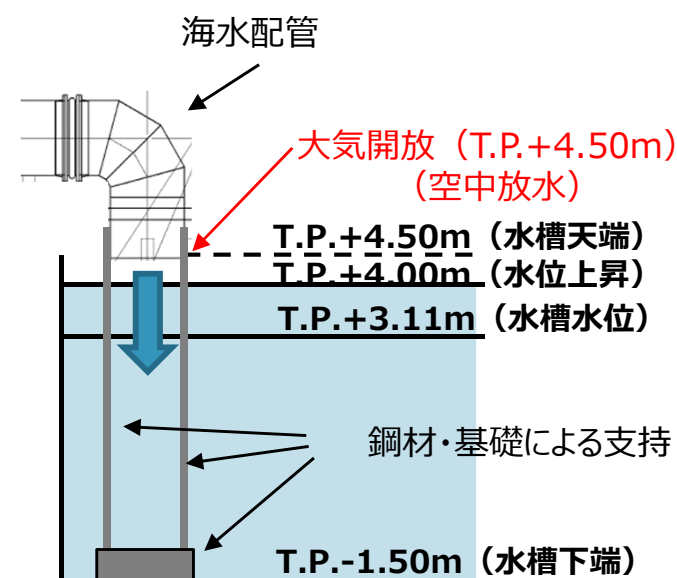
放水立坑（上流水槽）への流入
