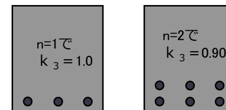
引張鋼材段数 n と k_3 の関係模式図
