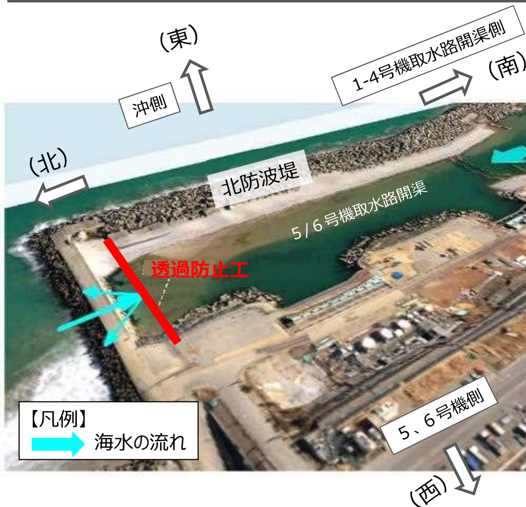
現況
