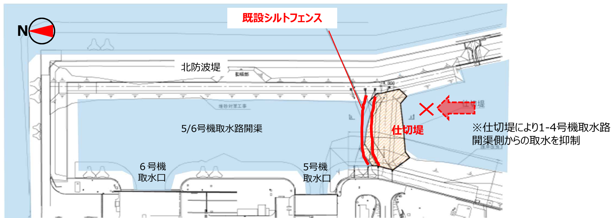
仕切堤位置図
