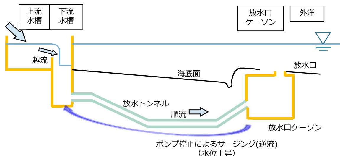
放流設備の概略図
