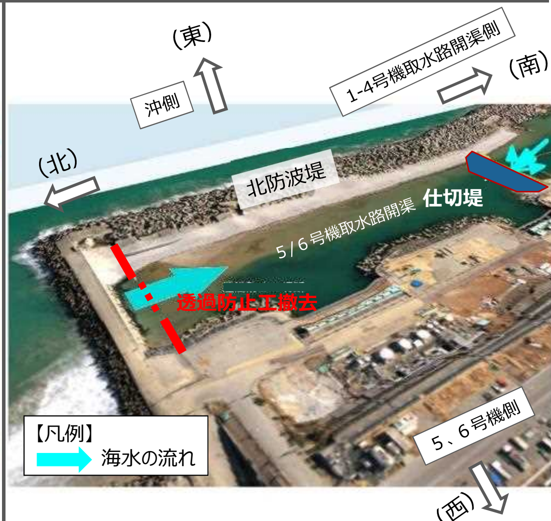
工事完了後
