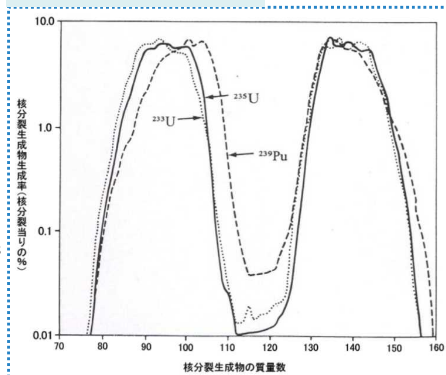
核分裂生成物の質量分布
