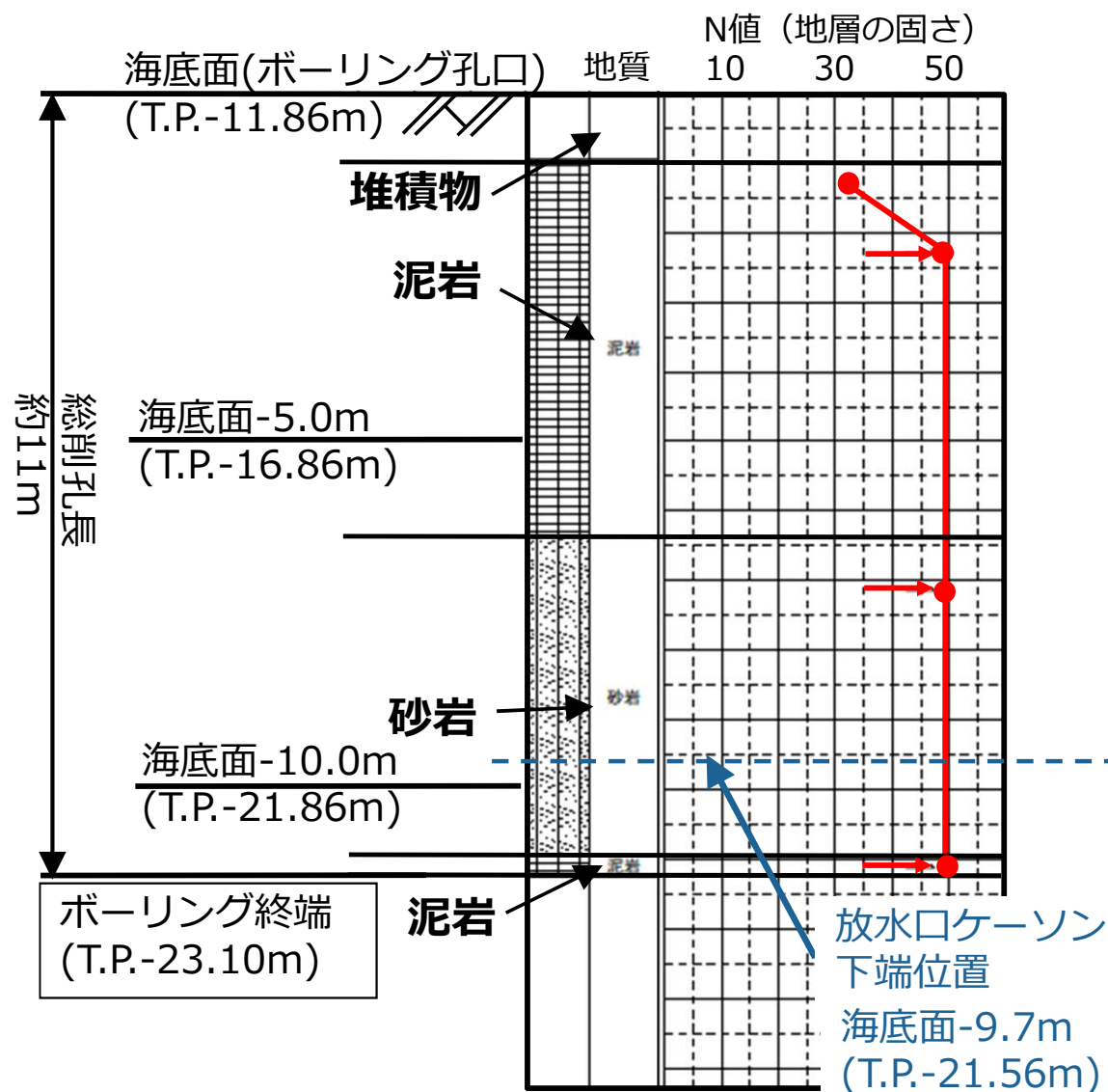
地質調査データ①の柱状図
