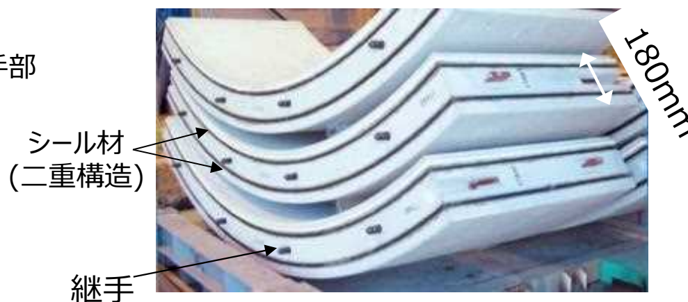
鉄筋コンクリート製セグメント
