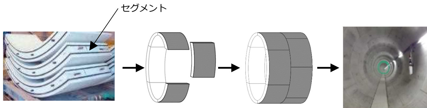
シールドトンネルの組立イメージ
