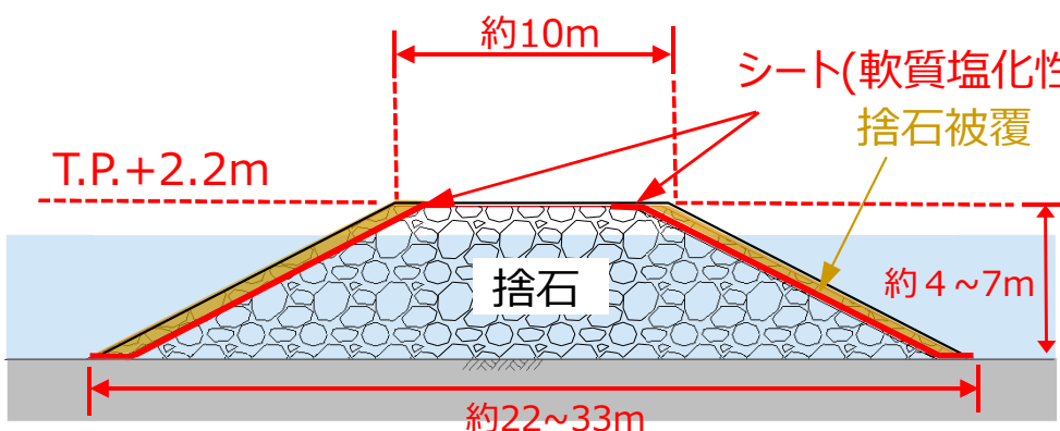
A-A断面図
