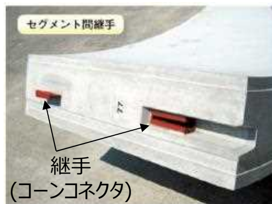
円周方向の継手(コーンコネクタ)
