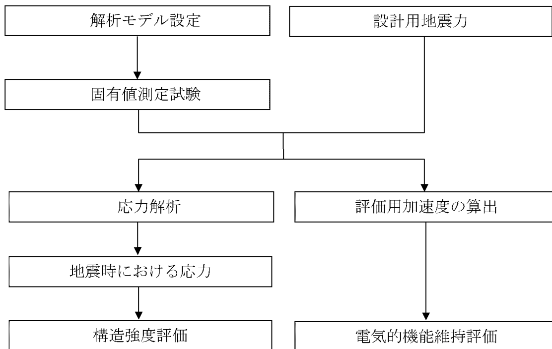
第 2-2 図 火災受信機盤の耐震評価フロー
