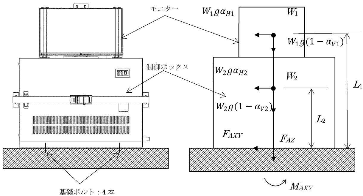
第 4-1 図 火災受信機盤②の基礎ボルトの応力評価モデル
