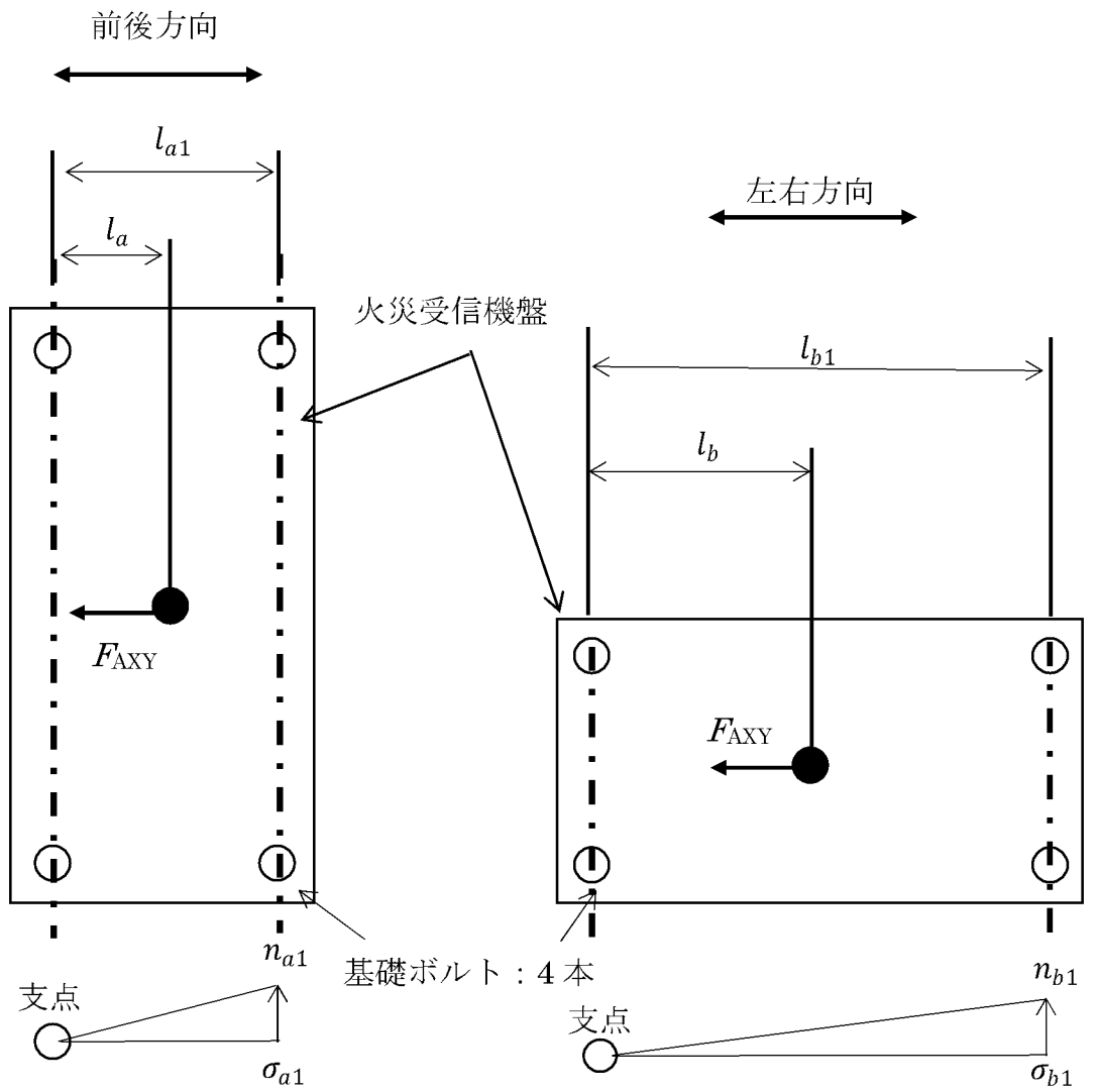
第 4-2 図 火災受信機盤②の基礎ボルトの応力評価モデル
