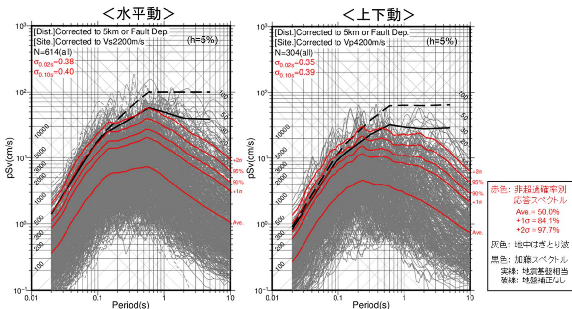
図 4.1 非超過確率別応答スペクトルの算出例
