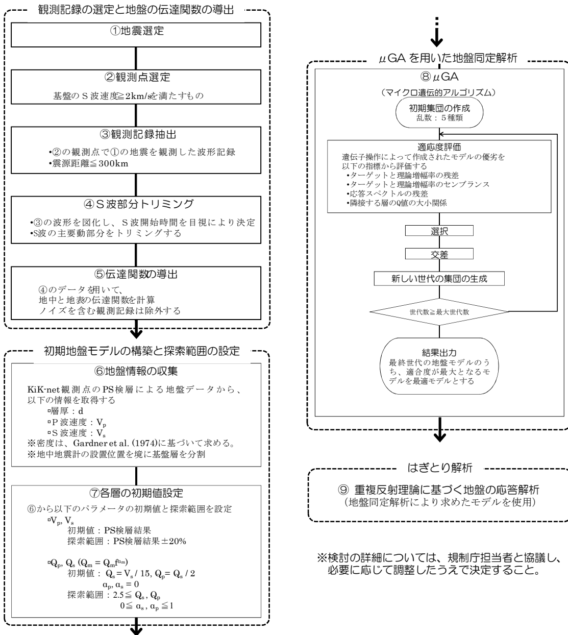
図 4.2 地盤同定及びはざとり解析の流れ
