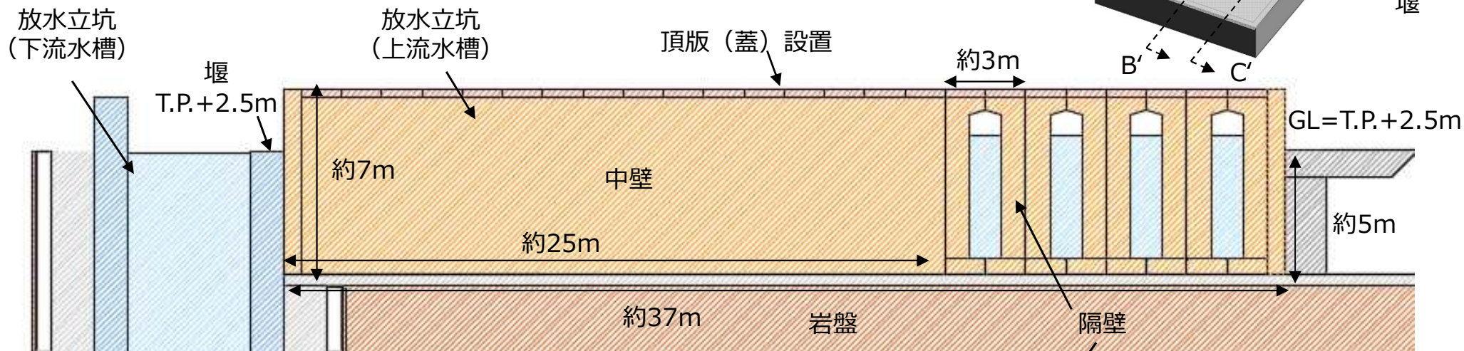
B-B'断面図
