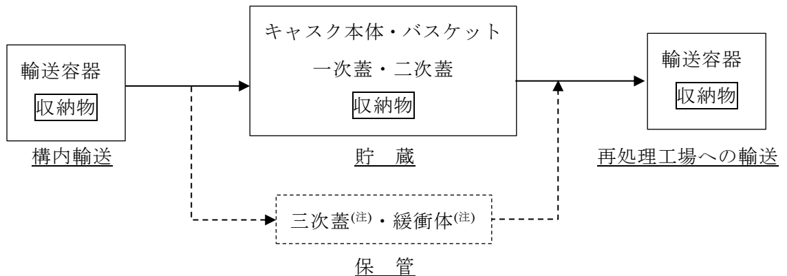
(ロ)-第F.1図 輸送容器の使用方法
