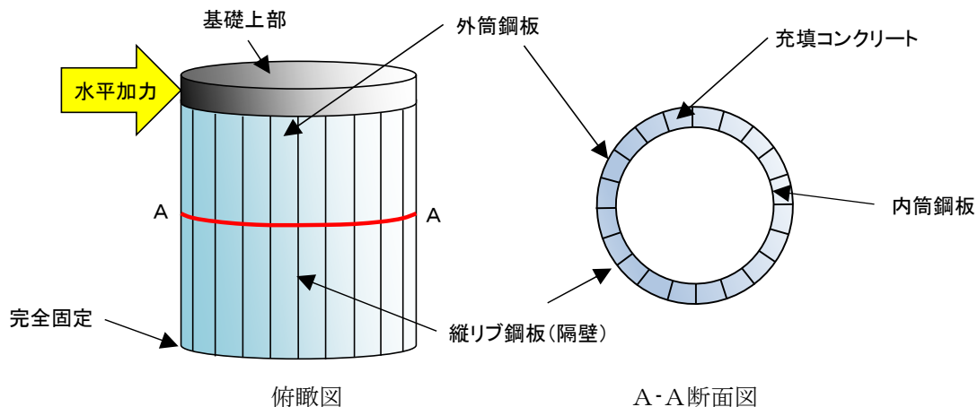
図1 鋼板コンクリート構造製の基礎構造物のイメージ
