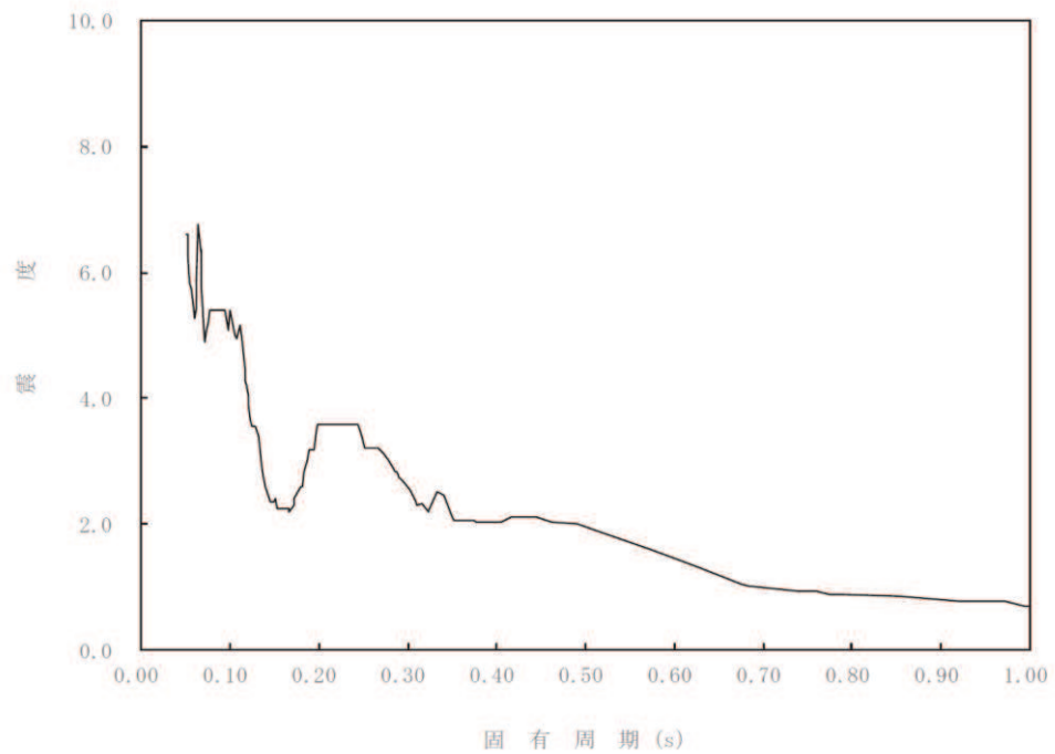
図6 制御建屋 (O.P. 8.00m) 設計用床応答曲線
