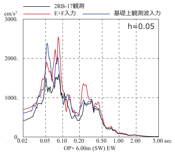
図 3-9 4.7 地震のはざとり波を入力に用いた場合と 基礎版上観測記録を用いたシミュレーション解析結果の比較 (原子炉建屋, EW 方向, 減衰 5%)
