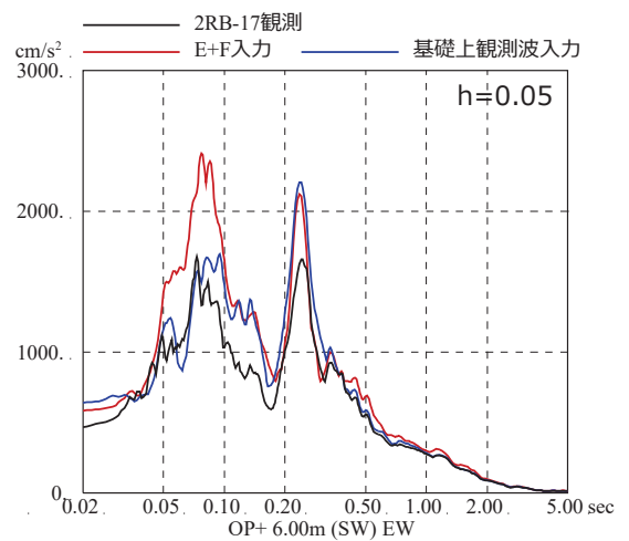
図 3-5 3.11 地震のはざとり波を入力に用いた場合と 基礎版上観測記録を用いたシミュレーション解析結果の比較 (原子炉建屋, EW 方向, 減衰 5%)
