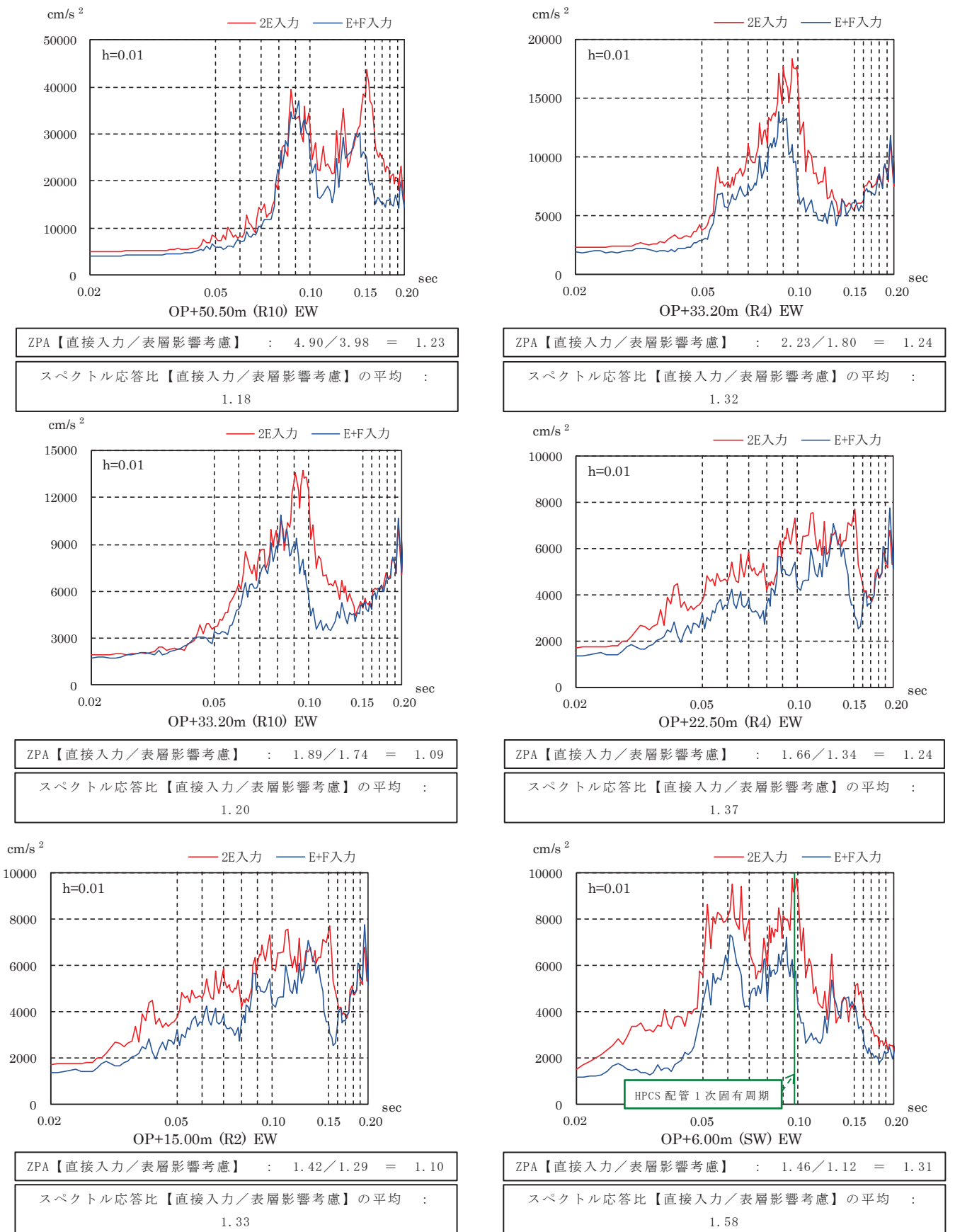
図 4-47 基準地震動 S s -D 2 を直接入力した場合 (2E 入力) と表層地盤の影響を考慮して評価した地震動を入力した場合 (E+F 入力) の機器・配管系評価の比較 (原子炉建屋, EW 方向, 建屋減衰 1%)
