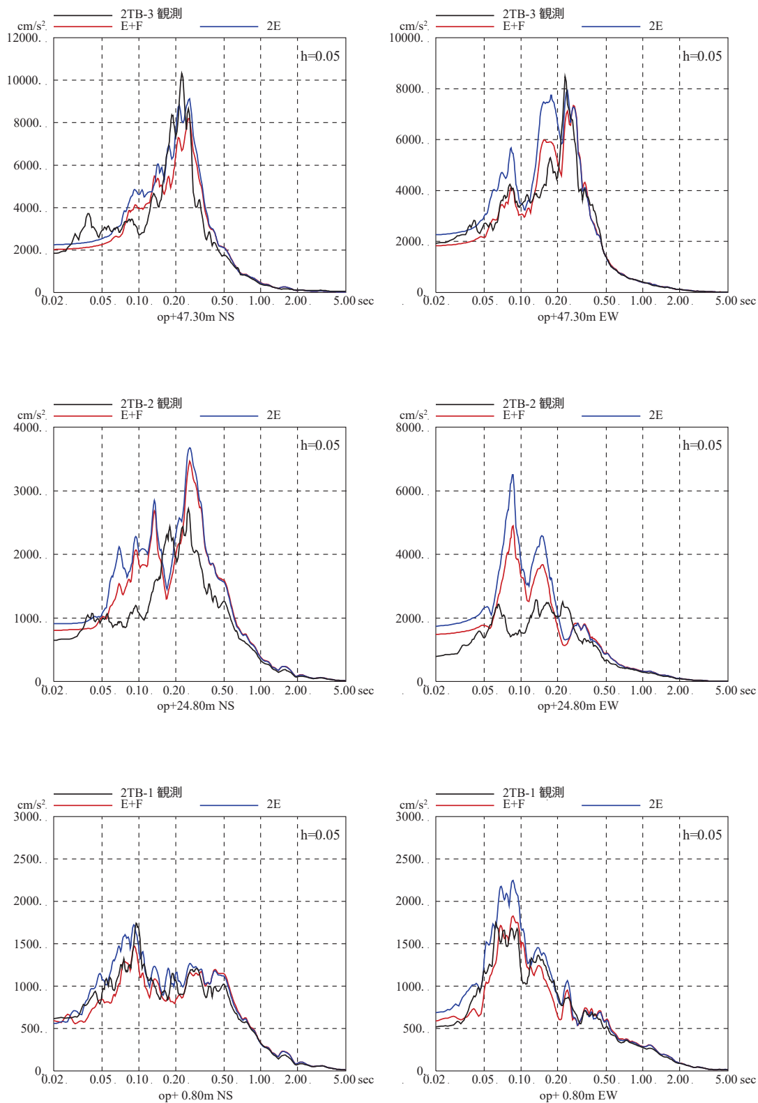
図 3-1 3.11 地震のはざとり波を用いたシミュレーション解析結果の比較 (タービン建屋)
