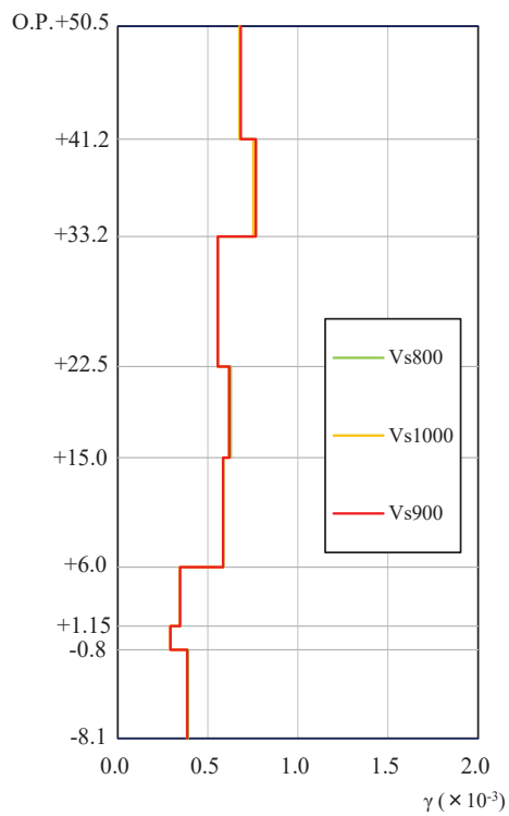
図 3-4 (2) 表層地盤下部のせん断波速度を変化させた場合の 最大応答せん断ひずみの比較 (Vs=800m/s~1000m/s, 基準地震動 S s - D 2, EW 方向)
