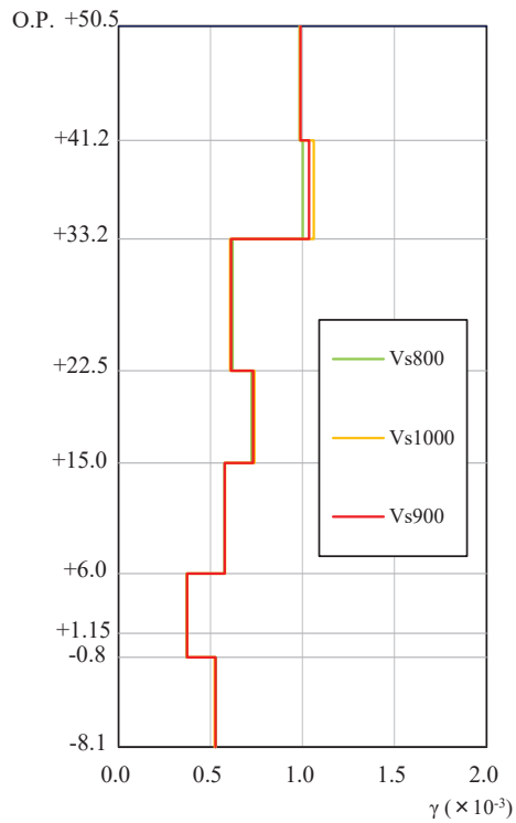
図 3-4 (1) 表層地盤下部のせん断波速度を変化させた場合の 最大応答せん断ひずみの比較 (Vs=800m/s~1000m/s, 基準地震動 S s - D 2, NS 方向)
