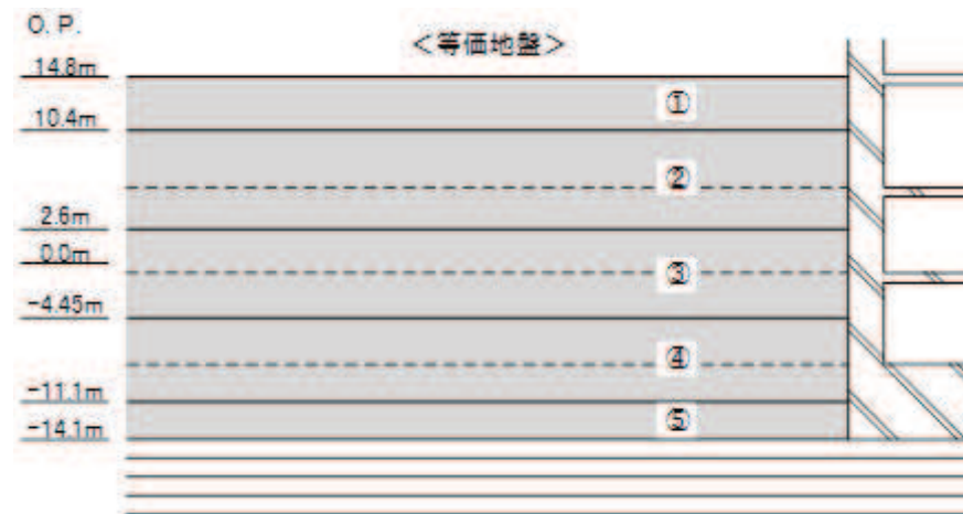
埋戻し土の形状
