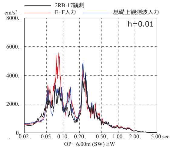
図 3-6 3.11 地震のはざとり波を入力に用いた場合と 基礎版上観測記録を用いたシミュレーション解析結果の比較 (原子炉建屋, EW 方向, 減衰 1%)
