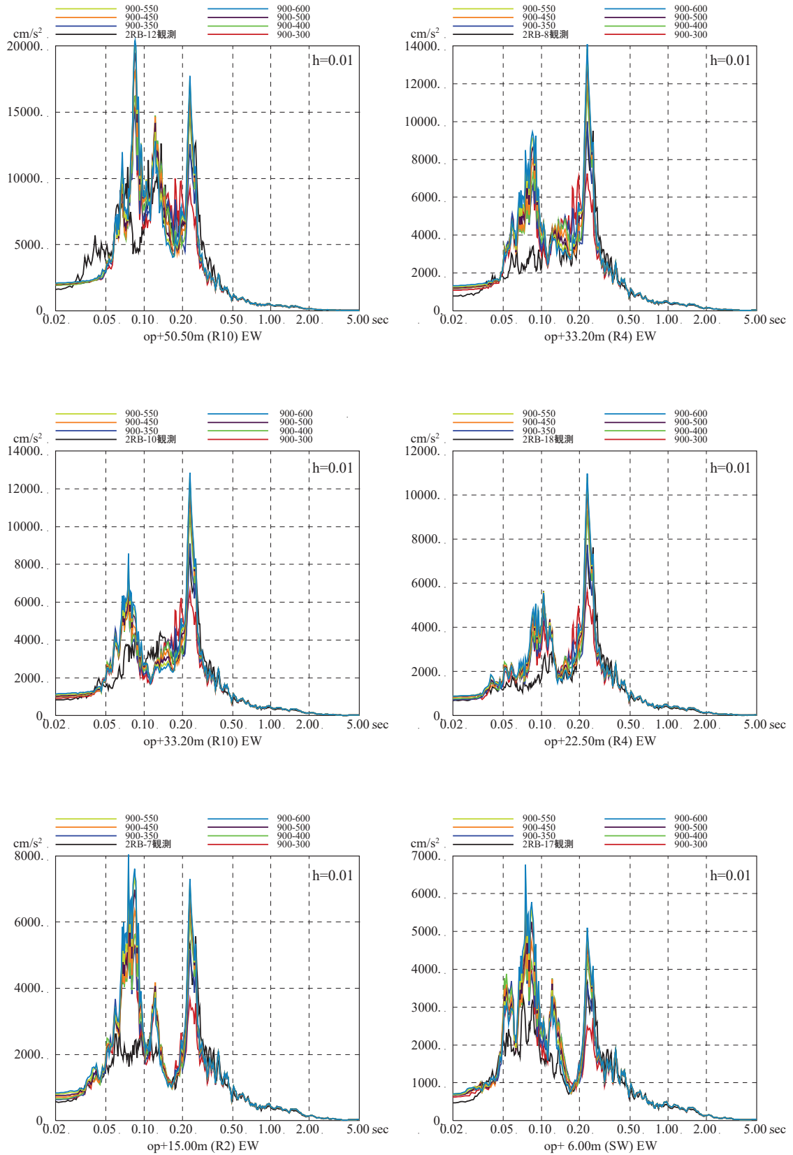
図 3-2 (4) 表層地盤上部の地盤物性の検討結果
