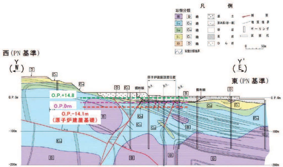
(b) 東西断面 (Y - Y')
