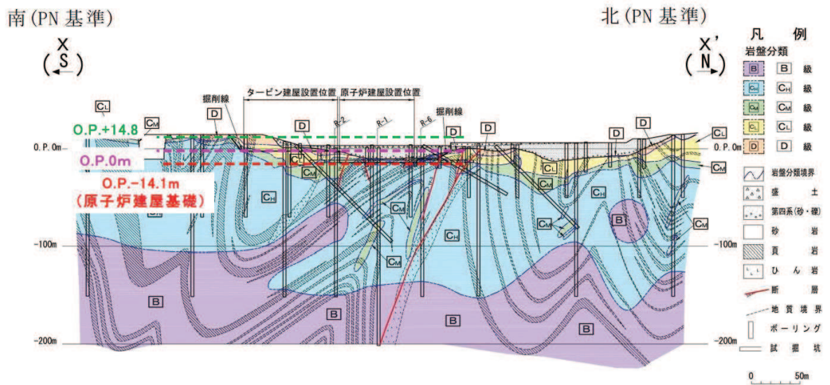
(a) 南北断面 (X - X')
