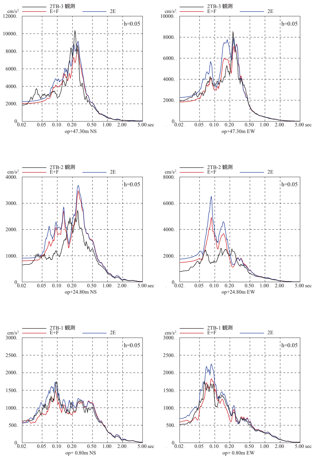
図 5-5 3.11 地震のはざとり波を用いたシミュレーション解析結果の比較 (タービン建屋)
