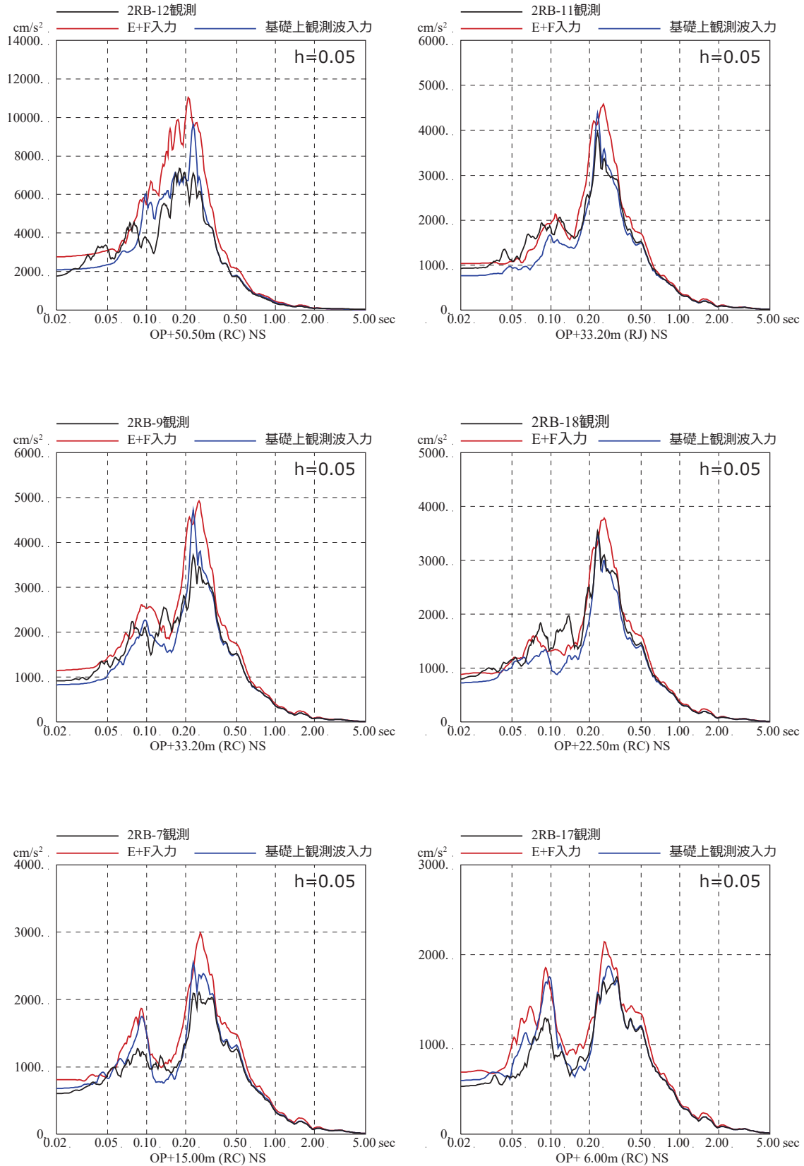
図 3-3 3.11 地震のはざとり波を入力に用いた場合と 基礎版上観測記録を用いたシミュレーション解析結果の比較 (原子炉建屋, NS 方向, 減衰 5%)
