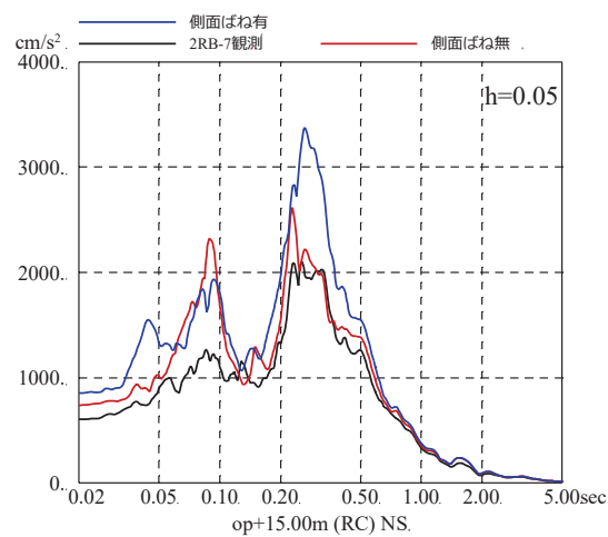
図 4-50 3.11 地震のはざとり波を用いた側面地盤ばねの有無による シミュレーション解析結果の比較 (原子炉建屋, NS 方向)
