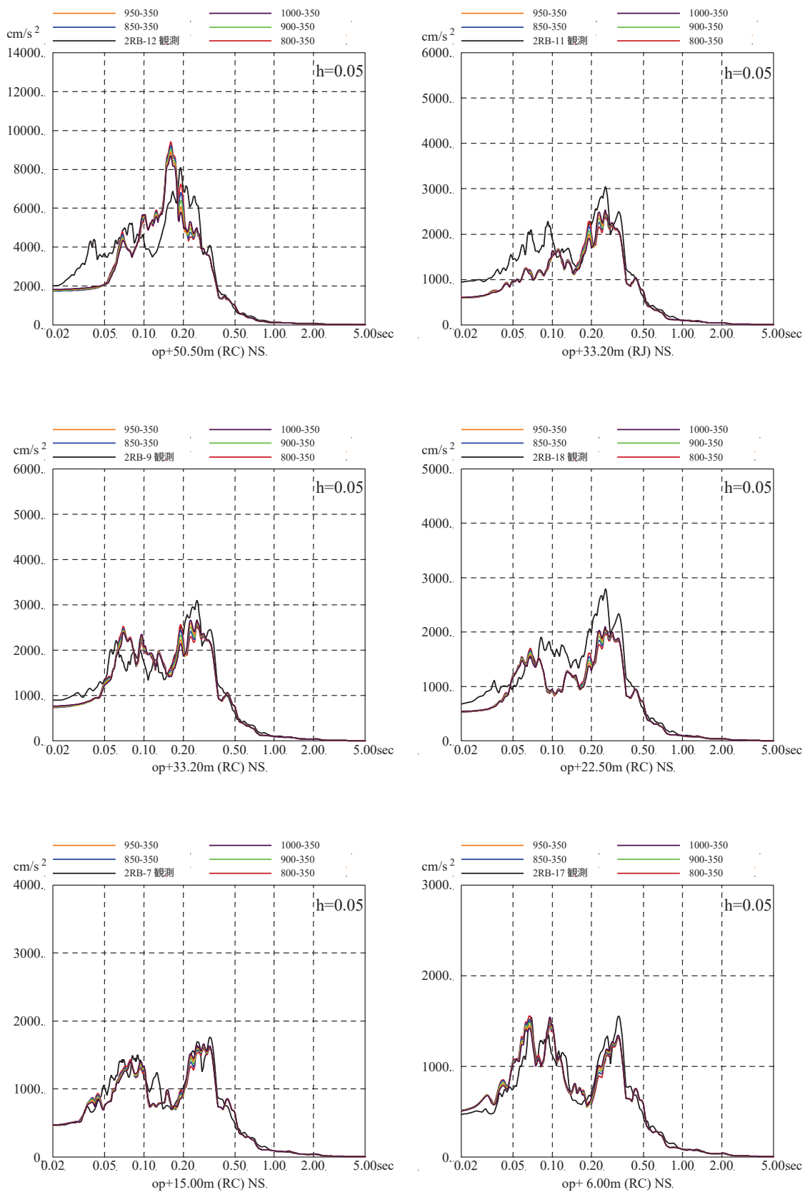
図 3-2 (5) 表層地盤下部の地盤物性の検討結果 (床応答スペクトルの比較) (4.7地震, NS方向, 減衰5%)
