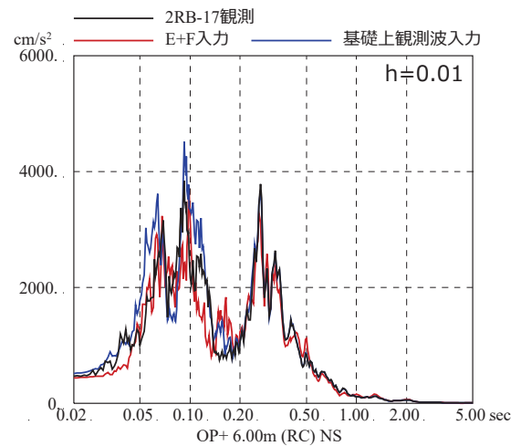
図 3-8 4.7 地震のはぎとり波を入力に用いた場合と 基礎版上観測記録を用いたシミュレーション解析結果の比較 (原子炉建屋, NS 方向, 減衰 1%)
