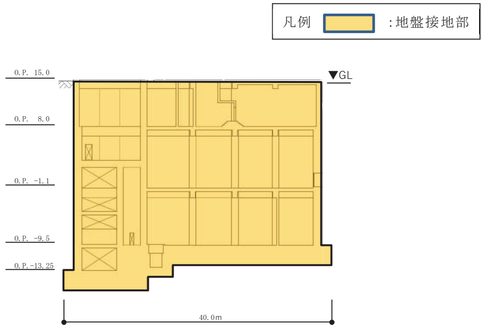
図5-1 第3号機海水熱交換器建屋（北面）の地盤の接地状況
