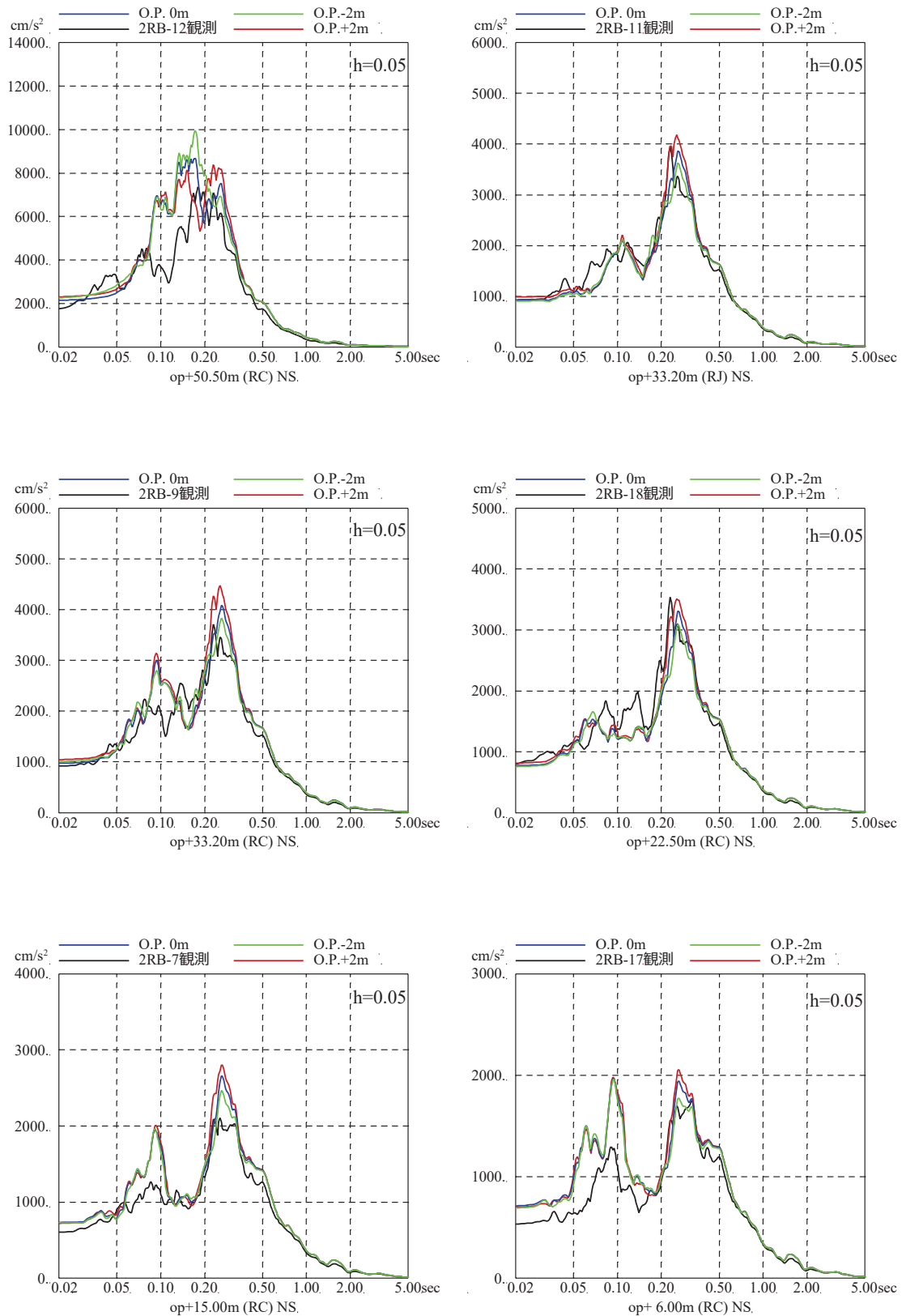
図 3-2 (1) 表層地盤の層境界に関する検討結果 (床応答スペクトルの比較)
