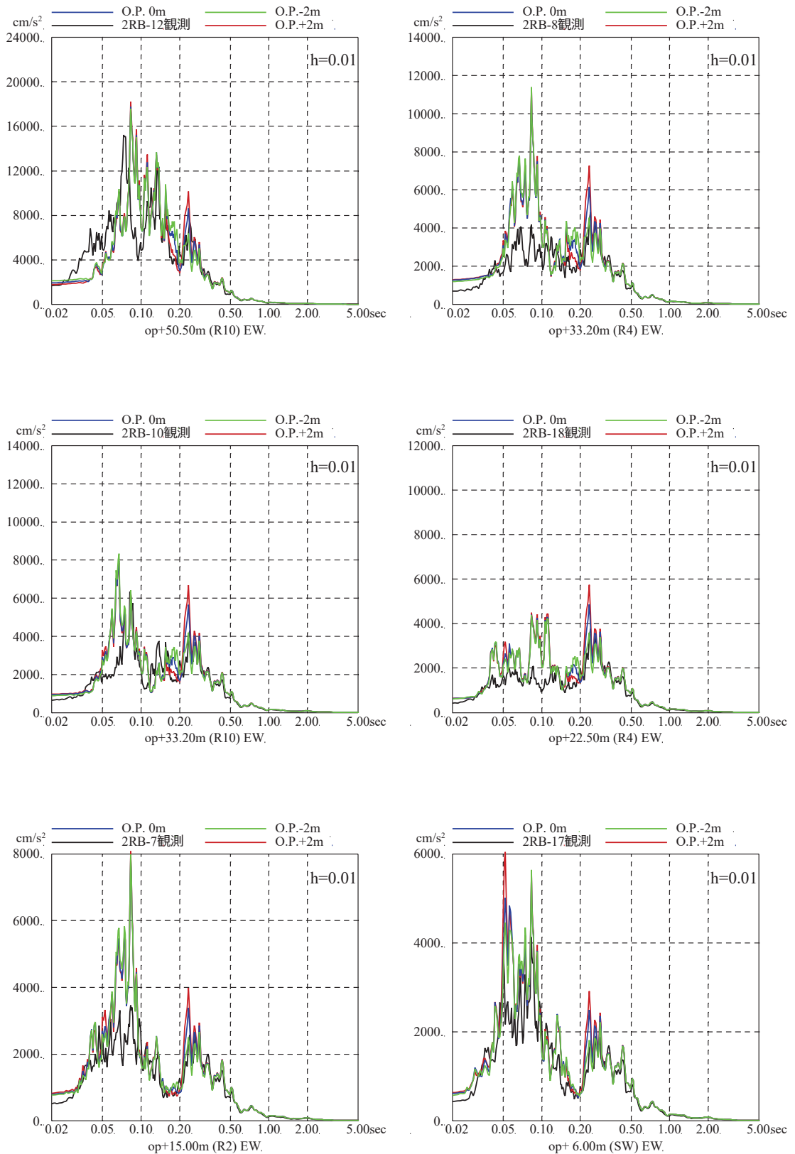
図 3-2 (8) 表層地盤の層境界に関する検討結果 (床応答スペクトルの比較)
