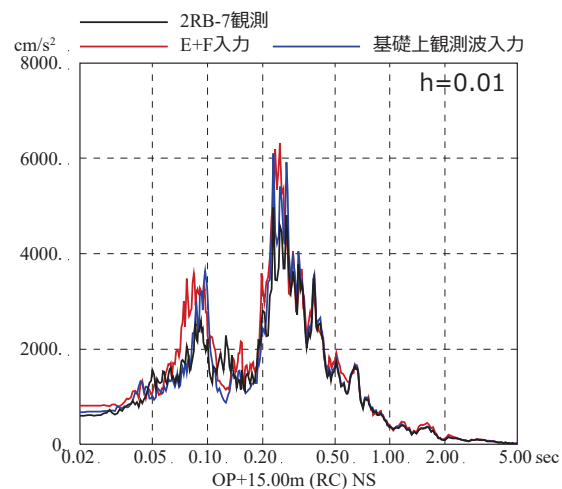
図 3-4 3.11 地震のはぎとり波を入力に用いた場合と 基礎版上観測記録を用いたシミュレーション解析結果の比較 (原子炉建屋, NS 方向, 減衰 1%)
