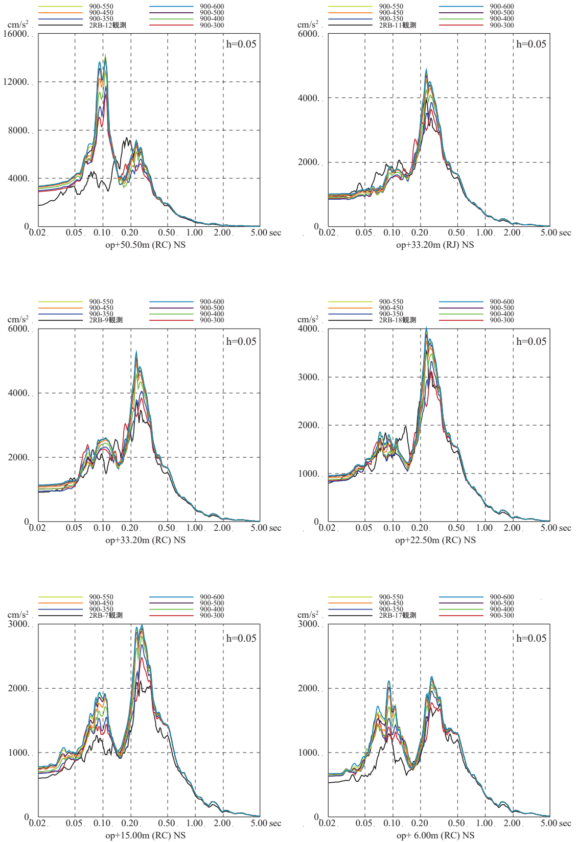
図 3-2 (1) 表層地盤上部の地盤物性の検討結果
