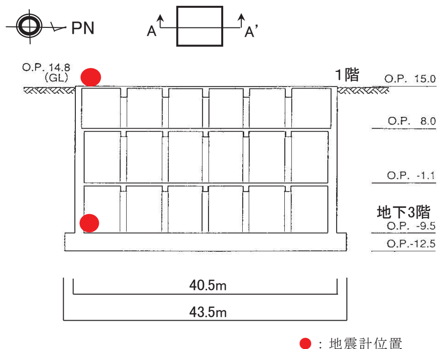
図4-51 第3号機海水熱交換器建屋の概要（A-A'）
