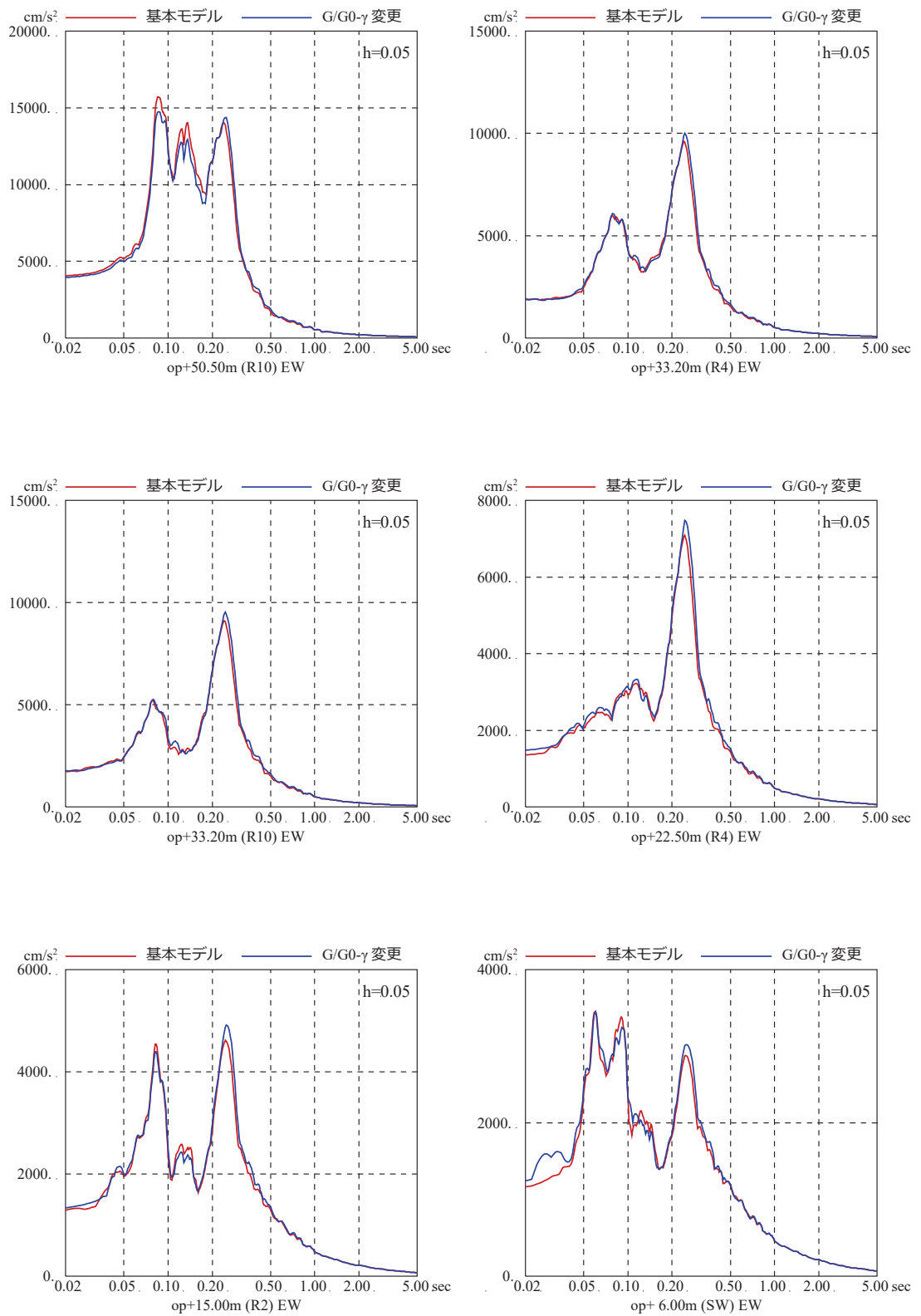
図-4 表層地盤の非線形特性を変えた場合の 床応答スペクトルの比較 (基準地震動 S s - D 2, EW 方向) (G/G 0 -γ 曲線のみ変更した場合)
