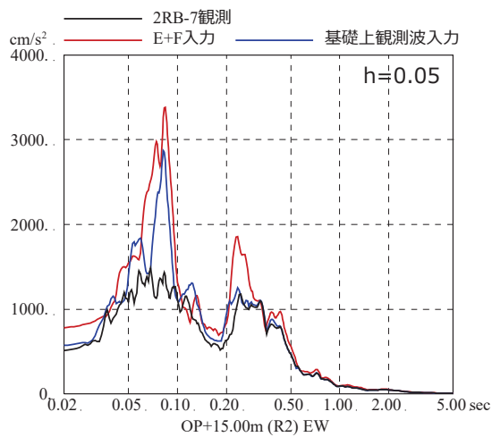
図 3-9 4.7 地震のはざとり波を入力に用いた場合と 基礎版上観測記録を用いたシミュレーション解析結果の比較 (原子炉建屋, EW 方向, 減衰 5%)
