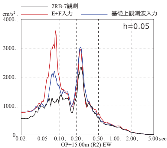
図 3-5 3.11 地震のはざとり波を入力に用いた場合と 基礎版上観測記録を用いたシミュレーション解析結果の比較 (原子炉建屋, EW 方向, 減衰 5%)
