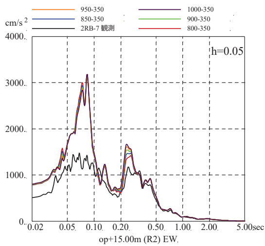
図 3-2 (6) 表層地盤下部の地盤物性の検討結果 (床応答スペクトルの比較) (4.7 地震, EW 方向, 減衰 5%)
