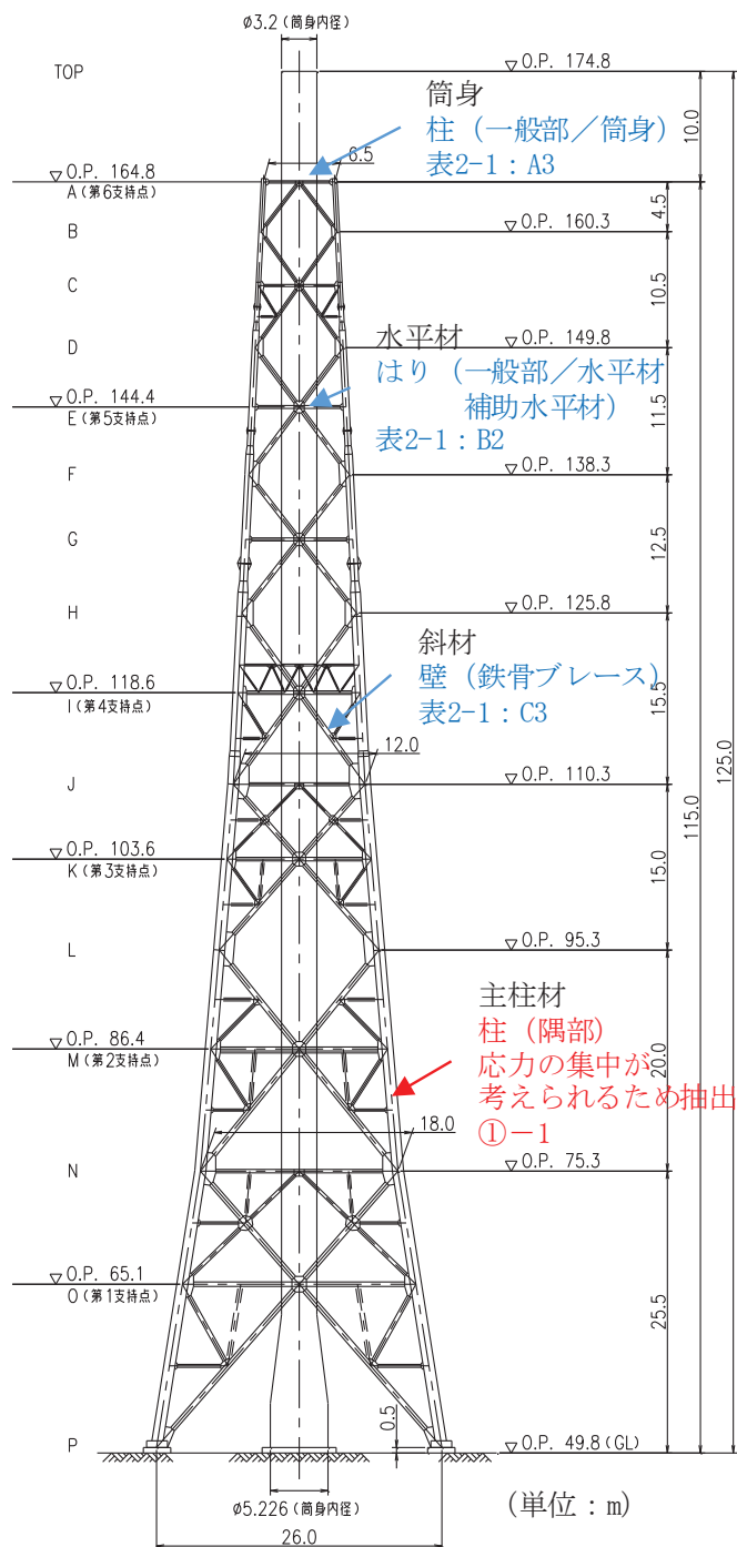
図2-10-1 第1号機排気筒の概要図
