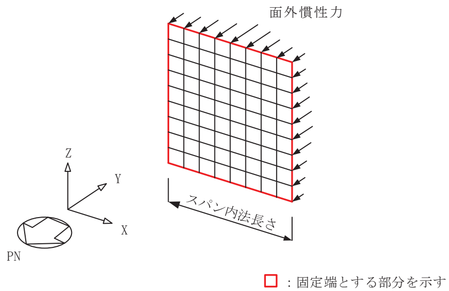
図 2-16 解析モデル
