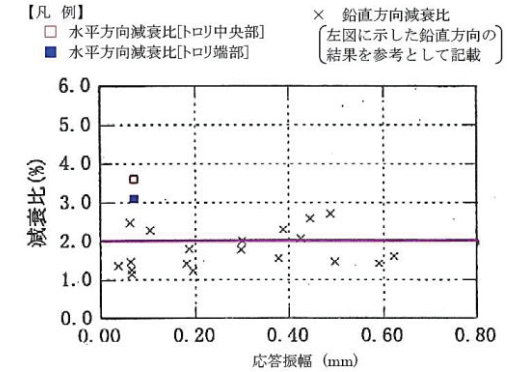
燃料取替機の減衰比と応答振幅の関係（水平方向） 燃料取替機の減衰比と応答振幅の関係（水平方向）
