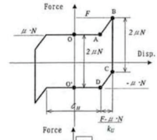
変位-荷重履歴のモデル
