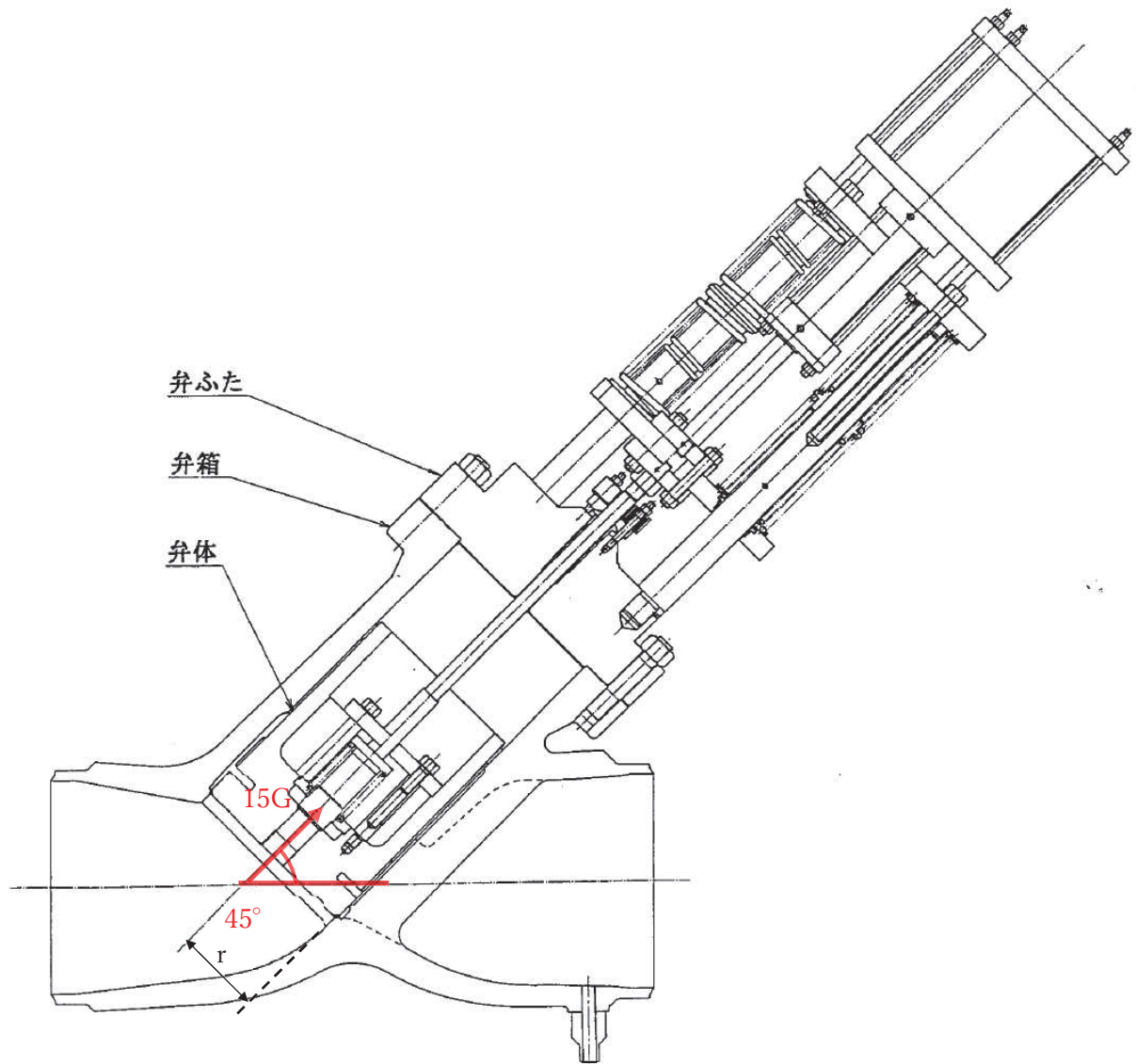
添付 8-7 図 主蒸気系境界弁構造図
