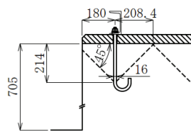
(引張時) X-X' 矢視図
