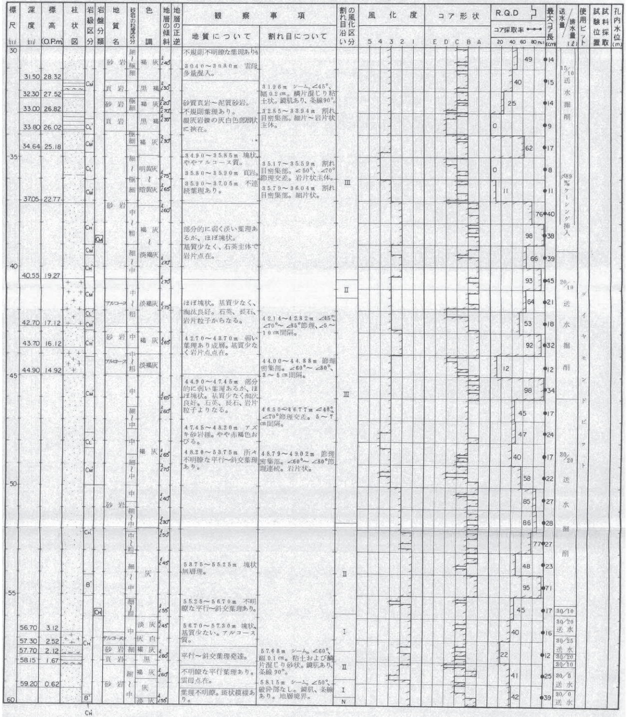
図 2-5(3) ボーリング柱状図 (3Rs-7) (深度 30~60m)
