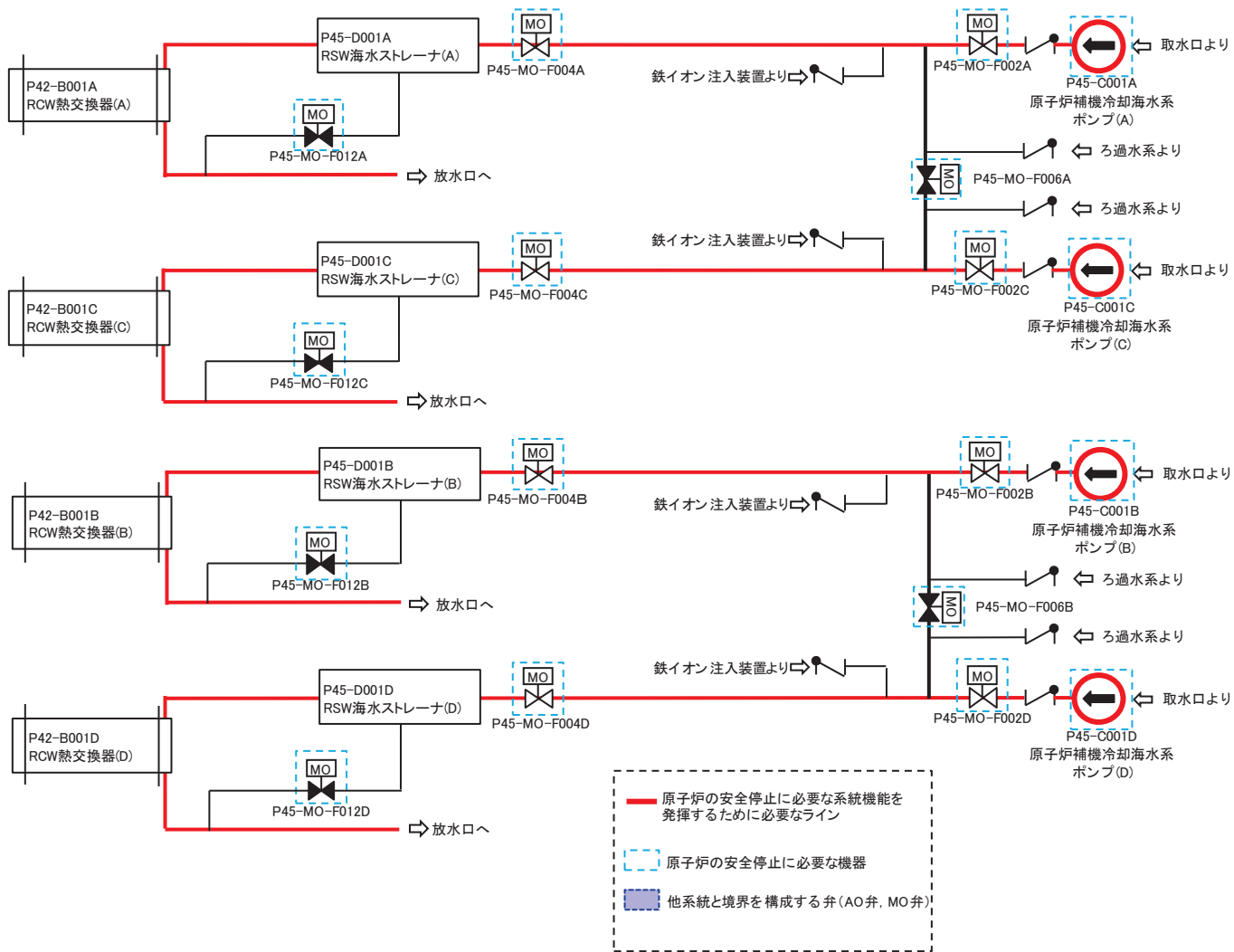
図 9 原子炉補機冷却海水系
