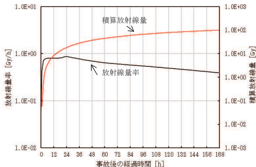
図 重大事故時における原子炉建屋原子炉棟内の放射線量率及び積算放射線量の経時変化
