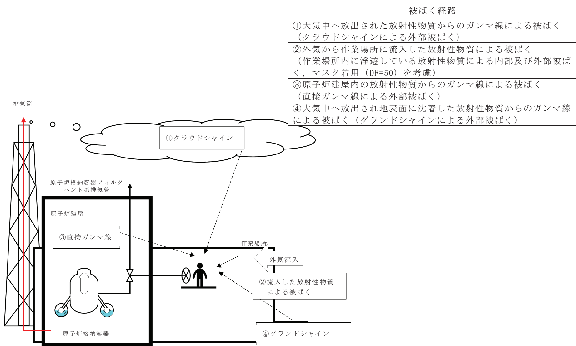
図 6-6 ベント操作に係る作業時の被ばく評価経路イメージ (屋内移動時及び原子炉格納容器第二隔離弁開操作時)
