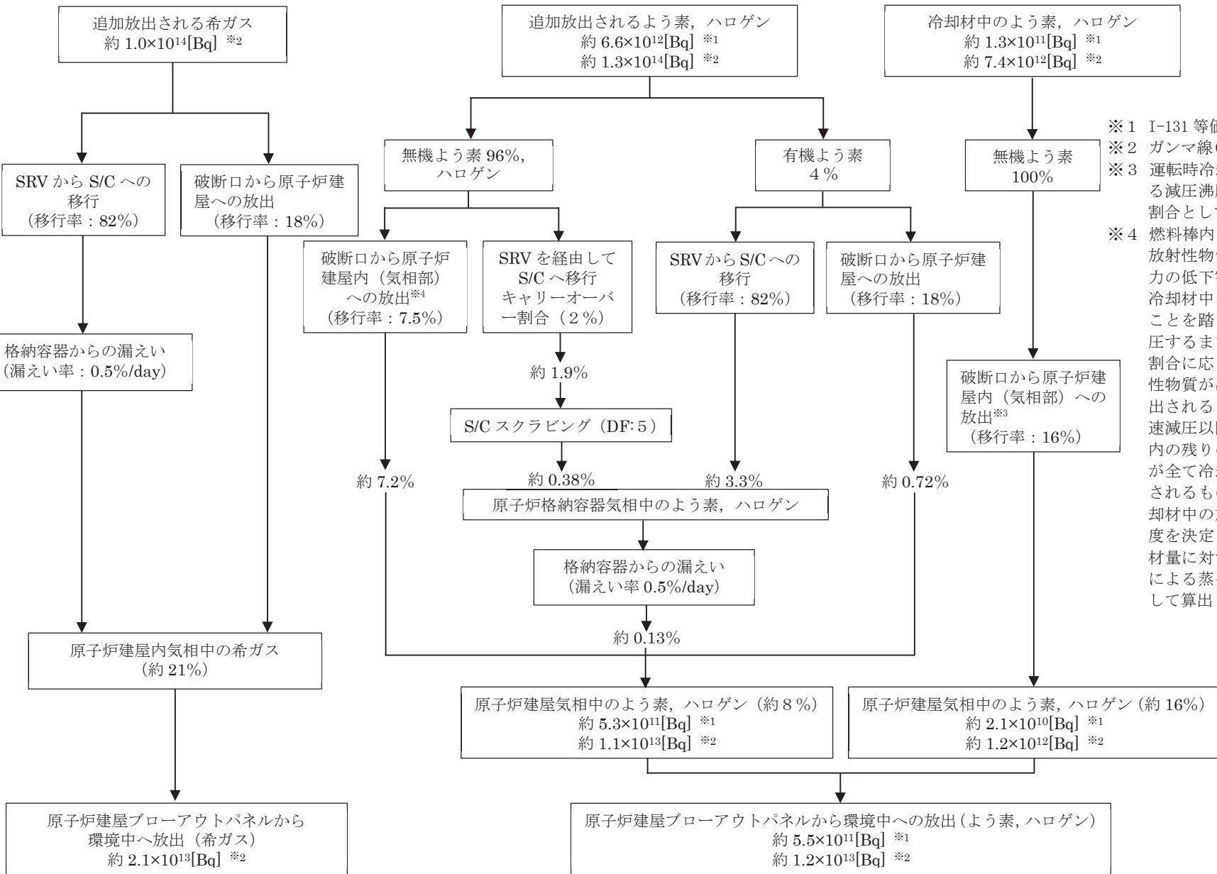
図 12 核分裂生成物の環境中への放出について (インターフェイスシステム LCA 時)
