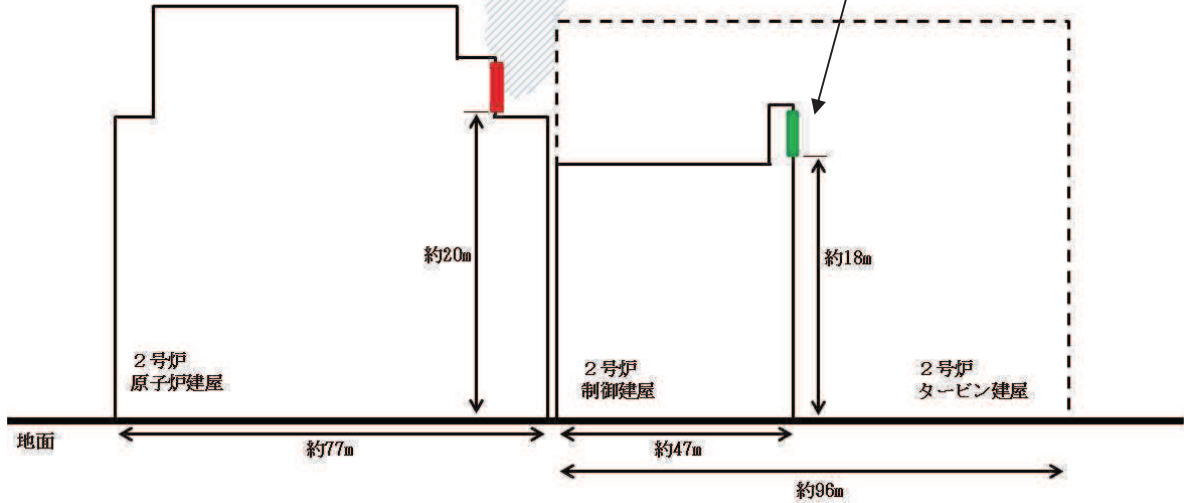
(b) 断面図
