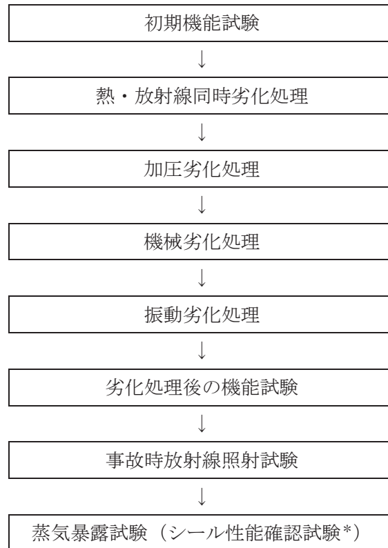
図4 試験手順
