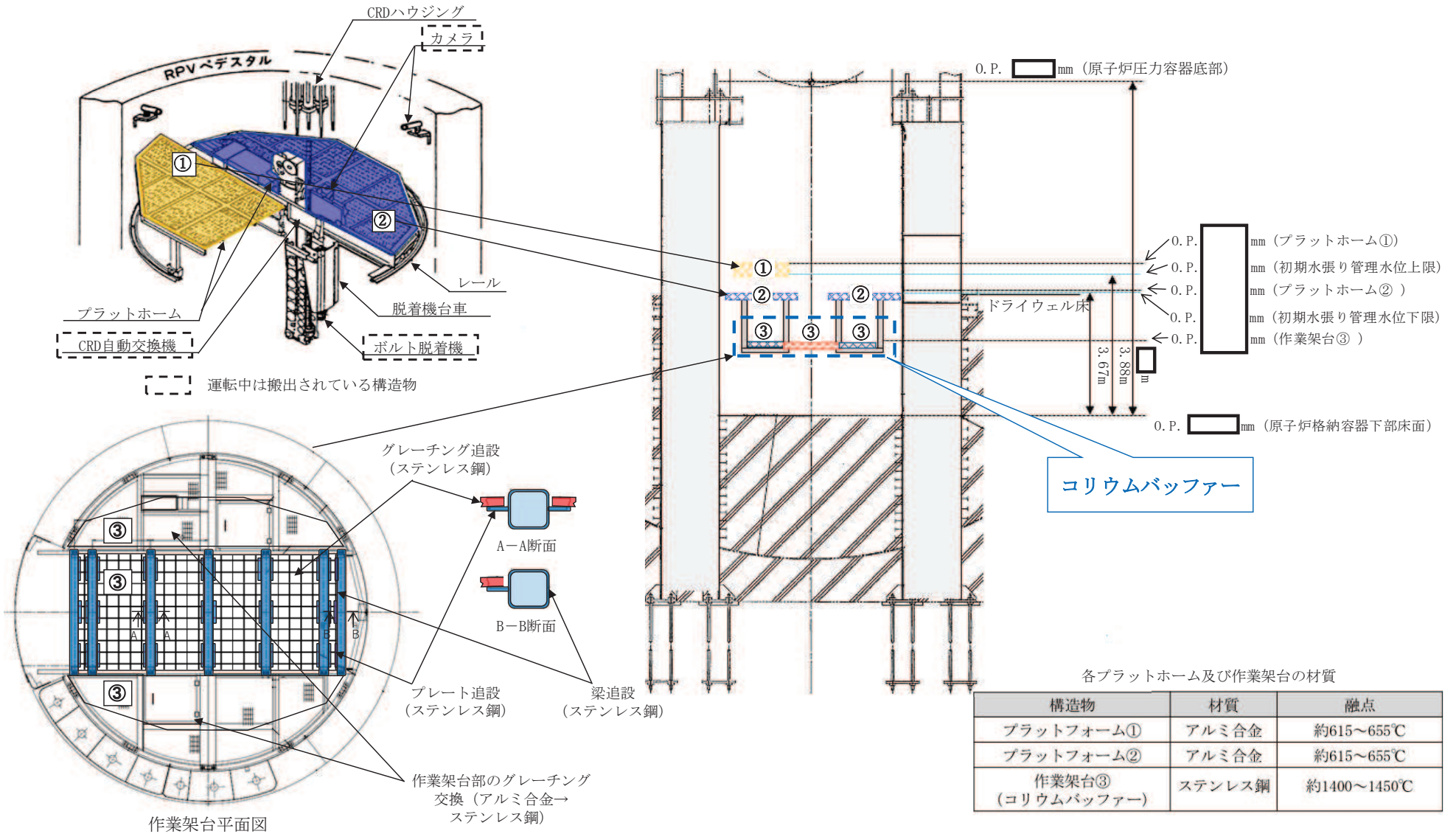
図1 コリウムバッファーの構造
