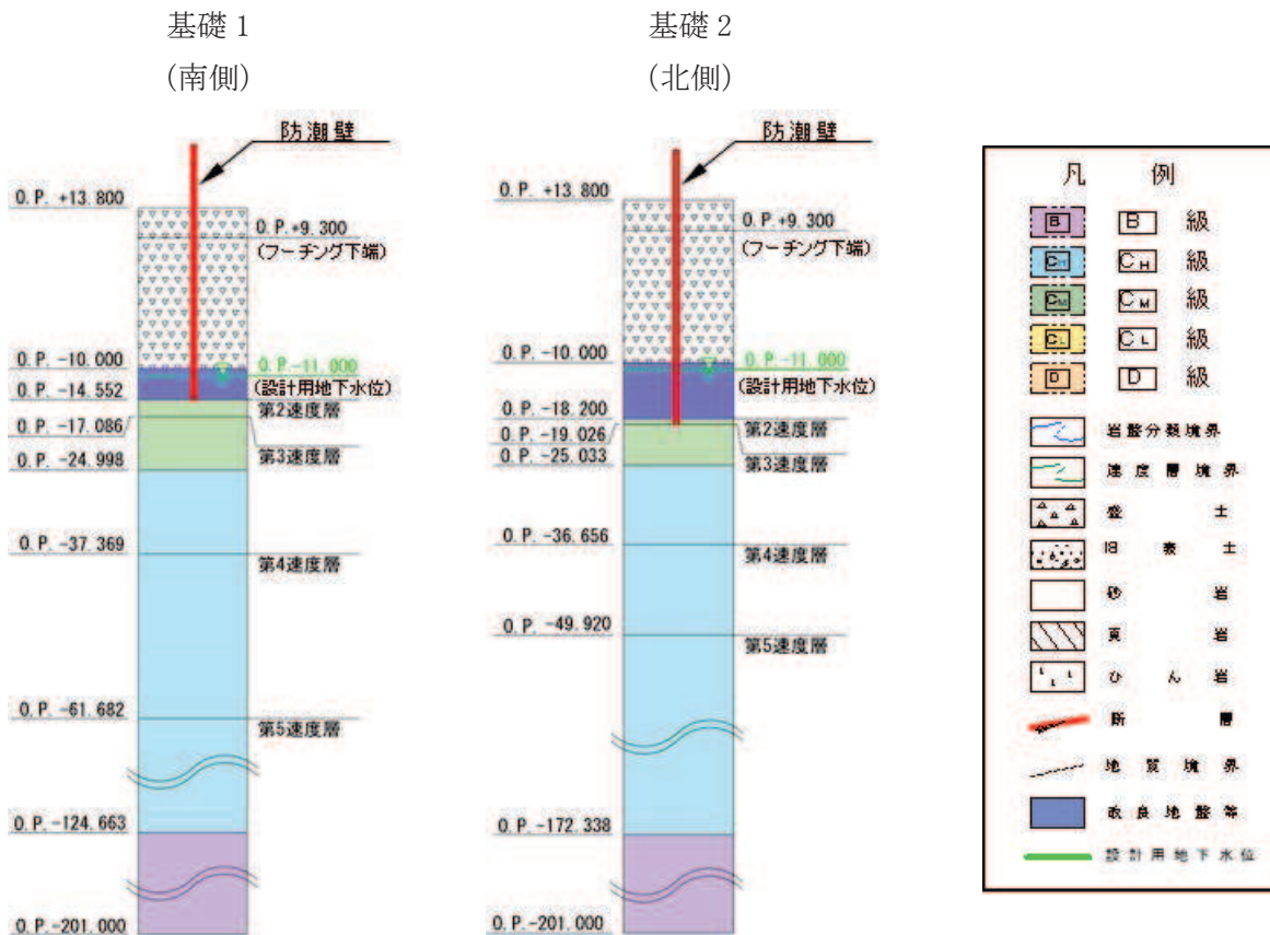
図 3.1-2(4) 評価対象断面の地層構成図 (鋼桁 4) (単位: m)
