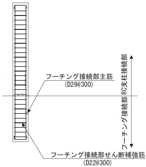
(3-3 断面 (接続部))
