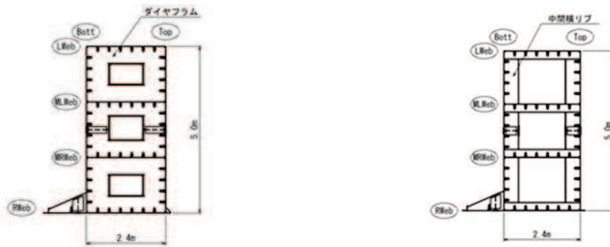
図 2.2-4(4) 鋼製遮水壁（鋼桁 1） 鋼桁構造図（底面図）
