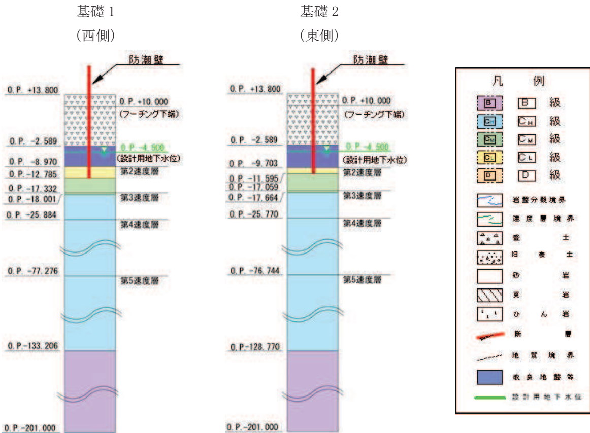
図 3.1-2(2) 評価対象断面の地層構成図 (鋼桁 2) (単位 : m)
