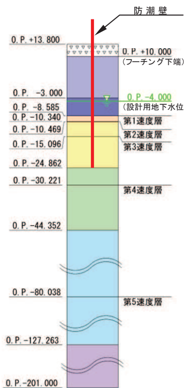
図 3.1-2(5) 評価対象断面の地層構成図 (鋼桁 5) (単位: m)
