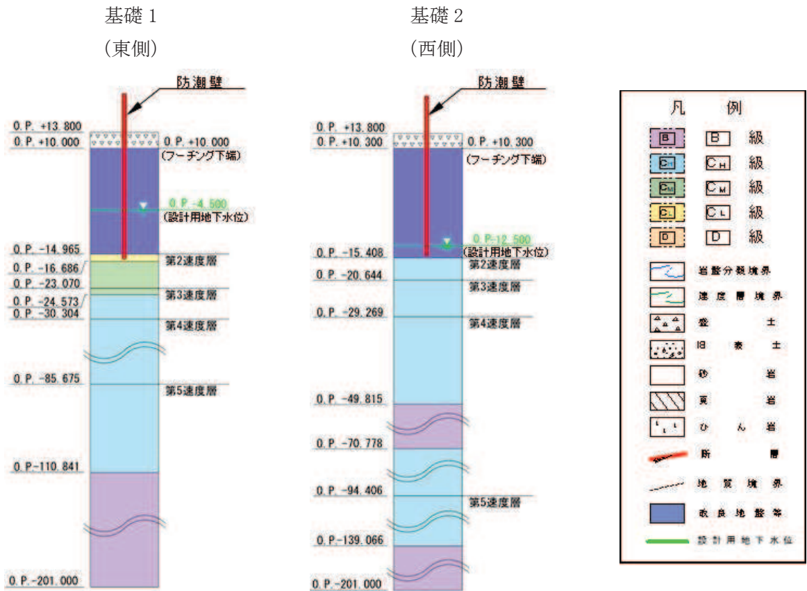
図 3.1-2(1) 評価対象断面の地層構成図 (鋼桁 1) (単位 : m)
