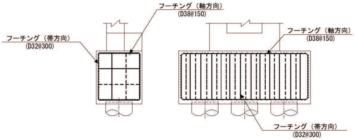
(1-1 断面)
