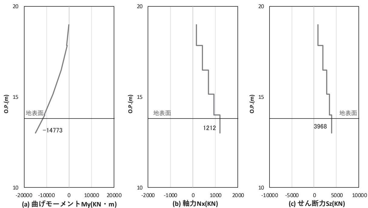
図 4.1-18(1) コンクリートの曲げ・軸力系の破壊に対する照査における 曲げモーメント最大時刻での断面力 (鋼桁 3 : 基礎 2, S_s - D_2 (+-), 桁軸方向加振時, t = 23.98s ) 解析ケース③ : 地盤物性のばらつき ( -1\sigma ) を考慮した解析ケース
