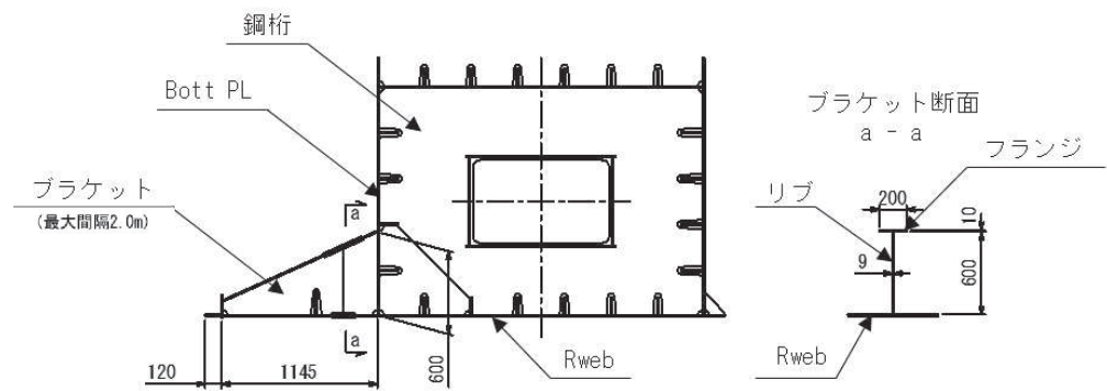
図 2.2-7(5) 鋼製遮水壁（鋼桁 4） 鋼桁構造図（断面図）
