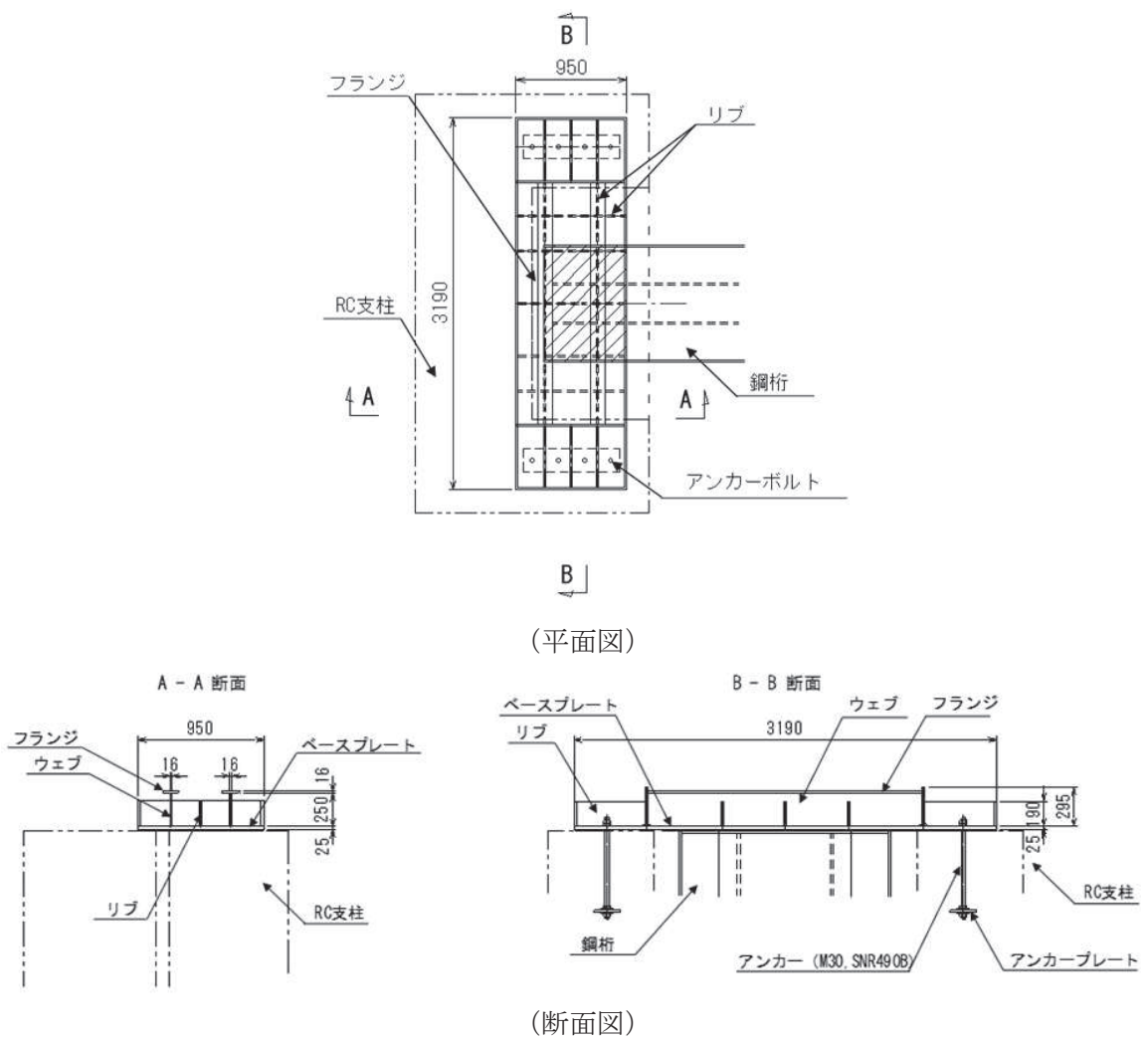
図 2.2-9(5) 鋼製遮水壁 (鋼桁 6) 上揚力反力梁
