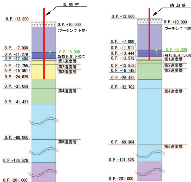
図 3.1-2(6) 評価対象断面の地層構成図 (鋼桁 6) (単位: m)
