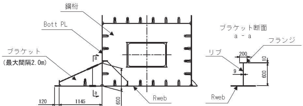
図 2.2-4(5) 鋼製遮水壁（鋼桁 1） 鋼桁構造図（断面図）
