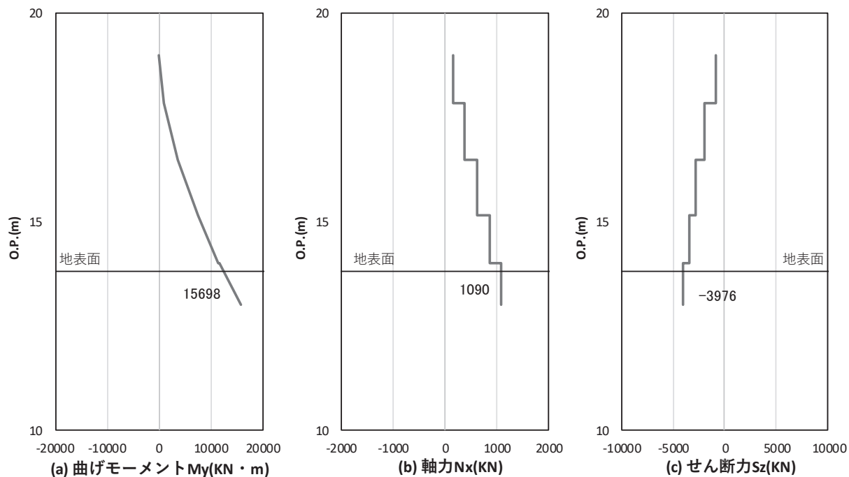
図 4.1-18(2) 鉄筋の曲げ・軸力系の破壊に対する照査における 曲げモーメント最大時刻での断面力 (鋼桁 3 : 基礎 2, S_s - D_2 (—), 桁軸方向加振時, t = 23.98s ) 解析ケース③ : 地盤物性のばらつき ( -1\sigma ) を考慮した解析ケース
