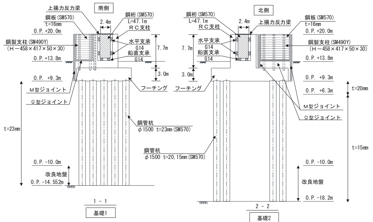
(断面図)
