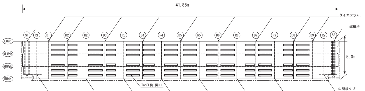
図 2.2-4(2) 鋼製遮水壁（鋼桁1） 平面図
