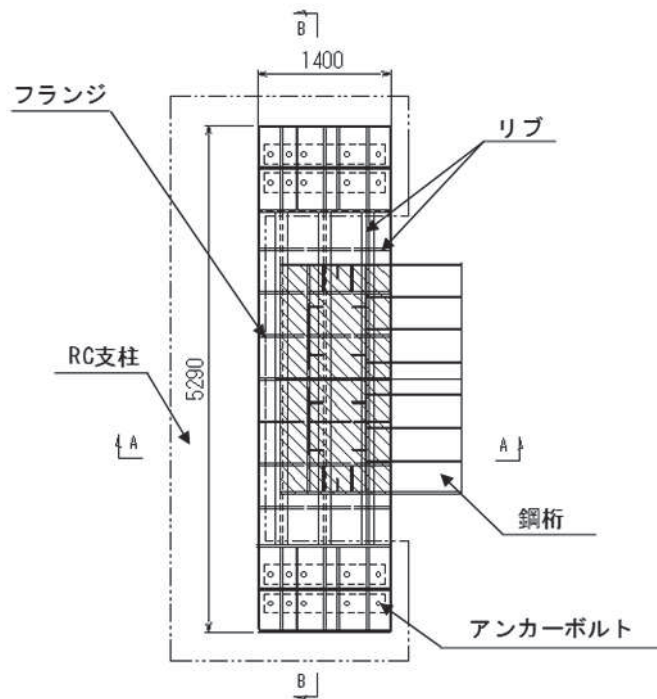
(平面図)
