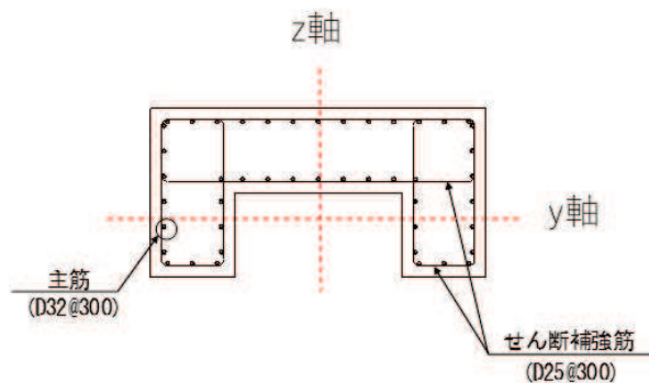
図 4.1-15 RC 支柱の配筋概要図 (鋼桁 2 の例)
