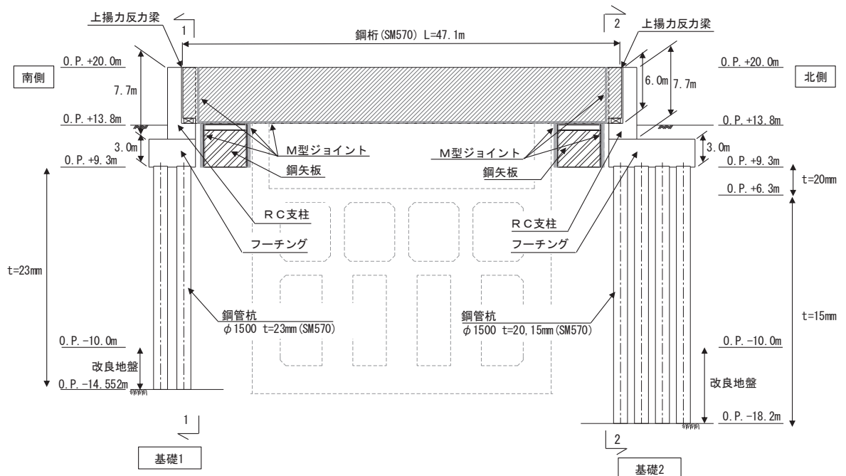
(正面図)
