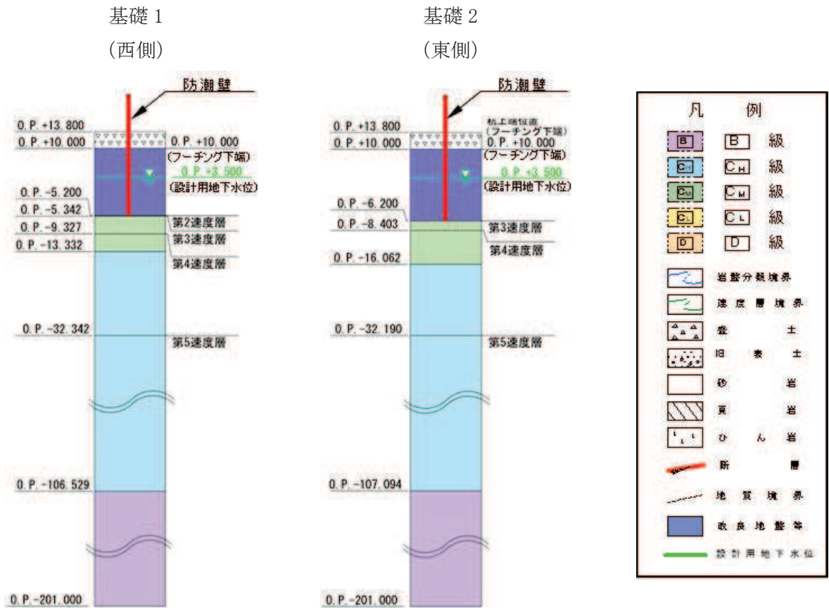
図 3.1-2(3) 評価対象断面の地層構成図 (鋼桁 3) (単位: m)
