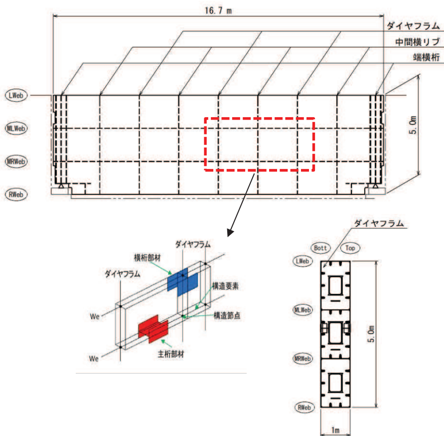
図 3.7-1 鋼桁詳細図
