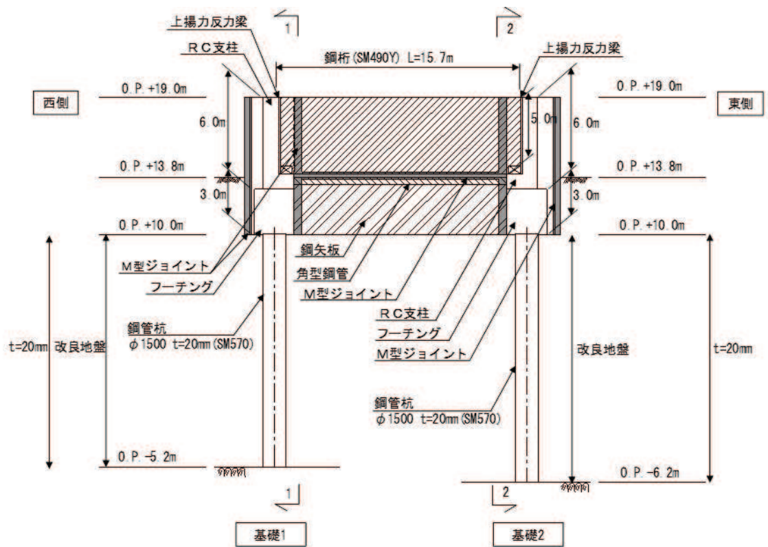
(正面図)
