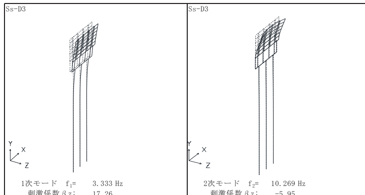
図 3.2-5(1) 固有値解析結果 (断面② : モード図)
