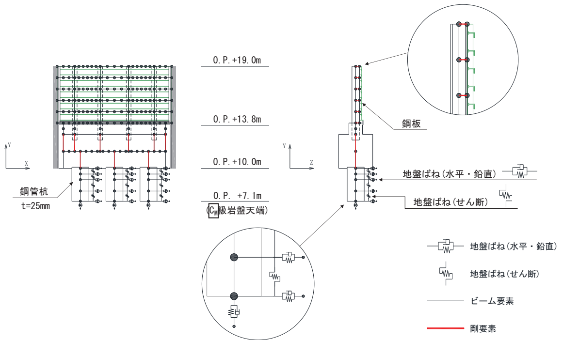
図 3.5-6 解析モデル (断面⑥)
