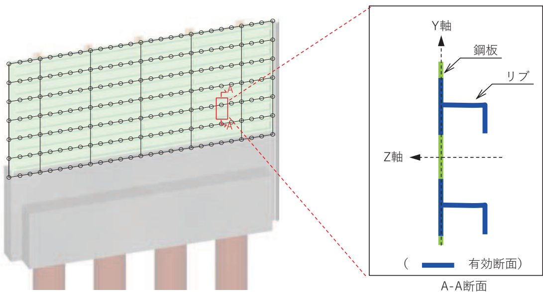
図 3.8-2 鋼板断面形状
