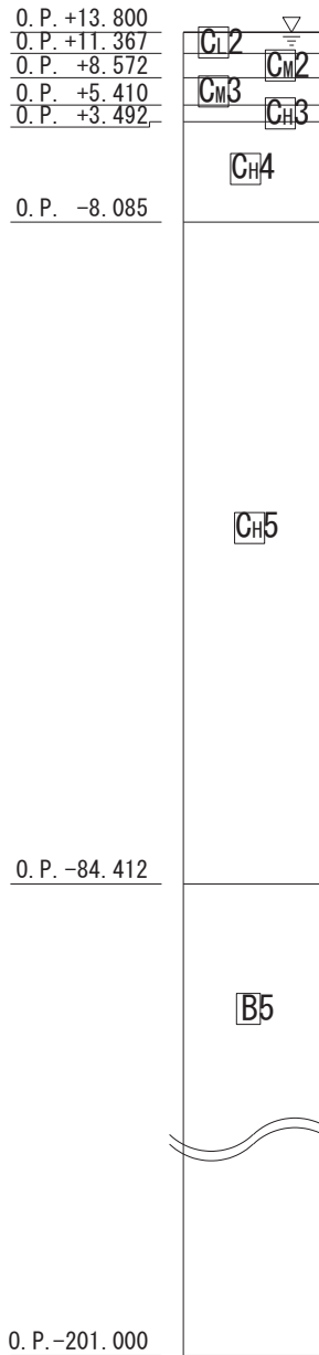
図 3.3-1(2) 入力地震動算定の概念図（引上げ地盤モデル）（単位：m）
