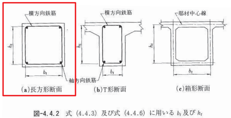
図 3.8-3 ねじりによる応力度算出に用いる b_t 及び h_t (道路橋示方書 (I 共通編・III コンクリート橋編) ・同解説 (平成 24 年 3 月) より抜粋)
