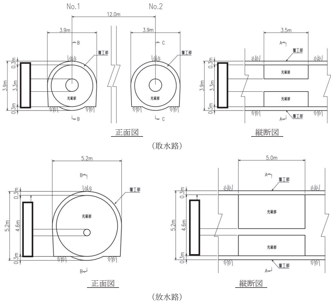
図 1-1 取放水路流路縮小工 構造概要図
