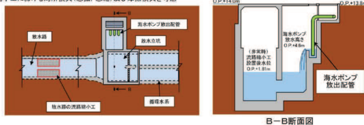
図 6.2.6-2(3) 第1号機の放水機能への影響確認結果(非常時)(2/2)
