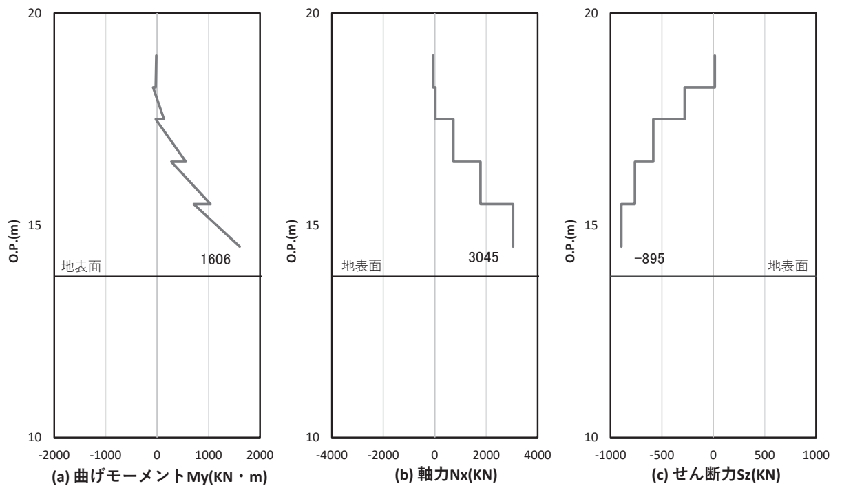
図 4.1-15(4) 鋼製支柱のせん断破壊に対する照査における照査時刻での断面力 (断面⑦張出部, S s - D 2 (++) , t = 26. 82s) 解析ケース③: 地盤物性のばらつき (-1σ) を考慮した解析ケース
