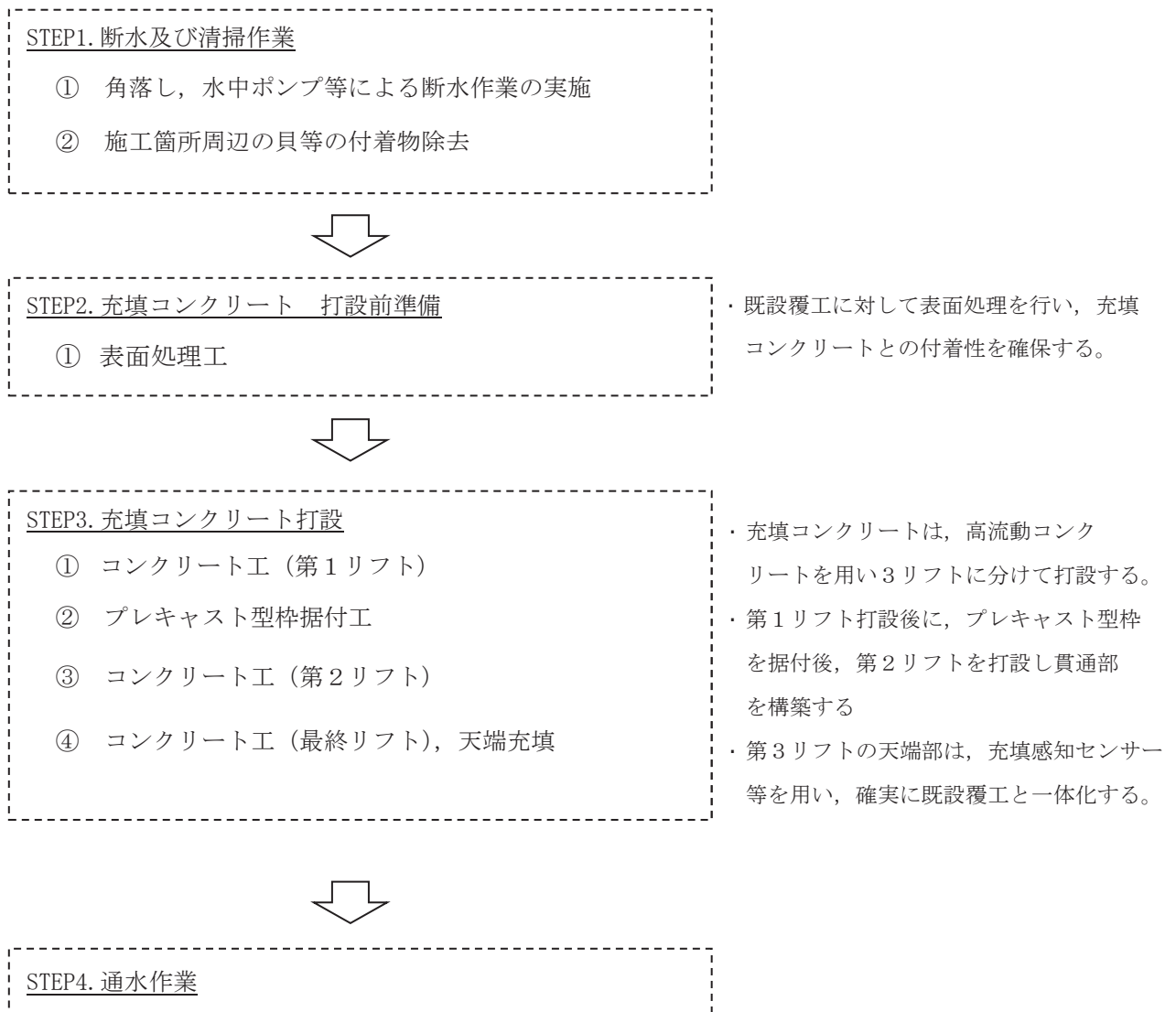
図5-1 取水路トンネル 施工フロー
