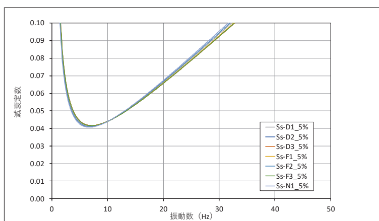
図 3.2-19(3) 設定した Rayleigh 減衰 (断面⑧) _減衰 5%
