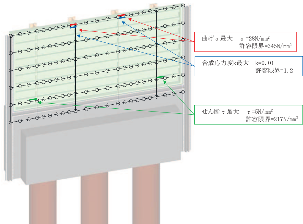
図 4.1-3 鋼板の曲げ・軸力系の破壊及びせん断破壊に対する 最大照査値発生個所 (断面③)
