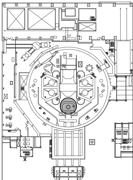
原子炉格納容器 E L. 39.0m
