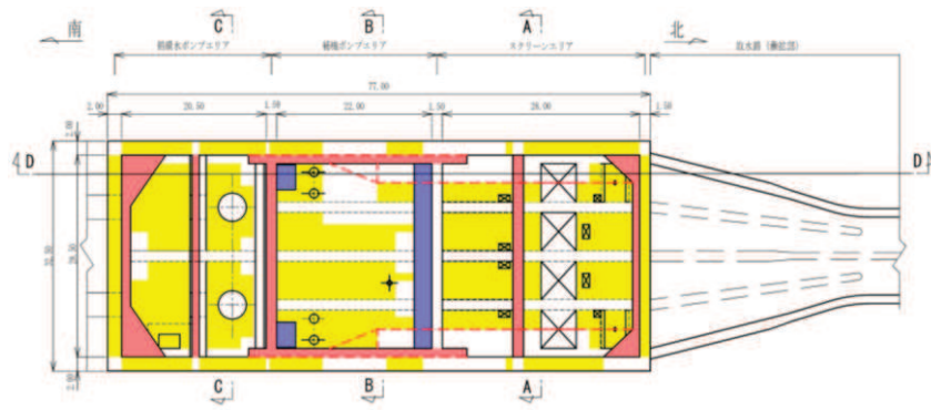
平面図
