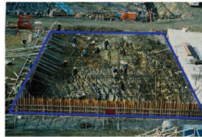
海水ポンプ室底盤写真
