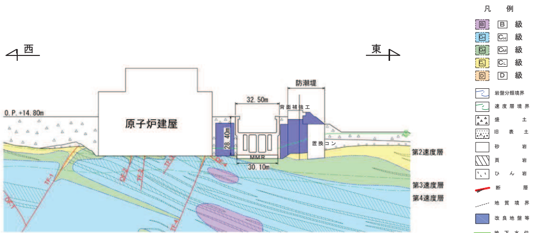
図 4.10-12(2) 海水ポンプ室 地震時荷重算出断面図 (東西方向：補機ポンプエリア)
