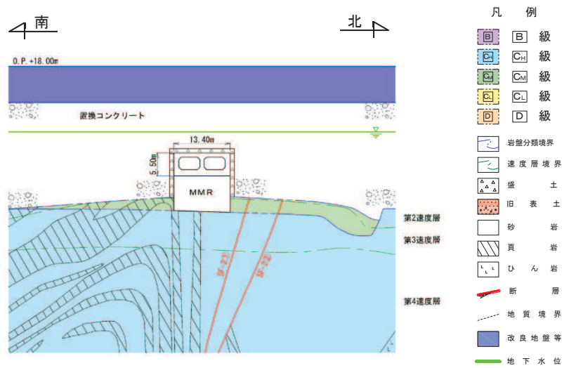
図 4.12-9 取水路（標準部）地質断面図（断面④）：直線部
