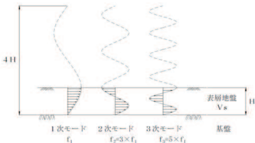
図 9.1-2 せん断振動の固有振動モード (実務に役立つ耐震設計入門（土木学会，2011））
