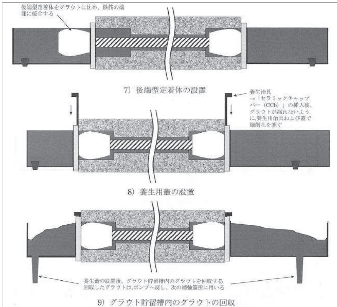
図Ⅱ-4.57 先充てん後挿入法（両端後端型）の施工手順（その3）
