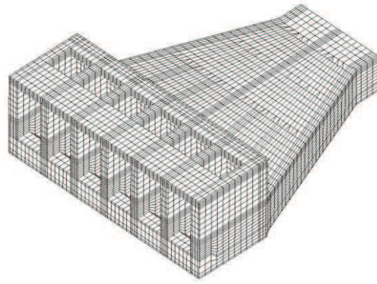
図 4.11-8 取水口，貯留堰 三次元モデル図
