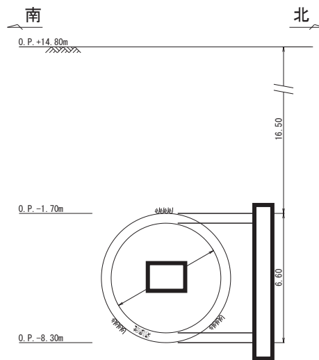
図 4.5-4 排気筒連絡ダクト断面図 (B-B 断面, 岩盤部)
