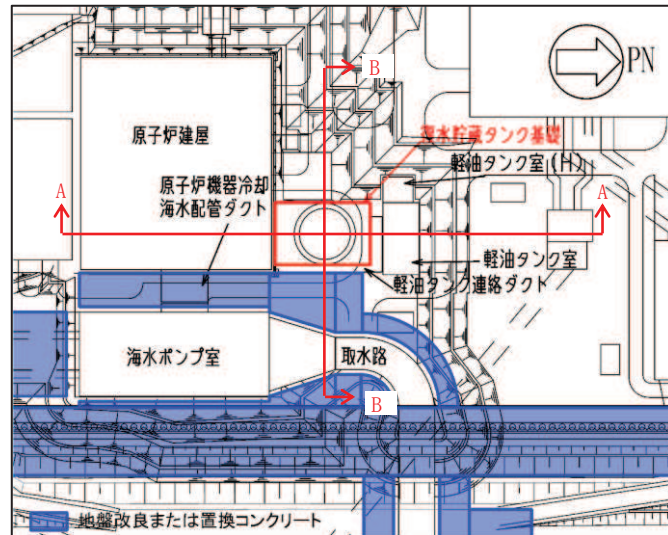
図 4.13-6 復水貯蔵タンク基礎掘削図
