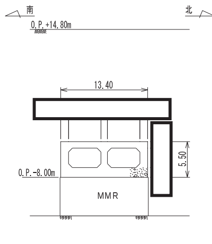
図 4.12-3 取水路（標準部）断面図（A-A 断面）
