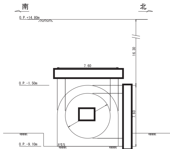
図 4.5-3 排気筒連絡ダクト断面図 (A-A 断面, 土砂部)
