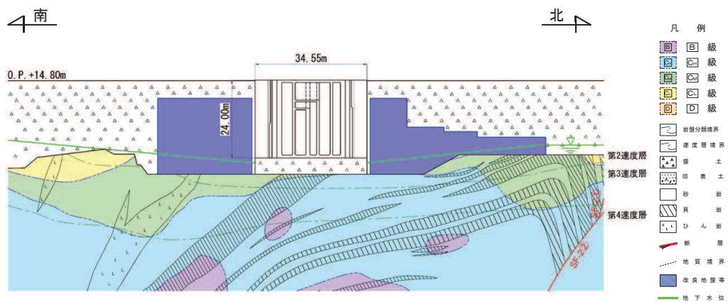
図 4.6-10 原子炉機器冷却海水配管ダクト（鉛直部）地質断面図（A-A 断面）
