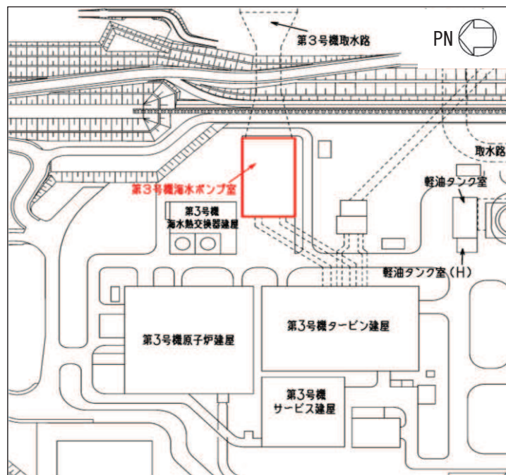
図4.15-1 第3号機海水ポンプ室配置図
