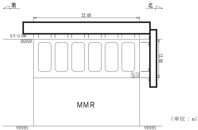
図11.2-7 取水口断面図 (A-A断面図, 標準部)
