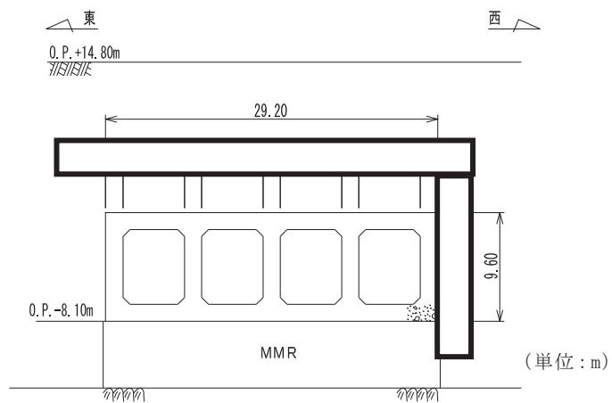
図 4.7-3 取水路（漸拡部）断面図（A-A 断面）
