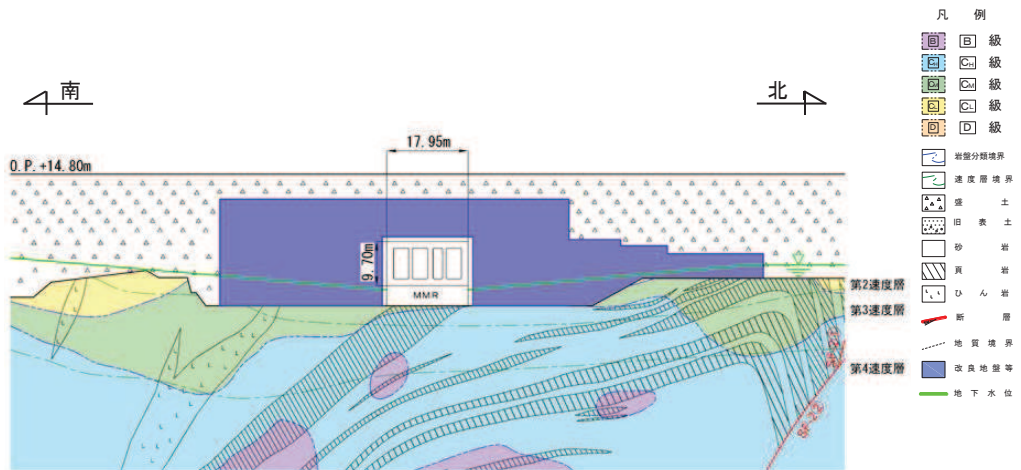
図 4.6-6 原子炉機器冷却海水配管ダクト（水平部）地質断面図（A-A 断面）
