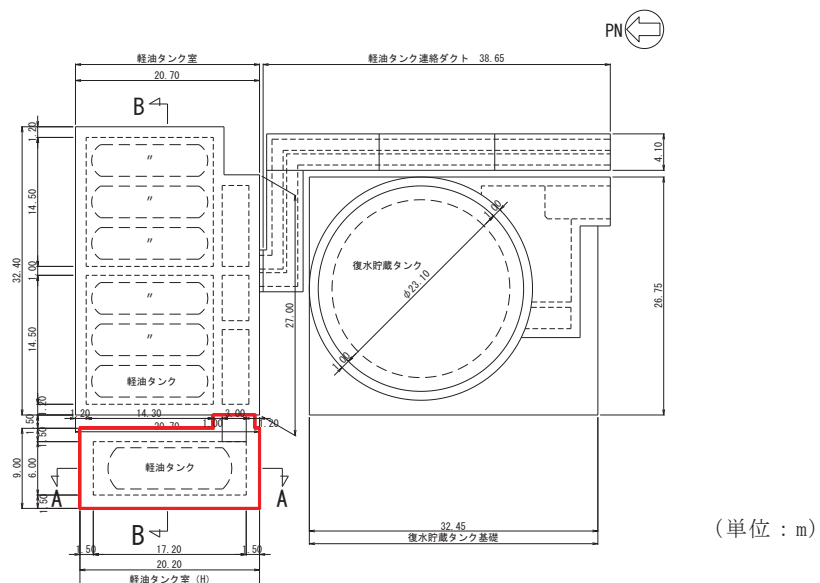
図 4.9-2 軽油タンク室 (H) 平面図
