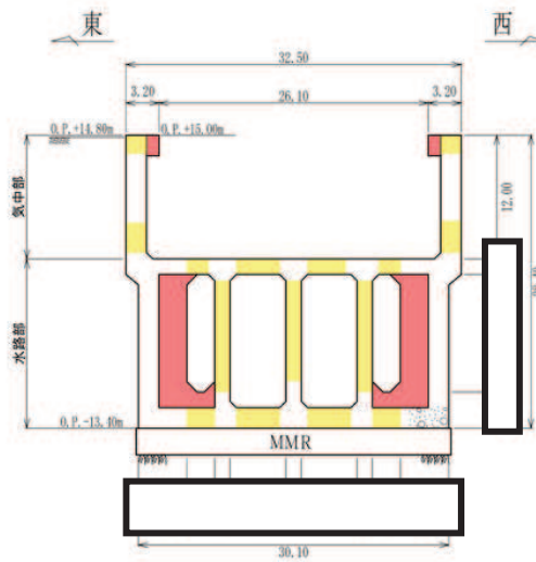
B-B 断面
