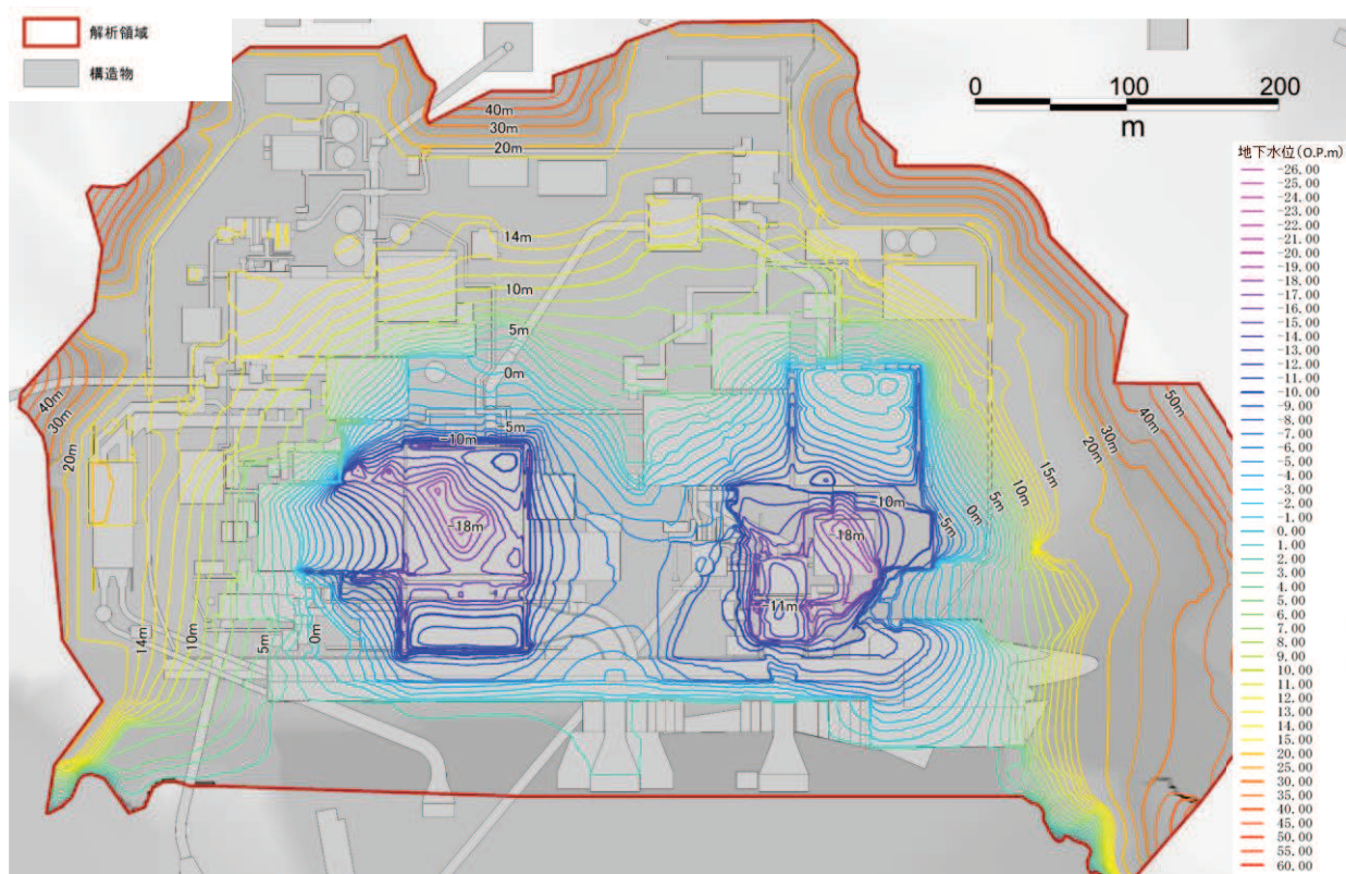
図 4.1-3 地下水水位コンター図
