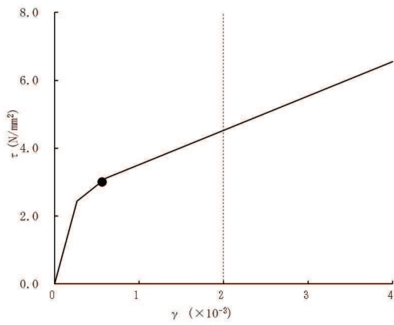
要素番号 (23)
