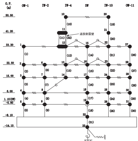
図 3-13(1) せん断スケルトンカーブ上の最大応答値 (EW 方向) (1/6)
