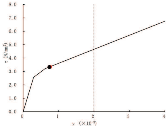
要素番号 (29)
