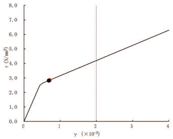
要素番号(19)
