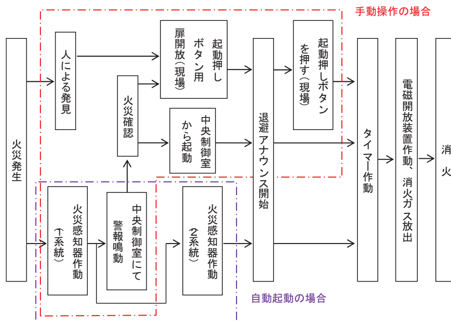
図13 火災時の信号の流れ（油内包機器）
