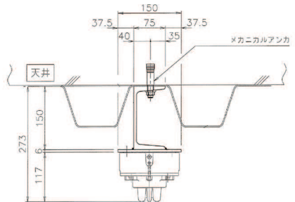
図 3-8 防爆型熱感知器の取付方法
