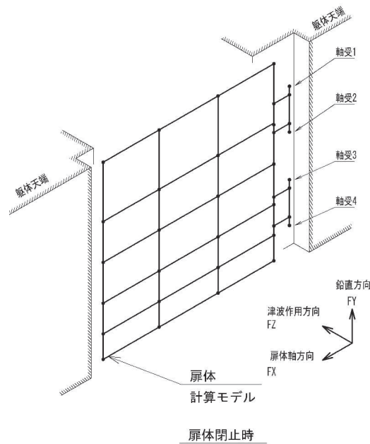
図 3.8-5 扉体の評価モデル概要図
