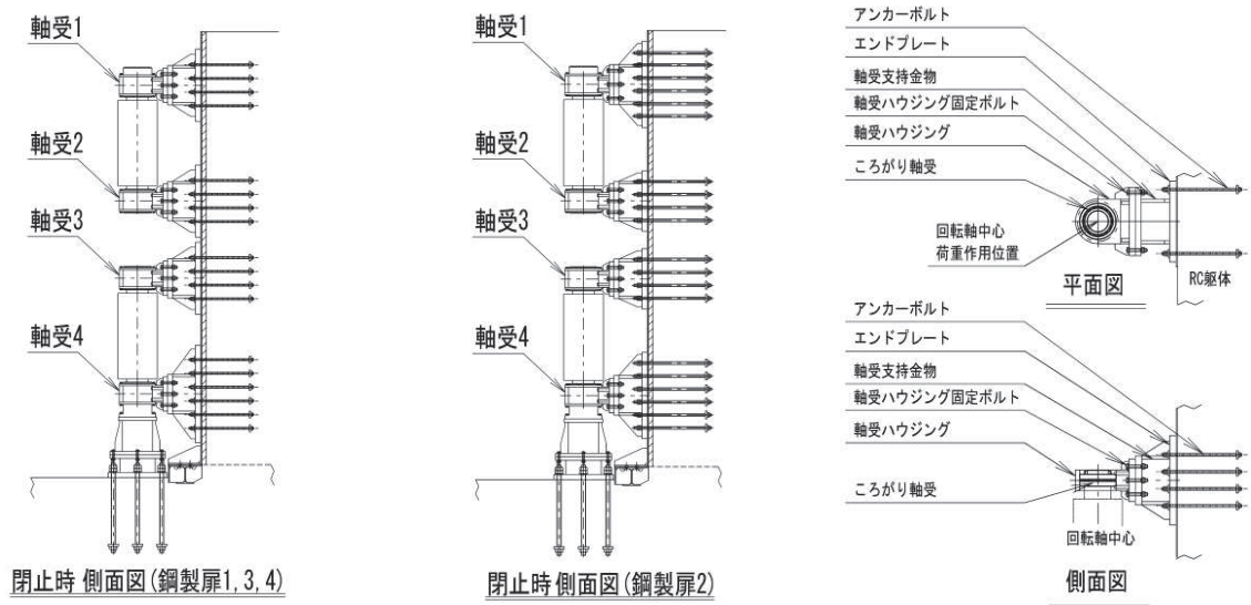
図 3.8-6 ヒンジ水平荷重支承部の概要図
