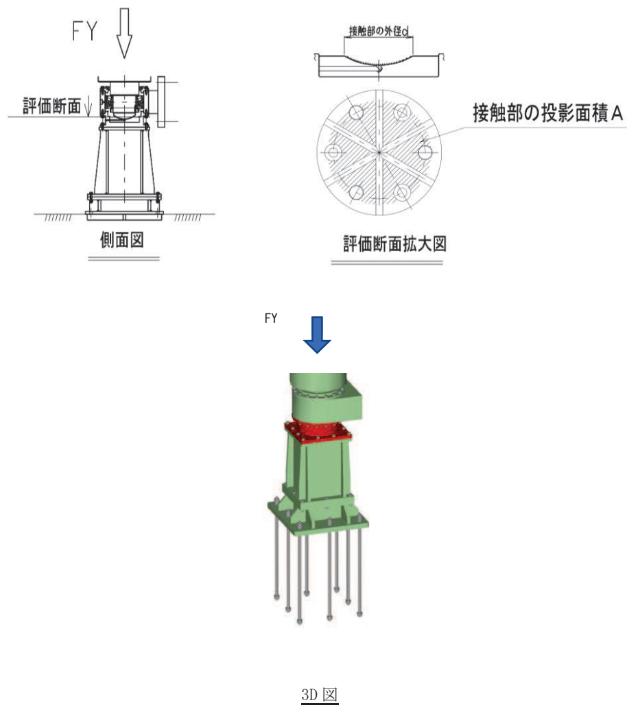
図 3.8-23 すべり軸受の構造概要及び計算モデルの概念図
