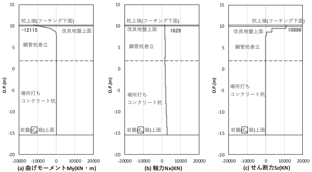
図 4.1-34(3) 場所打ちコンクリート杭のせん断破壊に対する照査における照査時刻での断面力 (鋼桁 1 : 基礎 2, S_s - D 2 (++) , 桁軸方向加振時, t = 29.98s ) 解析ケース② : 地盤物性のばらつき (+1 \sigma ) を考慮した解析ケース
