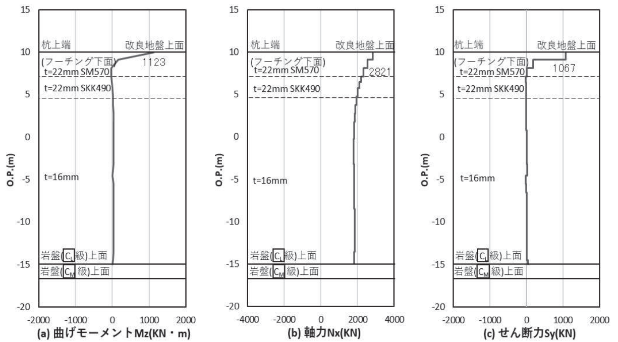
図 4.1-33(2) 鋼管杭の曲げ・軸力系の破壊に対する照査における照査時刻での断面力 (鋼桁 1: 基礎 1, S s - D 1 (+), 桁軸直交方向加振時, t = 25.50s) 解析ケース③: 地盤物性のばらつき (-1σ) を考慮した解析ケース
