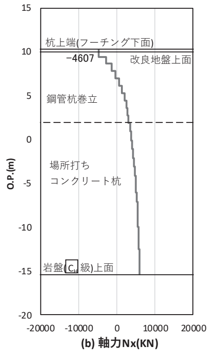
図 4.1-50(2) 基礎地盤の支持性能照査時刻での軸力（引き抜き） (鋼桁 1：基礎 2, S s - D 2 (++) , 桁軸方向加振時, t = 23.72s) 解析ケース③：地盤物性のばらつき (-1σ) を考慮した解析ケース
