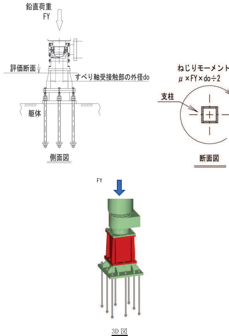
図 3.8-24 支柱の概要図及び計算モデルの概念図
