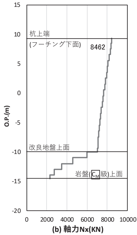
図 4.1-55(1) 基礎地盤の支持性能照査時刻での軸力（押し込み） (鋼桁 4：基礎 1, S s - N 1 (++) , 桁軸方向加振時, t = 7.89s) 解析ケース①：基本ケース
