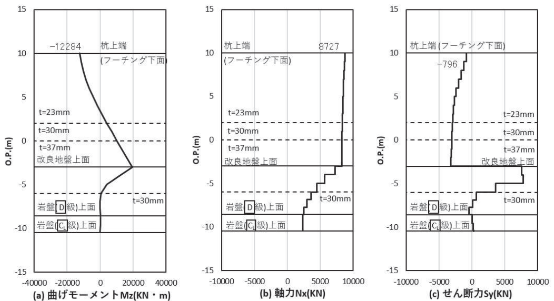
図 4.1-41(2) 鋼管杭の曲げ・軸力系の破壊に対する照査における照査時刻での断面力 (鋼桁 5 (地盤改良 (改良幅 2D 未満) 非考慮) : 基礎 2, S_s - N_1 (-+), 桁軸直交方向加振時, t = 7.84s ) 解析ケース①: 基本ケース
