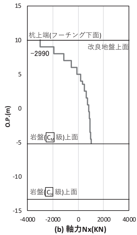
図 4.1-54 基礎地盤の支持性能照査時刻での軸力（引き抜き） （鋼桁 3：基礎 1，S s - D 2（+-），桁軸直交方向加振時， t = 17.76s ） 解析ケース③：地盤物性のばらつき（ -1\sigma ）を考慮した解析ケース
