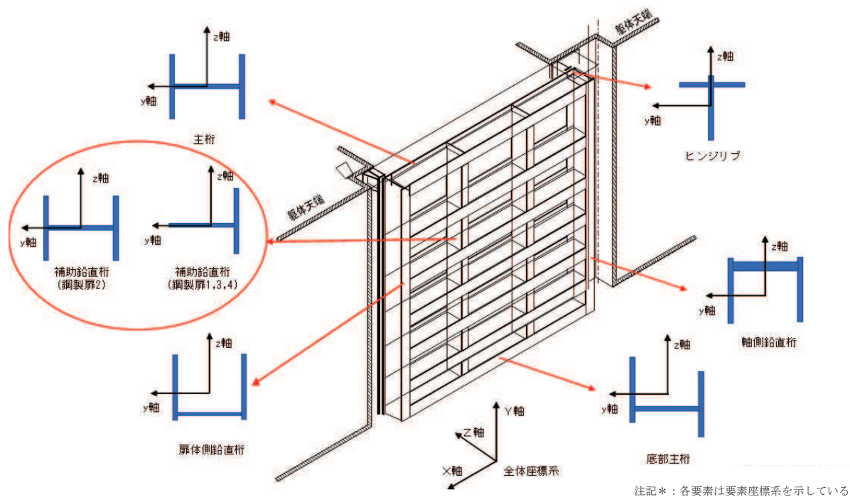
図 3.8-1 扉体の構造概要図
