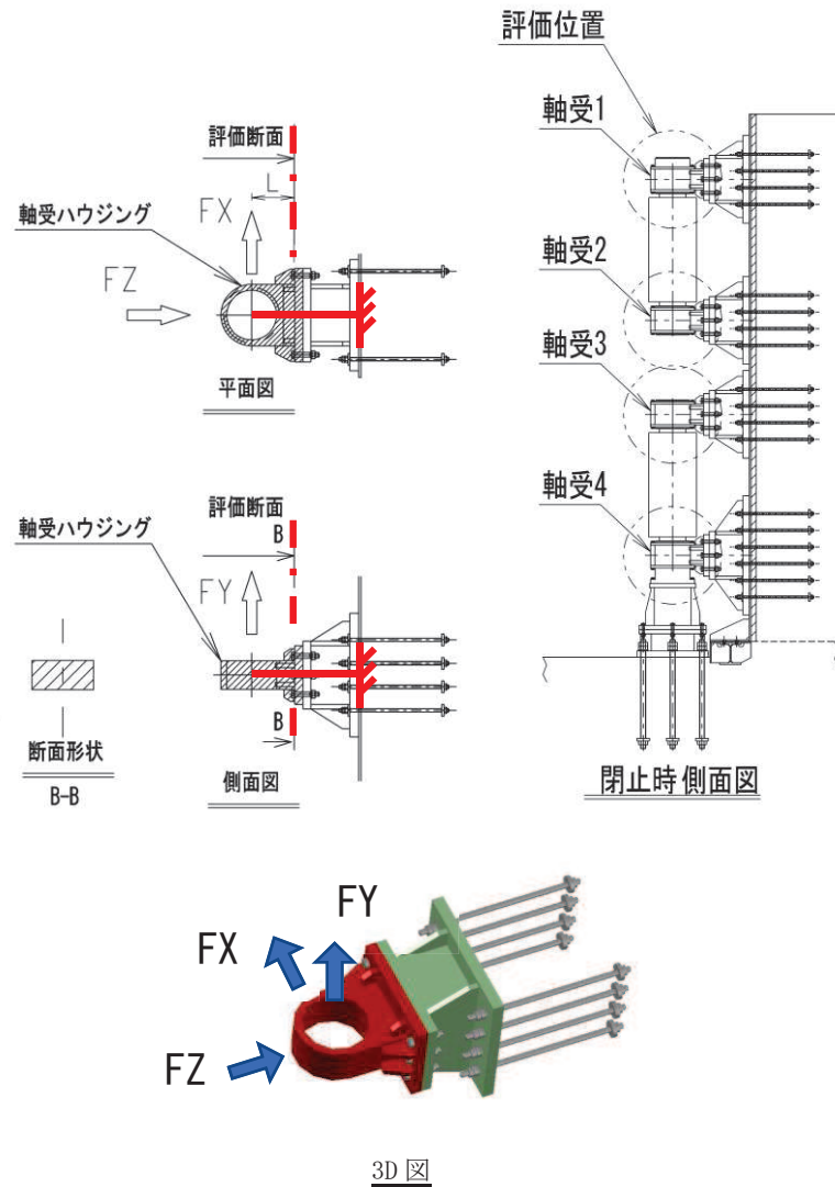
図 3.8-11 軸受ハウジング接合部の概要図及び計算モデルの概念図
