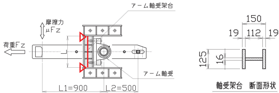
図 3.8-37 アーム軸受架台の概要図及び計算モデルの概念図
