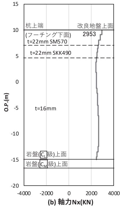
図 4.1-49(1) 基礎地盤の支持性能照査時刻での軸力（押し込み） (鋼桁 1：基礎 1, S s - D 2 (++) , 桁軸方向加振時, t = 23.56s) 解析ケース③：地盤物性のばらつき (-1σ) を考慮した解析ケース
