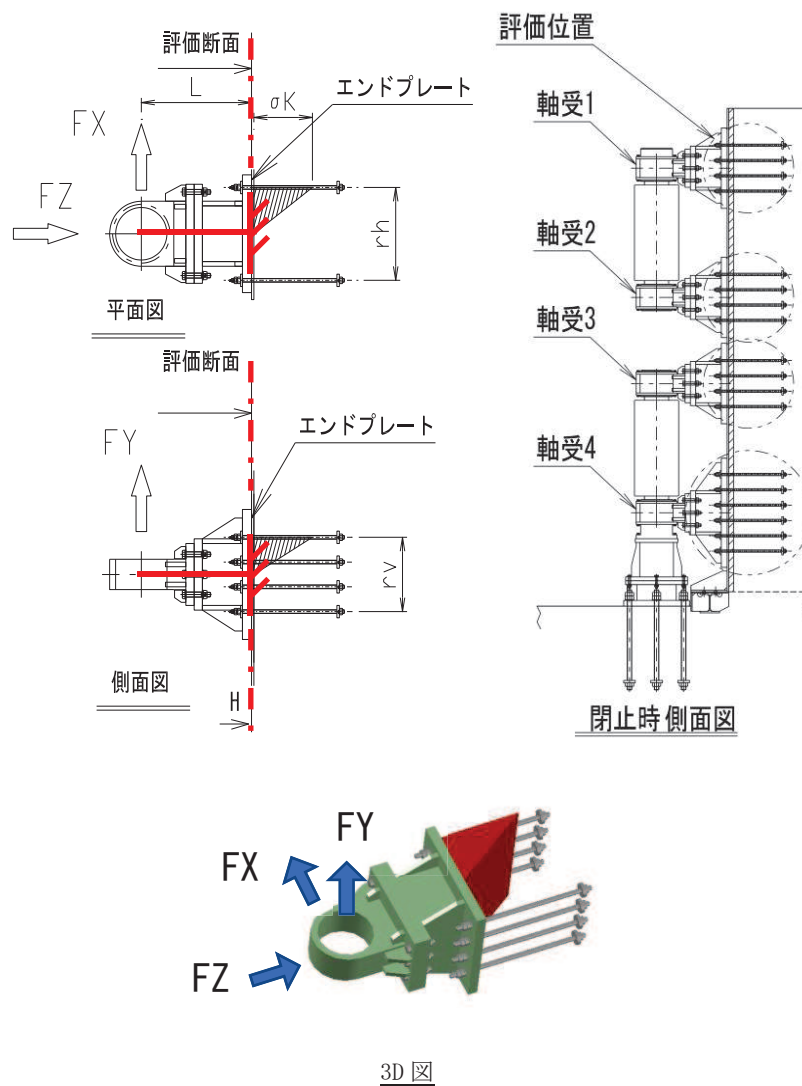
図 3.8-20 エンドプレートコンクリートの概要図及び支圧応力度に関する計算モデルの概念図
