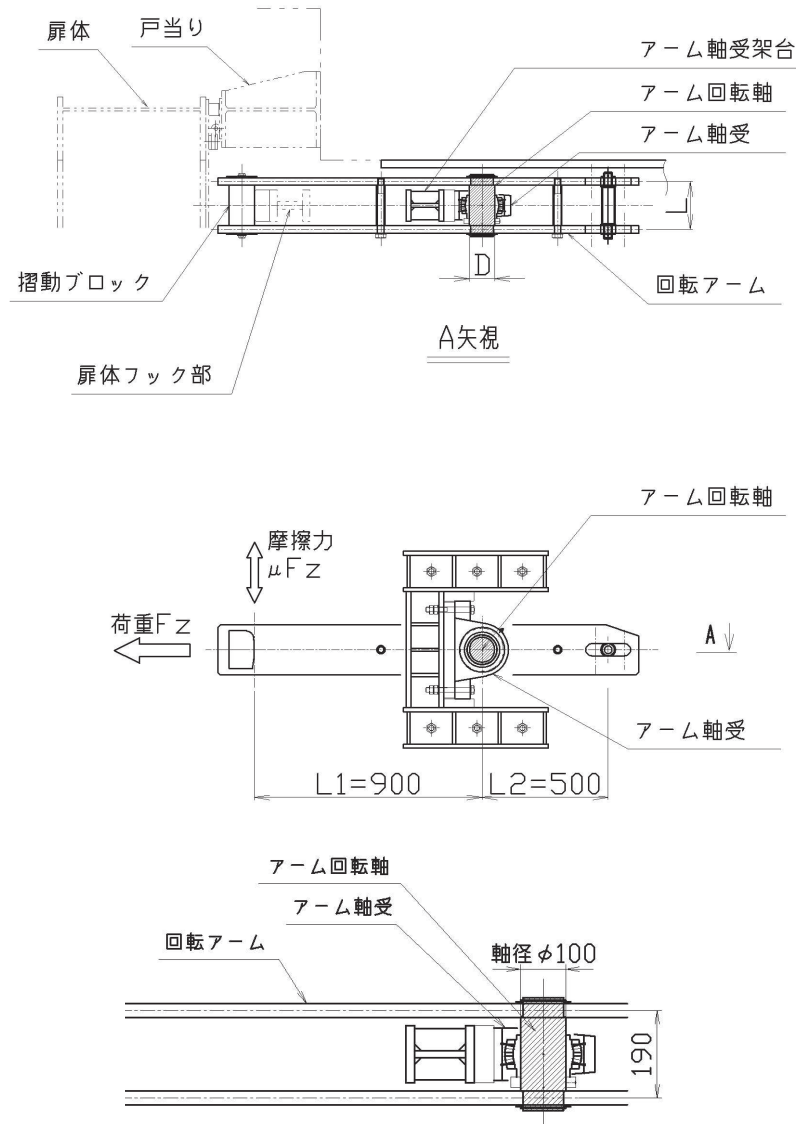
図 3.8-34 アーム回転軸の概要図及び計算モデルの概念図
