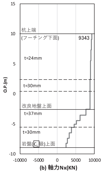
図 4.1-51(2) 基礎地盤の支持性能照査時刻での軸力（押し込み） (鋼桁 2：基礎 1, S s - N 1 (++) , 桁軸直交方向加振時, t = 7.84s) 解析ケース①：基本ケース
