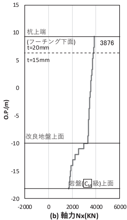
図 4.1-58(2) 基礎地盤の支持性能照査時刻での軸力（押し込み） (鋼桁 4：基礎 2, S s - N 1 (一+), 桁軸直交方向加振時, t = 7.88s) 解析ケース①：基本ケース
