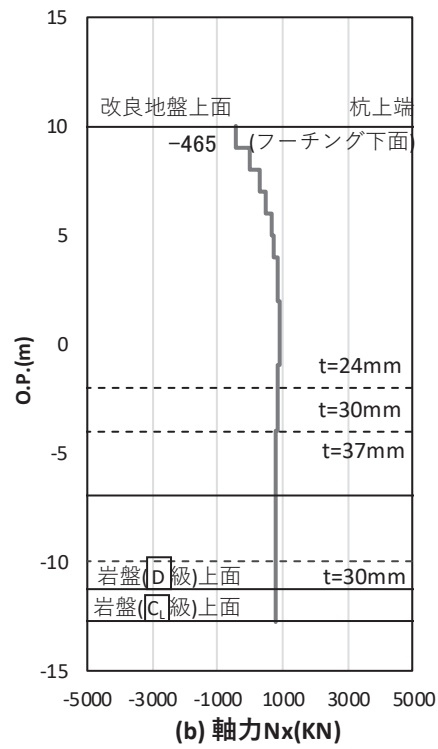
図 4.1-68(1) 基礎地盤の支持性能照査時刻での軸力（引き抜き） （鋼桁 6（地盤改良（改良幅 2D 未満）考慮）：基礎 1， S_s - F_3 （++），桁軸直交方向加振時， t = 26.93s ） 解析ケース①：基本ケース
