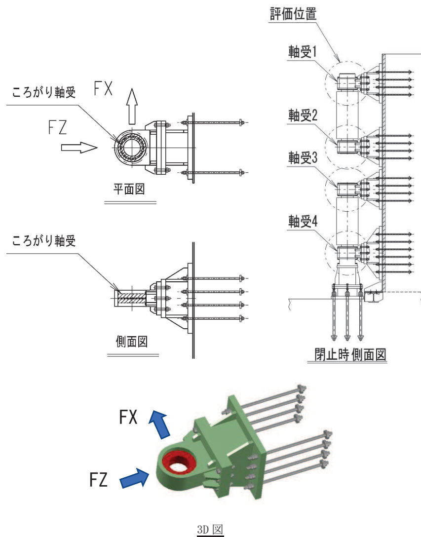
図 3.8-9 ころがり軸受の作用荷重の概要図
