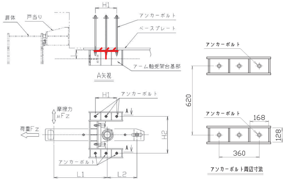
図 3.8-39 ベースプレート及びアンカーボルトの概要図及び計算モデルの概念図
