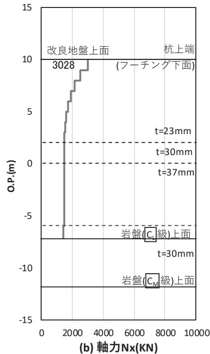
図 4.1-63(2) 基礎地盤の支持性能照査時刻での軸力（押し込み） （鋼桁 5（地盤改良（改良幅 2D 未満）考慮）：基礎 1， S s - D 2（++），桁軸直交方向加振時， t = 20.49\text{s} ） 解析ケース①：地盤物性のばらつき（ -1\sigma ）を考慮した解析ケース
