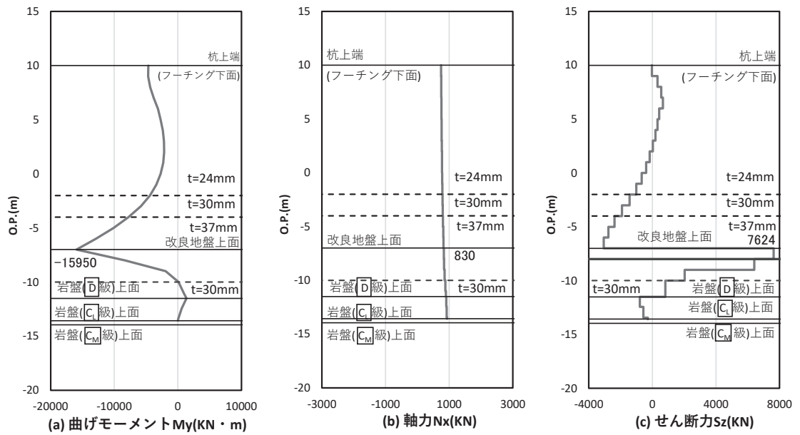
図 4.1-45(1) 鋼管杭の曲げ・軸力系の破壊に対する照査における照査時刻での断面力 (鋼桁 6 (地盤改良 (改良幅 2D 未満) 非考慮) : 基礎 2, S_s - N_1 (++) , 桁軸方向加振時, t = 7.78s ) 解析ケース① : 基本ケース
