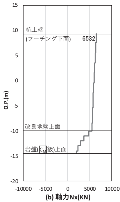
図 4.1-55(2) 基礎地盤の支持性能照査時刻での軸力（押し込み） (鋼桁 4：基礎 1, S s - N 1 (-+) , 桁軸直交方向加振時, t = 7.87s) 解析ケース①：基本ケース
