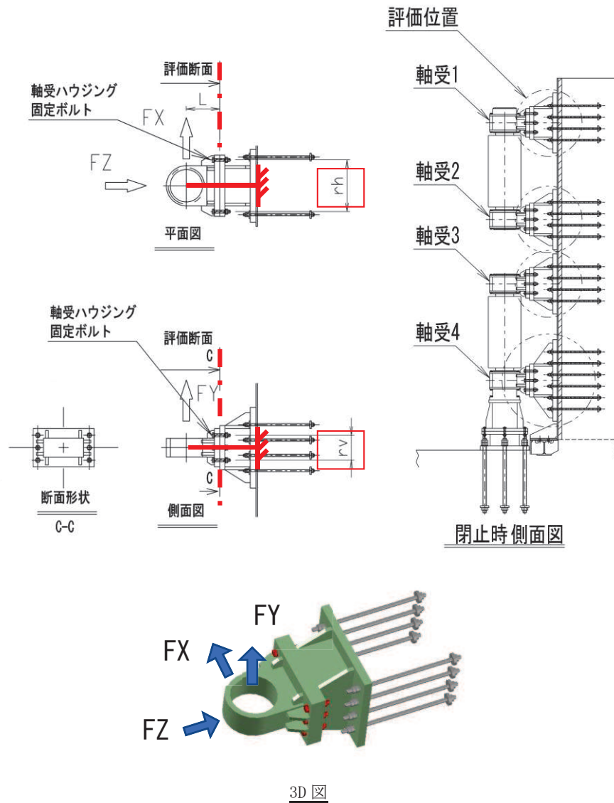
図 3.8-12 軸受ハウジング固定ボルトの概要図及び計算モデルの概念図
