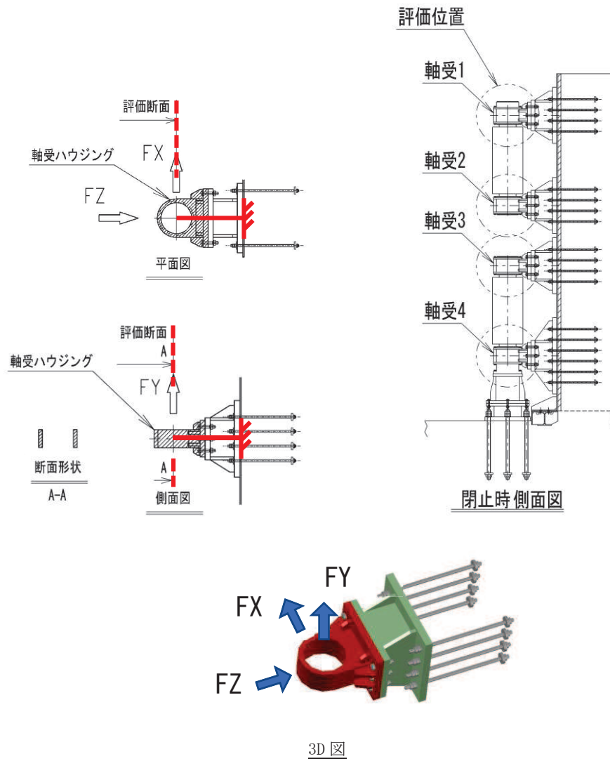
図 3.8-10 軸受ハウジング円筒部の概要図及び計算モデルの概念図
