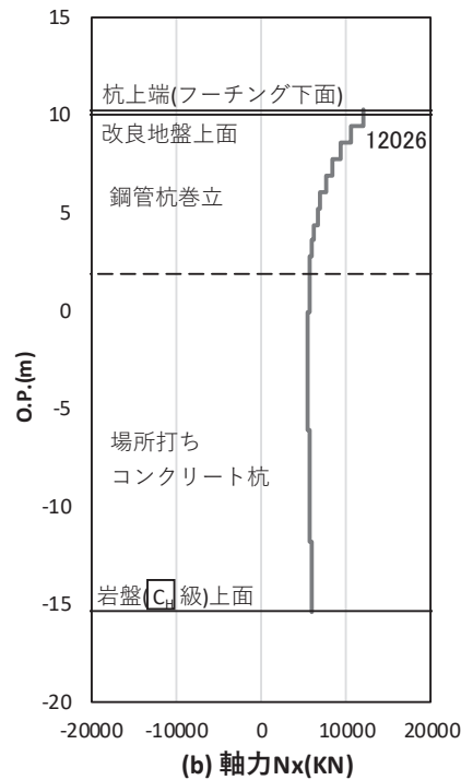
図 4.1-49(4) 基礎地盤の支持性能照査時刻での軸力（押し込み） (鋼桁 1：基礎 2， S_s - D 1 (+— )，桁軸直交方向加振時， t = 18.14s ) 解析ケース③：地盤物性のばらつき ( -1\sigma ) を考慮した解析ケース
