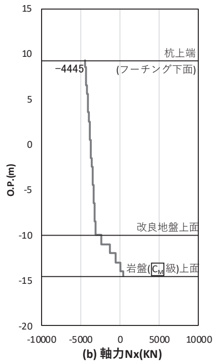
図 4.1-59(2) 基礎地盤の支持性能照査時刻での軸力（引き抜き） (鋼桁 4：基礎 1, S_s - N_1 (++) , 桁軸直交方向加振時, t = 7.83s ) 解析ケース①：基本ケース
