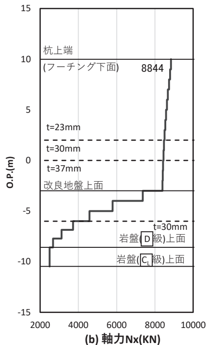
図 4.1-61(2) 基礎地盤の支持性能照査時刻での軸力（押し込み） （鋼桁 5（地盤改良（改良幅 2D 未満）非考慮）：基礎 2, S s - N 1（++），桁軸直交方向加振時， t = 7.85s ） 解析ケース①：基本ケース
