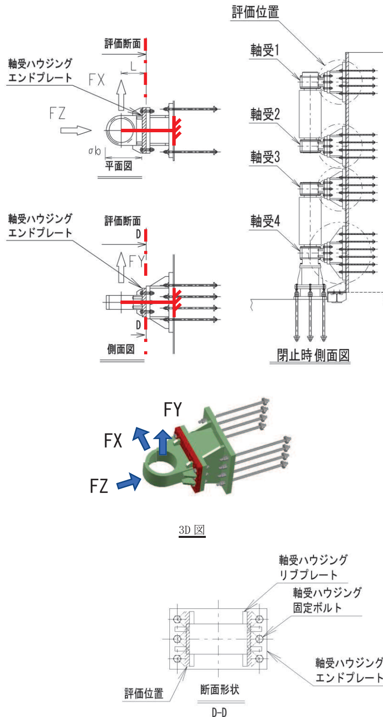
図 3.8-13 軸受ハウジングエンドプレートの概要図及び計算モデルの概念図
