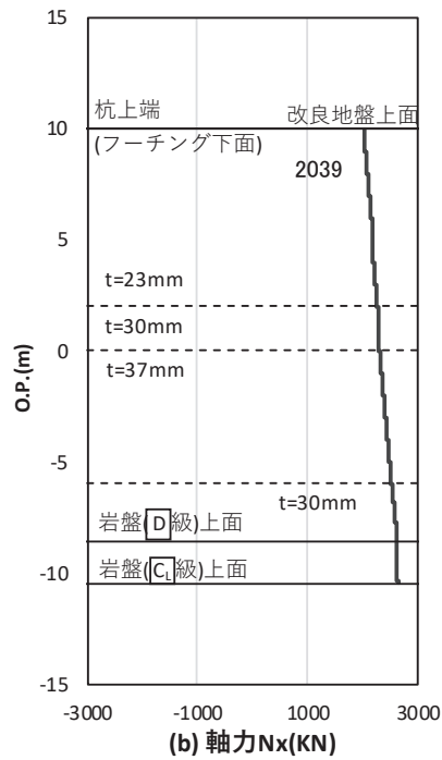
図 4.1-63(1) 基礎地盤の支持性能照査時刻での軸力（押し込み） （鋼桁 5（地盤改良（改良幅 2D 未満）考慮）：基礎 2， S s - D 2（-+），桁軸方向加振時， t = 23.56\text{s} ） 解析ケース③：地盤物性のばらつき（ -1\sigma ）を考慮した解析ケース
