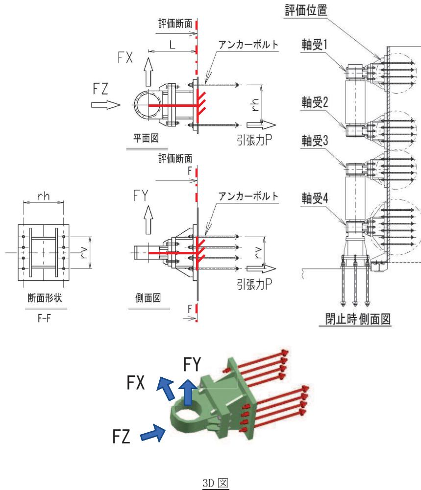
図 3.8-21 アンカーボルトの概要図及び計算モデルの概念図
