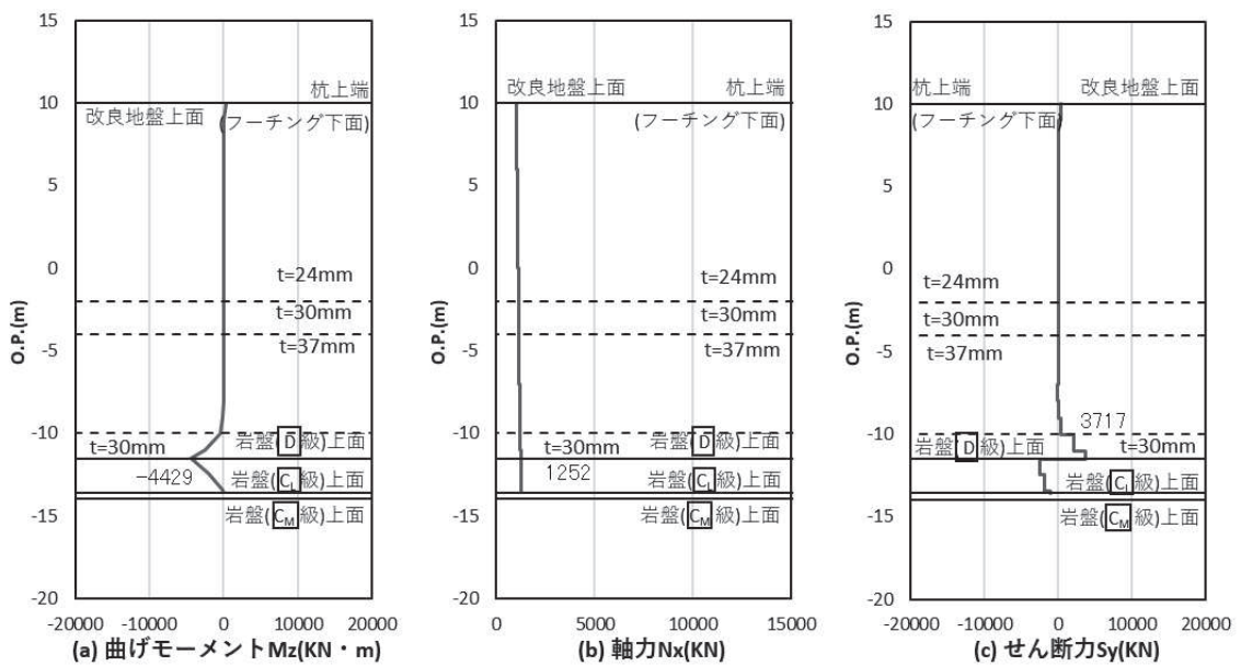
図 4.1-48(2) 鋼管杭のせん断破壊に対する照査における照査時刻での断面力 (鋼桁 6 (地盤改良 (改良幅 2D 未満) 考慮) : 基礎 2, S_s - N_1 (++) , 桁軸直交方向加振時, t = 7.64s ) 解析ケース② : 地盤物性のばらつき (+1 \sigma ) を考慮した解析ケース
