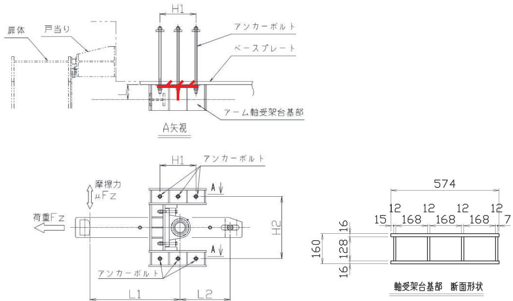
図 3.8-38 アーム軸受架台基部の概要図及び計算モデルの概念図
