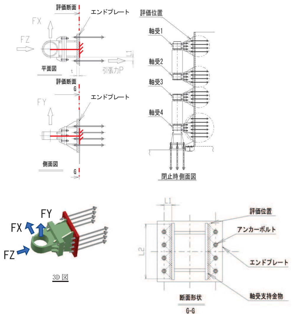
図 3.8-17 エンドプレート周辺の概要図及び計算モデルの概念図
