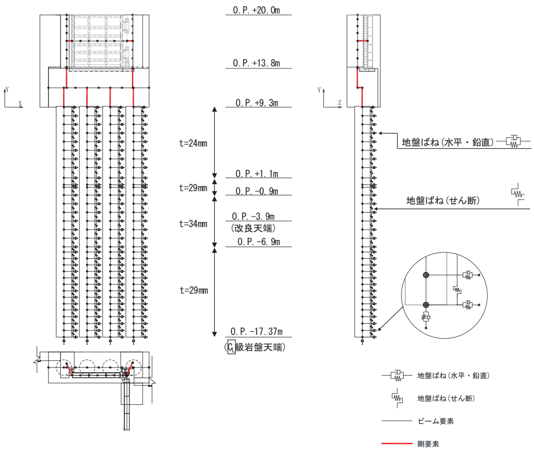
図 3.5-2 解析モデル (鋼製扉 3)
