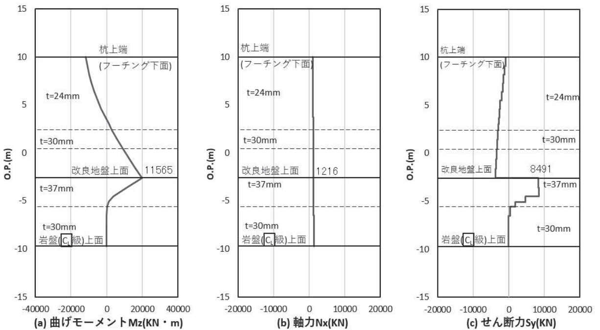
図 4.1-36(2) 鋼管杭のせん断破壊に対する照査における照査時刻での断面力 (鋼桁 2 : 基礎 2, S s - N 1 (++) , 桁軸直交方向加振時, t = 7. 81s) 解析ケース② : 地盤物性のばらつき (+ 1 σ) を考慮した解析ケース
