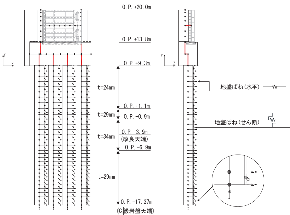
図 3.5-7 静的解析モデル (鋼製扉 3 の例)
