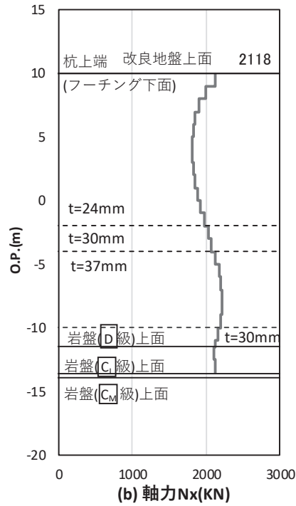
図 4.1-67(1) 基礎地盤の支持性能照査時刻での軸力（押し込み） （鋼桁 6（地盤改良（改良幅 2D 未満）考慮）：基礎 2， S s - D 2（- -），桁軸方向加振時， t = 21.56s ） 解析ケース③：地盤物性のばらつき（ -1\sigma ）を考慮した解析ケース
