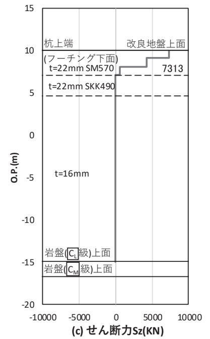
図 4.1-33(1) 鋼管杭の曲げ・軸力系の破壊に対する照査における照査時刻での断面力 (鋼桁 1: 基礎 1, S_s - D_2 (++) , 桁軸方向加振時, t = 24.00s )
