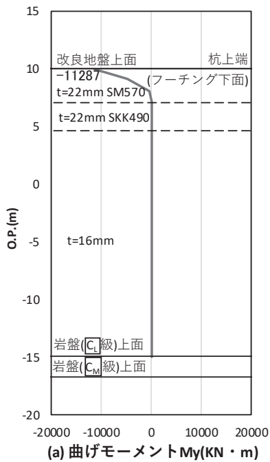
図 4.1-33(1) 鋼管杭の曲げ・軸力系の破壊に対する照査における照査時刻での断面力 (鋼桁 1: 基礎 1, S_s - D_2 (++) , 桁軸方向加振時, t = 24.00s )
