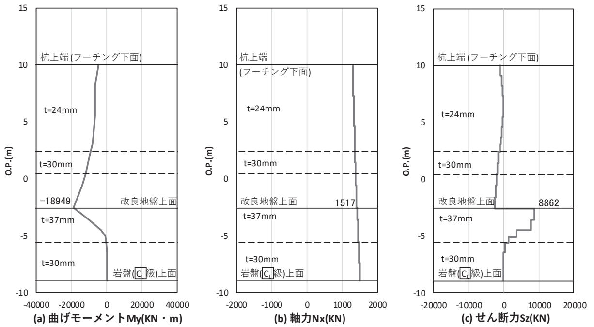
図 4.1-36(1) 鋼管杭のせん断破壊に対する照査における照査時刻での断面力 (鋼桁 2 : 基礎 1, S s - N 1 (++) , 桁軸方向加振時 t = 7. 82s) 解析ケース① : 基本ケース
