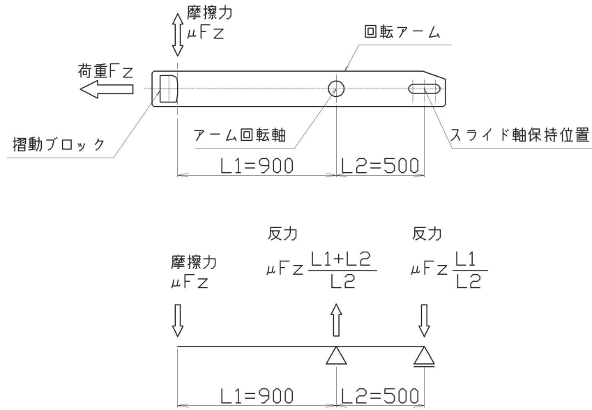
図 3.8-35 アーム回転軸の概要図及び計算モデルの概念図
