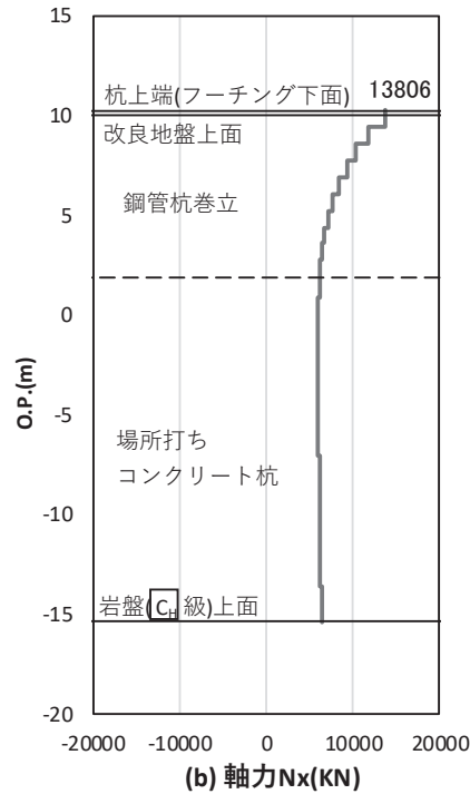
図 4.1-49(3) 基礎地盤の支持性能照査時刻での軸力（押し込み） (鋼桁 1：基礎 2， S_s - D 1 (—+ )，桁軸方向加振時， t = 18.09s ) 解析ケース③：地盤物性のばらつき ( -1\sigma ) を考慮した解析ケース
