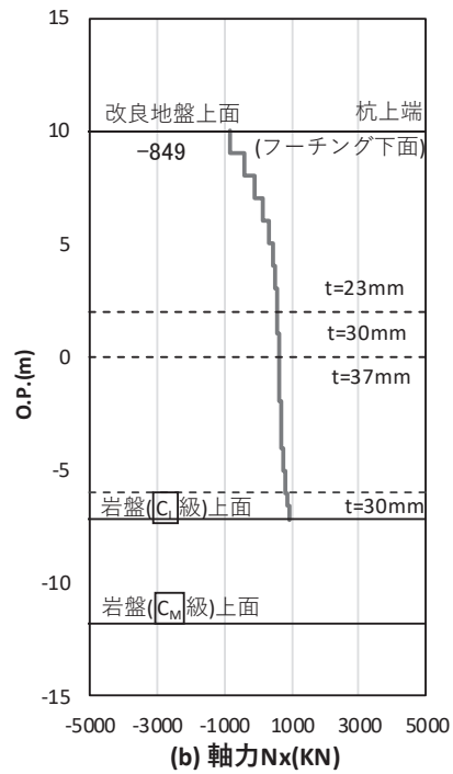
図 4.1-64 基礎地盤の支持性能照査時刻での軸力（引き抜き） （鋼桁 5（地盤改良（改良幅 2D 未満）考慮）：基礎 1， S_s - D_2 （++），桁軸直交方向加振時， t = 17.80\text{s} ） 解析ケース③：地盤物性のばらつき（ -1\sigma ）を考慮した解析ケース
