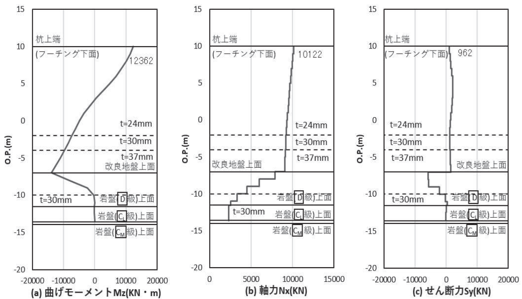
図 4.1-45(2) 鋼管杭の曲げ・軸力系の破壊に対する照査における照査時刻での断面力 (鋼桁 6 (地盤改良 (改良幅 2D 未満) 非考慮) : 基礎 2, S_s - N_1 (-+) , 桁軸直交方向加振時, t = 7.88s ) 解析ケース① : 基本ケース
