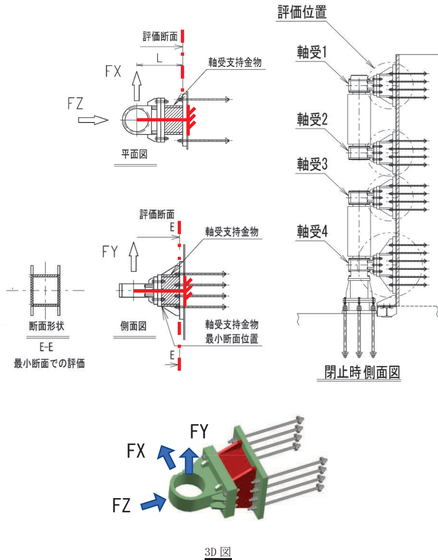
図 3.8-16 軸受支持金物の概要図及び計算モデルの概念図
