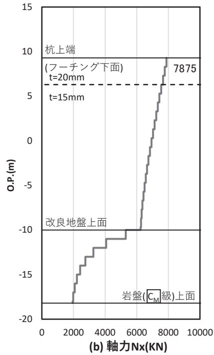
図 4.1-55(3) 基礎地盤の支持性能照査時刻での軸力（押し込み） (鋼桁 4：基礎 2, S s - N 1 (一+), 桁軸方向加振時, t = 7.88s) 解析ケース①：基本ケース
