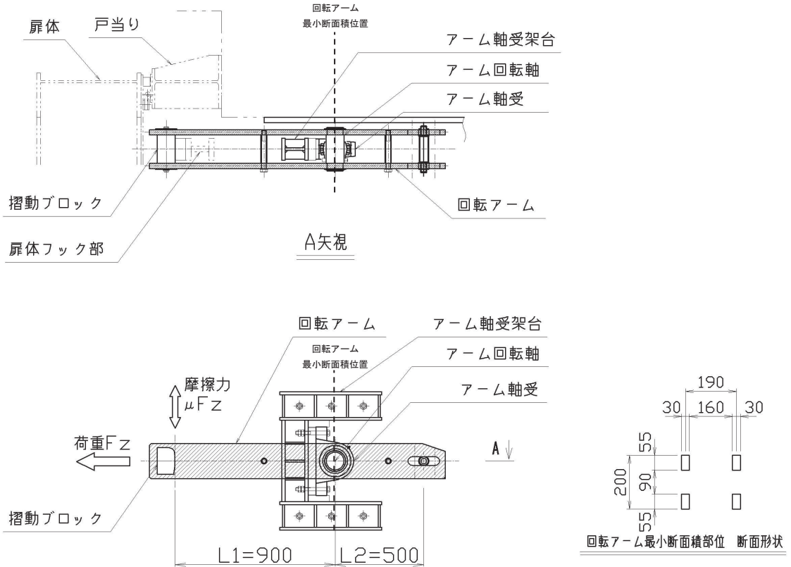
図 3.8-31 回転アームの概要図及び計算モデルの概念図
