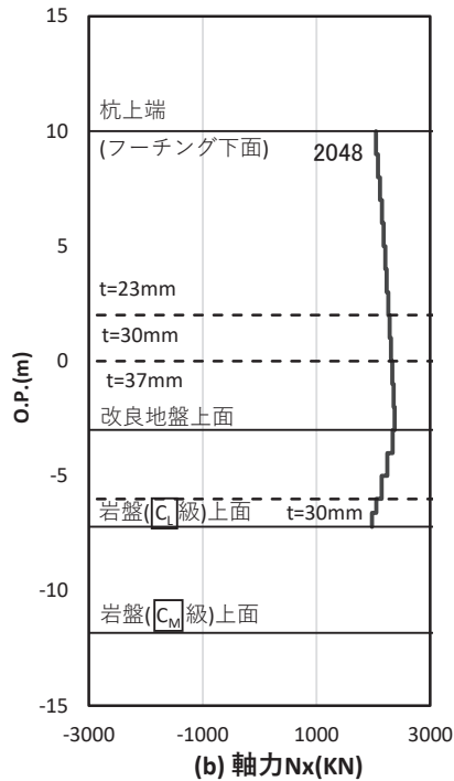
図 4.1-61(1) 基礎地盤の支持性能照査時刻での軸力（押し込み） （鋼桁 5（地盤改良（改良幅 2D 未満）非考慮）：基礎 1, S s - D 2（++），桁軸方向加振時， t = 23.55s ） 解析ケース①：基本ケース
