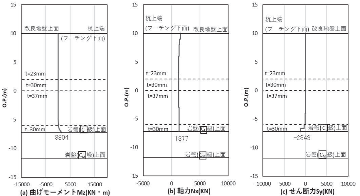
図 4.1-43 (2) 鋼管杭の曲げ・軸力系の破壊に対する照査における照査時刻での断面力
