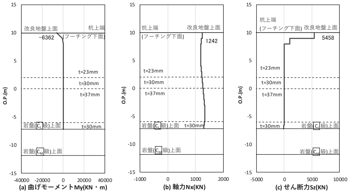
図 4.1-43 (1) 鋼管杭の曲げ・軸力系の破壊に対する照査における照査時刻での断面力
