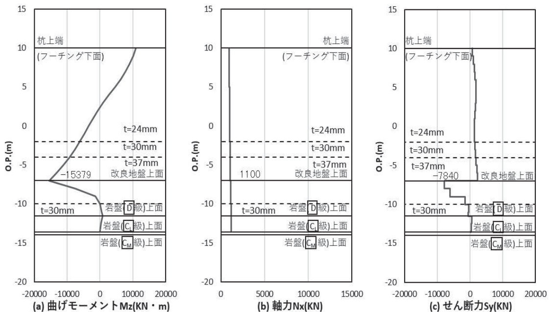
図 4.1-46(2) 鋼管杭のせん断破壊に対する照査における照査時刻での断面力 (鋼桁 6 (地盤改良 (改良幅 2D 未満) 非考慮) : 基礎 2, S_s - N_1 (-+) , 桁軸直角方向加振時, t = 7.81s ) 解析ケース② : 地盤物性のばらつき (+1 \sigma ) を考慮した解析ケース
