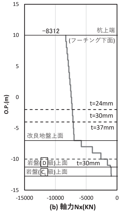
図 4.1-66(2) 基礎地盤の支持性能照査時刻での軸力（引き抜き） （鋼桁 6（地盤改良（改良幅 2D 未満）非考慮）：基礎 1， S s - N 1（++），桁軸直交方向加振時， t = 7.89s ）
