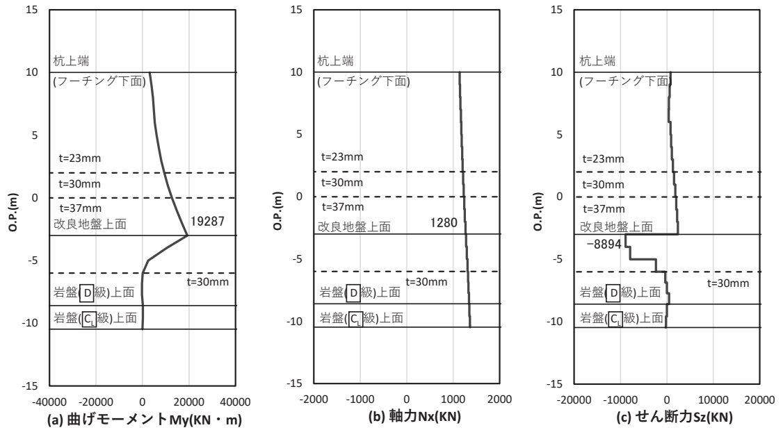
図 4.1-41(1) 鋼管杭の曲げ・軸力系の破壊に対する照査における照査時刻での断面力 (鋼桁 5 (地盤改良 (改良幅 2D 未満) 非考慮) : 基礎 2, S_s - N_1 (-+), 桁軸方向加振時, t = 7.84s ) 解析ケース①: 基本ケース
