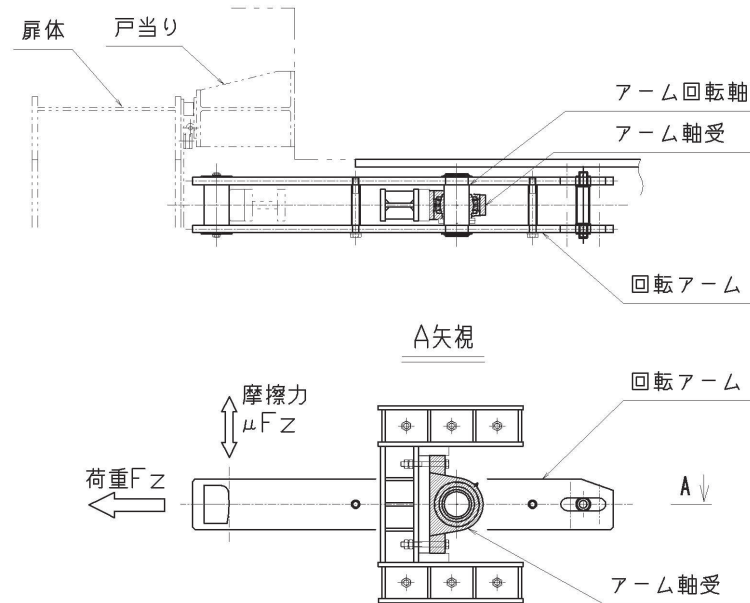
図 3.8-36 アーム軸受の概要図及び計算モデルの概念図
