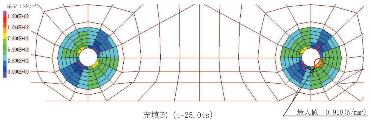
図 3.8-1(4) 解析ケース① 基準地震動 S s - D 2 (-+) に対する引張応力分布図
