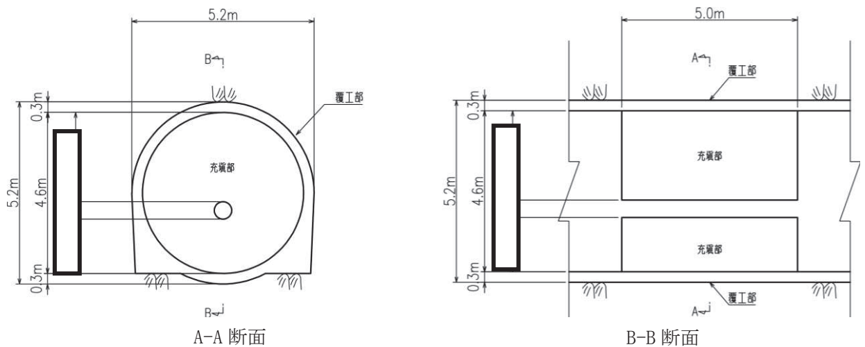
図 2.2-1(2) 取放水路流路縮小工（第1号機放水路） 断面図
