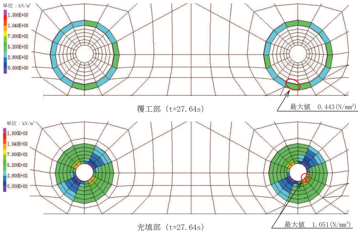
図 3.8-1(12) 解析ケース① 基準地震動 S s -F3 (-+) に対する引張応力分布図
