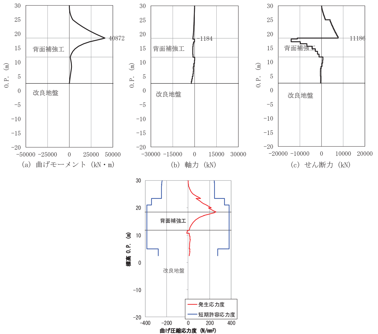
図 3-13 鋼管杭の曲げ・軸力系の破壊に対する照査における評価時刻での断面力及び曲げ圧縮応力度 (断面③, 短杭)
