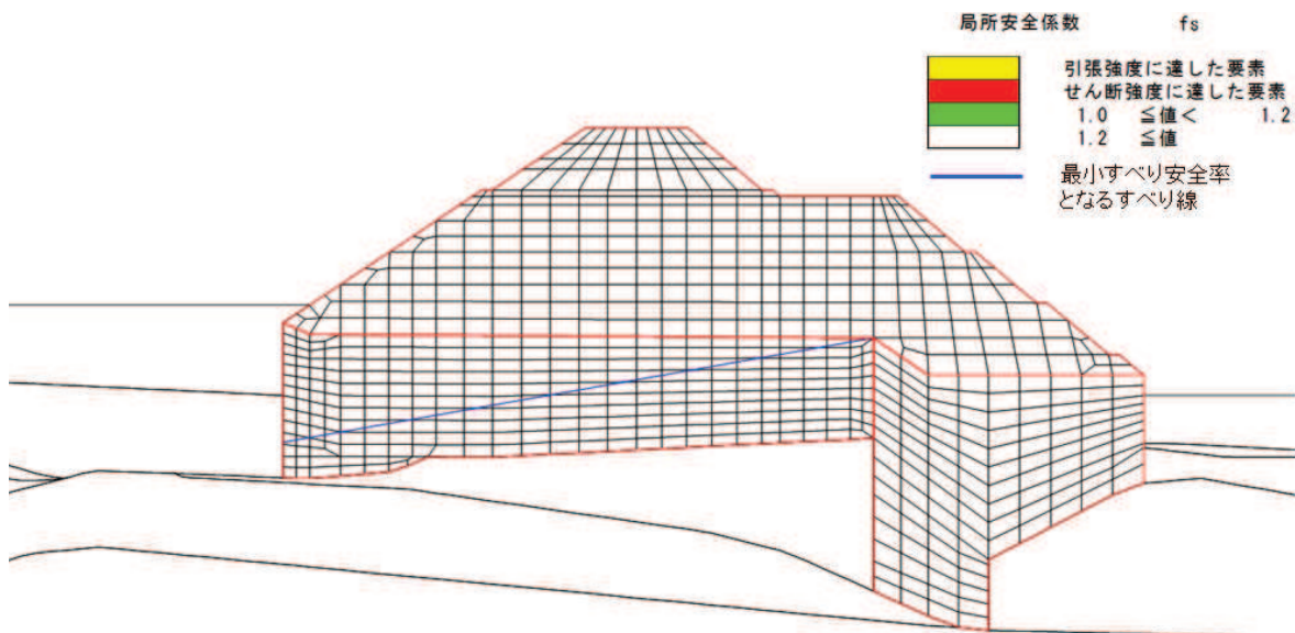
図 4.1-3 改良地盤の局所安全係数分布 (断面①) 解析ケース②：地盤物性のばらつきを考慮した解析ケース (平均値 + 1 \sigma )
