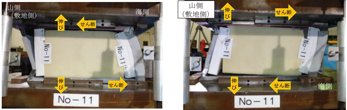
図2 ウレタンシリコーン目地変形試験状況
