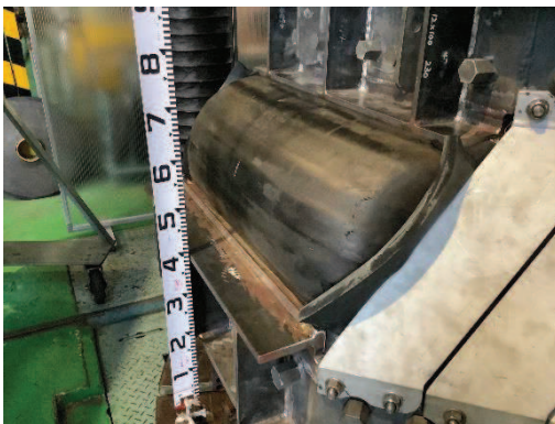
0.40MPa, 1時間保持後 (漏えい無し)
