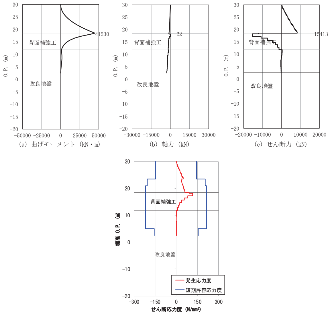
図 3-32 鋼管杭のせん断破壊に対する照査における評価時刻での 断面力及び曲げ圧縮応力度 (断面②， 短杭， S d - D 2（++）， t=6.93s)
