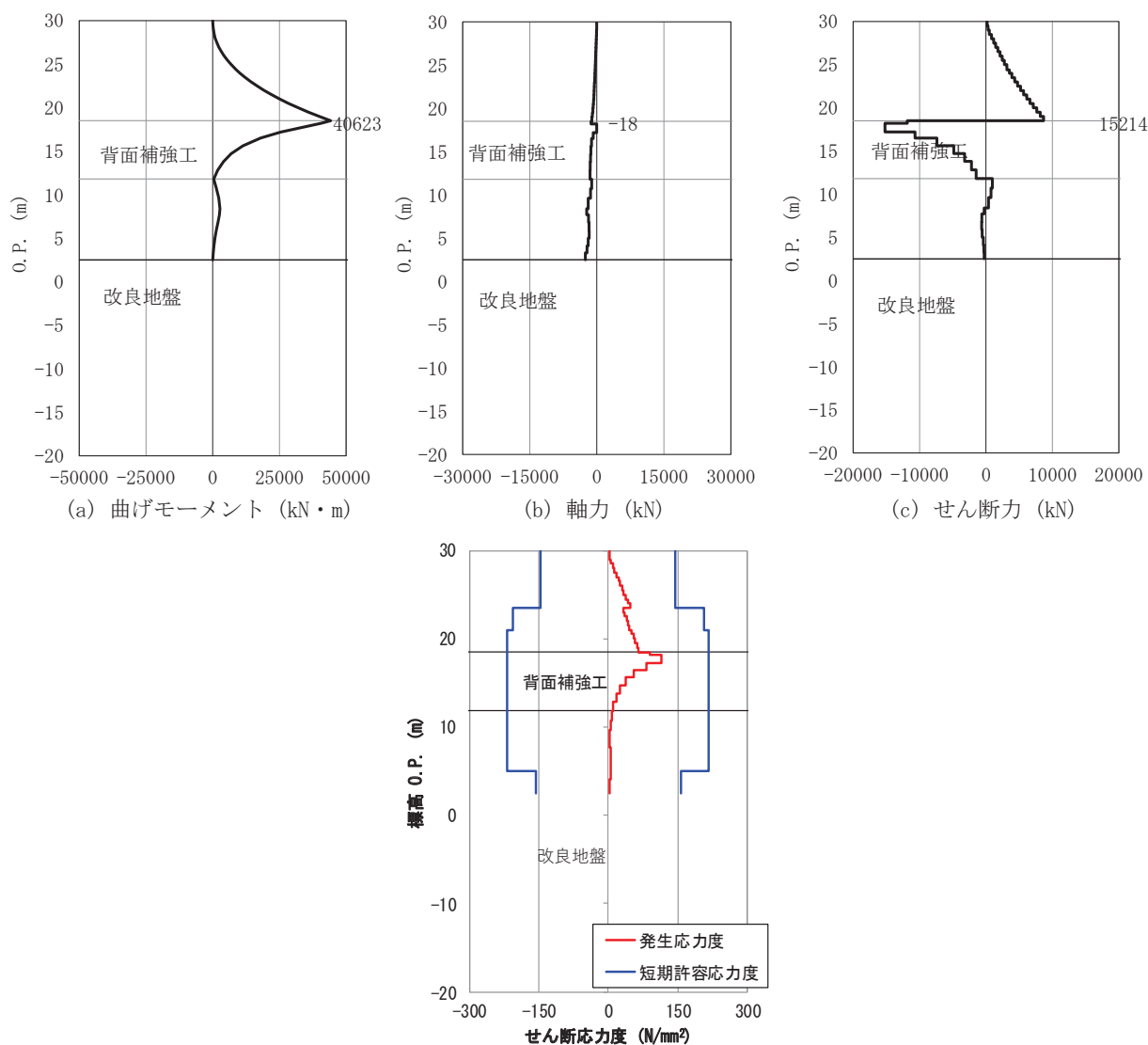
図 3-38 鋼管杭のせん断破壊に対する照査における評価時刻での断面力及び曲げ圧縮応力度
