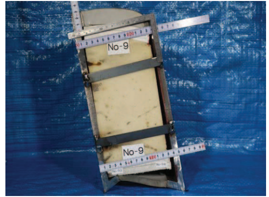
図 6.1.5-23(3) ウレタンシリコーン目地変形試験状況
