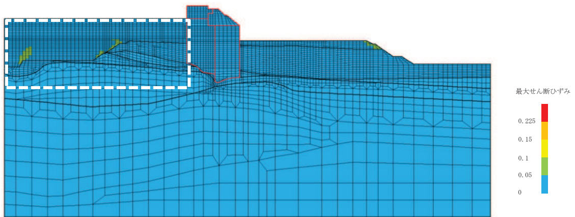
図 2-2 津波時における最大せん断ひずみ分布（断面②）
