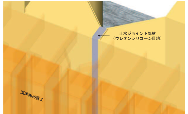
(ゴムジョイント部材の設置イメージ) (ウレタンシリコーン目地の設置イメージ)
