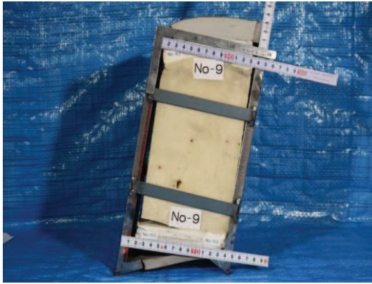
図 6.1.5-23(3) ウレタンシリコーン目地変形試験状況
