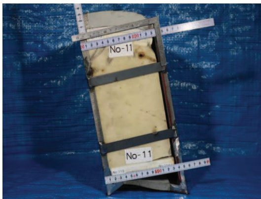
図3 ウレタンシリコーン目地変形試験状況
