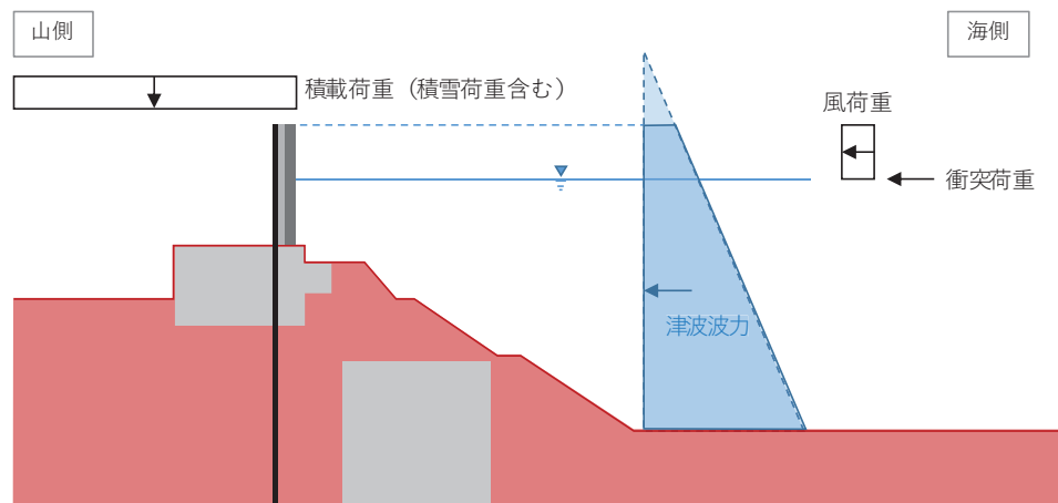
図 1-1(1) 荷重作用図（一般部，津波時）
