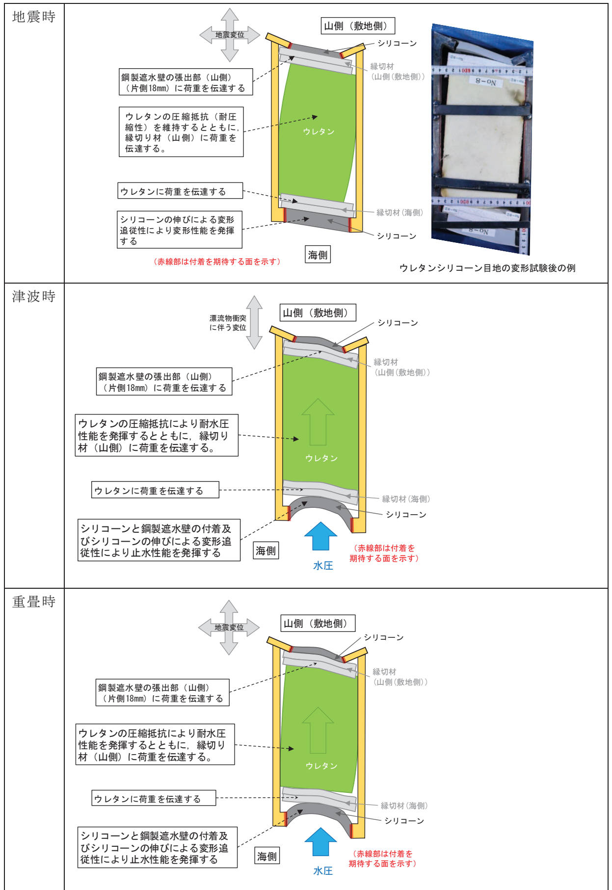
図 6. 1. 5-16 荷重伝達の概要及び止水性能発揮のメカニズム
