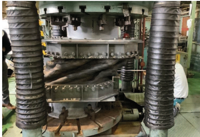
図 6.1.5-12(5) 変形試験全体状況（伸び 150mm，せん断 350mm，水圧 0MPa）
