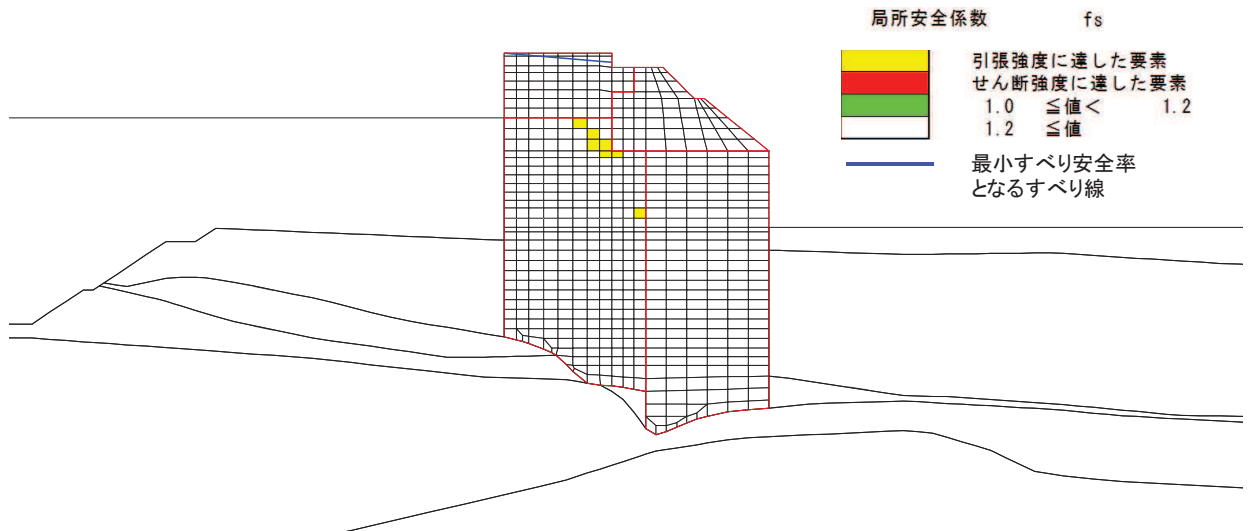
図 3-3 背面補強工の最小すべり安全率時刻における局所安全係数分布 (断面②, ジョイント要素追加設定)
