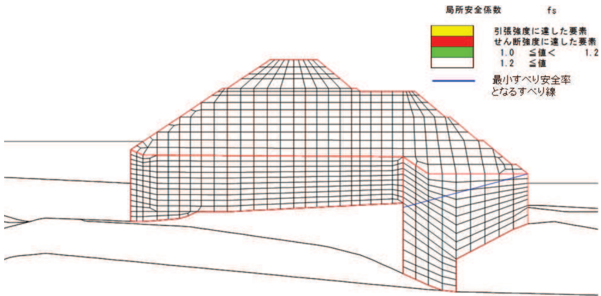
図 4.1-2 置換コンクリートの局所安全係数分布 (断面①) 解析ケース②：地盤物性のばらつきを考慮した解析ケース (平均値 + 1 \sigma )
