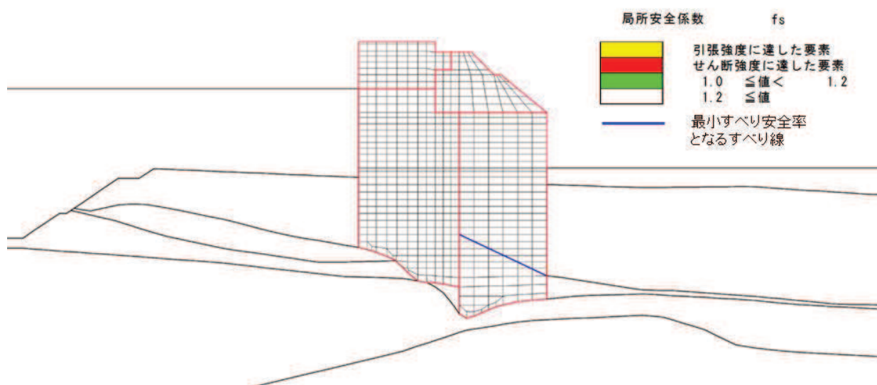
図 3-34 置換コンクリート工の最小すべり安全率時刻における局所安全係数分布 (断面②, 短杭, S d - D 2 ( + + ) , t=12.91s)
