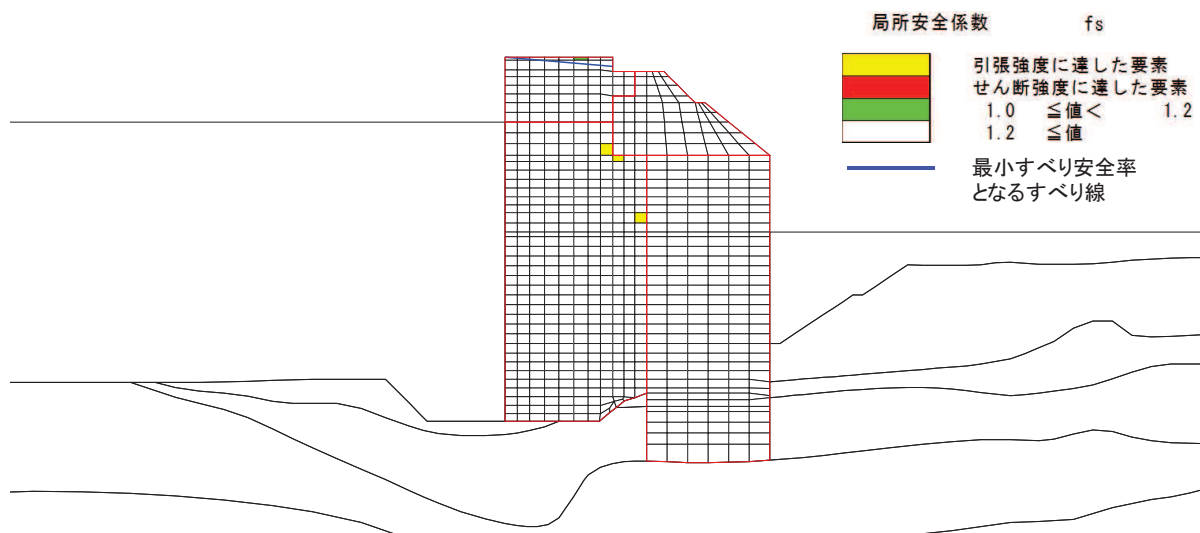
図 3-9 背面補強工の最小すべり安全率時刻における局所安全係数分布 (断面①, ジョイント要素追加設定, S d - D 2 ( - + ) , t=17.48s)
