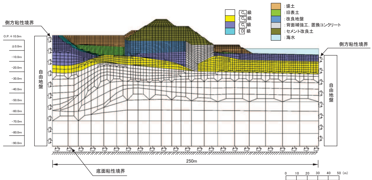
図 3.5-4 防潮堤（盛土堤防）の解析モデル（断面①）
