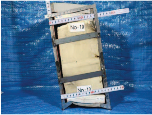
図 6.1.5-23(4) ウレタンシリコーン目地変形試験状況
