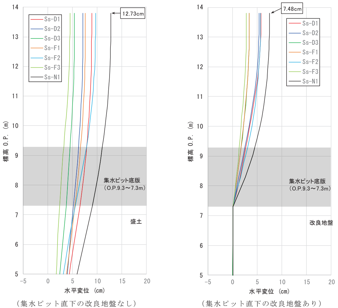
図 1-4 一次元地震応答解析による最大水平変位分布
