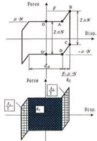
変位-荷重履歴のモデル
