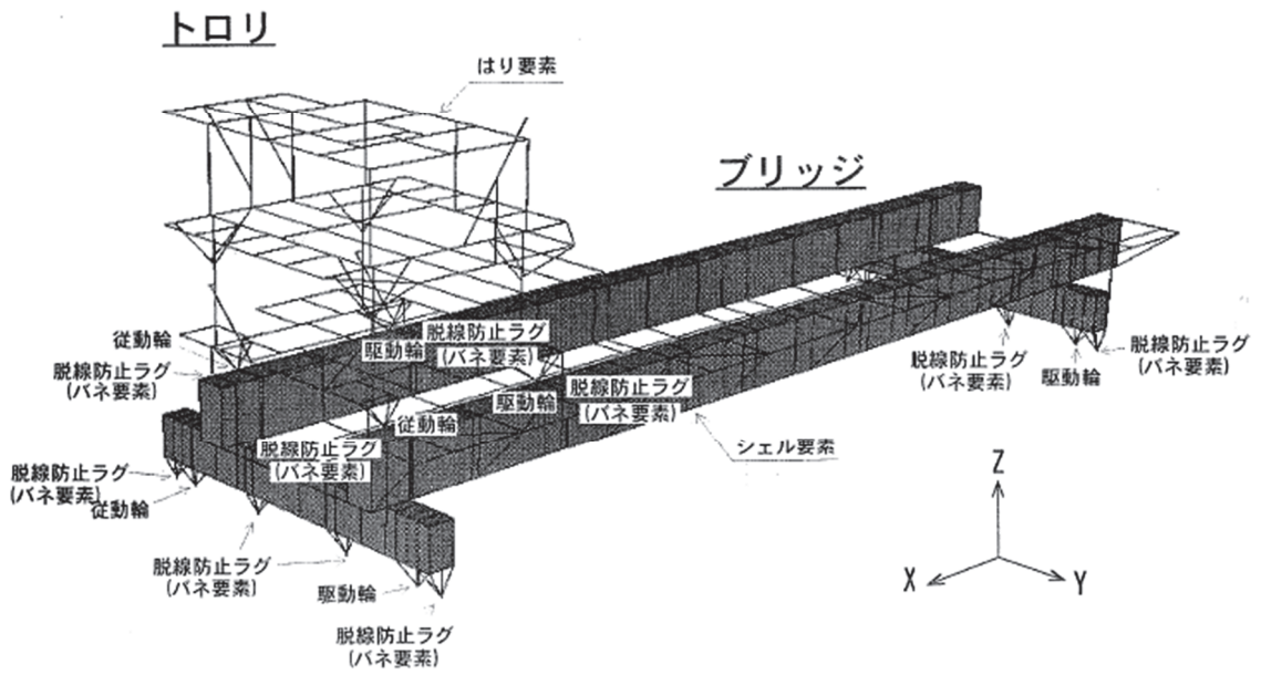
(2) トロリがブリッジの端部にある場合
