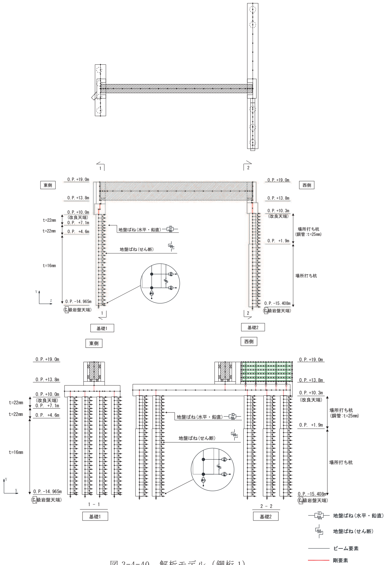
図 3-4-40 解析モデル (鋼桁 1)
