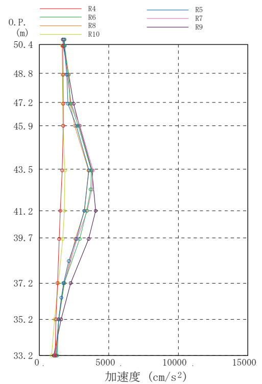
(d) 西面壁
