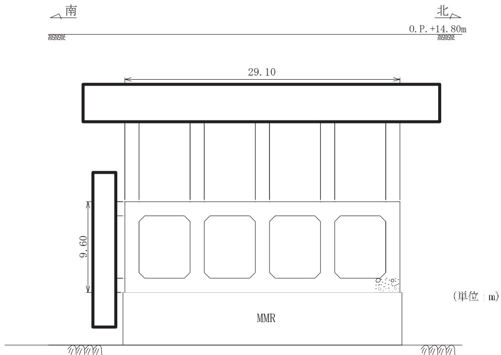
図 3-3-23 第 3 号機取水路断面図 (A-A 断面)
