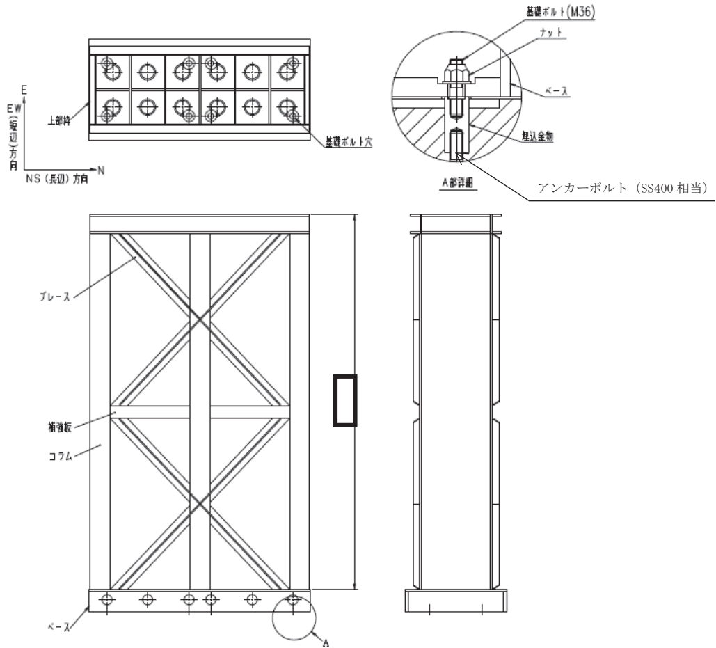
添付 9-6 図 制御棒貯蔵ラック構造図
