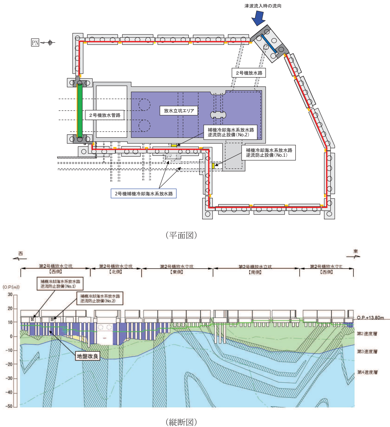
添付 10-2 図 補機冷却海水系放水路逆流防止設備の配置概要
