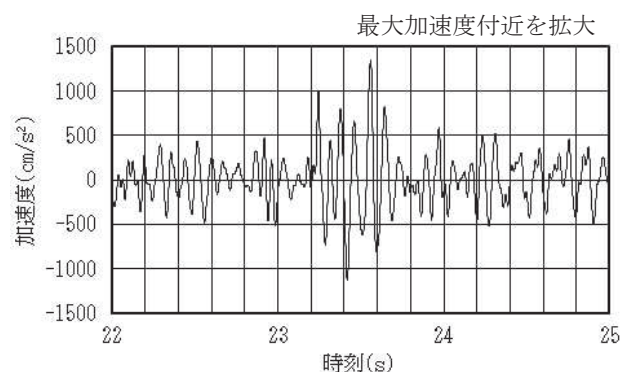
図6 鉛直方向応答加速度時刻歴* 2 （S s - D 2 原子炉建屋 OP. 33. 200）
