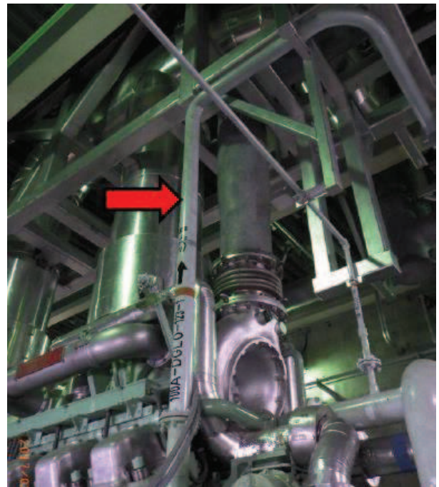
(b) 高圧炉心スプレイ系ディーゼル機関 ミスト
