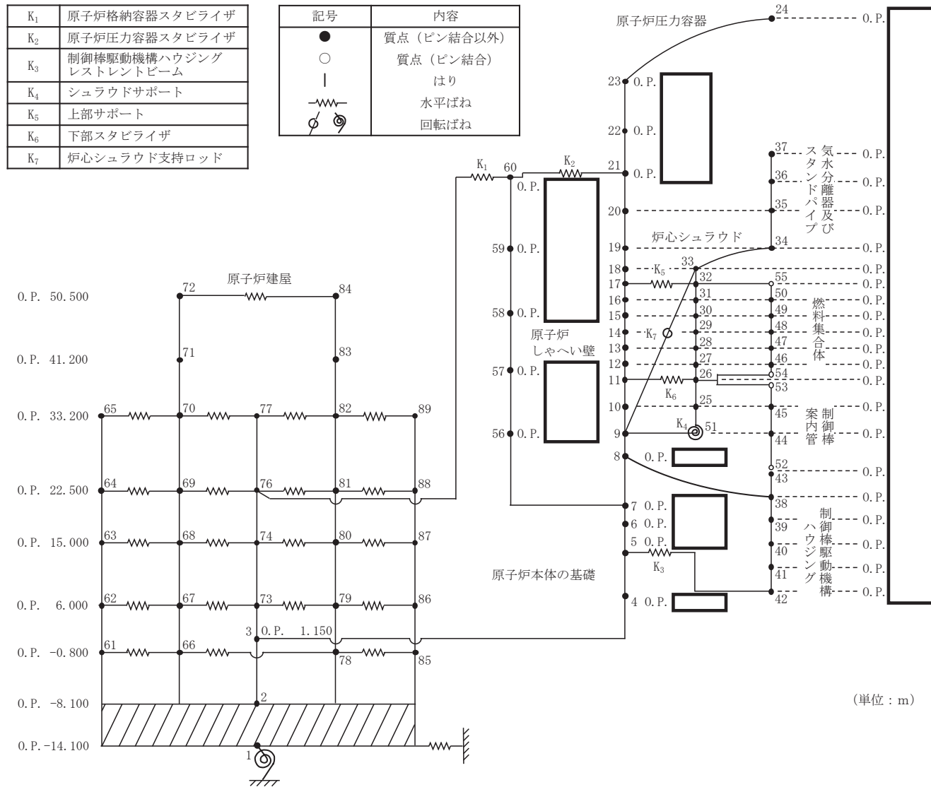
別図 1 炉内構造物系地震応答解析モデル図 (NS 方向)
