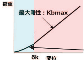
滑り変位とばね力の関係
