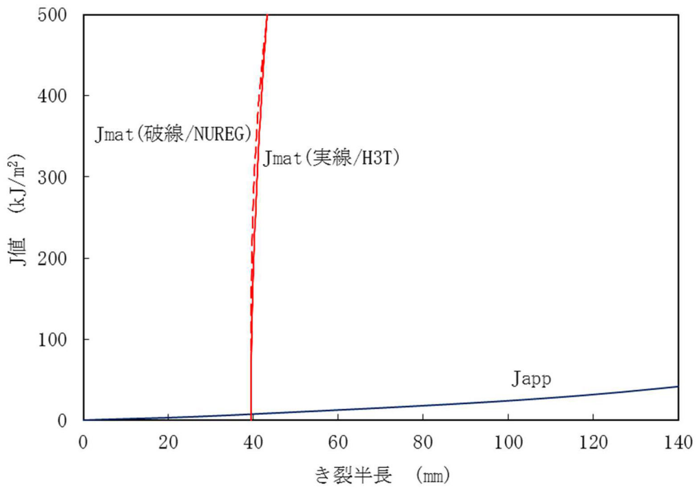
図4 クロスオーバーレグRCP側 90° エルボ
