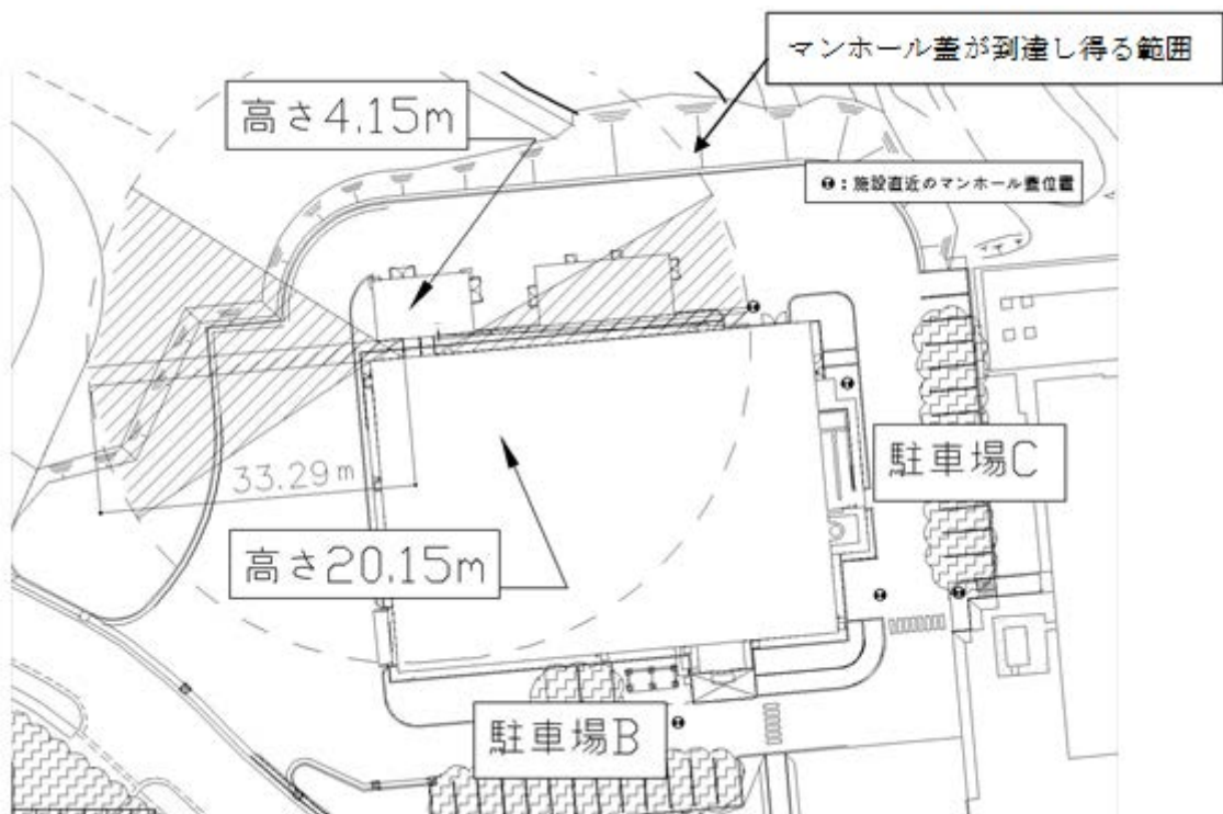
図-25 屋外のガス消火設備の配管類に到達し得る飛来範囲 ⑥【マンホール蓋】
