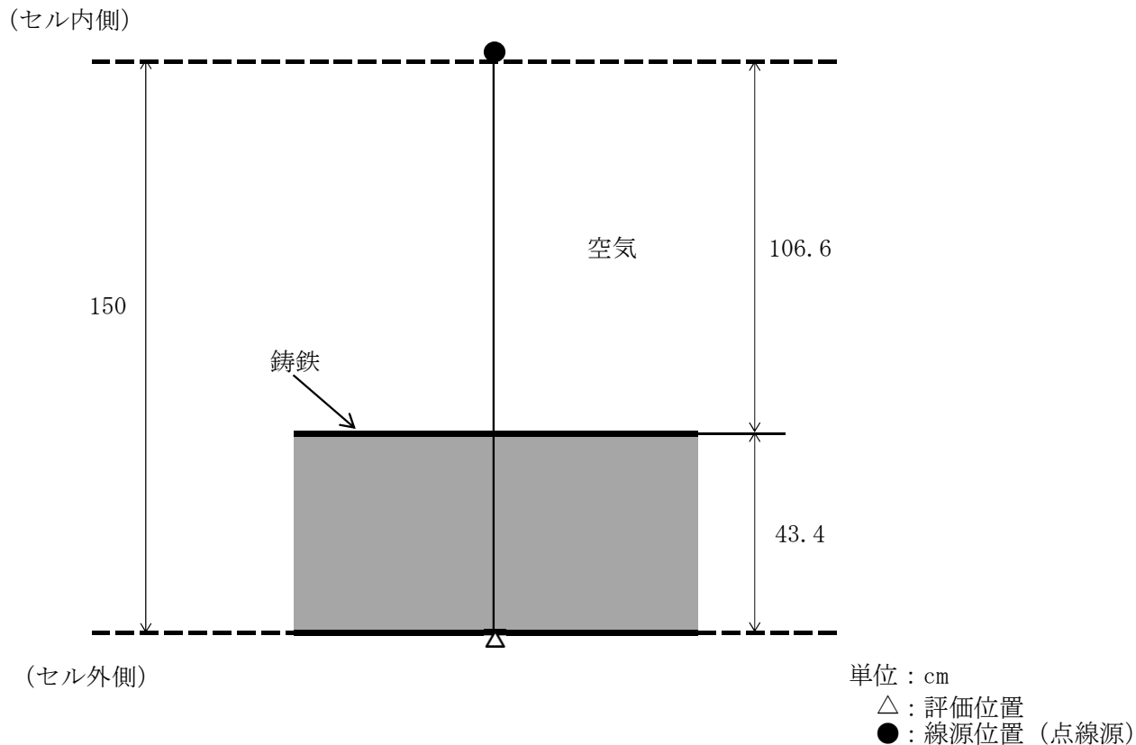
図-1 セル系排気設備の配管類 (埋設部) (210-302) の評価計算の体系モデル
