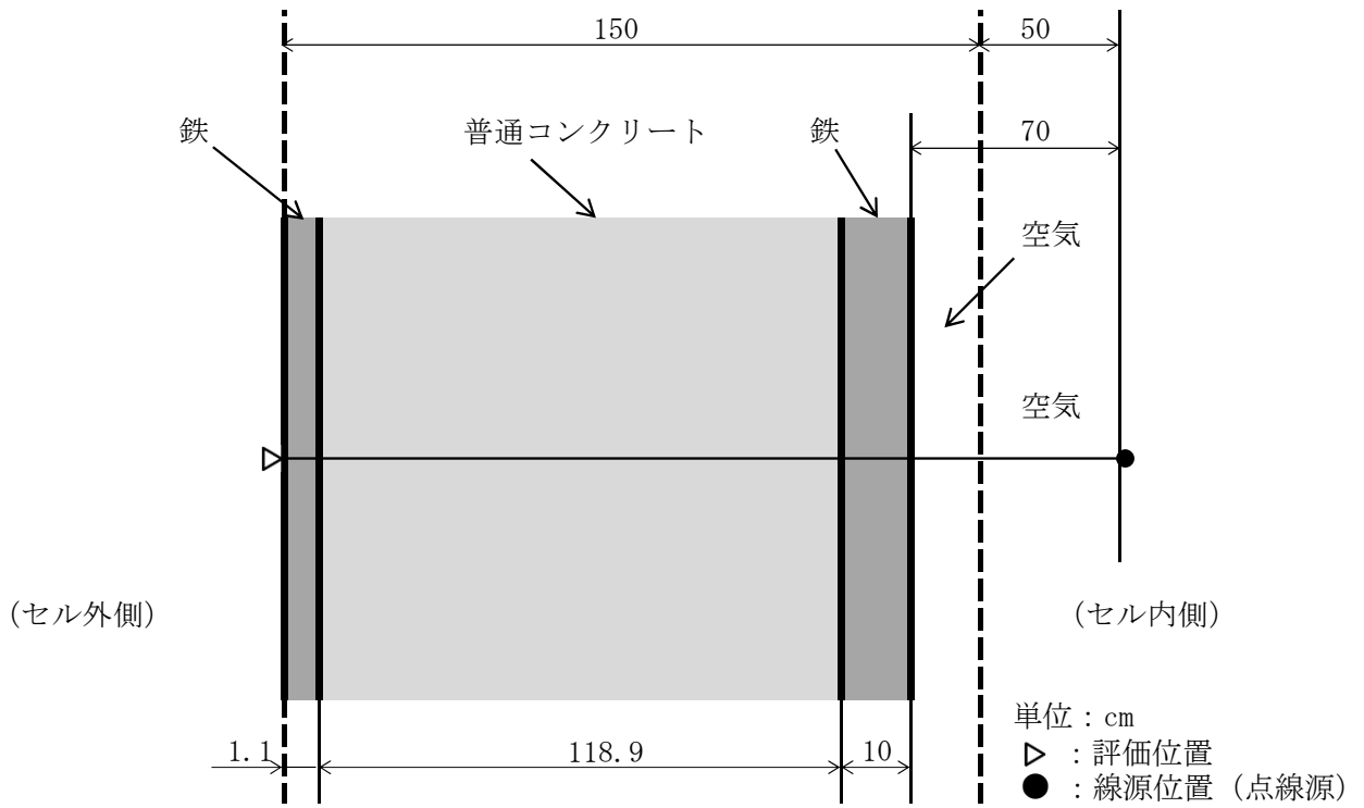
図-3 焼却熔融セルの遮蔽扉 (90-SD-005) の評価計算の体系モデル
