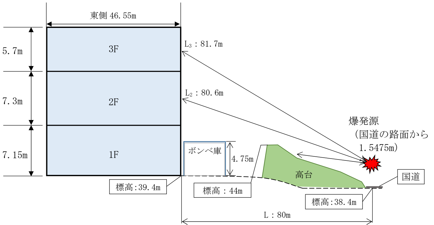
図-7 国道 51 号タンクローリの爆発における各階層の離隔距離
