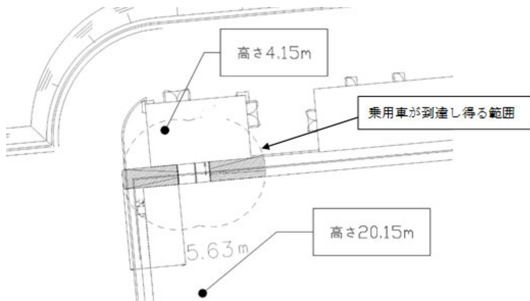
図-22 屋外のガス消火設備の配管類に到達し得る飛来範囲 ③ 【乗用車】
