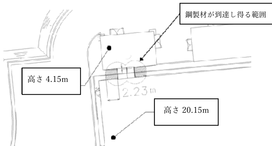
図-19 屋外のガス消火設備の配管類に到達し得る飛来範囲 ①【鋼製材】
