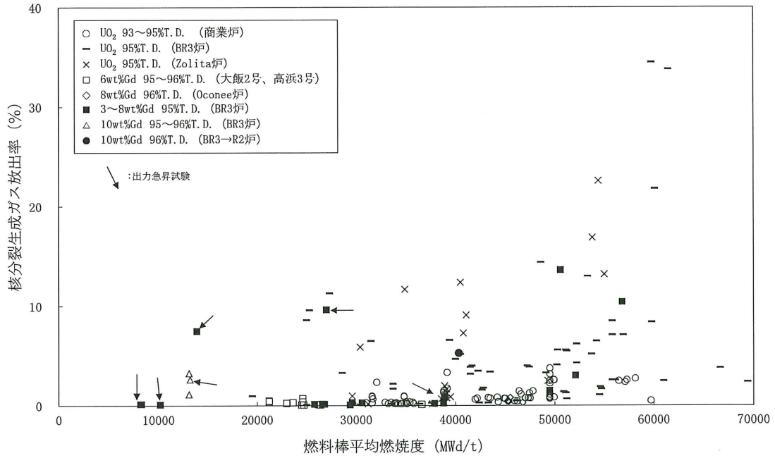
図 3-3 (1) 二酸化ウランペレット及びガドリニア混合二酸化ウランペレットの FP ガス放出率 (20)
