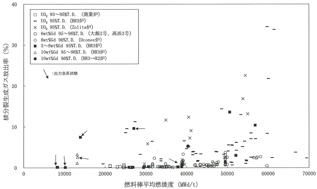
図 3-3 (1) 二酸化ウランペレット及びガドリニア混合二酸化ウランペレットの FP ガス放出率 (20)
