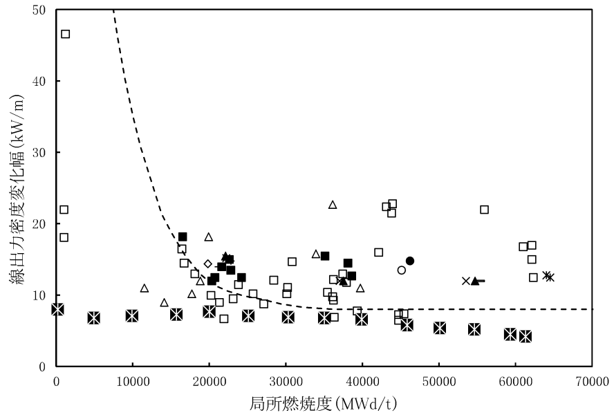
図 3-29 (1) 被覆管の出力ランプ試験結果 (最大線出力密度が最大の場合の出力変化)
