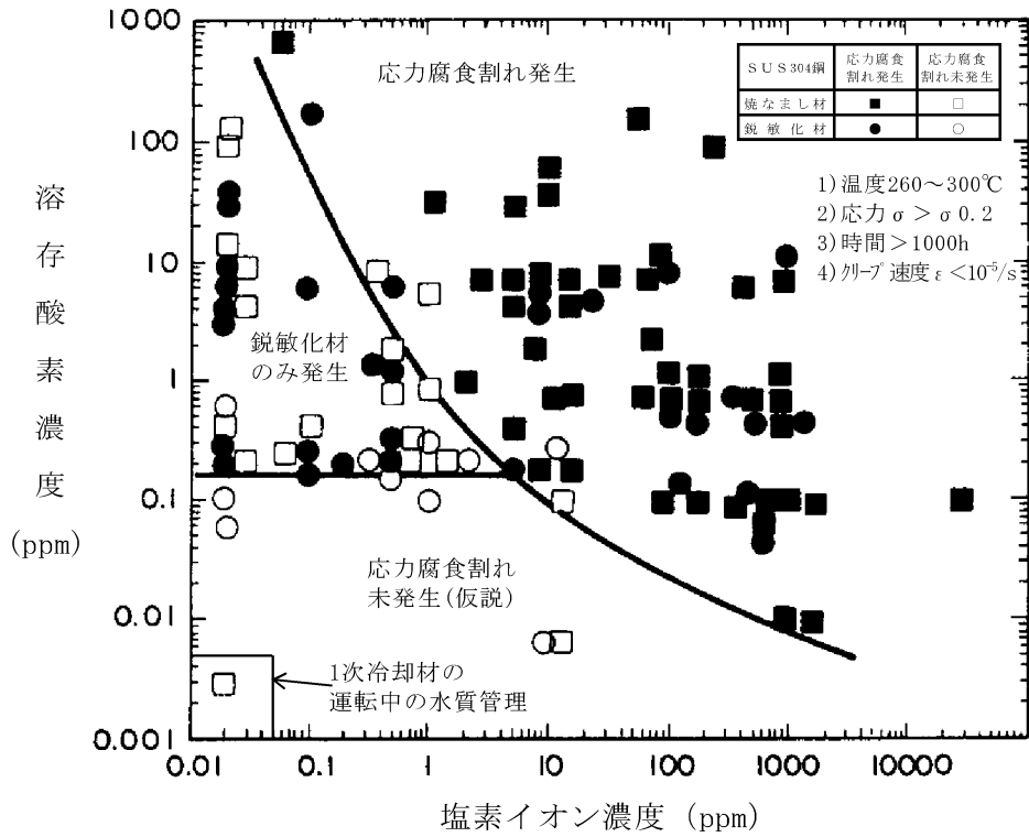
図 9-5 SUS304 鋼の応力腐食割れ発生におよぼす塩素イオン濃度及び溶解酸素濃度の限界量 (44)
