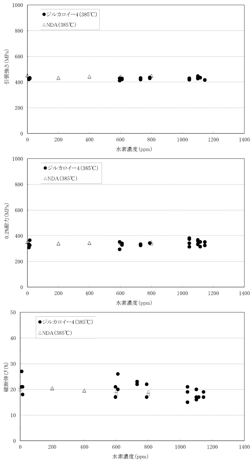
図 5-2 未照射 NDA 被覆管の機械特性と水素濃度の関係 (20)
