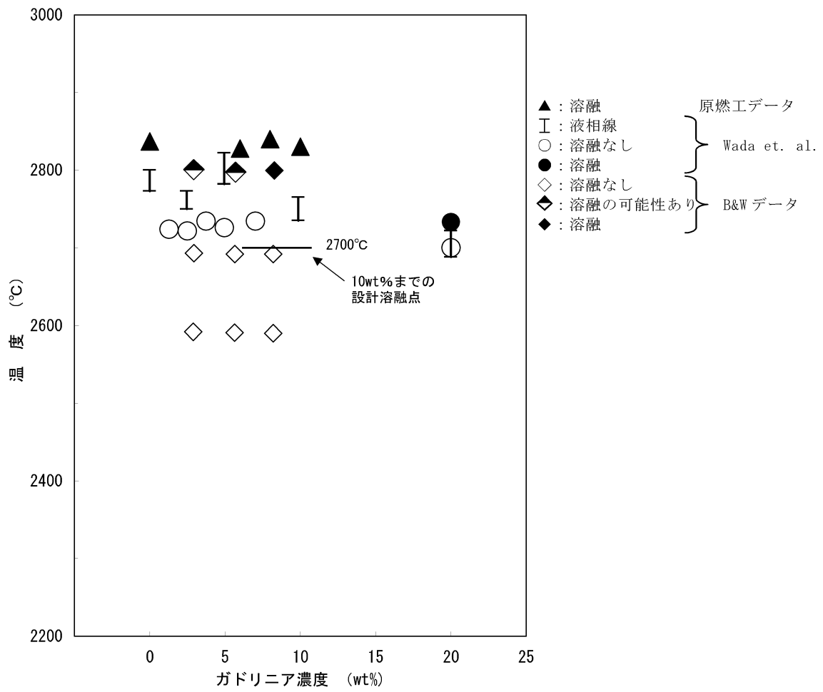
図 4-1 ガドリニア混合二酸化ウランペレットの溶融点 (20)
