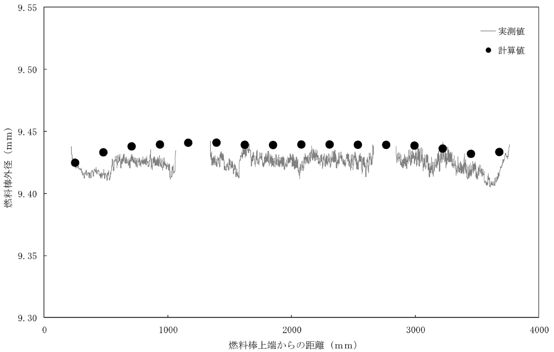
図 3-9 (2) 燃料棒外径の計算値と実測値との比較 (McGuire1 号機 ガドリニア混合燃料棒-NDA 被覆管)
