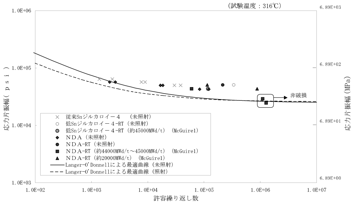
図 5-4 NDA 被覆管の疲労強度 (20)
