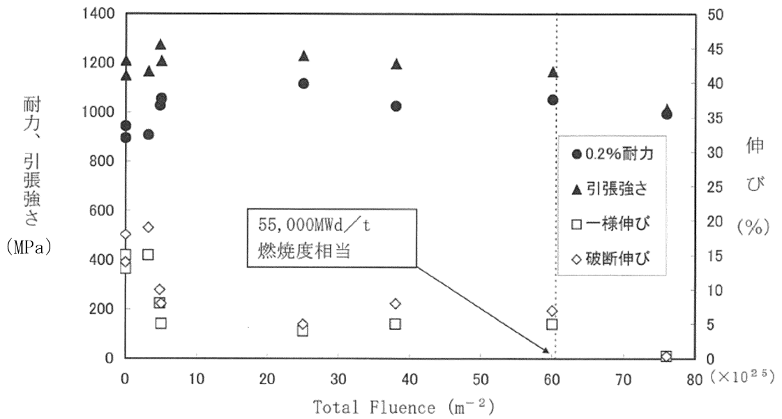
図 7-2 718 合金の照射による引張性質の変化 (35) (照射温度 400~430°C、試験温度 427°C)
