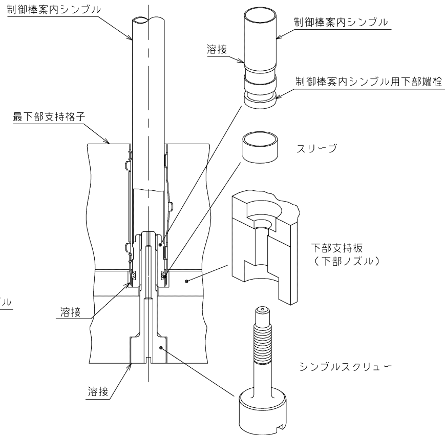
下部支持板(下部ノズル)との結合
