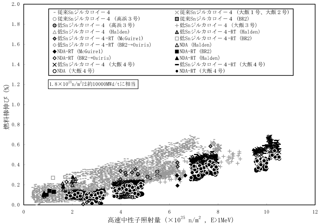
図 5-6 NDA 被覆管の照射成長 (20)
