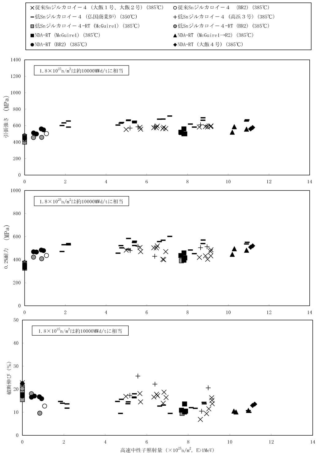
図 5-1 NDA 被覆管の機械特性 (20)
