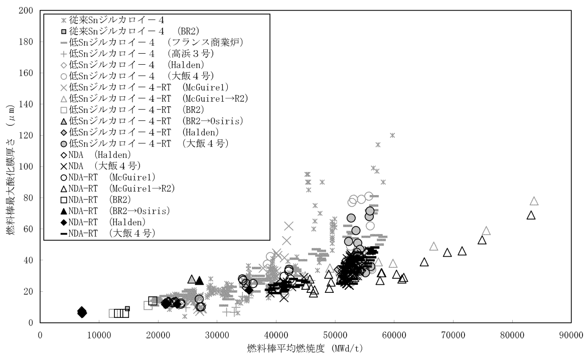
図 5-8 NDA 被覆管の炉内酸化膜厚さ (20)
