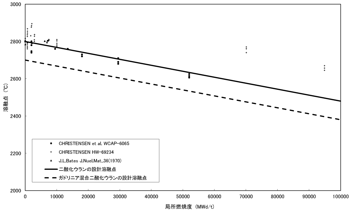
図 3-1 二酸化ウラン及びガドリニア混合二酸化ウランの溶融点 (17) (18) (19)
