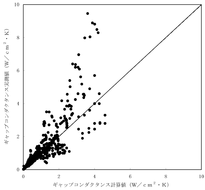
図 3-3 ギャップコンダクタンス式の実測値 (4) (15) (16) と計算値との比較
