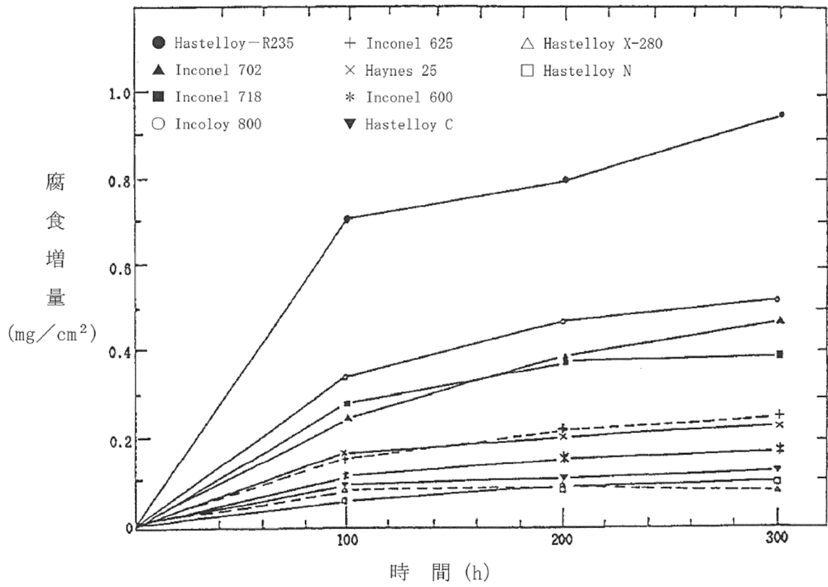
図 7-4 ニッケル基合金の腐食増量 (815°C) (37)
