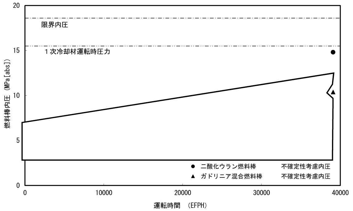
図 3-17 内圧評価上で最も厳しくなる燃料棒の内圧履歴（通常運転時）
