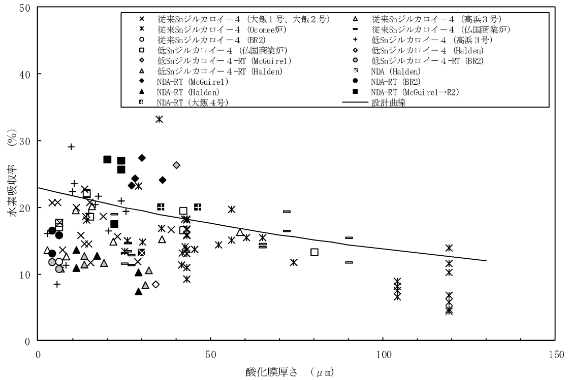
図 5-10 NDA 被覆管の酸化膜厚さと水素吸収率の関係 (20)
