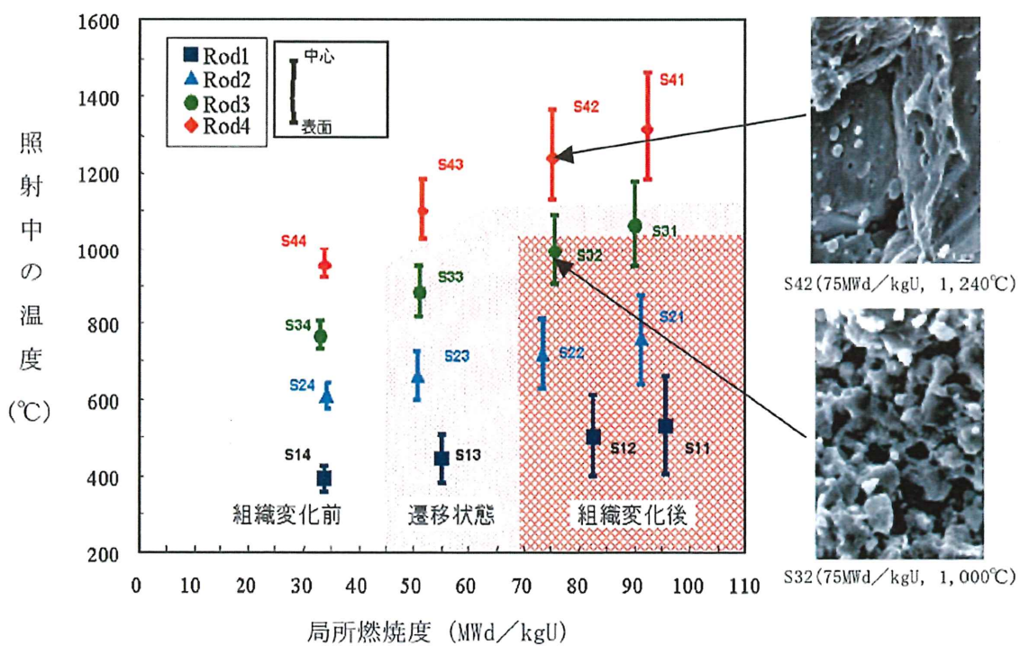
図 3-5 リム組織形成のための温度及び燃焼度
