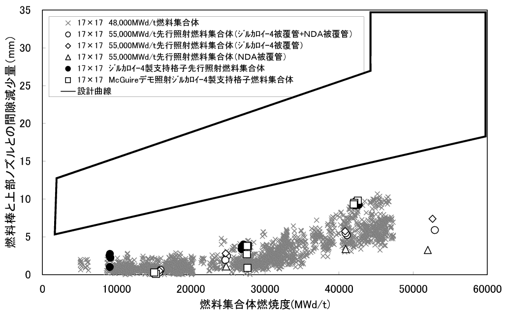
図 3-26 (2) トータルギャップ減少量 (35)
