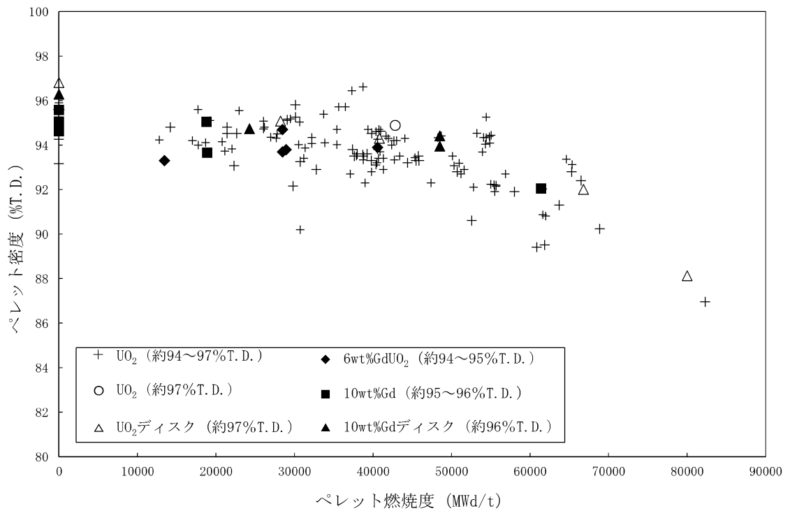
図 3-2 ペレット密度の燃焼に伴う変化 (20)
