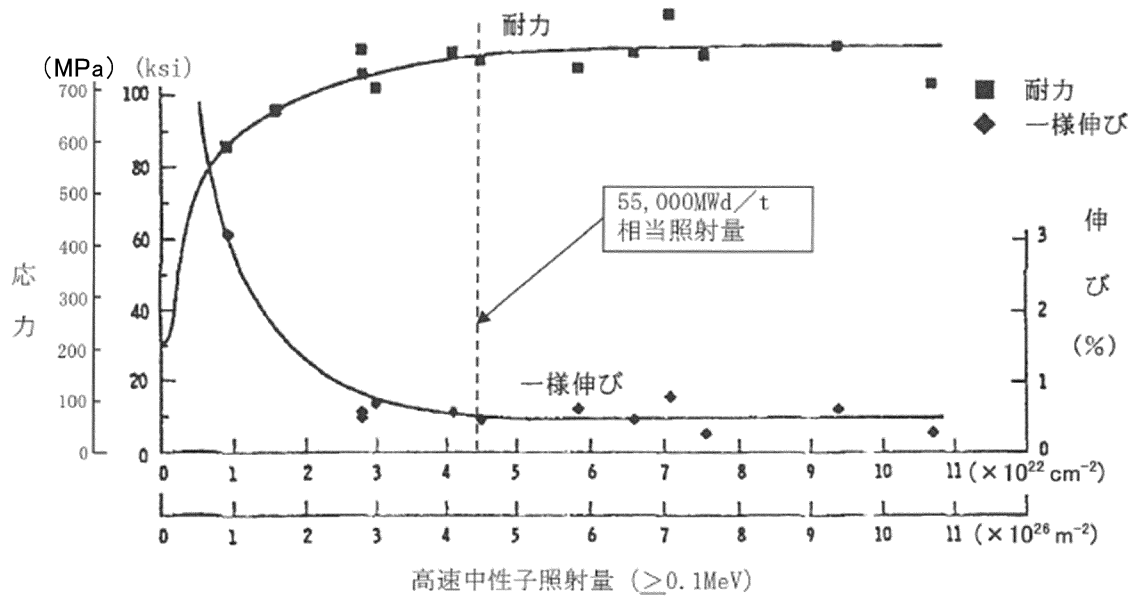
図 9-1 SUS304 鋼の照射による機械的性質の変化 (41) (照射温度 370°C、試験温度 370°C)
