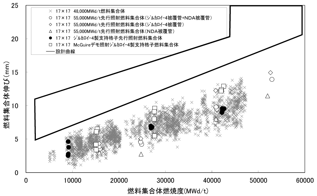
図 3-25 (2) 燃料集合体伸び (35)
