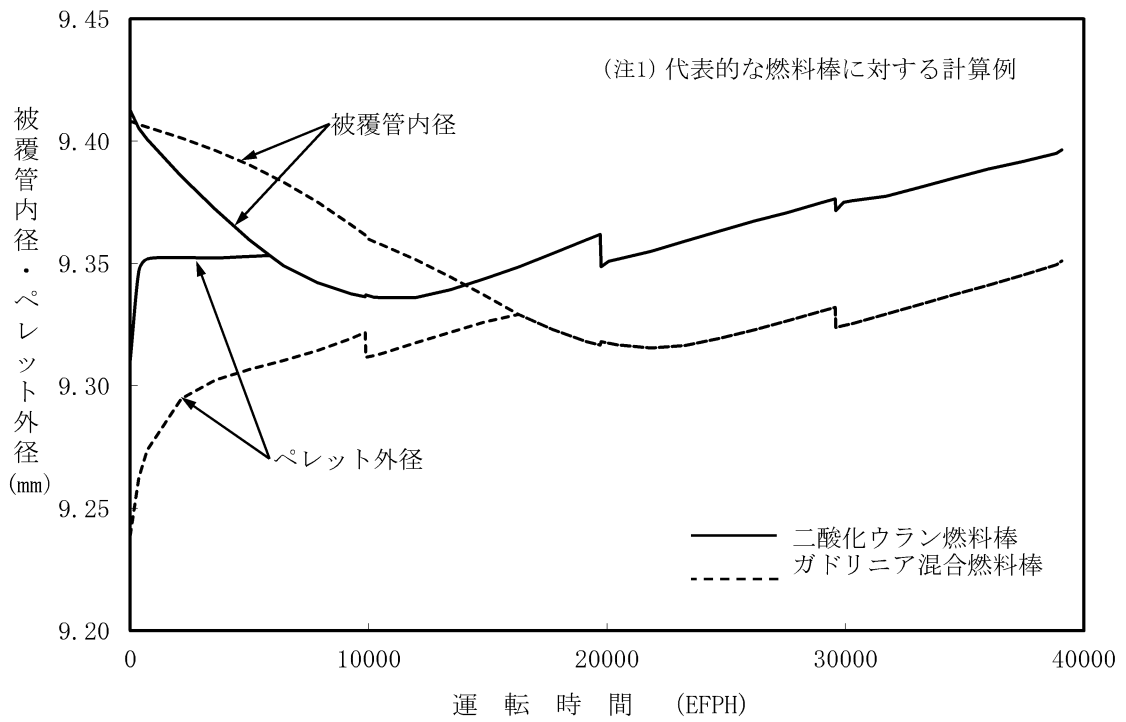
図 3-18 被覆管内径及びペレット外径変化
