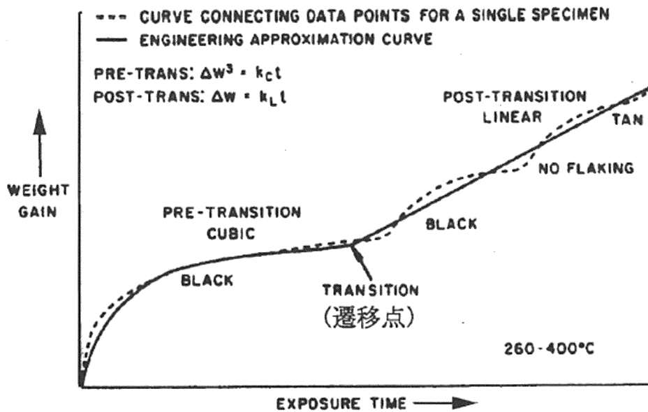
図 5-7 炉外腐食試験におけるジルカロイ-2 とジルカロイ-4 の典型的な腐食増量曲線 (30)
