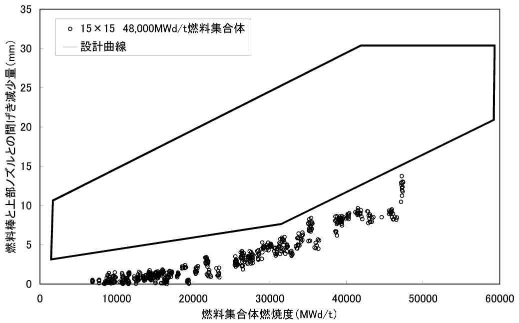
図 3-26 (1) トータルギャップ減少量 (34)
