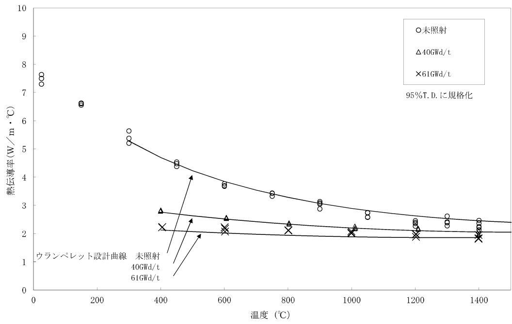
図 3-6 照射後二酸化ウランペレットの熱伝導率 (18) (20) (21)
