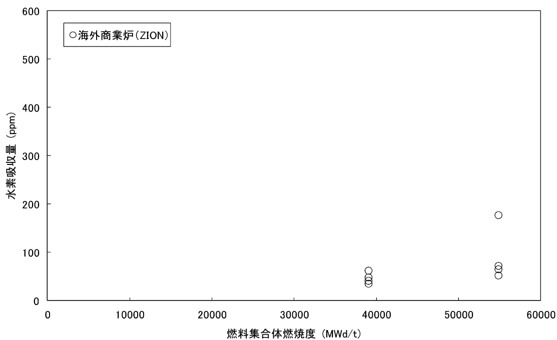
図 6-3 実機で照射された案内シンプルの水素吸収量データ (32)
