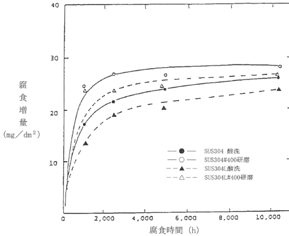
図 9-3 SUS304 鋼の高温水中腐食 (試験温度 300°C) (43)
