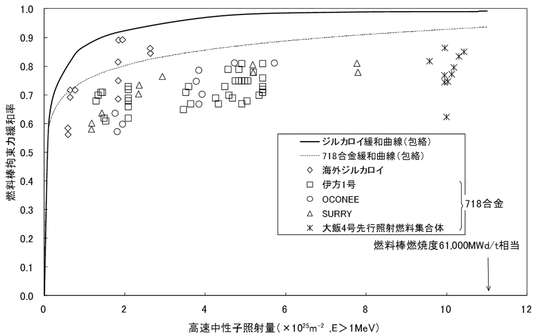
図 3-30 支持格子拘束力の緩和率実測データ (31) (32)
