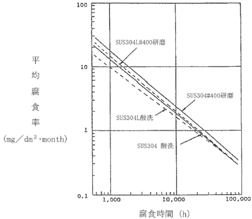
図 9-4 SUS304 鋼の溶存酸素を含まない 300°C の 0.92% ホウ酸水中における平均腐食率 (43)
