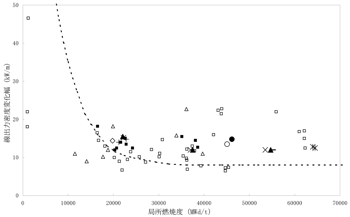
図 5-11 NDA 被覆管の耐 PCI 性 (20)
