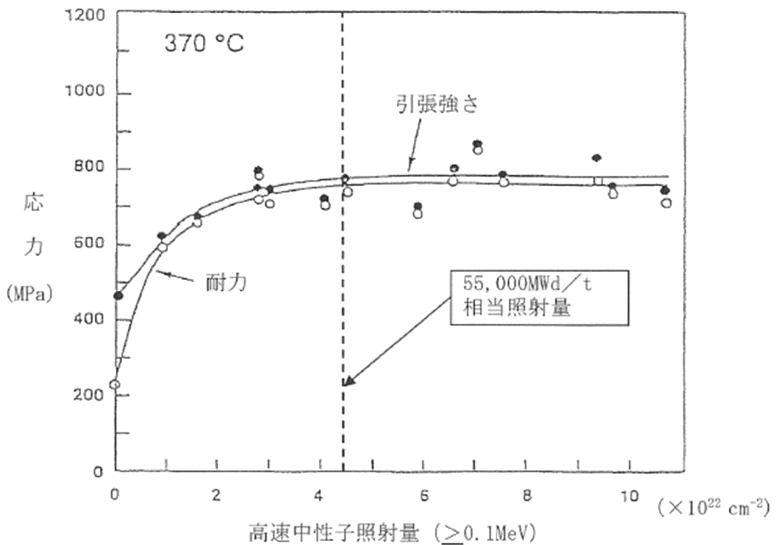
図 9-2 SUS304 鋼の照射による機械的性質の変化 (41) (照射温度 370°C、試験温度 370°C)
