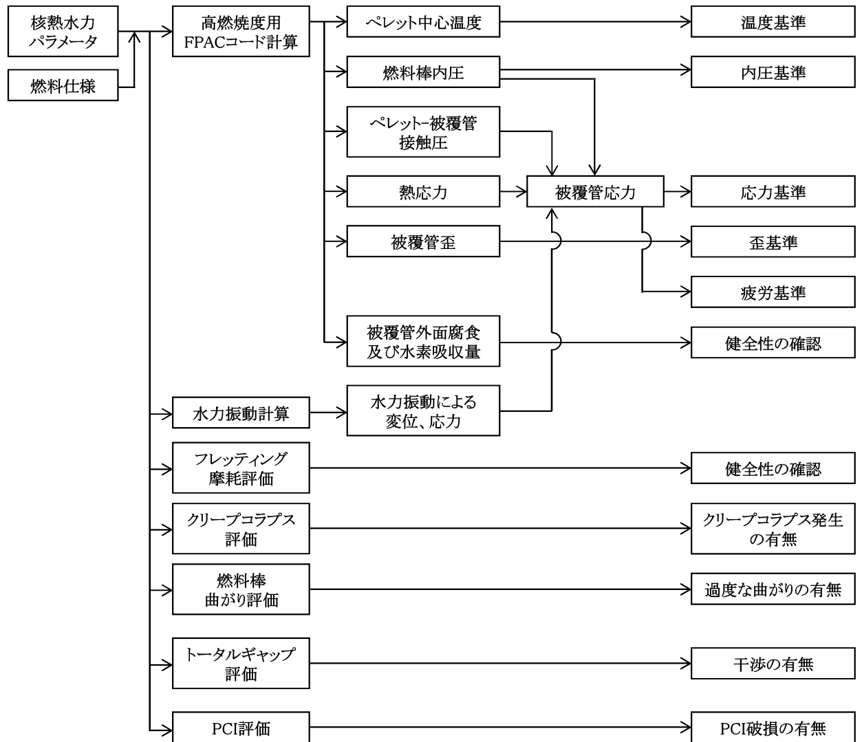
図 3-1 燃料棒強度評価流れ図
