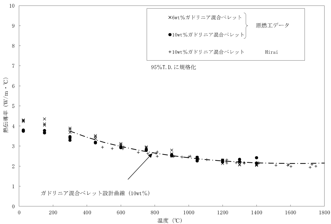
図 3-5 ガドリニア混合二酸化ウランペレットの熱伝導率 (未照射) (18) (19)
