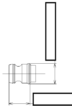
上部端栓詳細
