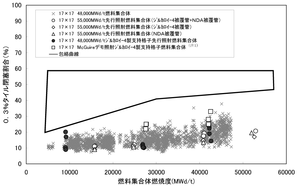
図 3-24 (1) 燃料棒間隔の閉塞割合 (34)
