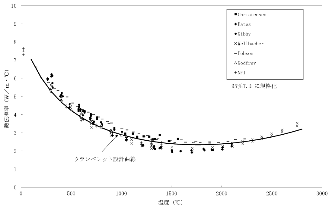
図 3-4 二酸化ウランペレットの熱伝導率 (未照射) (17) (18)
