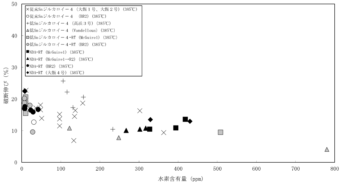
図 5-3 被覆管水素濃度と破断伸びの関係 (9) (20)
