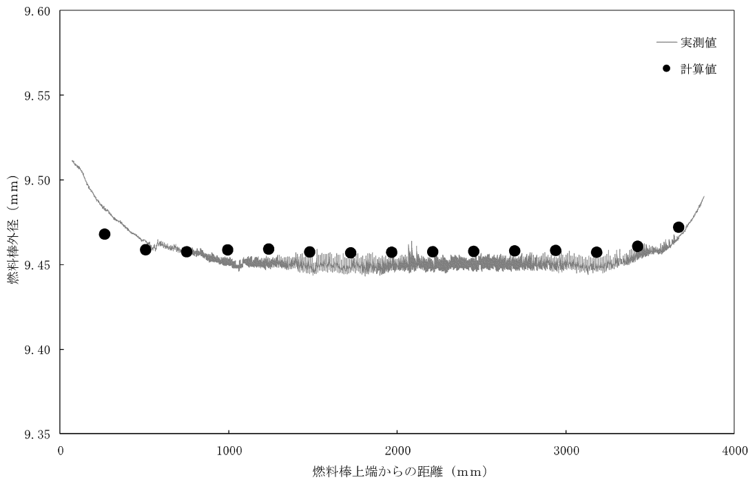
図 3-9 (1) 燃料棒外径の計算値と実測値との比較 (高浜 3 号機 二酸化ウラン燃料棒-低 Sn ジルカロイ-4 被覆管)
