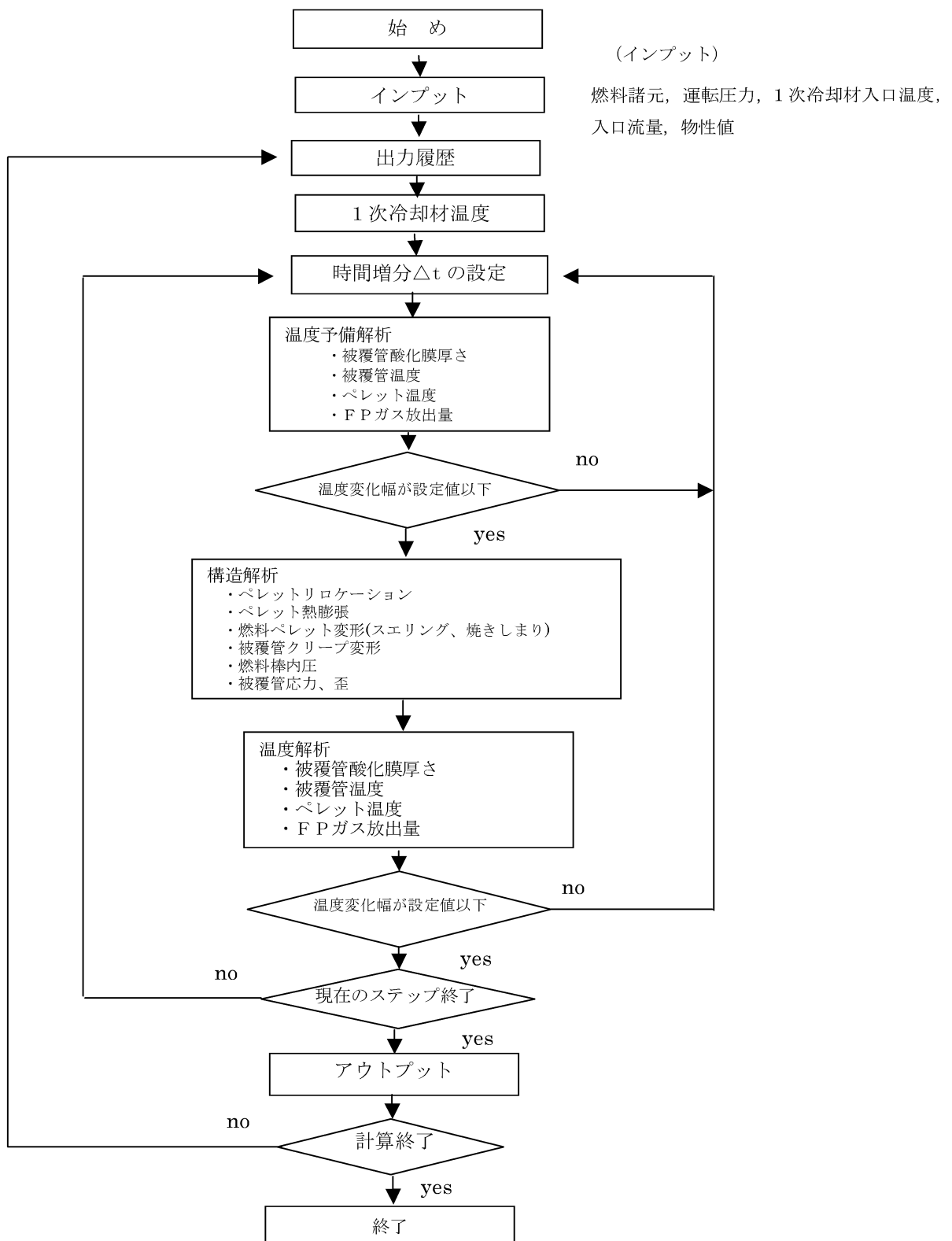
図 3-2 高燃焼度用 FPAC コードの流れ図
