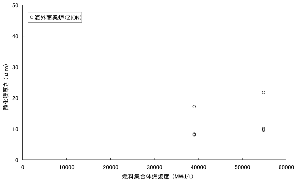
図 6-2 実機で照射された案内シンプルの腐食データ (32)
