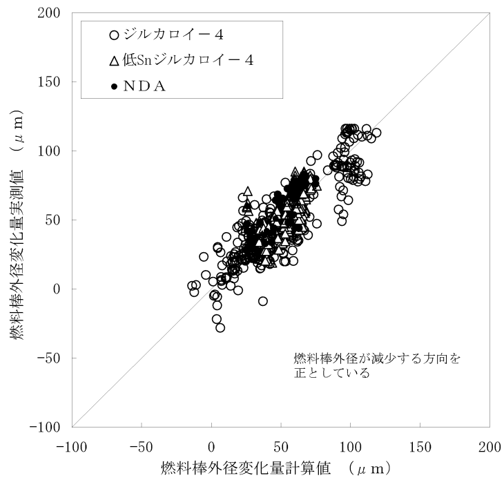
図 3-9 (3) 燃料棒外径の計算値と実測値との比較
