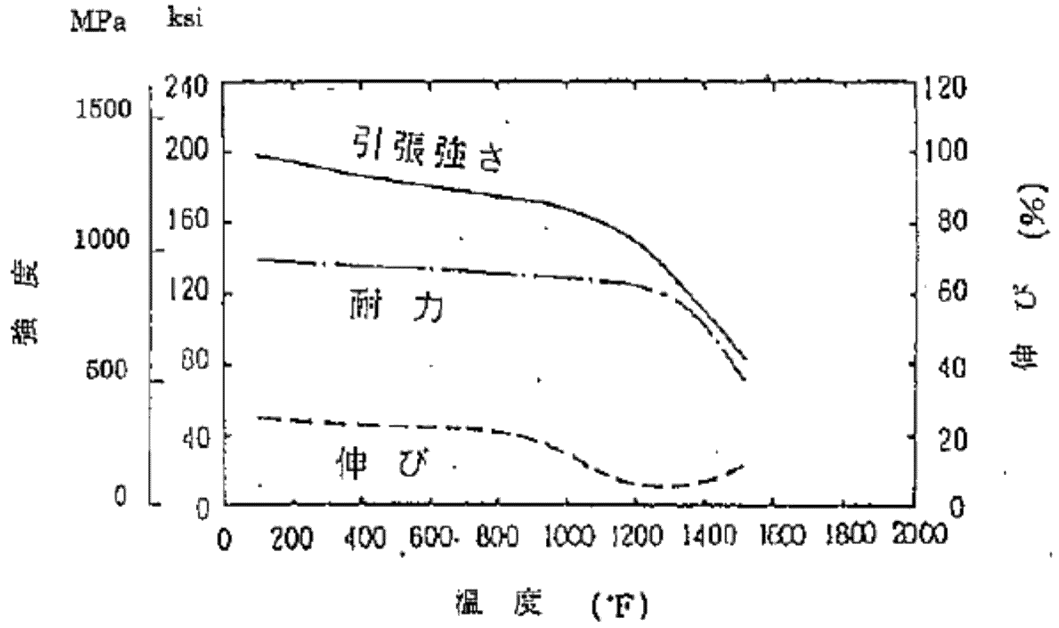
図 7-1 [ ] の温度による機械的性質の変化 (34)
