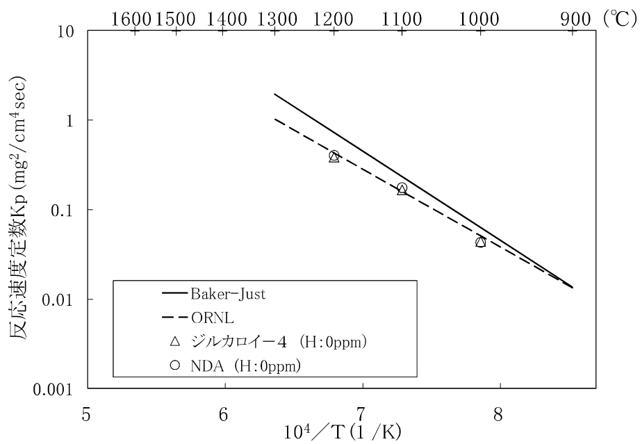
図 5-13 未照射管のジルコニウム-水反応速度定数 (受取管) (20)
