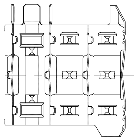
断面A-A
