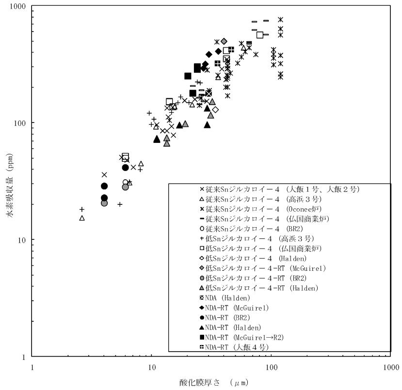
図 5-9 NDA 被覆管の炉内酸化膜厚さと水素吸収量の関係 (20)
