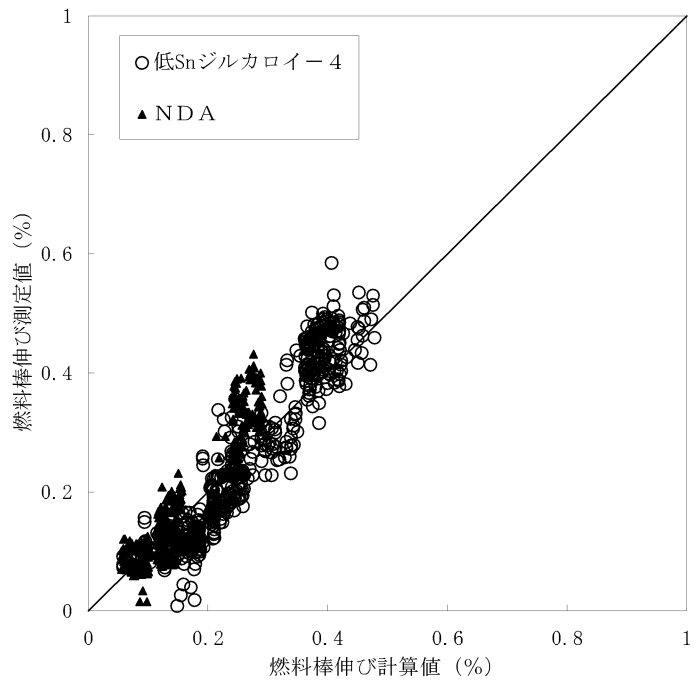
図 3-13 燃料棒の伸びの計算値と実測値との比較
