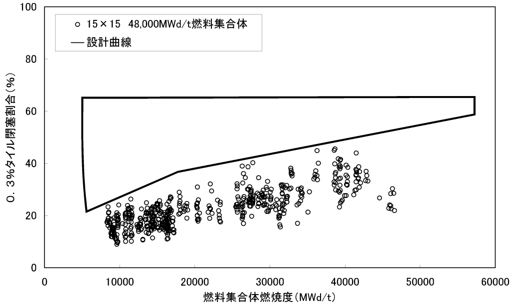
図 3-24 (1) 燃料棒間隔の閉塞割合 (34)
