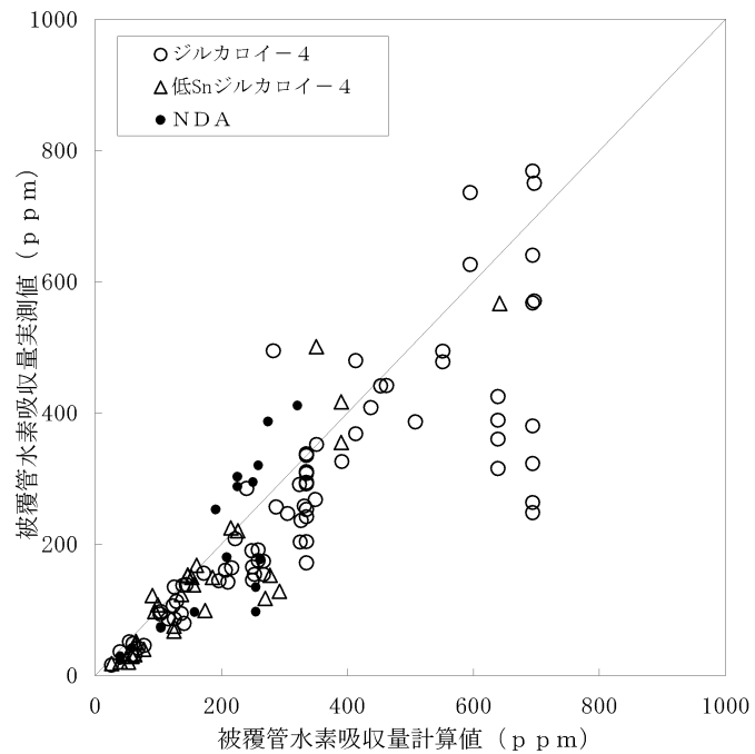
図 3-28 被覆管水素吸収量の実測値と予測値の比較
