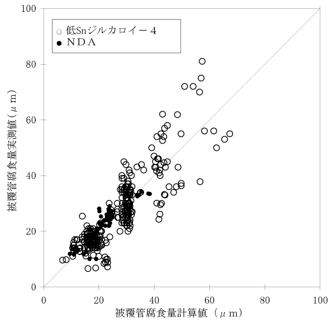
図 3-27 被覆管腐食量（最大酸化膜厚）の実測値と予測値の比較
