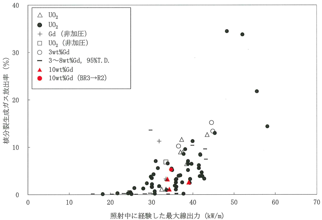
図 3-3 (2) 二酸化ウランペレット及びガドリニア混合二酸化ウランペレットの FP ガス放出率と線出力密度の関係 (20)
