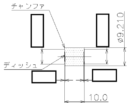
ペレット詳細
