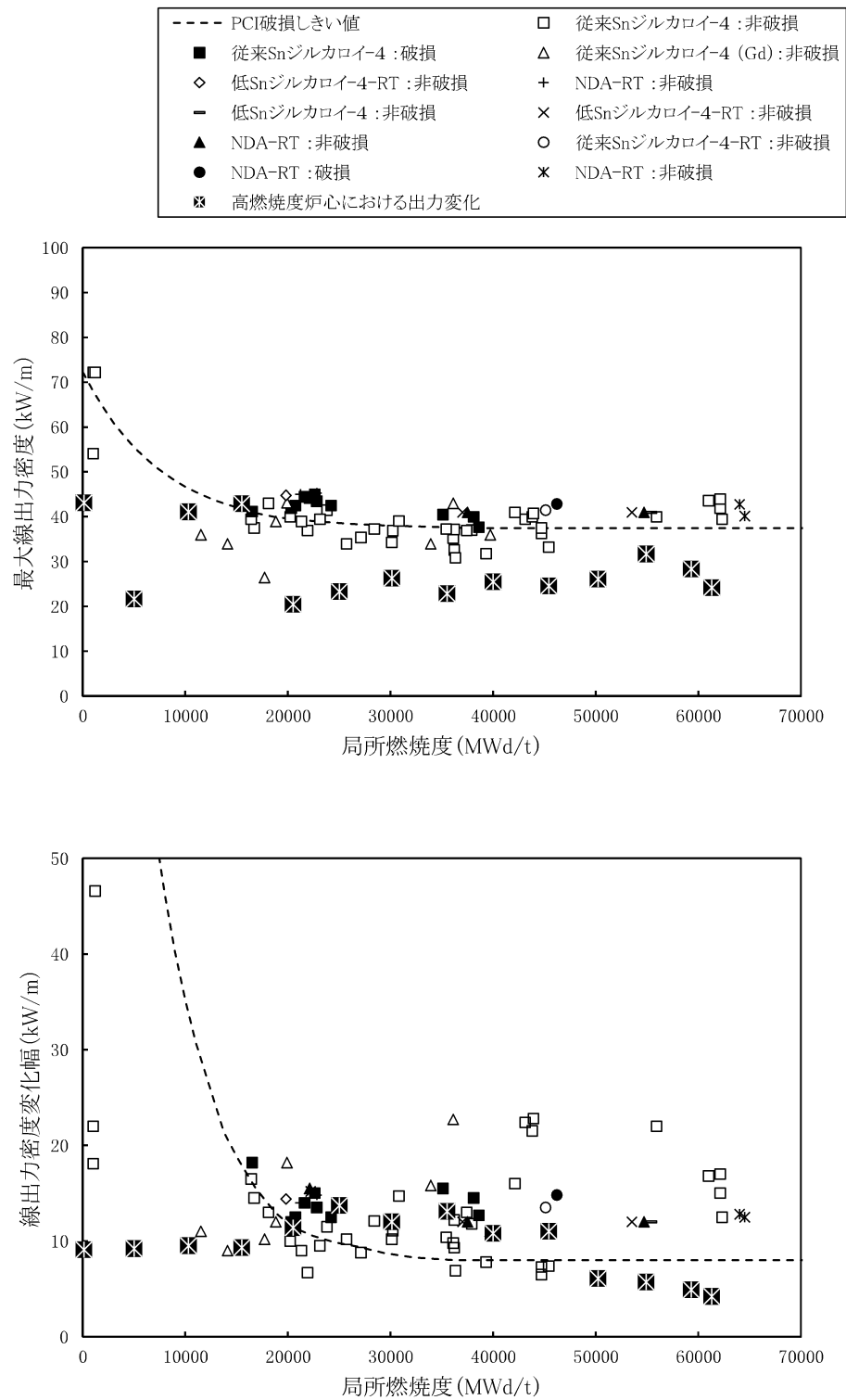
図 3-29 (2) 被覆管の出力ランプ試験結果 (線出力密度変化幅が最大の場合の出力変化)
