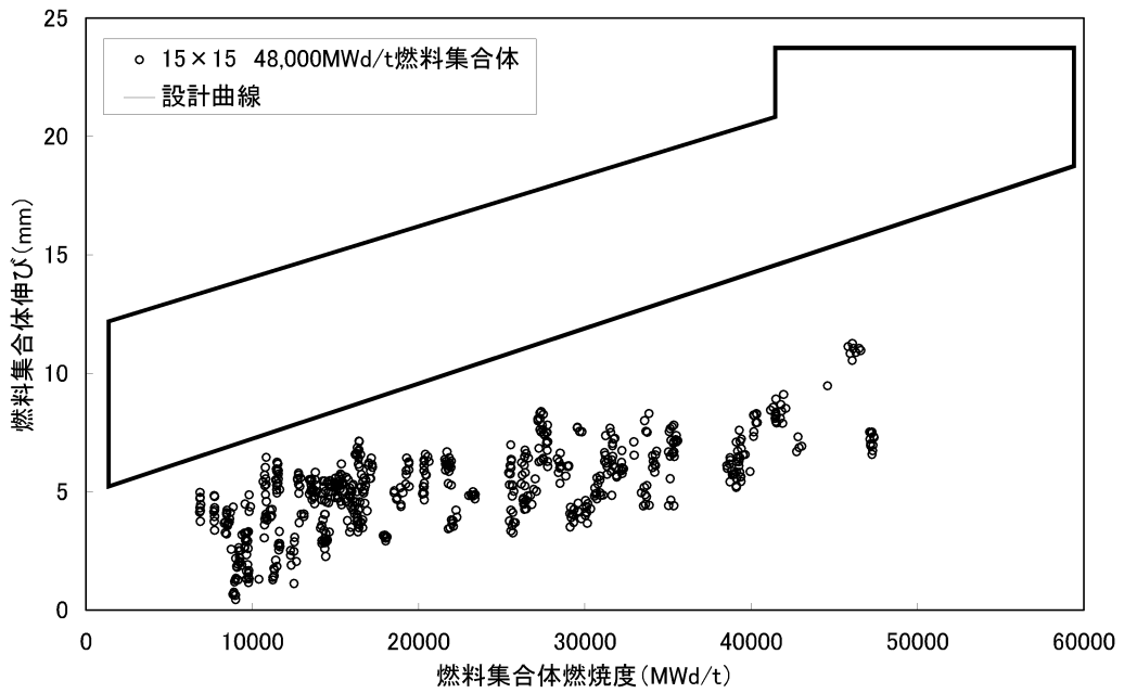
図 3-25 (1) 燃料集合体伸び (34)
