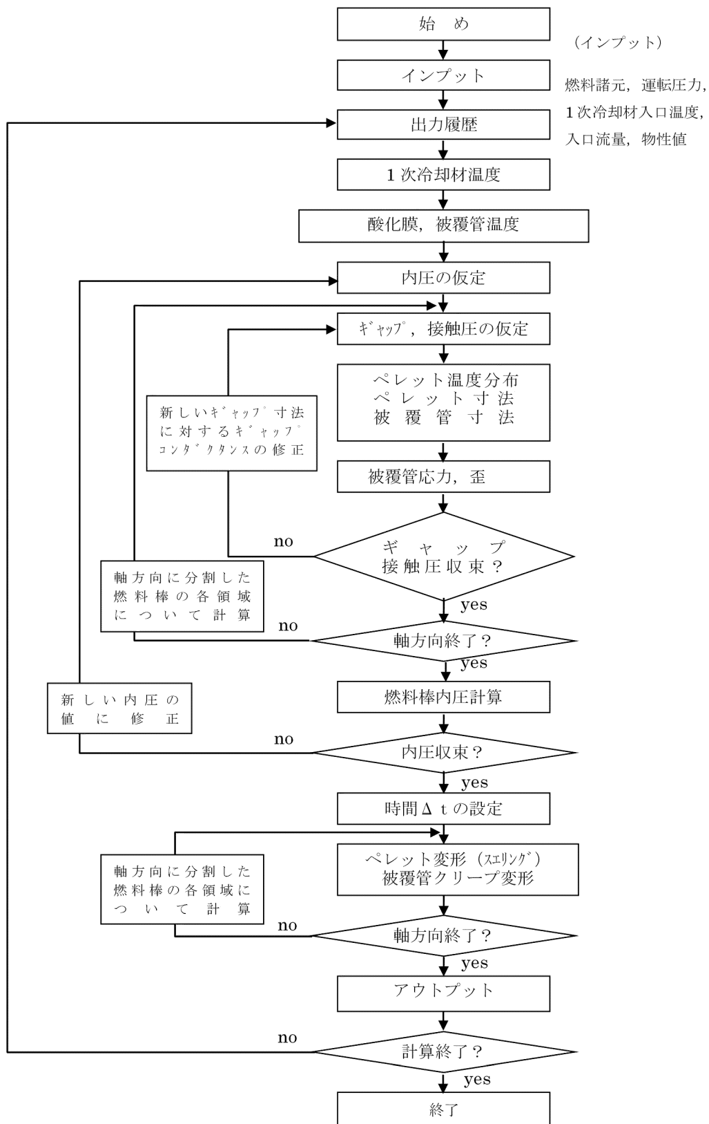
図 3-2 FPAC コードの流れ図
