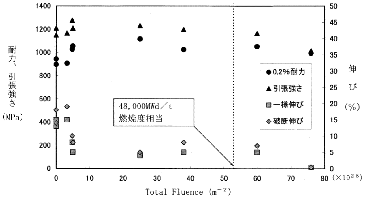
図 6-2 718 合金の照射による引張性質の変化 (33)
