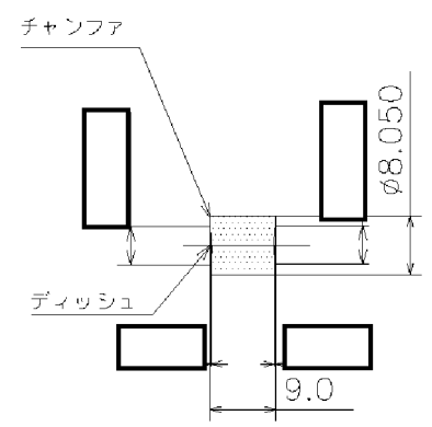
ペレット詳細
