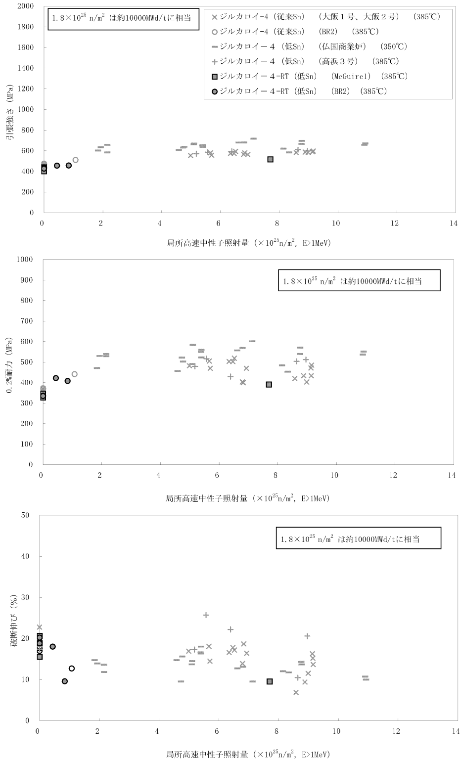
図 5-1 ジルカローイ-4 被覆管の機械特性 (23)
